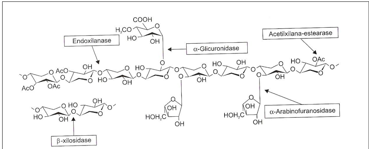
Figura 4 - Enzimas xilanolíticas envolvidas na degradação da xilana.
