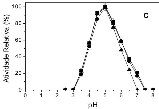
Figura 1 - Efeito do pH sobre as atividades de (A) endoglucanase (B) FPase (C) celobiase presentes nos extratos (■) C011 (●) C012 (▲) C013.
