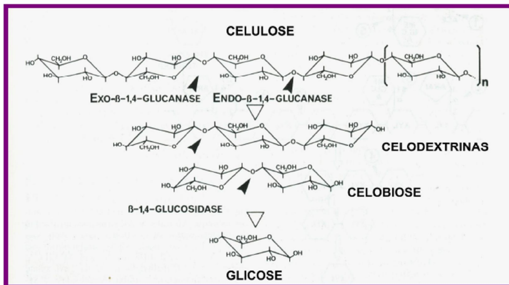
Figura 3 - Ação do complexo celulase na hidrólise da celulose e compostos intermediários.
