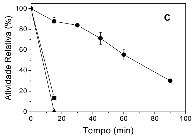
Figura 3 – Estabilidade térmica de endoglicanase nas temperaturas de (A) 40°C (B) 45°C (C) 50°C presentes nos extratos (■) C011 (●) C012 (▲) C013.
