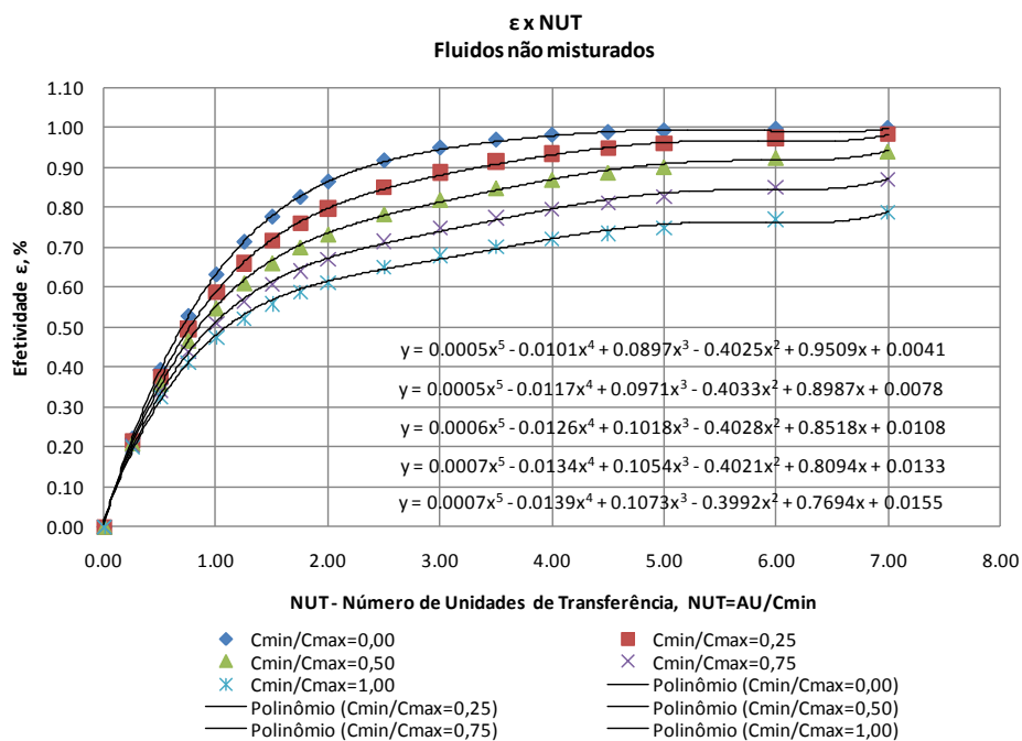
Figura 20 – Gráfico que relaciona a efetividade de transferência de calor ( \epsilon ) com o número de unidades de transferência (NUT) e a razão entre as taxas de capacidade calorífica ( \text{C}_{\text{min}}/\text{C}_{\text{max}} ), reproduzido conforme o trabalho de Kays e London (1984).
