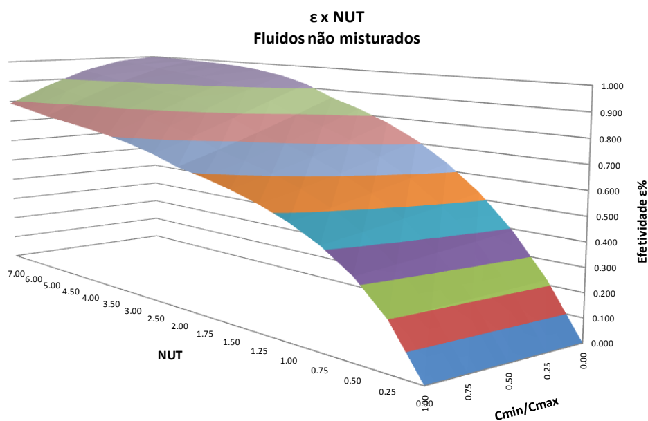
Figura 21 – Superfície que relaciona a efetividade de transferência de calor ( \epsilon ) com o número de unidades de transferência (NUT) e a razão entre as taxas de capacidade calorífica ( \text{C}_{\text{min}}/\text{C}_{\text{max}} ).
