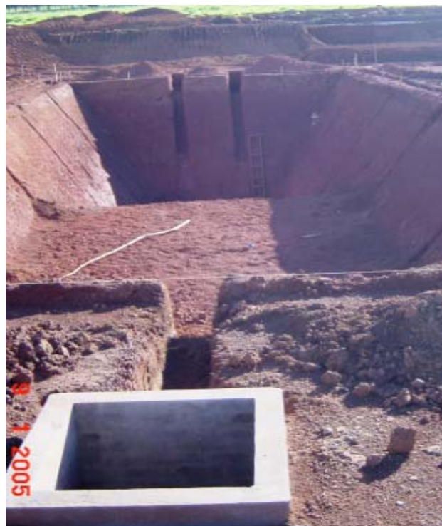
FIGURA 3.4 – Abertura de valas para tubulações.
