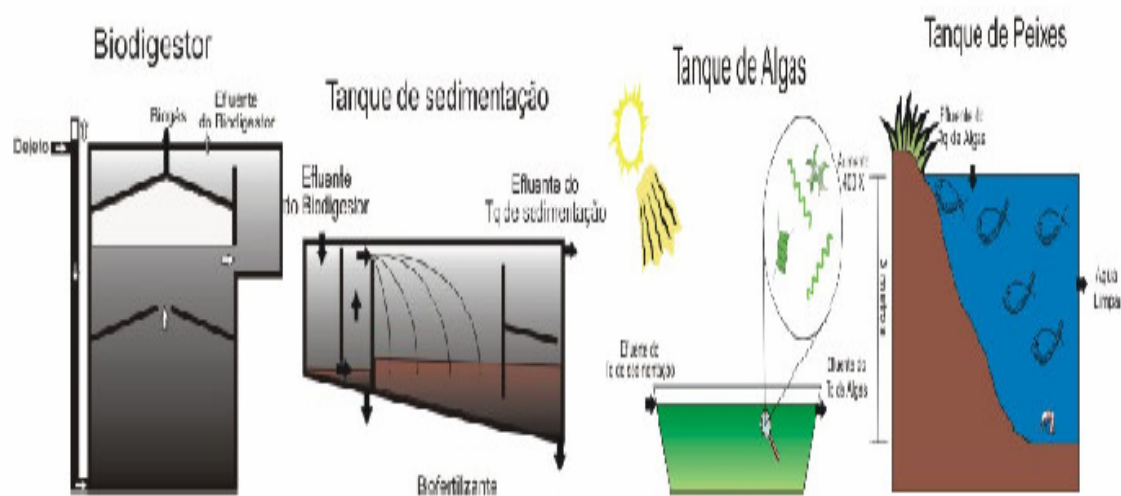
FIGURA 2.3 – Exemplo de um biosistema integrado.
