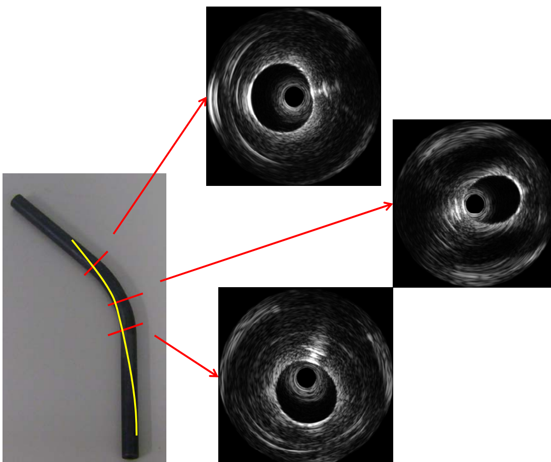
Figura C-6. Alguns cortes longitudinais durante o caminho do cateter para tubo com uma curva. Em amarelo está nossa suposição do caminho do cateter dentro do tubo com uma curva.
