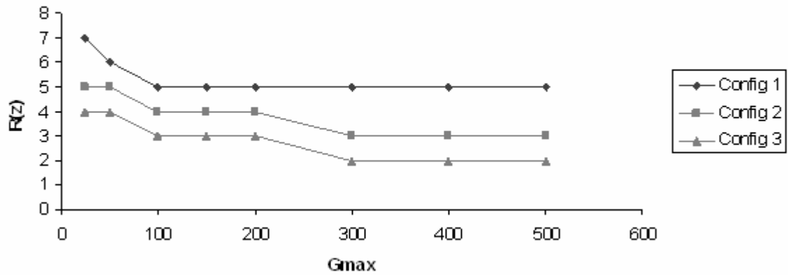
Figura 132 – Comparação de índices R(z) entre configurações para caso II.
