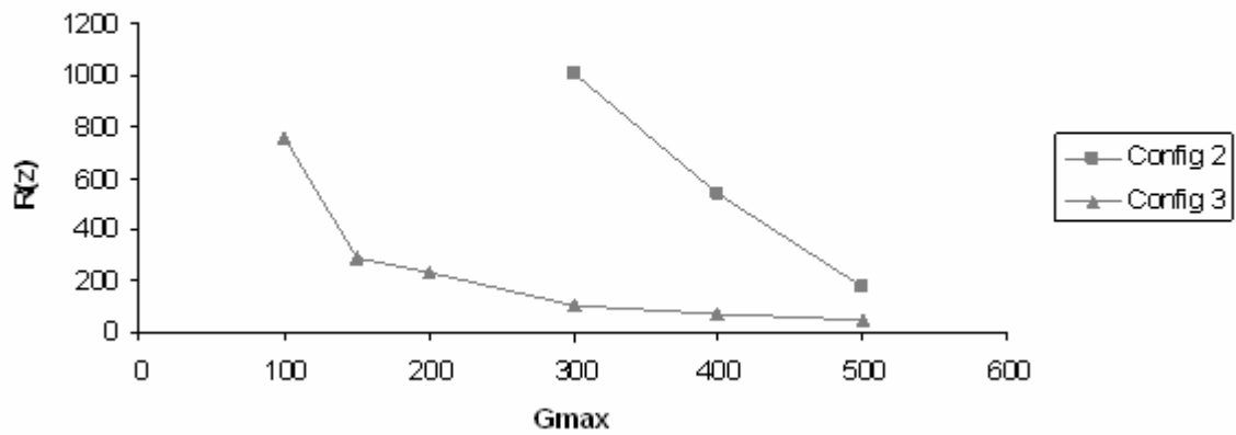
Figura 133 – Comparação de índices R(z) entre configurações para caso III.
