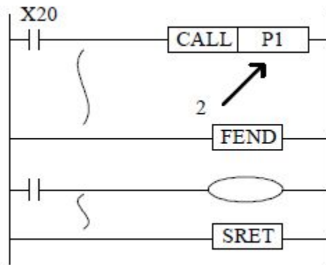
Figura 29 – Comando CALL
