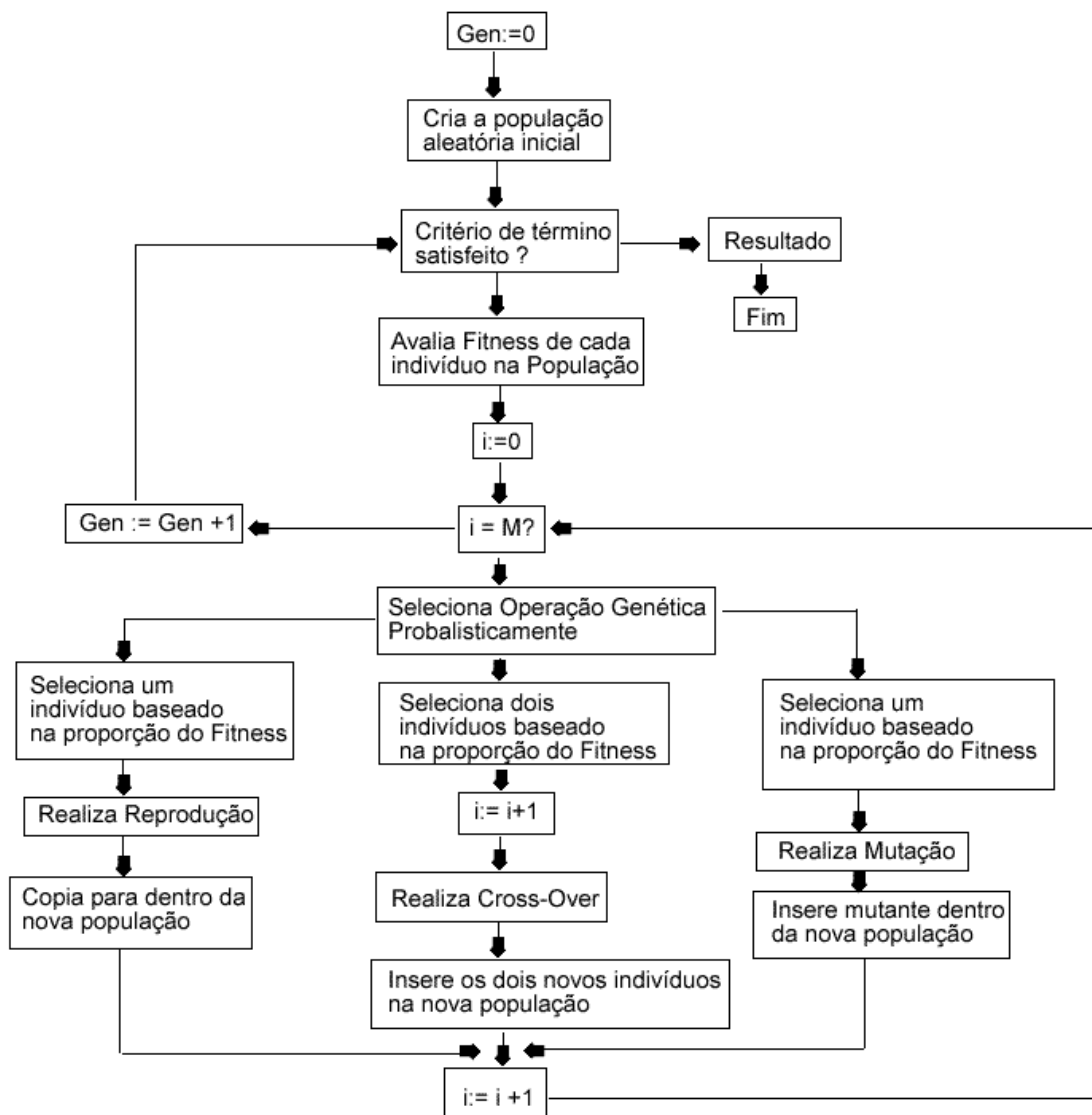
Figura 32 – Fluxograma do programa com seleção proporcional
