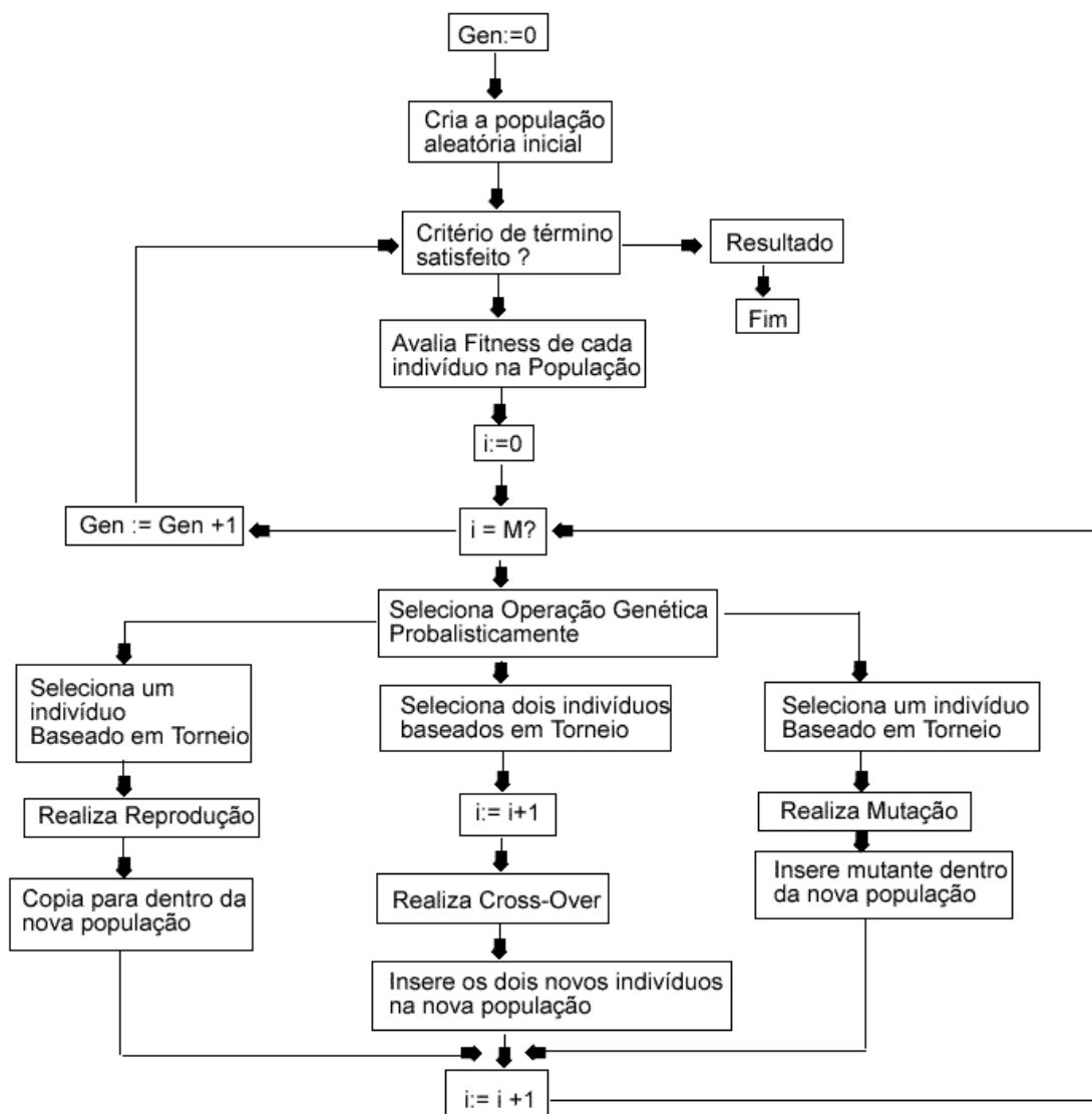
Figura 33 – Fluxograma do programa com seleção por Torneio
