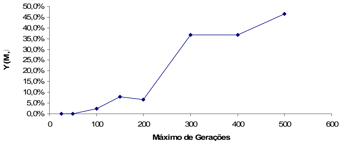
Figura 106 – Probabilidade de sucesso Y(M,i) por número máximo de gerações para cross-over 10% e mutação 80% – Partida direta de motor com reversão.
