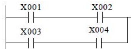
Figura 16 – Comando ORB
