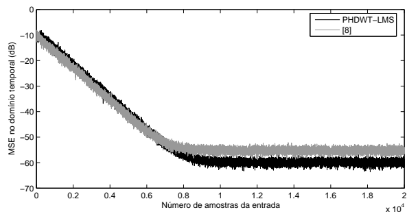
Figura B.97: MSE por amostra da entrada.
