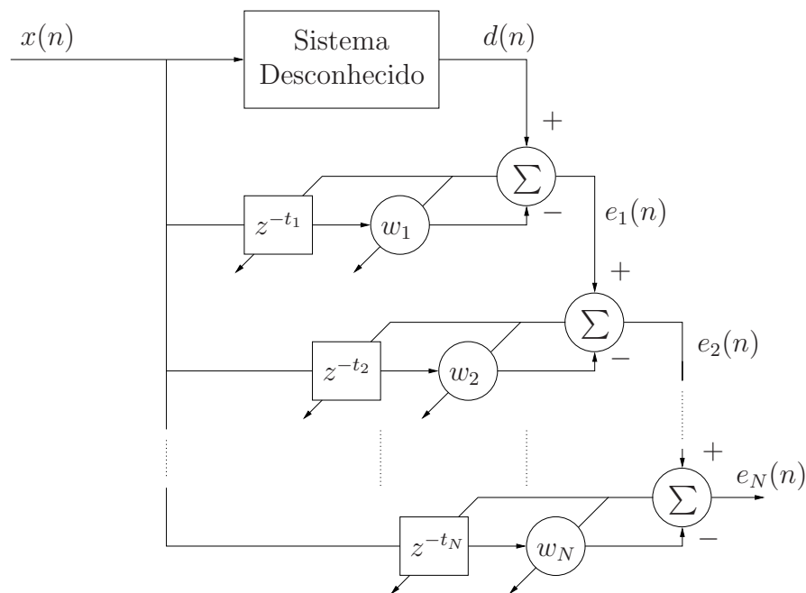
Figura 2.2: ADF modificado para o esquema seqüencial.
