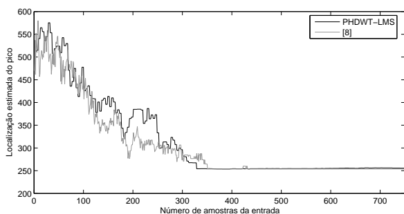
Figura B.140: LEP por amostra da entrada.
