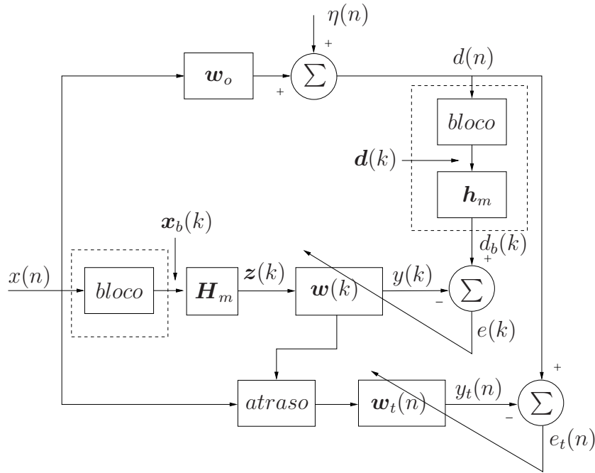
Figura 3.5: Diagrama de blocos da solução proposta.
