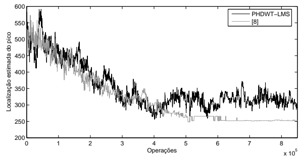
Figura B.159: LEP por operações.
