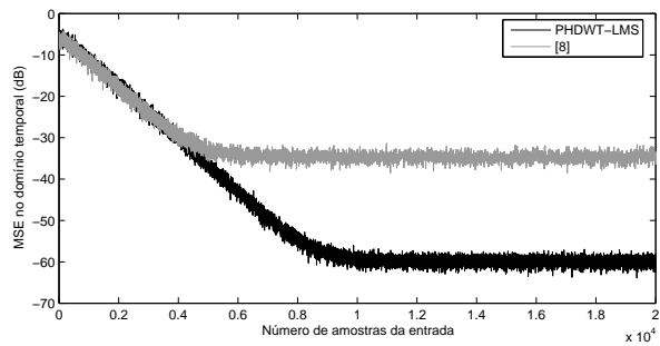
Figura B.34: MSE por amostra da entrada.
