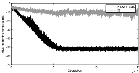
Figura B.71: MSE por operações.
