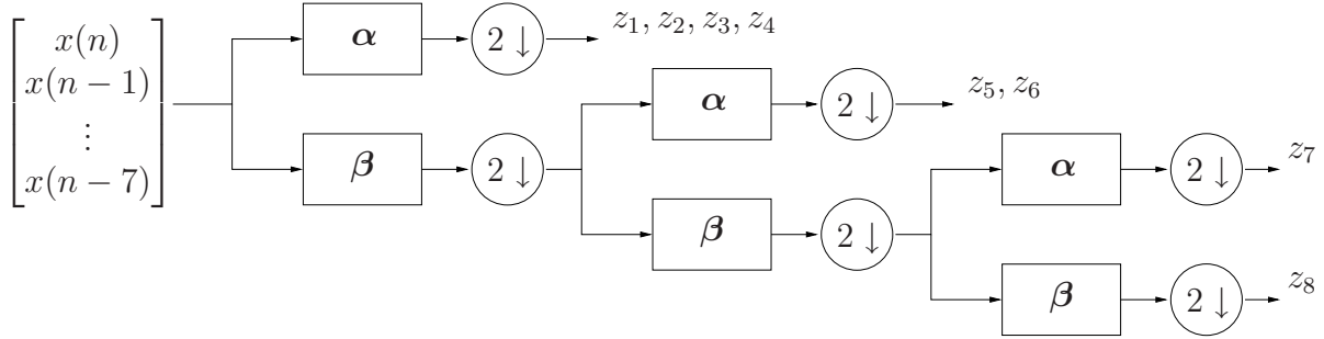
Figura 3.4: Transformada Haar por banco de filtros.
