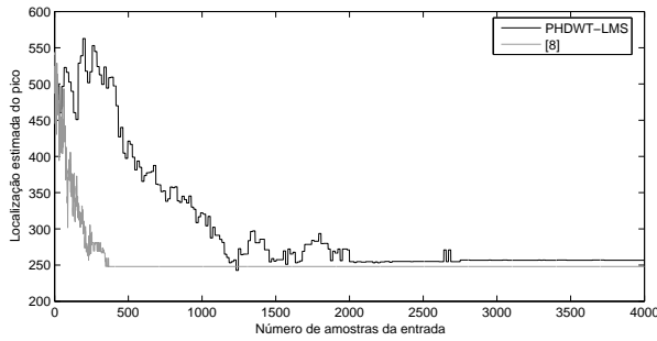
Figura B.23: LEP por amostra da entrada.
