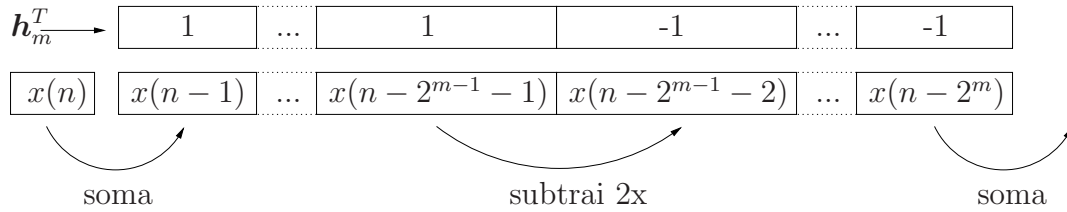
Figura 3.12: Ilustração do cálculo recursivo da transformada Haar parcial.
