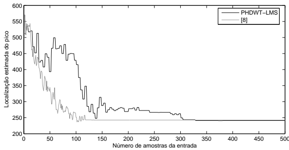
Figura 6.5: LEP por amostra da entrada.
