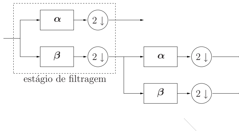
Figura 3.3: Banco de filtros
