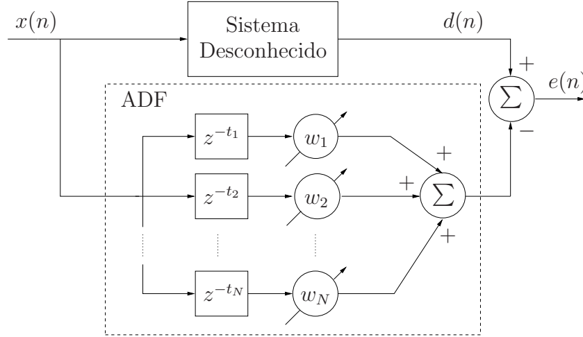
Figura 2.1: Filtro Adaptativo de Atraso.
