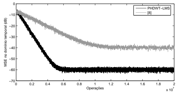
Figura 6.17: MSE por operações.
