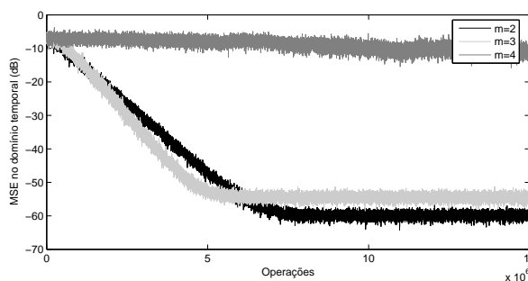
Figura B.221: MSE por operações.
