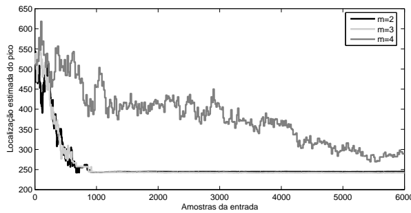
Figura B.208: LEP por amostras da entrada.
