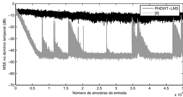
Figura B.160: MSE por amostra da entrada.
