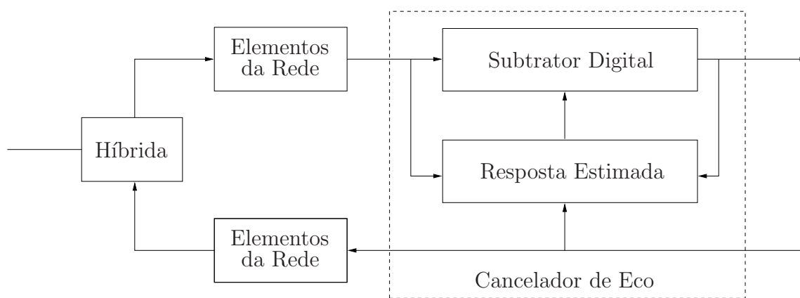
Figura 1.3: Cancelador de eco.
