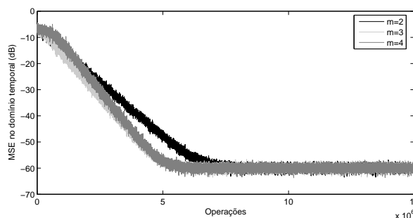
Figura B.171: MSE por operações.
