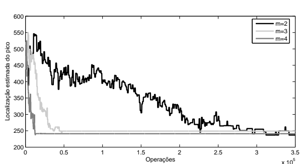
Figura B.199: LEP por operações.
