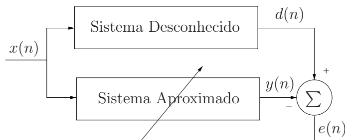
Figura 1.1: Identificação clássica de sistemas.
