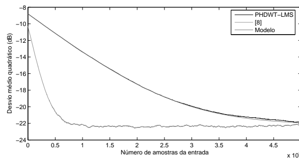
Figura 6.9: Desvio médio quadrático
