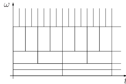
Figura 3.2: Transformada wavelet
