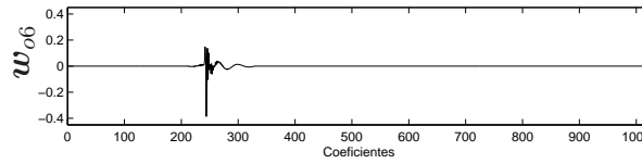
Figura B.128: Resposta w_{o6} criada com g_6
