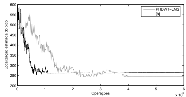
Figura 6.42: LEP por operações.
