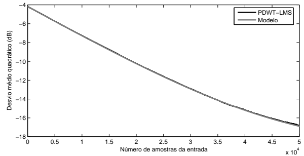
Figura 6.84: MSD e modelo para PDWT-LMS
