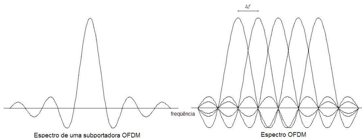
Figura 2.4: Espectro de frequência do sistema OFDM.
