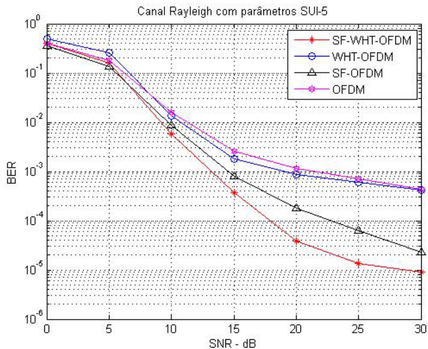
Figura 5.5: Canal Rayleigh SUI-5.
