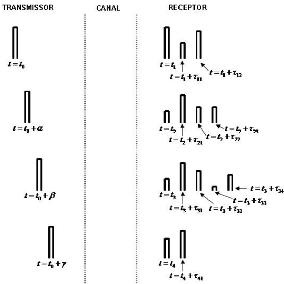
Figura 1.2: Exemplo do mesmo sinal sendo transmitido várias vezes em um canal com multipercurso, mostrando sua variação no receptor.
