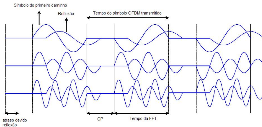
Figura 2.11: Transmissão de um símbolo OFDM apenas com tempo de guarda, sem símbolo estendido, em um canal com dois percursos 7 [17].
