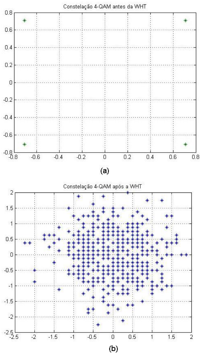
Figura 3.4: Sinal de informação antes (a) e depois (b) da WHT (em banda base).
