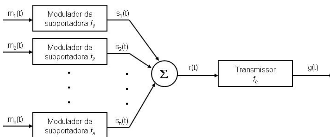
Figura 2.3: Modulação multiportadora.
