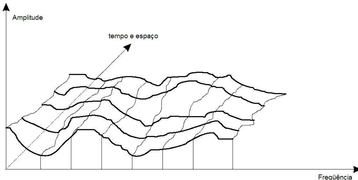
Figura 1.4: Resposta em freqüência típica de um canal com multipercurso (em banda-base).
