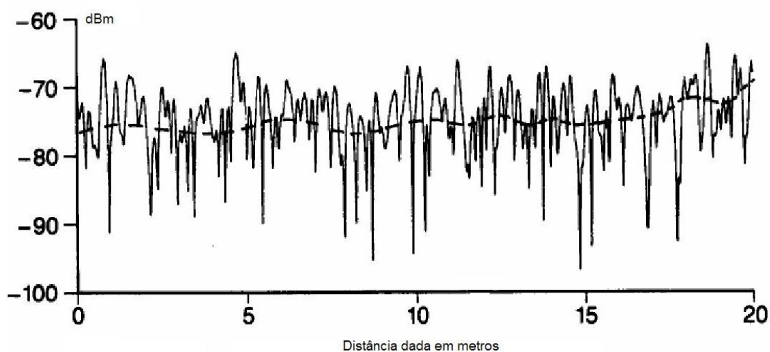
Figura 1.3: Exemplo de uma conexão com desvanecimento.
