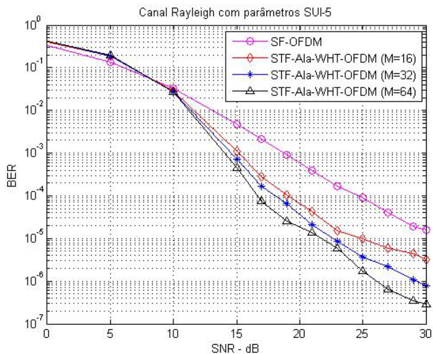
Figura 5.12: Canal Rayleigh SUI-5 para os sistemas com STF.
