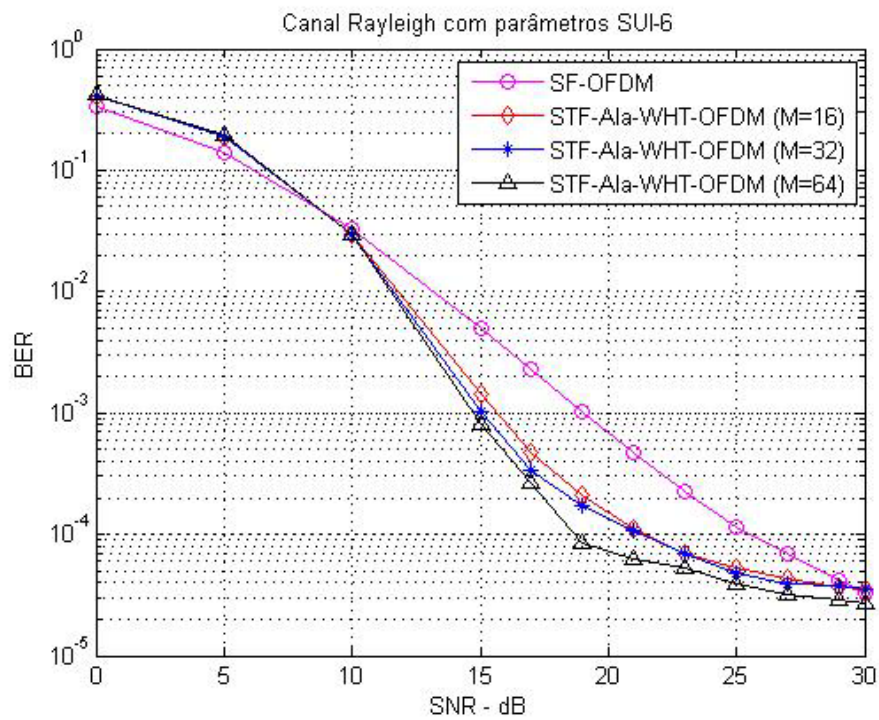
Figura 5.13: Canal Rayleigh SUI-6 para os sistemas com STF
