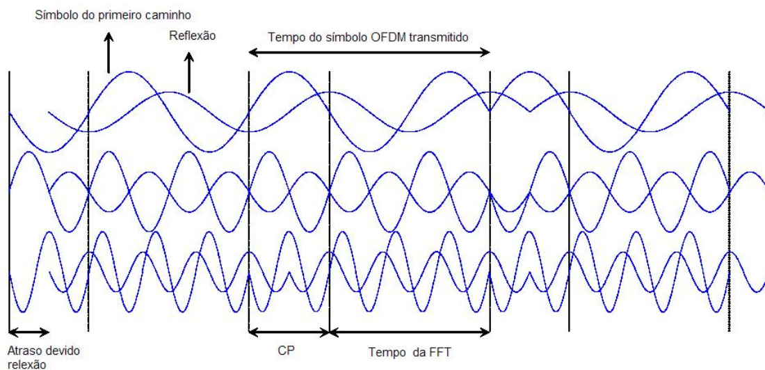
Figura 2.12: Transmissão de um símbolo OFDM com prefixo cíclico, em um canal com dois percursos, usando a modulação BPSK nas três sinusóides [17].
