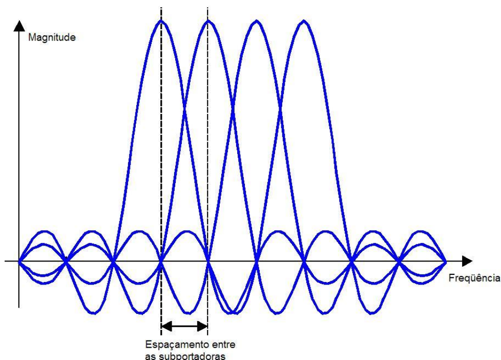
Figura 2.7: Espectro do símbolo OFDM.
