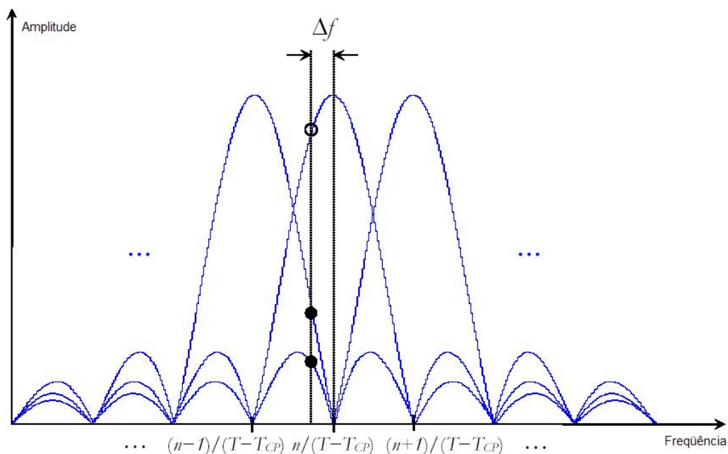
Figura 2.15: Erro devido ao deslocamento em frequência. Quando há deslocamento em frequência, as outras subportadoras passam a interferir, como mostra os pontos indicados na figura.
