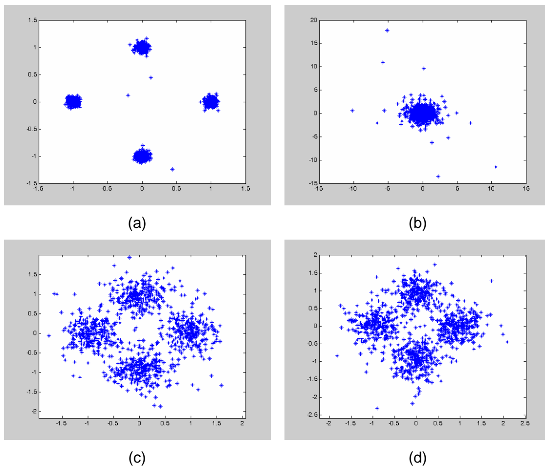
Figura 3.5: Exemplo do efeito da utilização da WHT em um sistema OFDM, com uma subportadora sendo transmitida por um canal com desvanecimento profundo. As figuras ilustram como as subportadoras foram recebidas no receptor. (a) Subportadora P do símbolo OFDM que não sofre desvanecimento profundo; (b) Subportadora J do símbolo OFDM que sofre com desvanecimento profundo; (c) e (d) Subportadoras P e J com a introdução da WHT no sistema OFDM, respectivamente.
