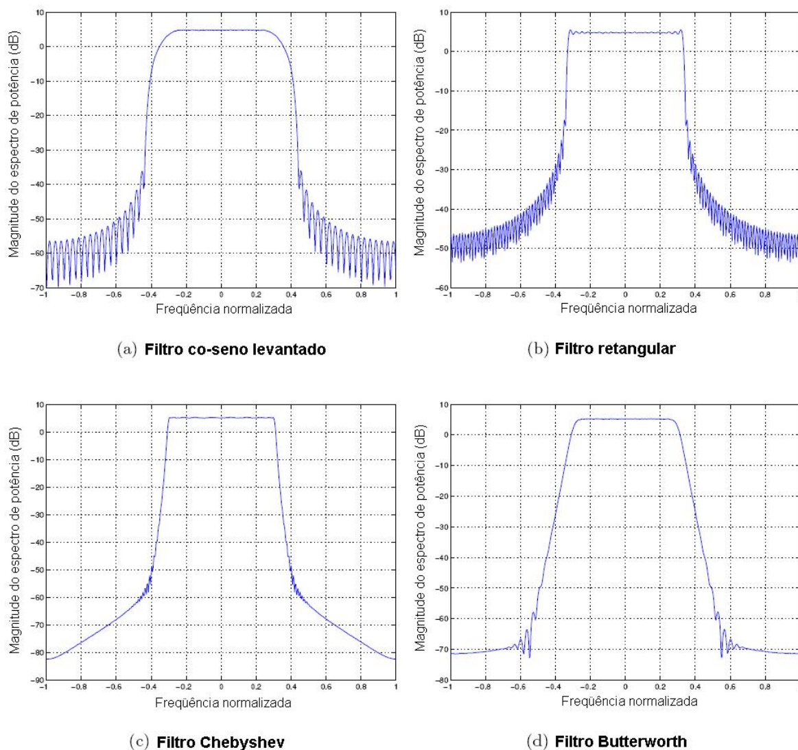
Figura 2.13: Resposta em frequência de diferentes filtros [36].
