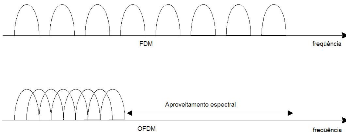
Figura 2.6: Comparação do aproveitamento espectral entre o sistema FDM e OFDM.
