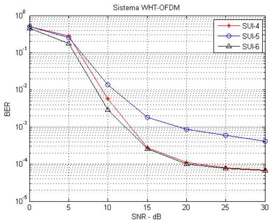
Figura 5.8: Sistema WHT-OFDM.
