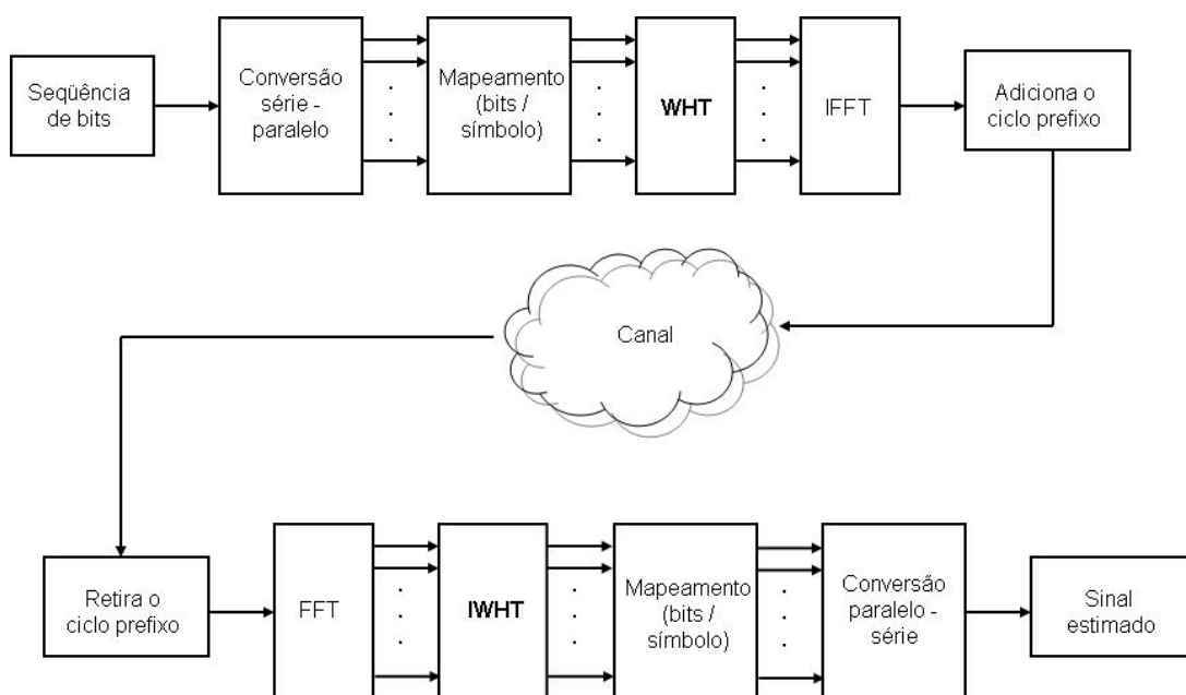
Figura 3.3: Sistema WHT-OFDM.
