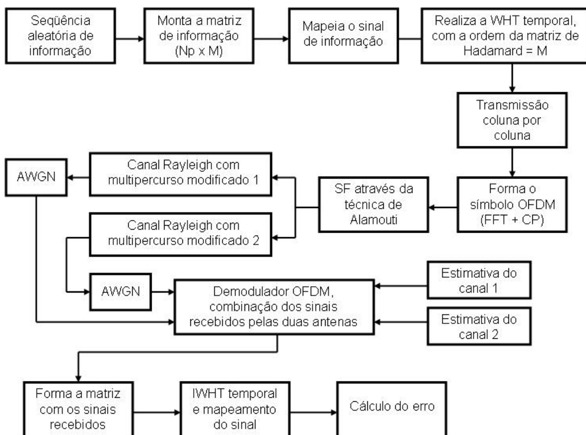
Figura 5.3: Algoritmo usado para os sistemas que envolvem o esquema STF.
