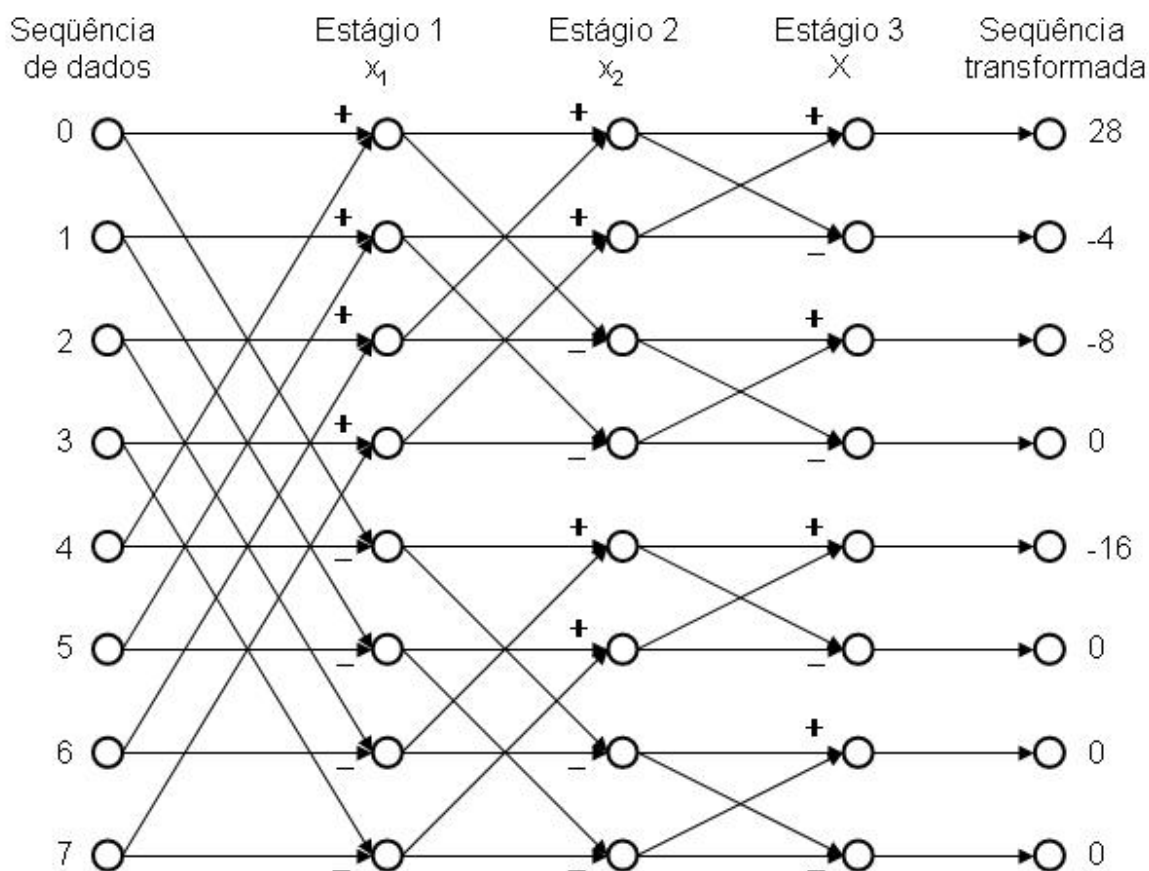
Figura 3.2: Exemplo de uma FWHT com seqüência de dados de oito pontos.
