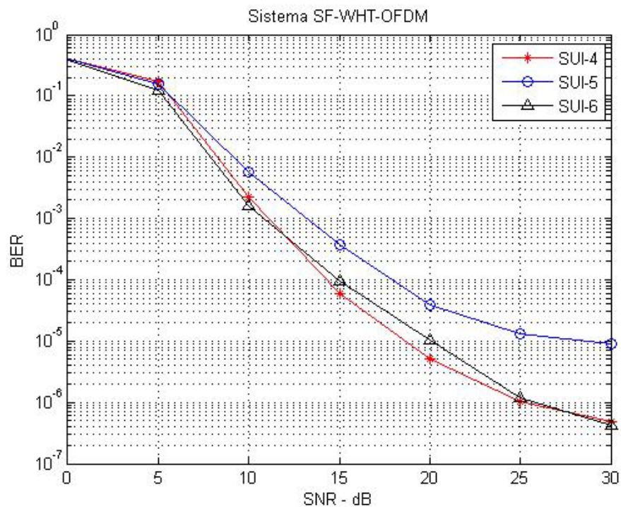
Figura 5.10: Sistema SF-WHT-OFDM.
