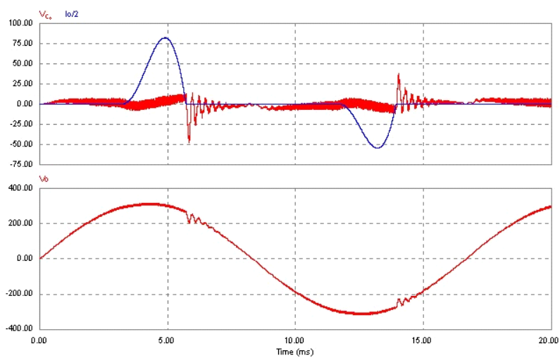
Fig. 73 – v_i , i_o/2 e v_o para V_{i\_eficaz} = 220V(nominal) .
