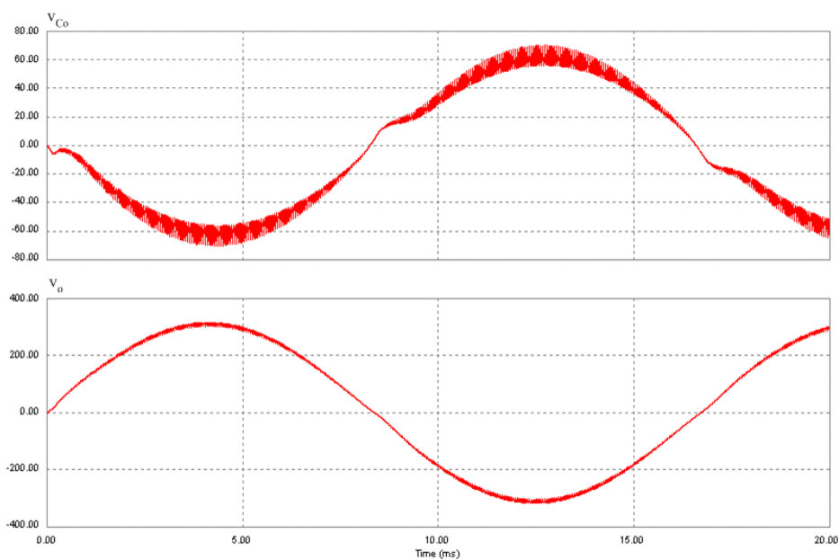
Fig. 70 – V_{Co} e v_o para V_{i\_eficaz} = 264V .
