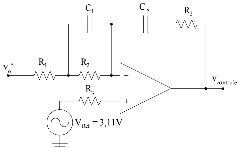
Fig. 109 – Controlador PID.
