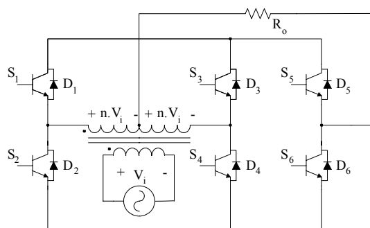
Fig. 11 – Segunda e quarta etapas de operação.
