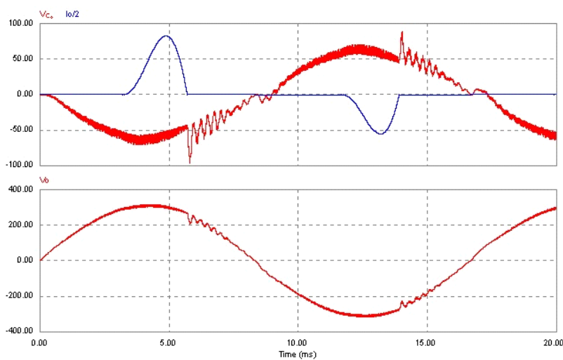
Fig. 74 – v_i , i_o/2 e v_o para V_{i\_eficaz} = 264V(+20\%) .
