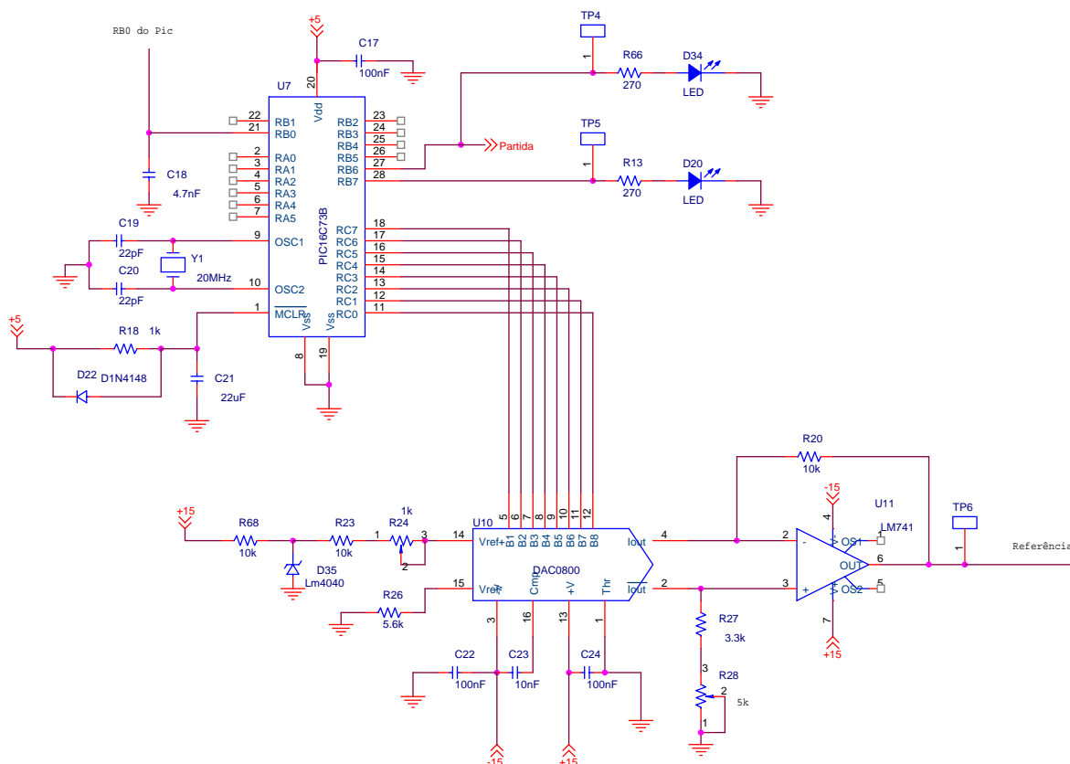
Fig. 103 – Gerador da Senóide de Referência Retificada.
