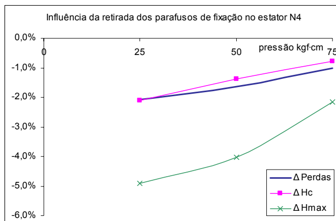
Fig. 4.2 – Diferenças com e sem parafuso no estator com revestimento C-0 (N4).
