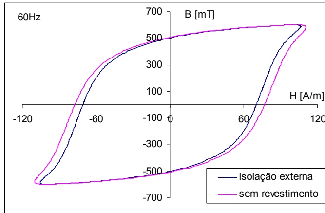
Fig. 4.14 - Laço BH do estator L4 nos casos com isolação natural e externa entre lâminas a 0,6 T.
