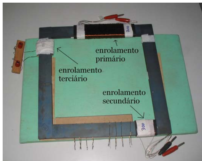
Fig. 5.5 – Protótipo construído para medição da interferência dos anéis de curto circuito
