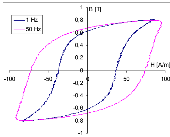
Fig. 1.2 – Laços BH medidos a 1Hz e 50 Hz
