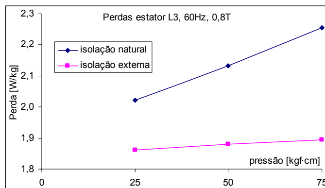
Fig. 4.5 – Medidas das perdas magnéticas no estator L3 com isolamento natural e com acréscimo de isolamento externa entre lâminas.
