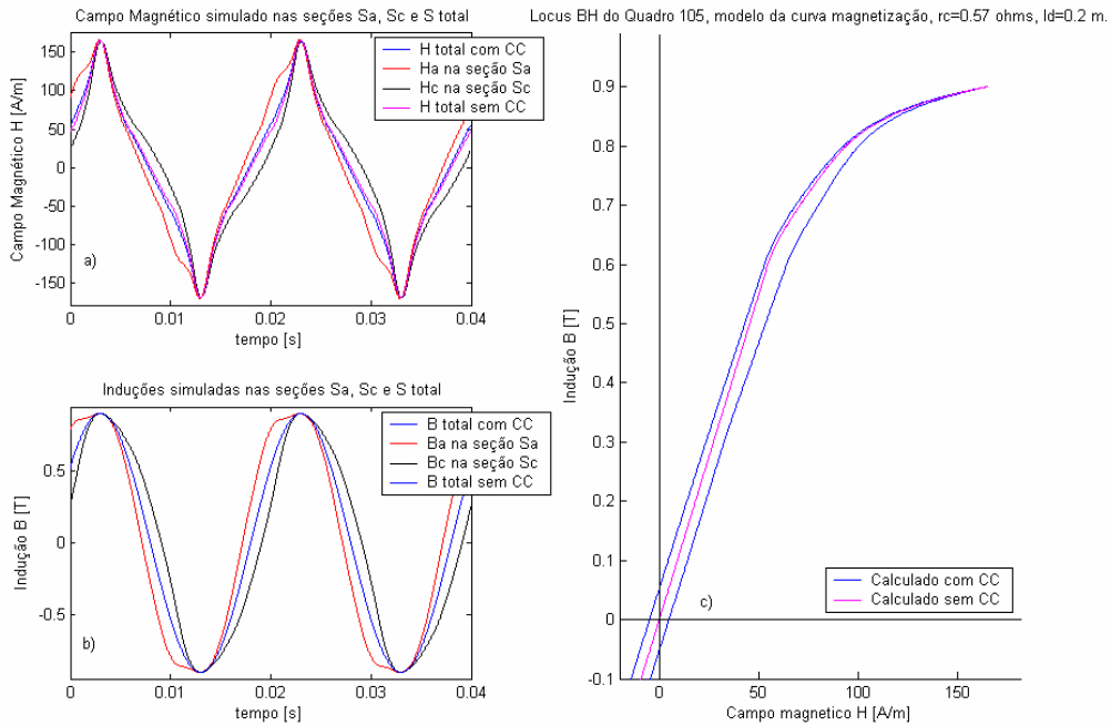
Fig. 6.6 - Valores simulados de campo H , indução B e lócus BH para quadro 105, utilizando a permeabilidade obtida da curva de magnetização inicial de acordo com a indução
