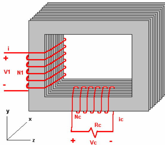
Fig. 6.1 – representação do circuito magnético com espira de Curto Circuito (CC)
