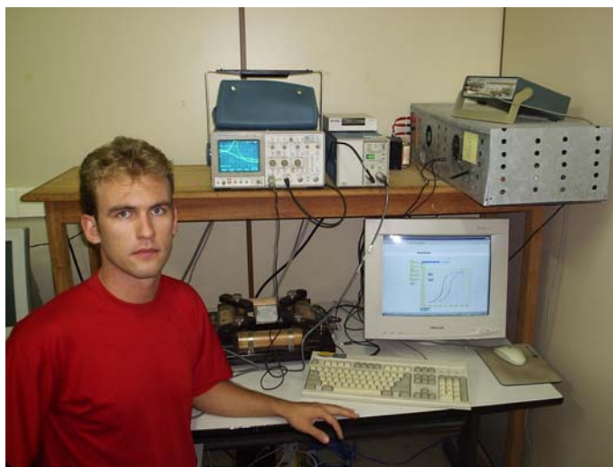
Fig. A.4 – Bancada de caracterização de materiais magnéticos desenvolvida no GRUCAD
