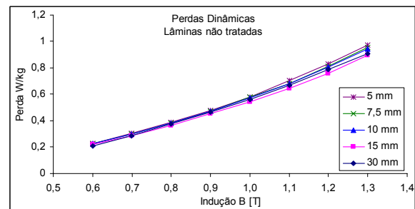
Fig. 2.16 – Valores calculados da perda dinâmica à 50 Hz
