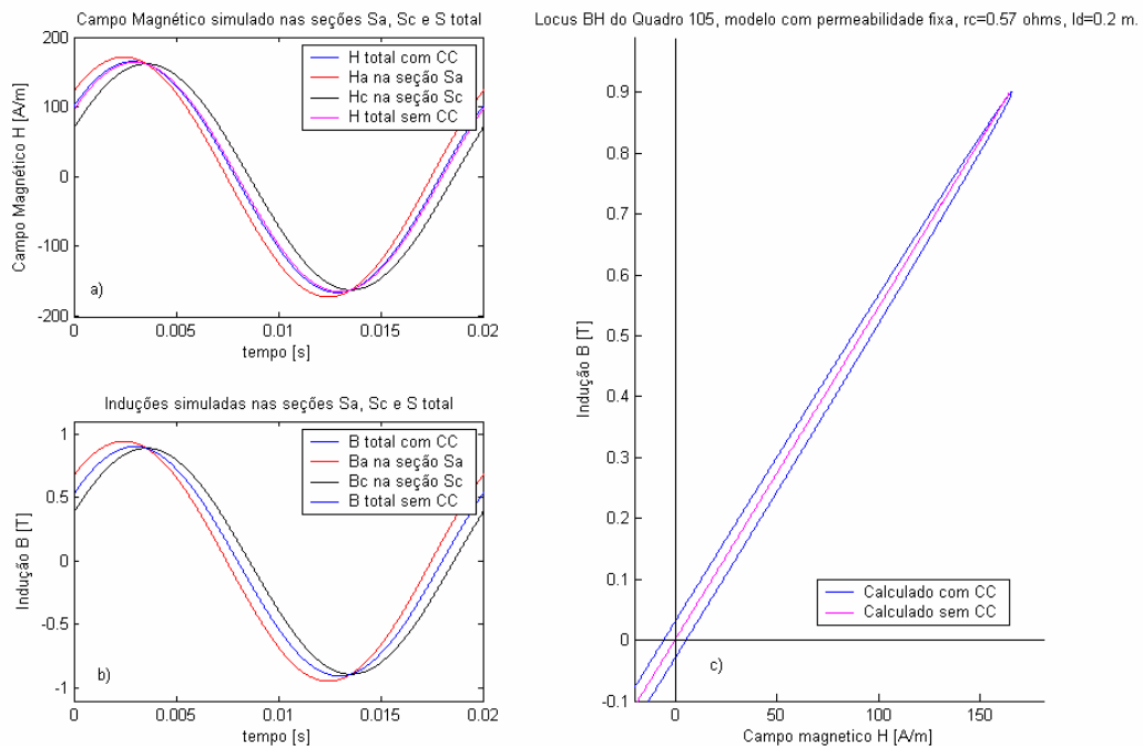
Fig. 6.5 – Valores simulados de campo H , indução B e locus BH para quadro com l_m=1050\text{mm} , utilizando uma permeabilidade constante
