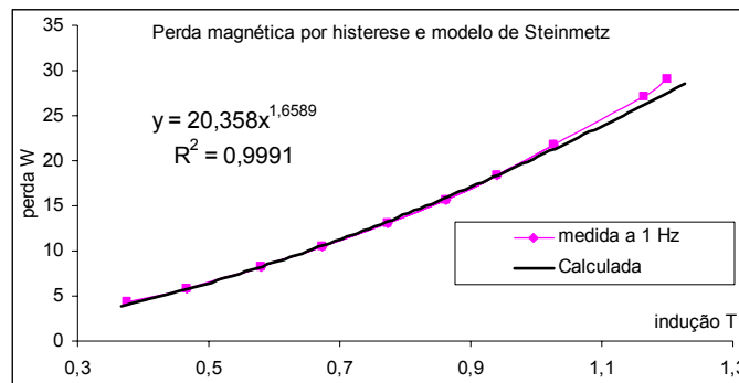
Fig. 1.1 – Medição das perdas e modelo de Steinmetz.
