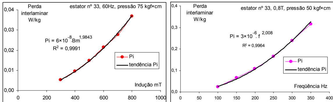
Fig. 4.19 – Perdas interlaminares medidas no estator nº 33, em função da frequência e indução
