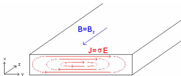
Fig. 1.3 – Distribuição das correntes induzidas na lâmina
