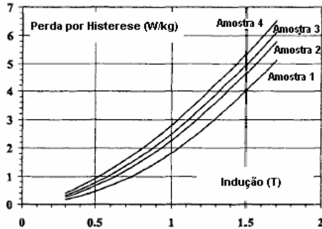
Fig. 2.11 – Perda por histerese das amostras toroidais [17]
