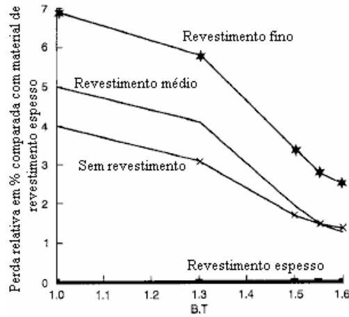
Fig. 3.3 - Efeito do revestimento na perda total [23]
