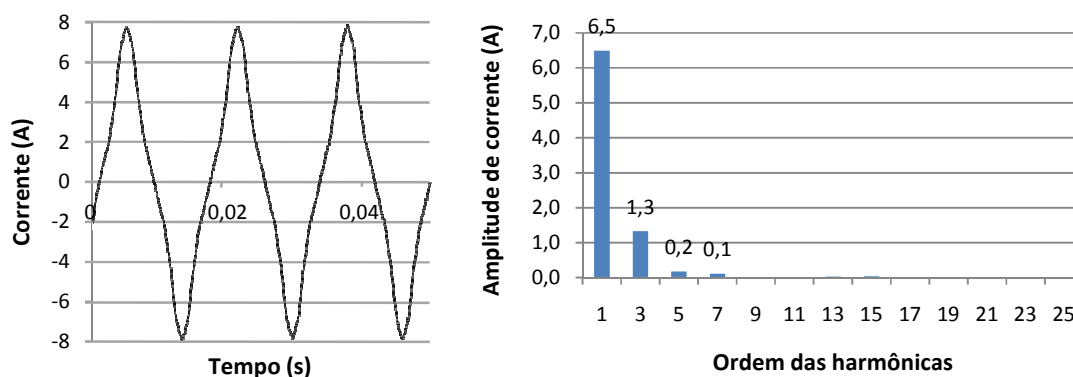
Fig. 6-9 – Forma de onda e espectro harmônico da corrente para aspirador de pó (C9).
