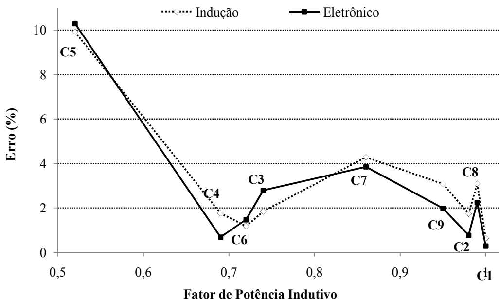
Fig. 6-12 – Erro dos medidores monofásicos em função do fator de potência.
