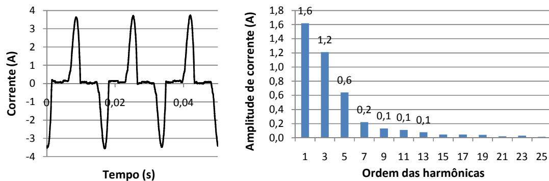
Fig. 6-15 – Forma de onda e espectro harmônico da corrente para lâmpadas eletrônicas (sistema trifásico) (C2).
