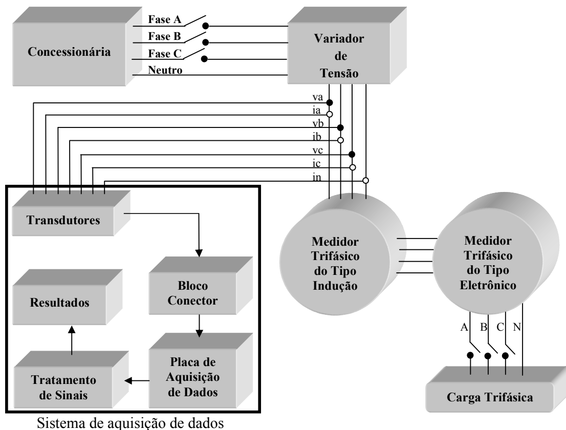
Fig. 5-6 – Sistema de medição trifásico implementado.
