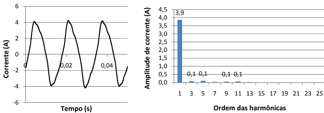
Fig. 6-6 – Forma de onda e espectro harmônico da corrente para enceradeira com FP igual a 0,72 (C6).
