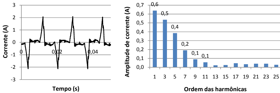
Fig. 6-20 – Forma de onda e espectro harmônico da corrente para computadores (sistema trifásico) (C7).
