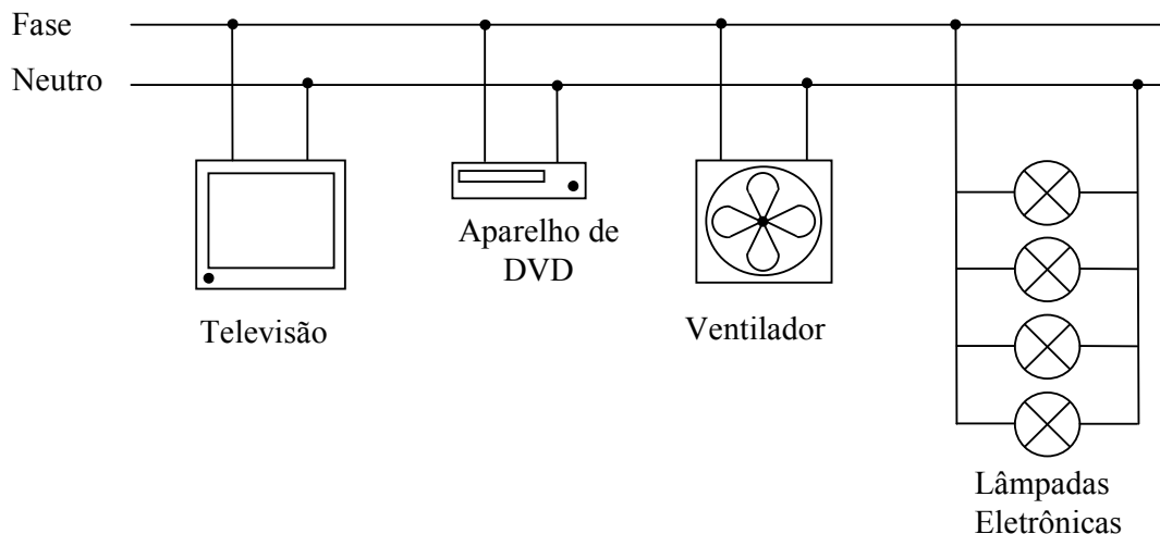
Fig. 5-13 – Televisão, aparelho de DVD, lâmpadas eletrônicas e ventilador.
