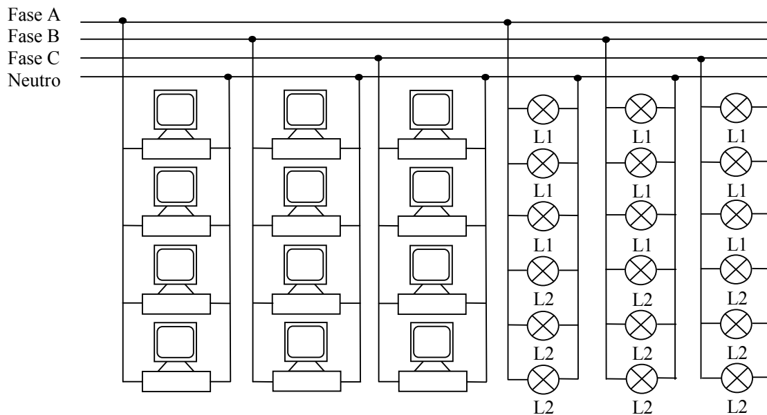
Fig. 5-23 – Computadores e lâmpadas eletrônicas (sistema trifásico).
