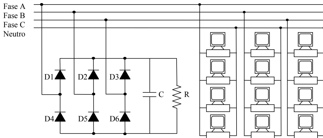
Fig. 5-26 – Retificador trifásico de onda completa com filtro capacitivo de 1080\ \mu\text{F} na saída e computadores.
