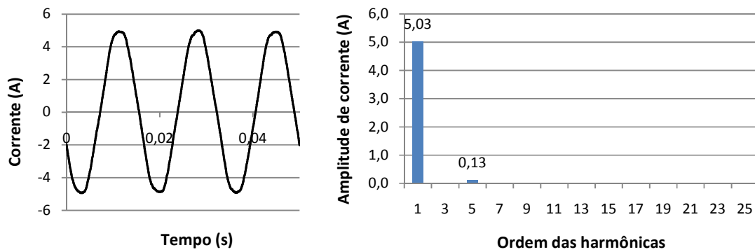
Fig. 6-14 – Forma de onda e espectro harmônico da corrente para carga linear (sistema trifásico) (C1).
