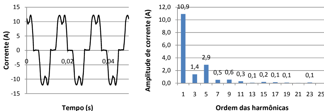
Fig. 6-23 – Forma de onda e espectro harmônico da corrente para retificador trifásico de onda completa com filtro capacitivo de 1080 \mu\text{F} na saída e lâmpadas eletrônicas (C10).
