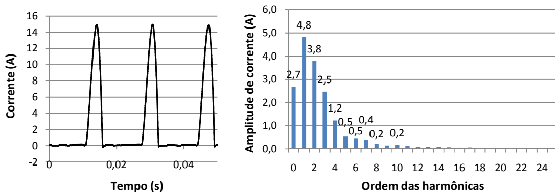
Fig. 6-22 – Forma de onda e espectro harmônico da corrente para retificador trifásico de meia onda com filtro capacitivo de 990 \mu\text{F} (C9).
