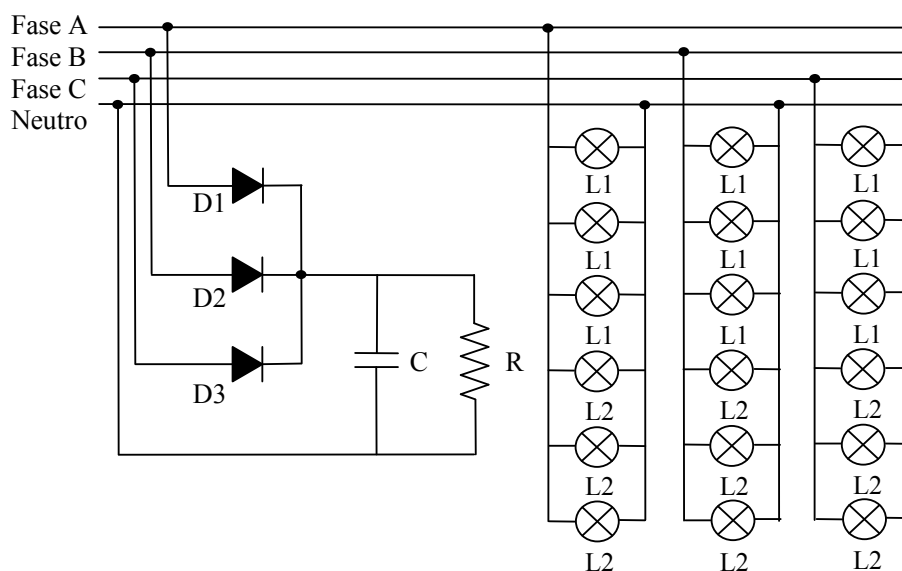
Fig. 5-18 – Retificador trifásico de meia onda com filtro de 990 \mu\text{F} e lâmpadas eletrônicas.
