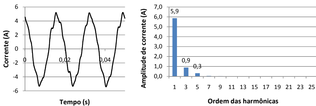
Fig. 6-19 – Forma de onda e espectro harmônico da corrente para motor de indução trifásico com FP igual a 0,90 (C6).
