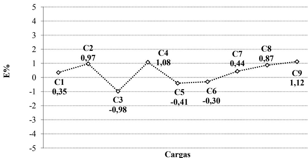
Fig. 6-11 – Erro entre os medidores monofásicos em função da carga.
