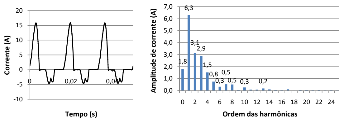
Fig. 6-16 – Forma de onda e espectro harmônico da corrente para retificador trifásico de meia onda com filtro capacitivo de 990 \mu\text{F} na saída e lâmpadas eletrônicas (C3).
