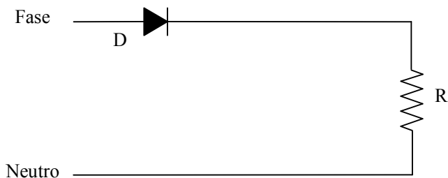
Fig. 5-10 – Retificador monofásico de meia onda.
