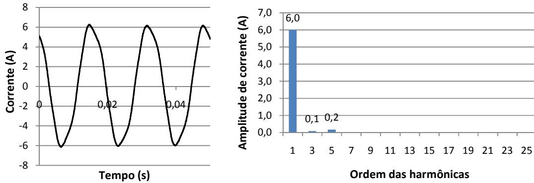
Fig. 6-5 – Forma de onda e espectro harmônico da corrente para enceradeira com FP igual a 0,52 (C5).
