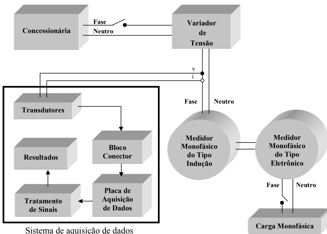
Fig. 5-5 – Sistema de medição monofásico implementado.
