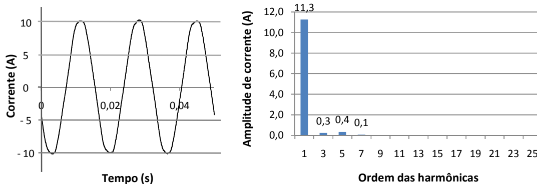
Fig. 6-8 – Forma de onda e espectro harmônico da corrente para ar condicionado (C8).
