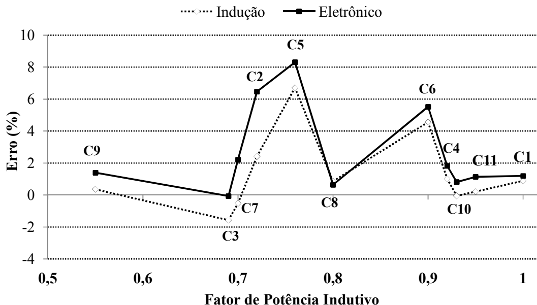
Fig. 6-27 – Erro dos medidores trifásicos em função do fator de potência.
