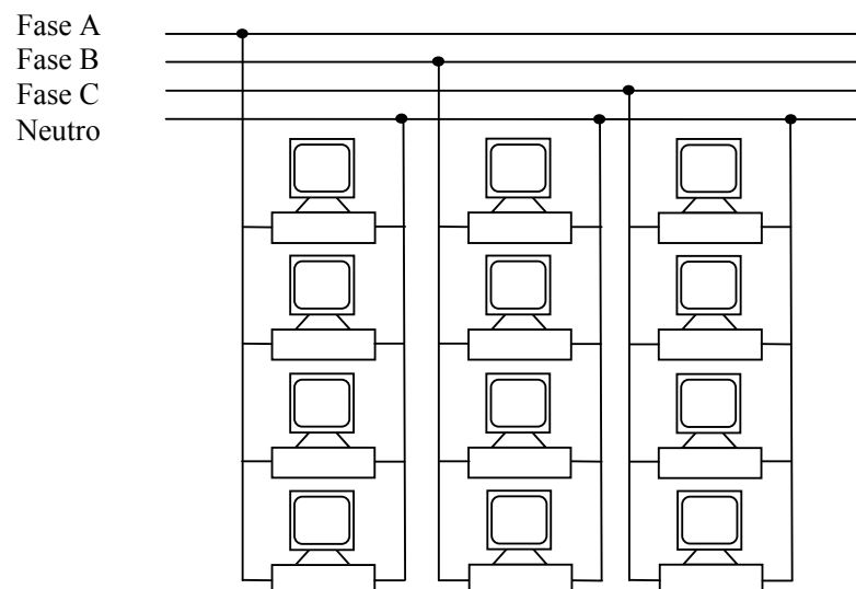
Fig. 5-22 – Computadores (sistema trifásico).
