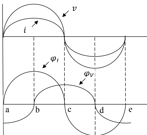
Fig. 4-3 – Formas de onda da tensão, da corrente e dos fluxos induzidos.
