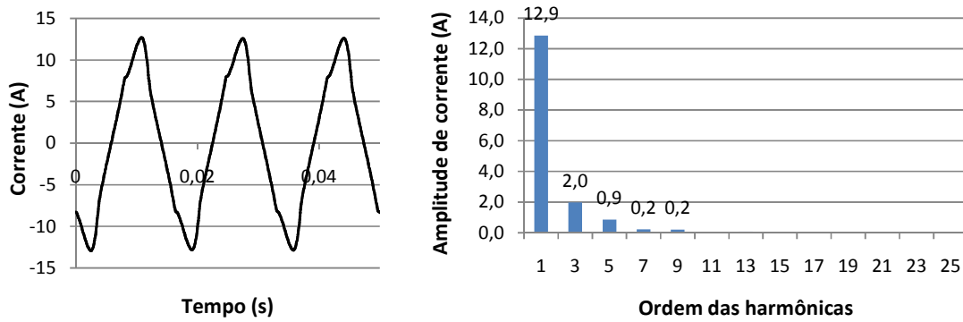
Fig. 6-2 – Forma de onda e espectro harmônico de corrente para carga linear e computadores (sistema monofásico) (C2).
