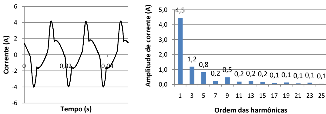
Fig. 6-7 – Forma de onda e espectro harmônico da corrente para televisão, aparelho de DVD, lâmpadas eletrônicas e ventilador (C7).
