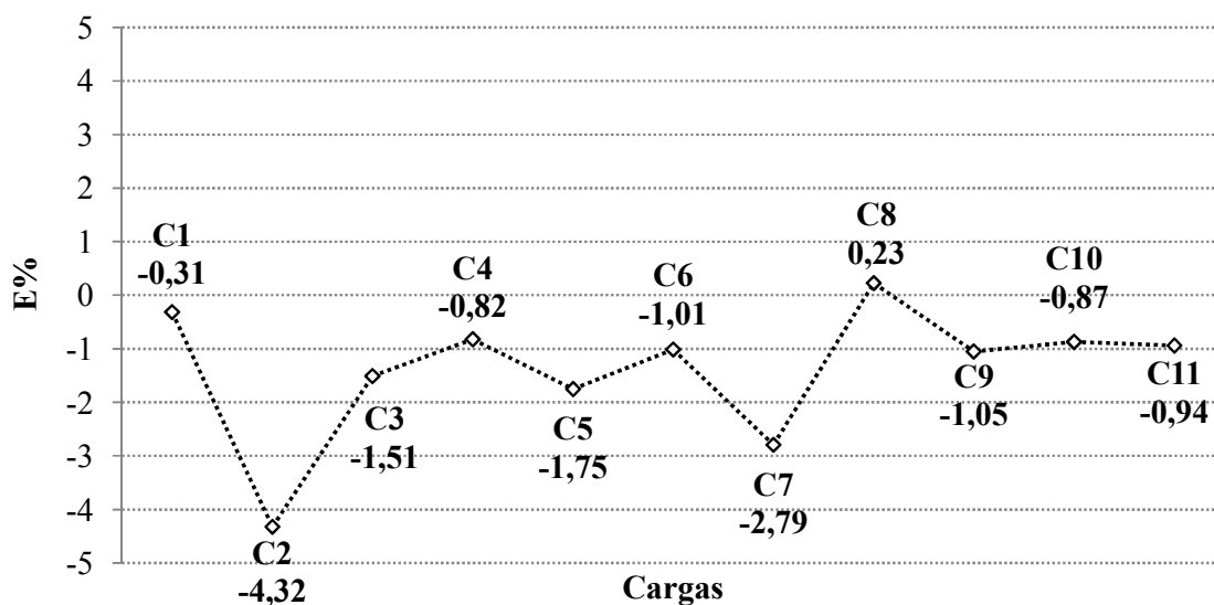
Fig. 6-26 – Erro entre os medidores trifásicos dos tipos eletromecânico e eletrônico em função da carga.
