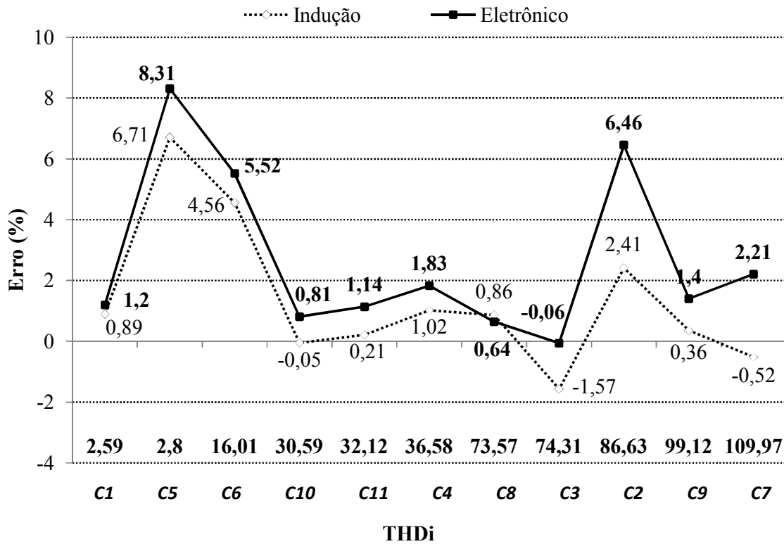
Fig. 6-28 – Erro dos medidores trifásicos em função do THD_i .
