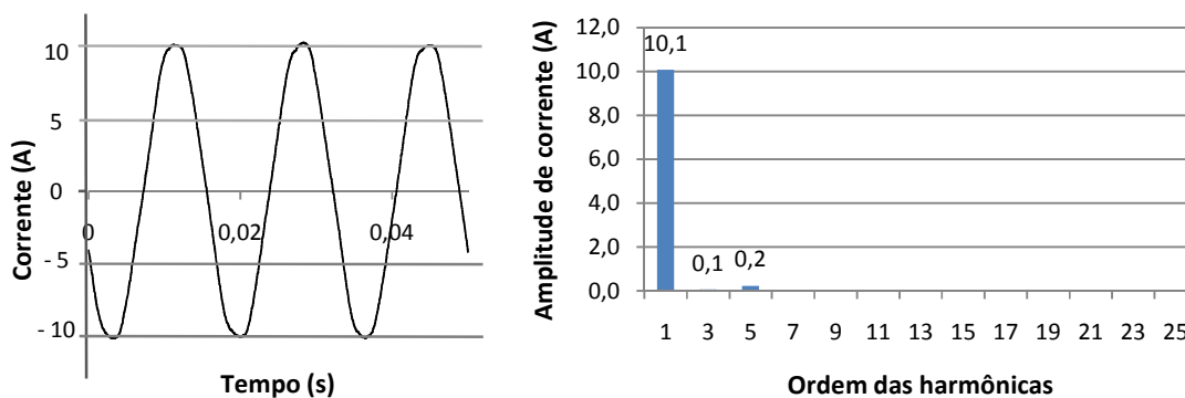
Fig. 6-1 – Forma de onda e espectro da corrente para carga linear (sistema monofásico) (C1).
