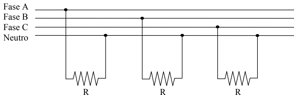
Fig. 5-16 – Carga linear (sistema trifásico).
