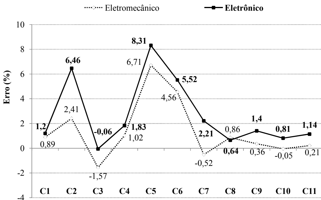
Fig. 6-25 – Erro entre os medidores trifásicos dos tipos eletromecânico e eletrônico em função do tipo de carga.
