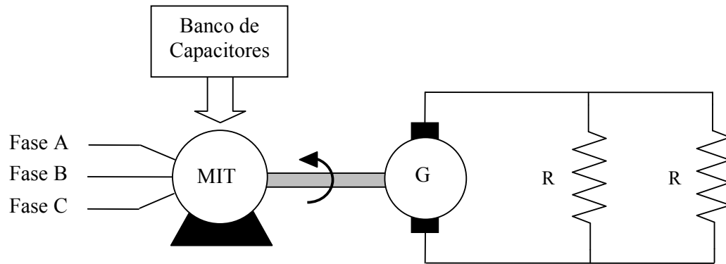
Fig. 5-21 – Motor de indução trifásico com FP igual a 0,90.
