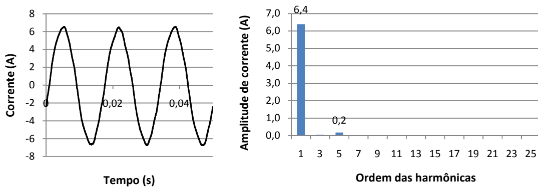
Fig. 6-18 – Forma de onda e espectro harmônico da corrente para motor de indução trifásico com FP igual a 0,76 (C5).
