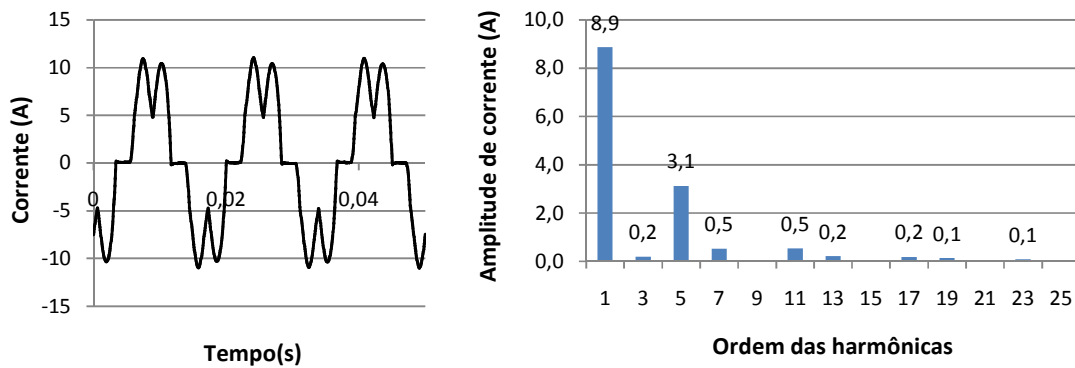
Fig. 6-17 – Forma de onda e espectro harmônico da corrente para retificador trifásico de onda completa com filtro capacitivo de 1080 \mu F na saída (C4).
