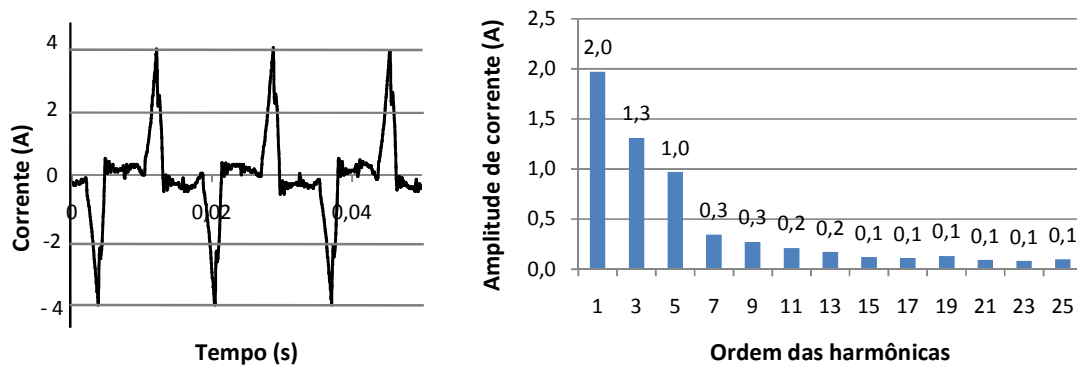
Fig. 6-3 – Forma de onda e espectro harmônico da corrente para carga computadores (sistema monofásico) (C3).
