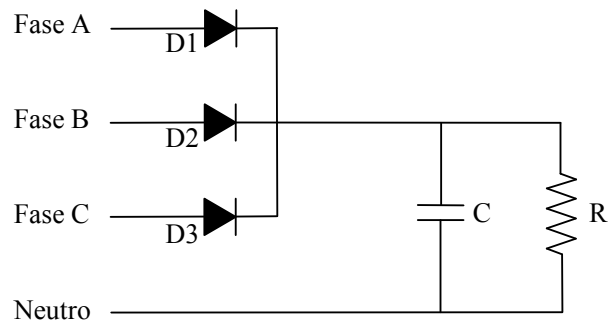
Fig. 5-24 – Retificador trifásico de meia onda com filtro capacitivo de 990 \mu\text{F} .
