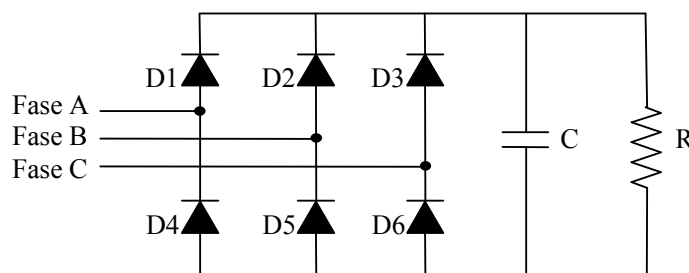
Fig. 5-19 – Retificador trifásico de onda completa com filtro capacitivo de 1080 \mu\text{F} na saída.
