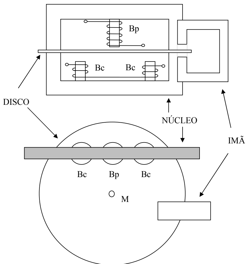
Fig. 4-1 – Componentes elementares do medidor eletromecânico.
