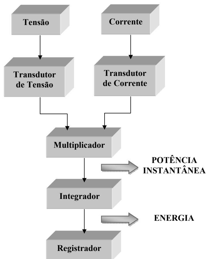
Fig. 4-5 – Diagrama em blocos de um medidor eletrônico.
