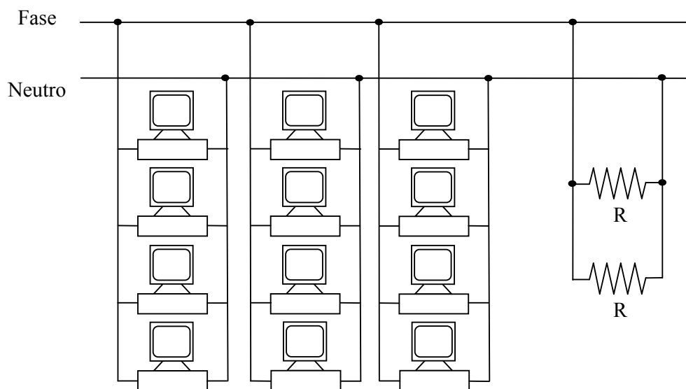
Fig. 5-8 – Carga linear e computadores (sistema monofásico).
