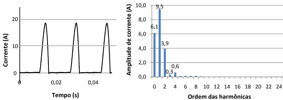
Fig. 6-4 – Forma de onda e espectro harmônico da corrente para retificador monofásico de meia onda (C4).
