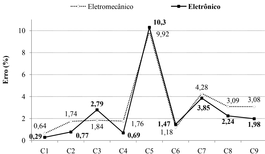
Fig. 6-10 – Erro entre os medidores monofásicos em função do tipo de carga.
