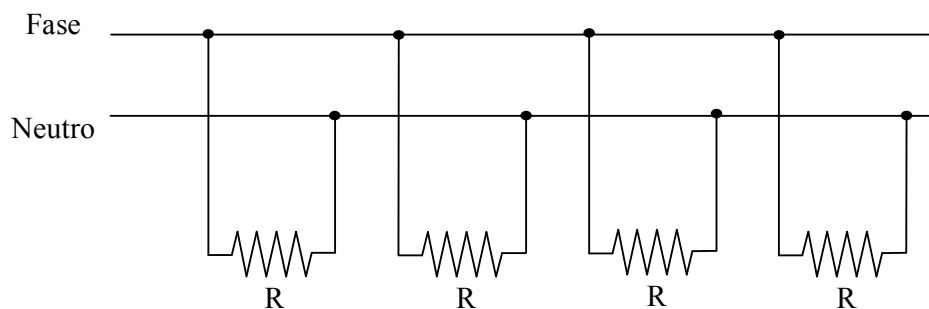
Fig. 5-7 – Carga linear com fator de potência unitário (sistema monofásico).
