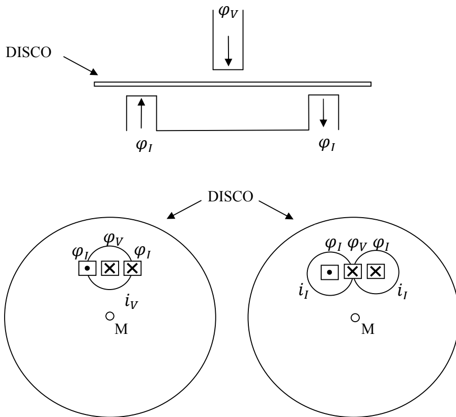
Fig. 4-2 – Fluxos induzidos no disco.
