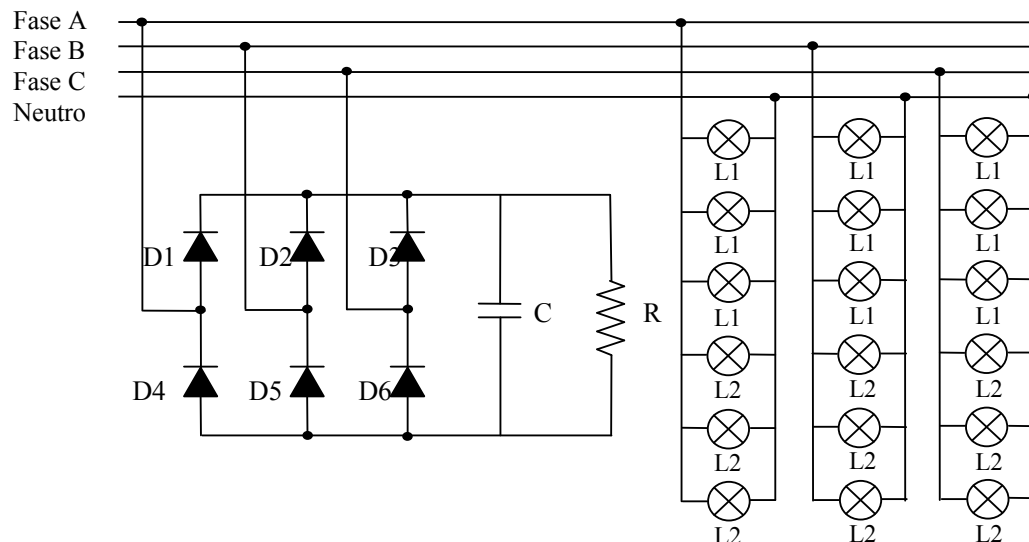
Fig. 5-25 – Retificador trifásico de onda completa com filtro 1080 \mu\text{F} e lâmpadas eletrônicas.
