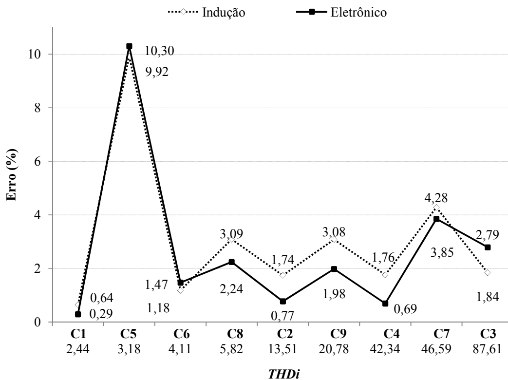
Fig. 6-13 – Erro dos medidores trifásicos em função do THD_i .
