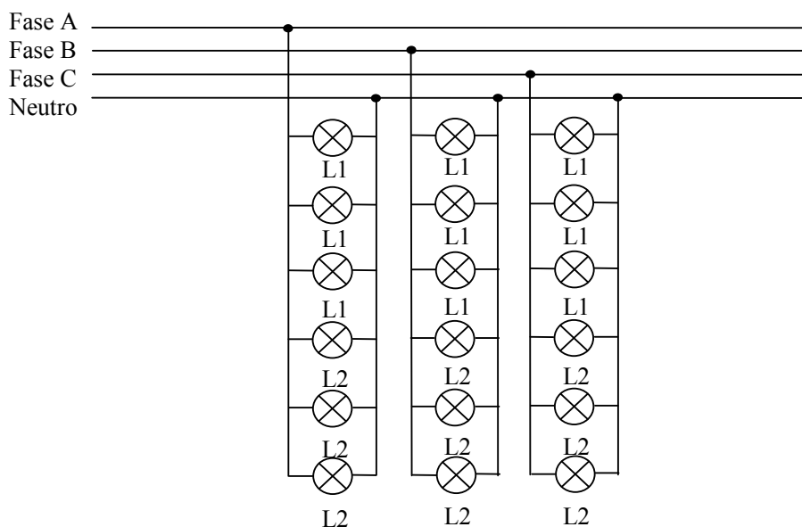
Fig. 5-17 – Lâmpadas eletrônicas (sistema trifásico).
