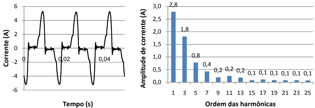
Fig. 6-21 – Forma de onda e espectro harmônico da corrente para computadores e lâmpadas eletrônicas (sistema trifásico) (C8).
