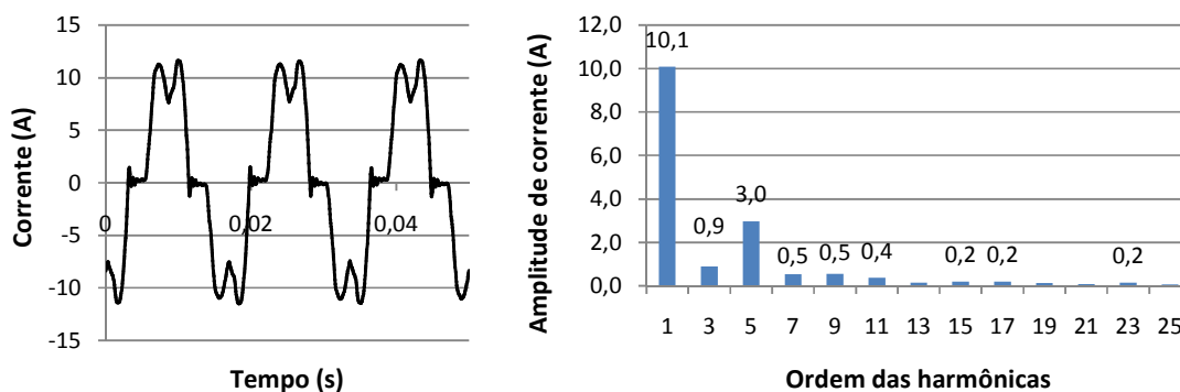
Fig. 6-24 – Forma de onda e espectro harmônico da corrente para retificador trifásico de onda completa com filtro capacitivo de 1080 \mu\text{F} na saída e computadores (C11).
