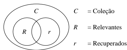
Figura 2.1: Precisão-Revocação
