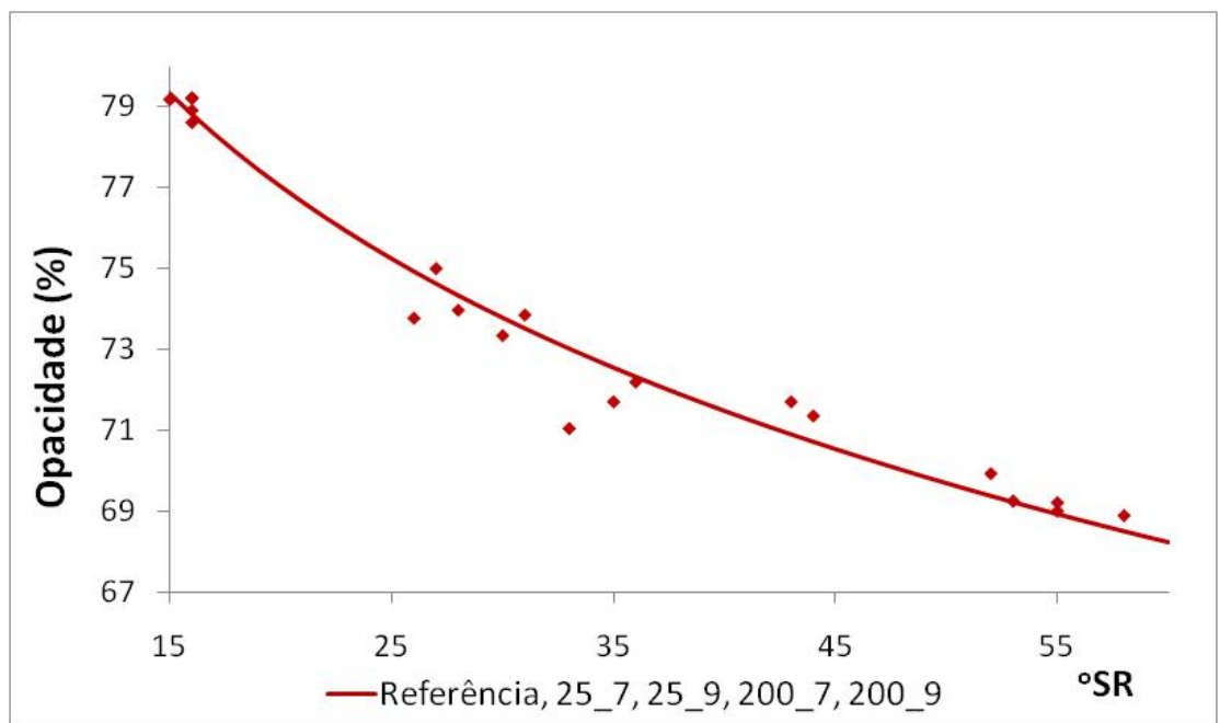
Figura 14. (a) Opacidade em função da Energia (Wh); (b) Opacidade em função do Grau Schopper Riegler (°SR). Representação por uma mesma curva dos tratamentos que não apresentaram diferença significativa entre si pelo teste de identidade de modelo a 5% de probabilidade.
