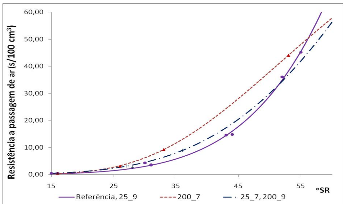
Figura 12. (a) Resistência à passagem de ar em função da Energia (Wh); (b) Resistência à passagem de ar em função do Grau Schopper Riegler (°SR). Representação por uma mesma curva dos tratamentos que não apresentaram diferença significativa entre si pelo teste de identidade de modelo a 5% de probabilidade.
