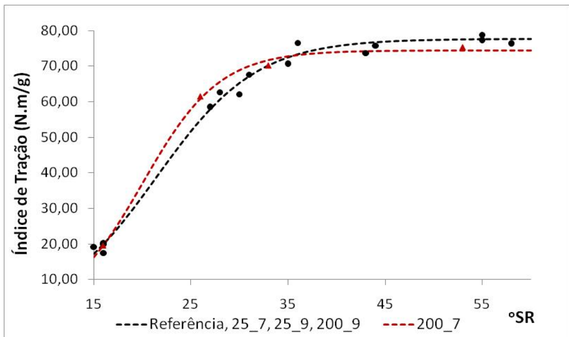
Figura 13. (a) Índice de tração em função da Energia (Wh); (b) Índice de tração em função do Grau Schopper Riegler (°SR). Representação por uma mesma curva dos tratamentos que não apresentaram diferença significativa entre si pelo teste de identidade de modelo a 5% de probabilidade.
