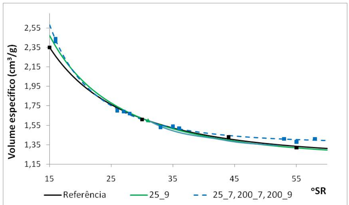
Figura 9. a) Volume específico em função da Energia (Wh); (b) Volume específico em função do Grau Schopper Riegler (°SR). Representação por uma mesma curva dos tratamentos que não apresentaram diferença significativa entre si pelo teste de identidade de modelo a 5% de probabilidade.
