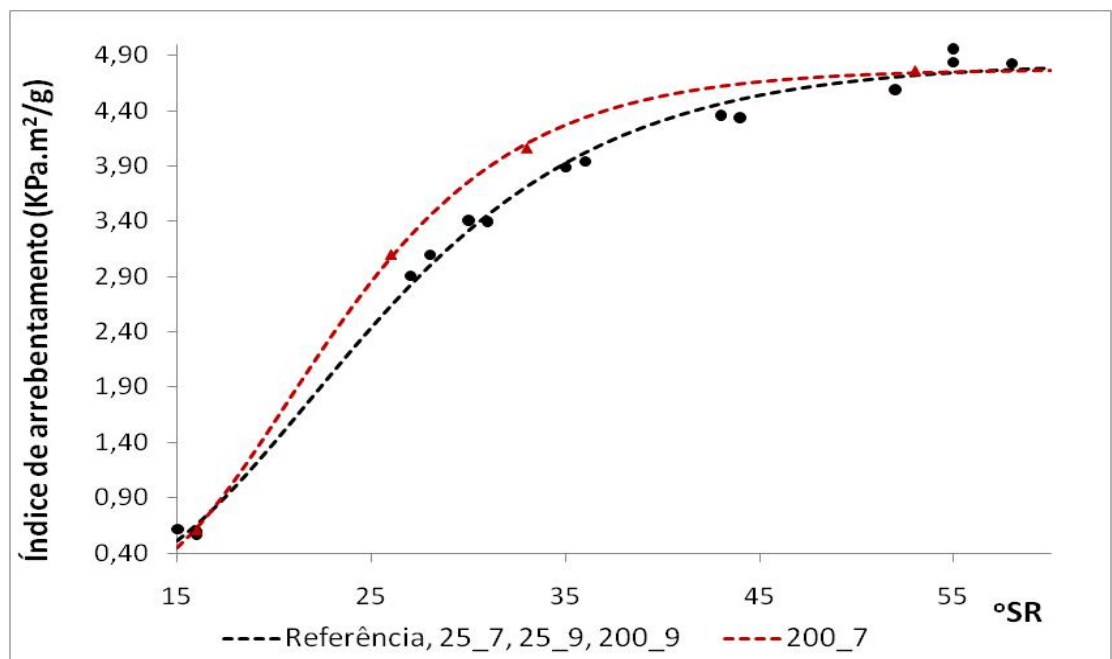
Figura 10. (a) Índice de arrebentamento em função da Energia (Wh). (b) Índice de arrebentamento em função Grau Schopper Riegler (°SR). Representação por uma mesma curva dos tratamentos que não apresentaram diferença significativa entre si pelo teste de identidade de modelo a 5% de probabilidade.
