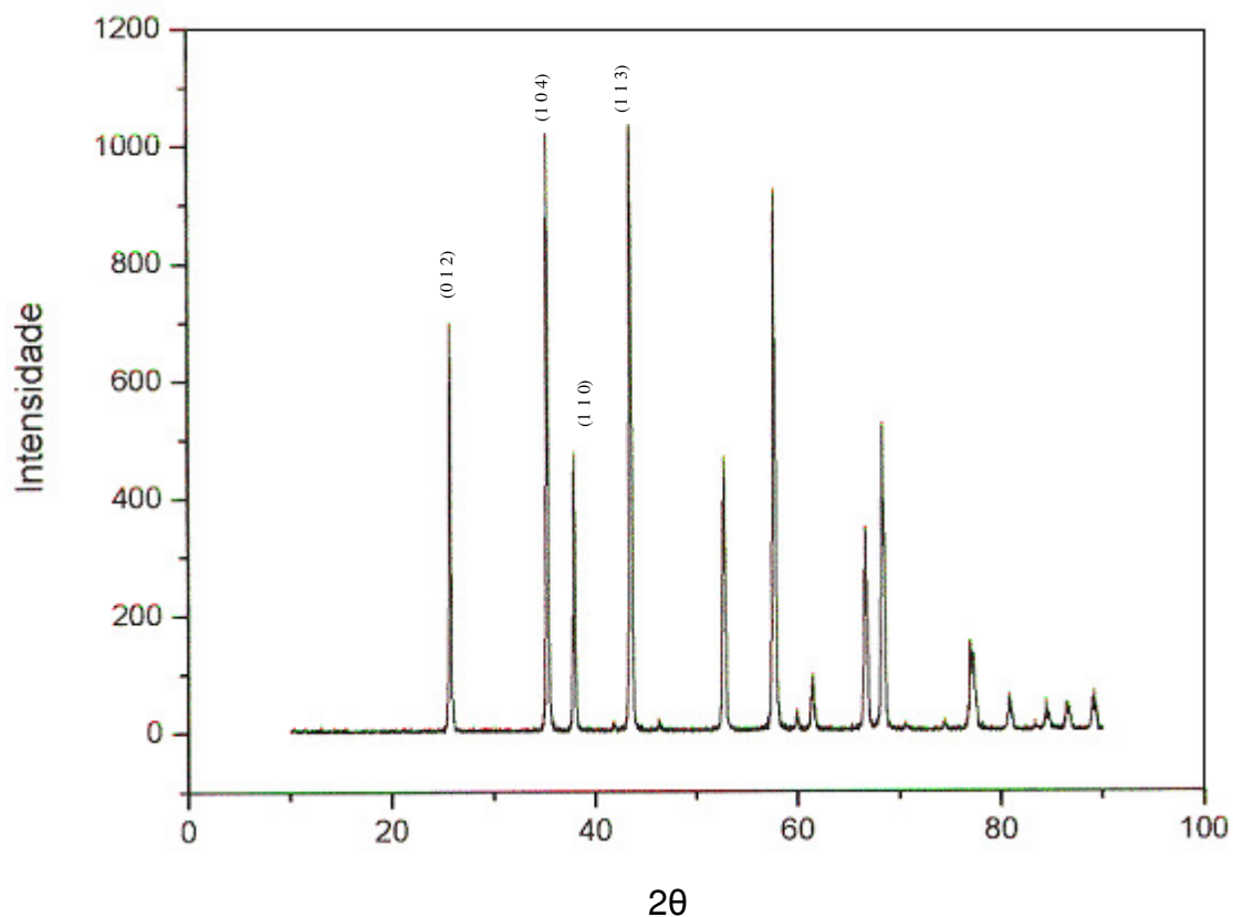
Figura 30 – Difratograma padrão da alumina
