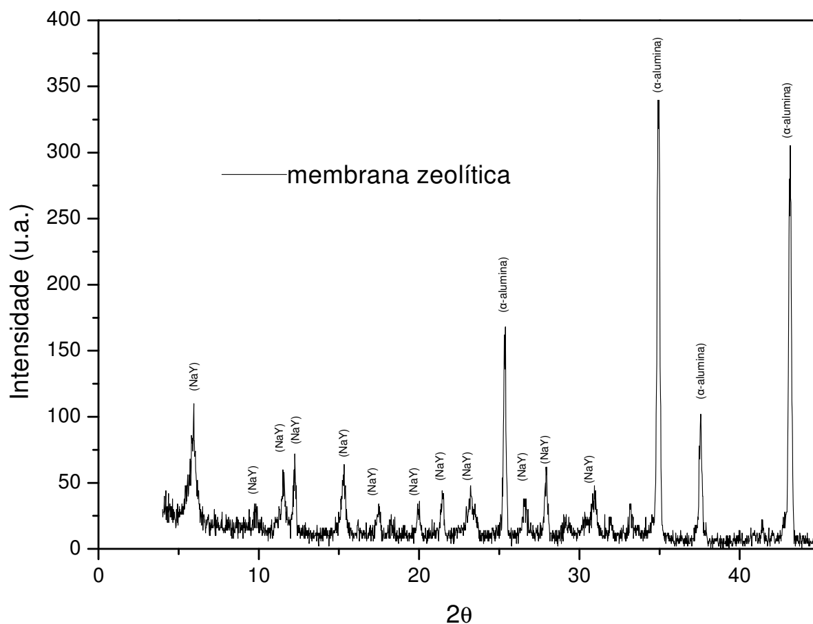
Figura 32 – Difratograma de raios X da membrana zeolítica (zeólita Y/(α-alumina)).
