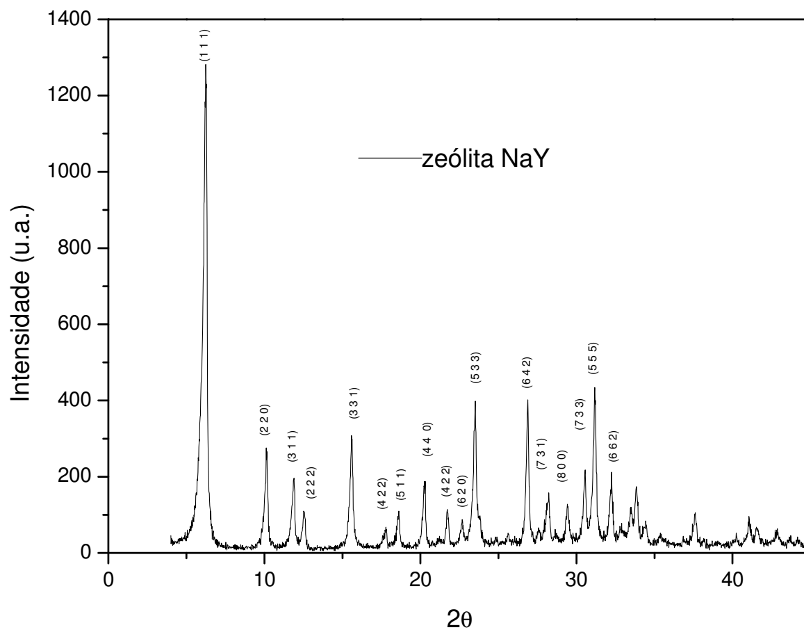
Figura 24 – Difratograma de Raios X da zeólita sintetizada Y (forma sódica).
