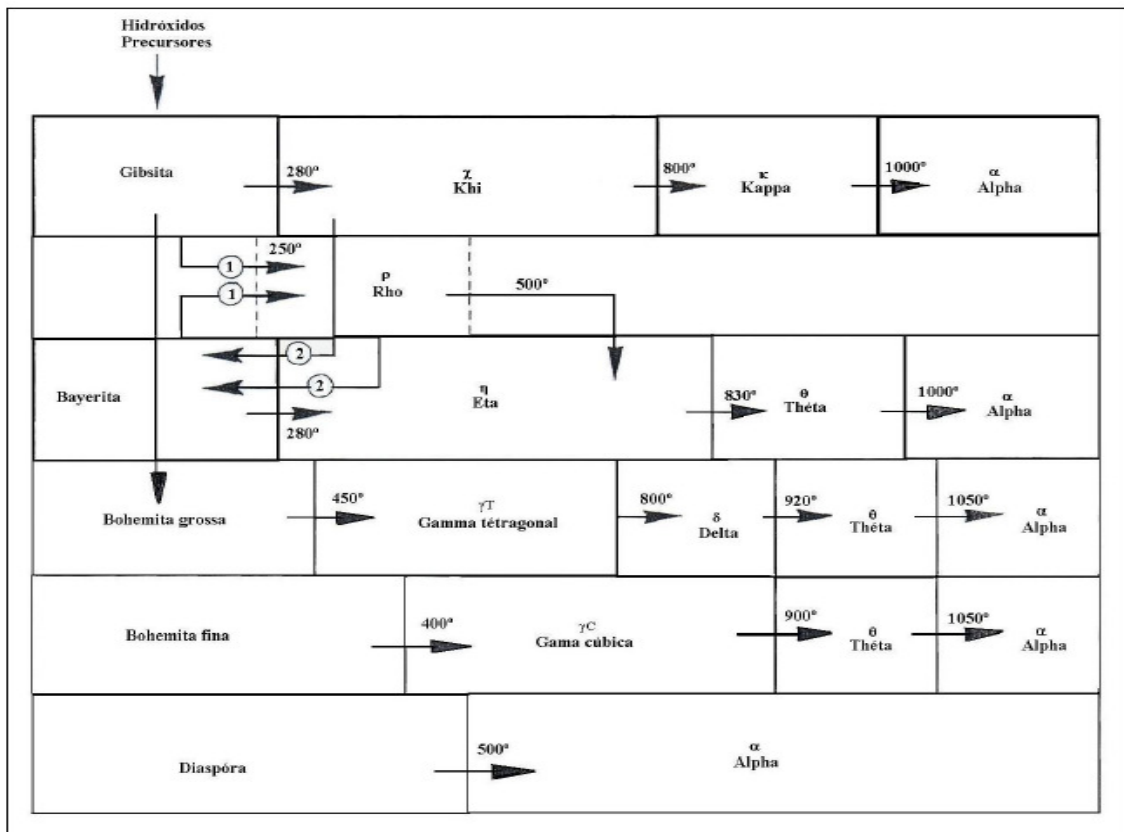
Figura 10 – Fases Cristalográficas da Alumina
