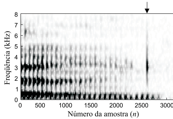
Fig. 4.7: Espectrograma de um segmento de fala contendo um clique involuntário.
