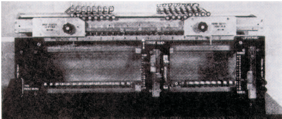
Fig. 2.6: “Electrical Vocal Tract” de H. K. Dunn.
