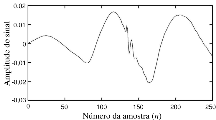
Fig. 4.2: Segmento de fala com clique.
