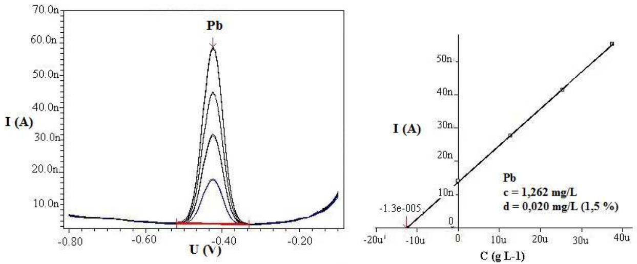
Figura 31: Voltamograma e curva de adição de padrão para recuperação de Pb adicionado em amostras de planta do Salto São Francisco.
