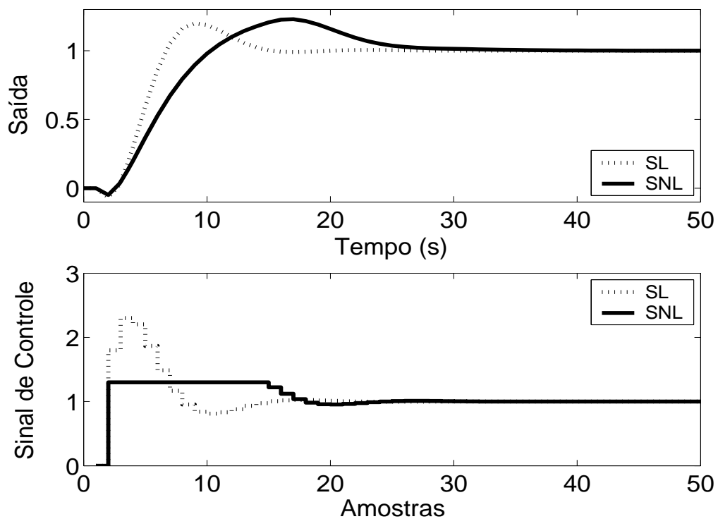
Figura 5.33: Saída e Sinal de Controle dos casos com e sem saturação em amplitude.
