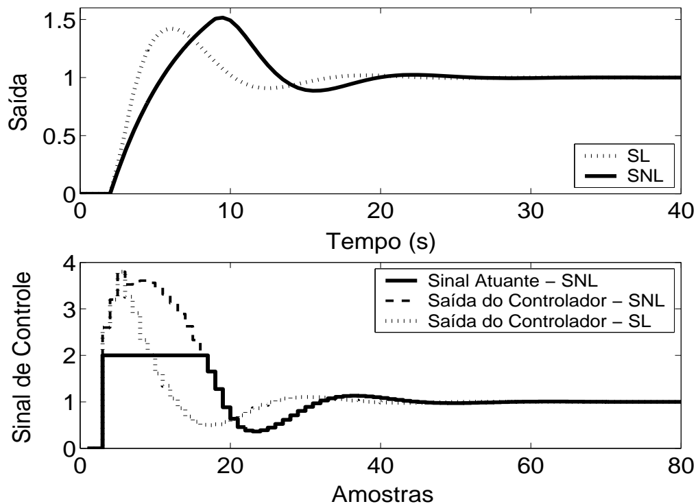
Figura 5.65: Saída e Sinal de Controle dos casos com e sem saturação em amplitude.
