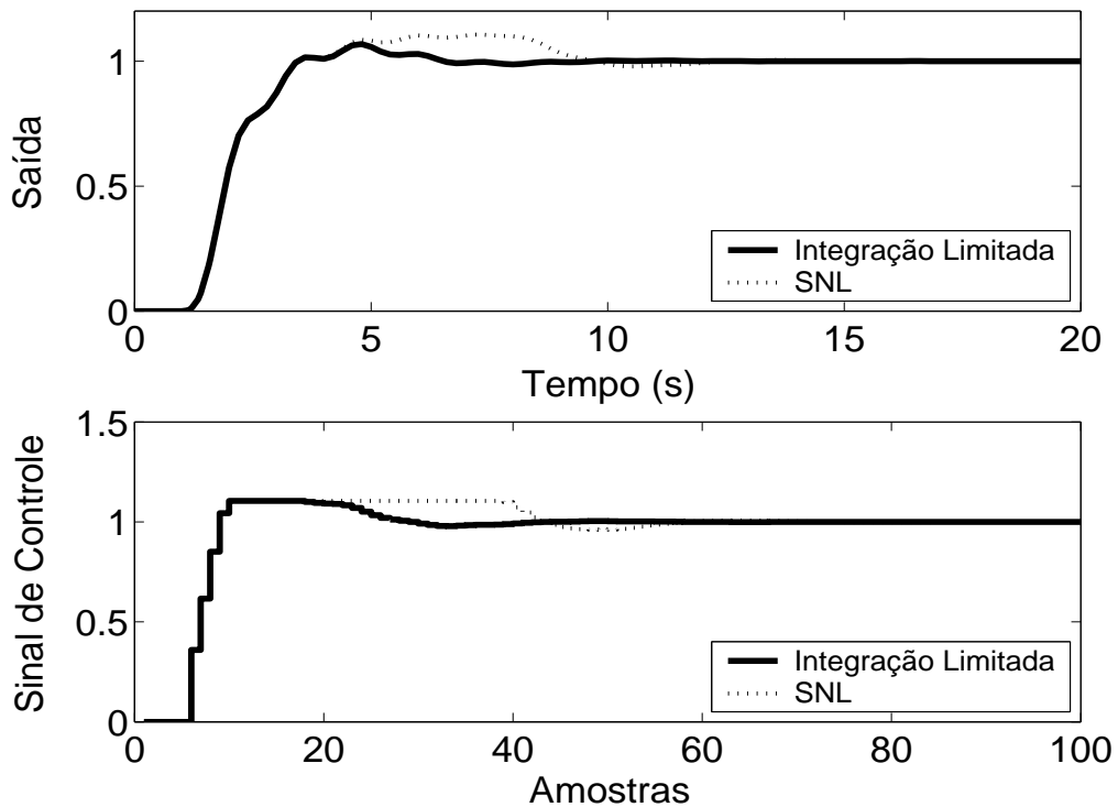
Figura 5.116: Saída e Sinal de Controle - Método Integração Limitada com l_{inf} = 0 , l_{sup} = 1.1 e b = 10 .
