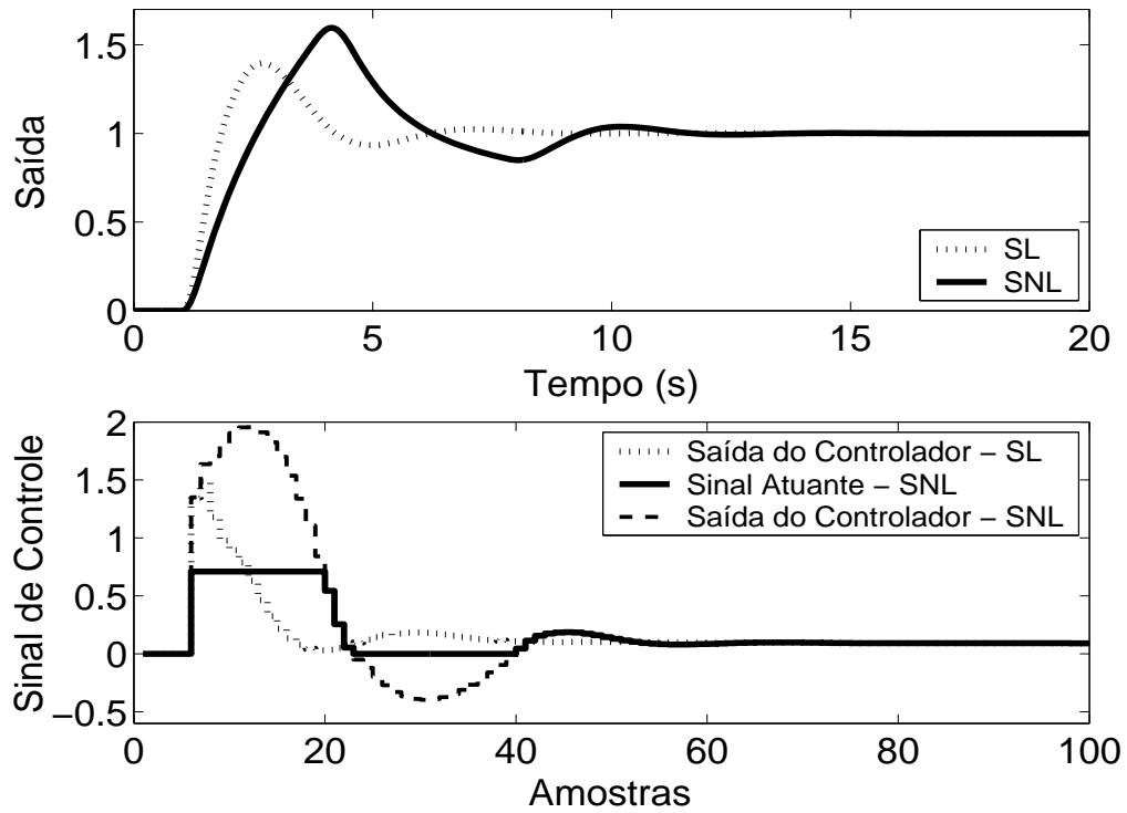
Figura 5.81: Saída e Sinal de Controle dos casos com e sem saturação em amplitude.
