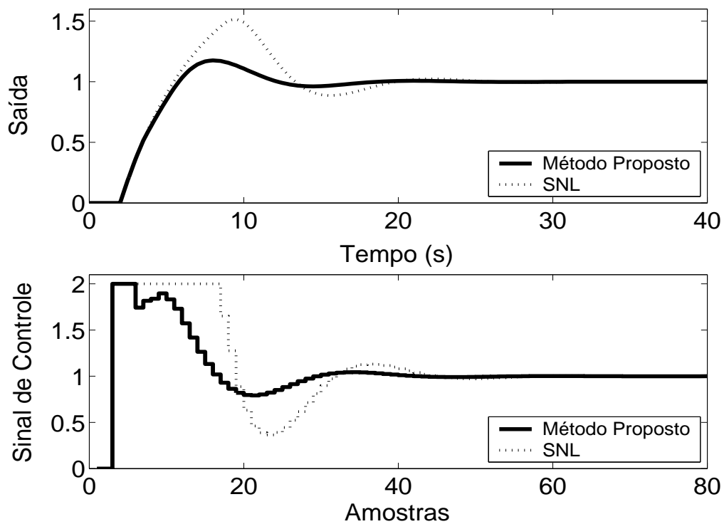
Figura 5.68: Saída e Sinal de Controle - Método Proposto por A. Visioli com K_t = 100 .
