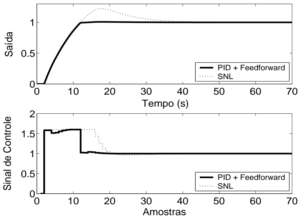
Figura 5.56: Saída e Sinal de Controle - Método PID + Feedforward com \tau = 9s e modelo de primeira ordem dado por (1 - 0.9048z^{-1})y(t) = z^{-2}0.0956u(t) .
