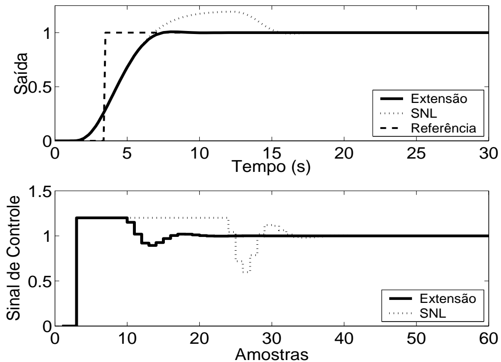
Figura 5.15: Técnica da Extensão Anti-Windup com margem de fase requerida igual a 45^\circ .
