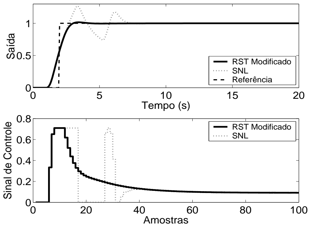
Figura 5.92: Saída e Sinal de Controle - Técnica RST Modificado com E(z^{-1}) = 1 - 0.06 .
