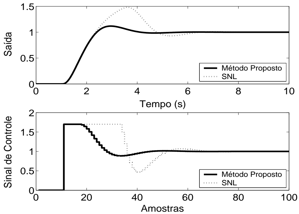
Figura 5.20: Saída e Controle - Método Proposto por A. Visioli com K_I = 10 .
