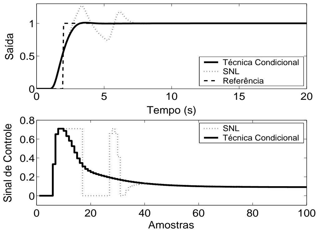
Figura 5.93: Saída e Sinal de Controle - Técnica Condicional - RST com k = 100 .
