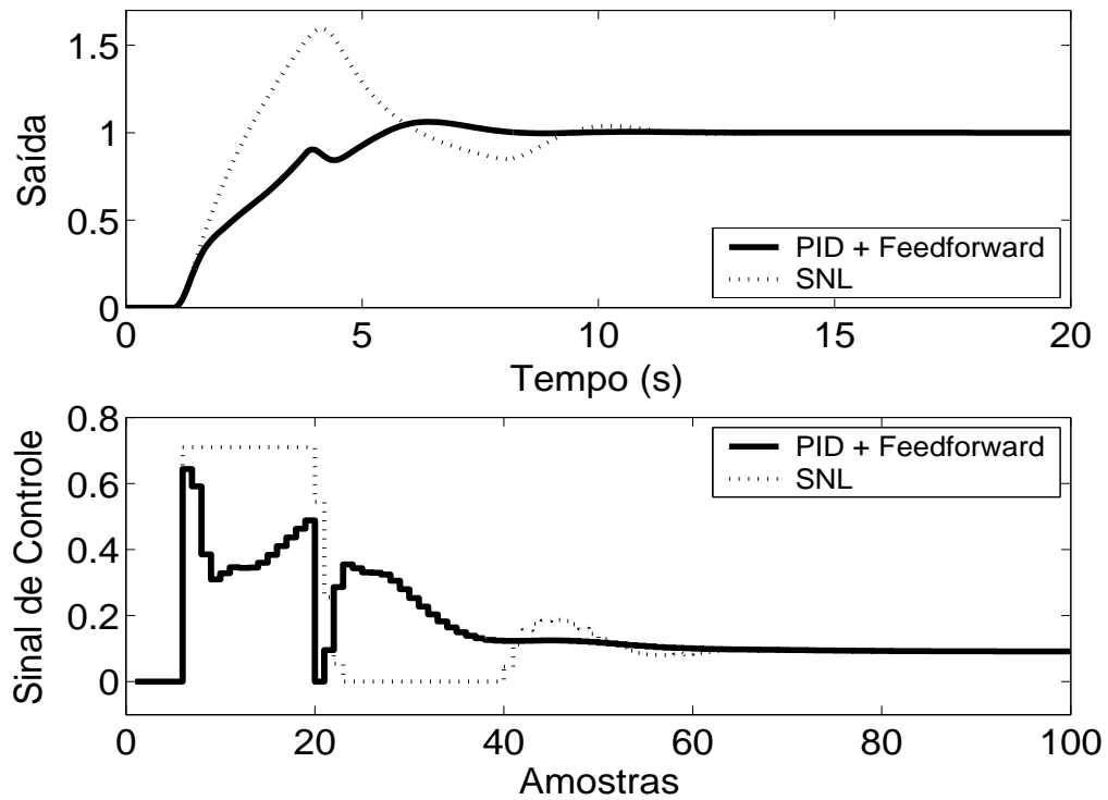
Figura 5.88: Saída e Sinal de Controle - Método PID + Feedforward com \tau = 2.8s e modelo de primeira ordem dado por (1 - 0.9899z^{-1})y(t) = z^{-1}0.1111u(t) .
