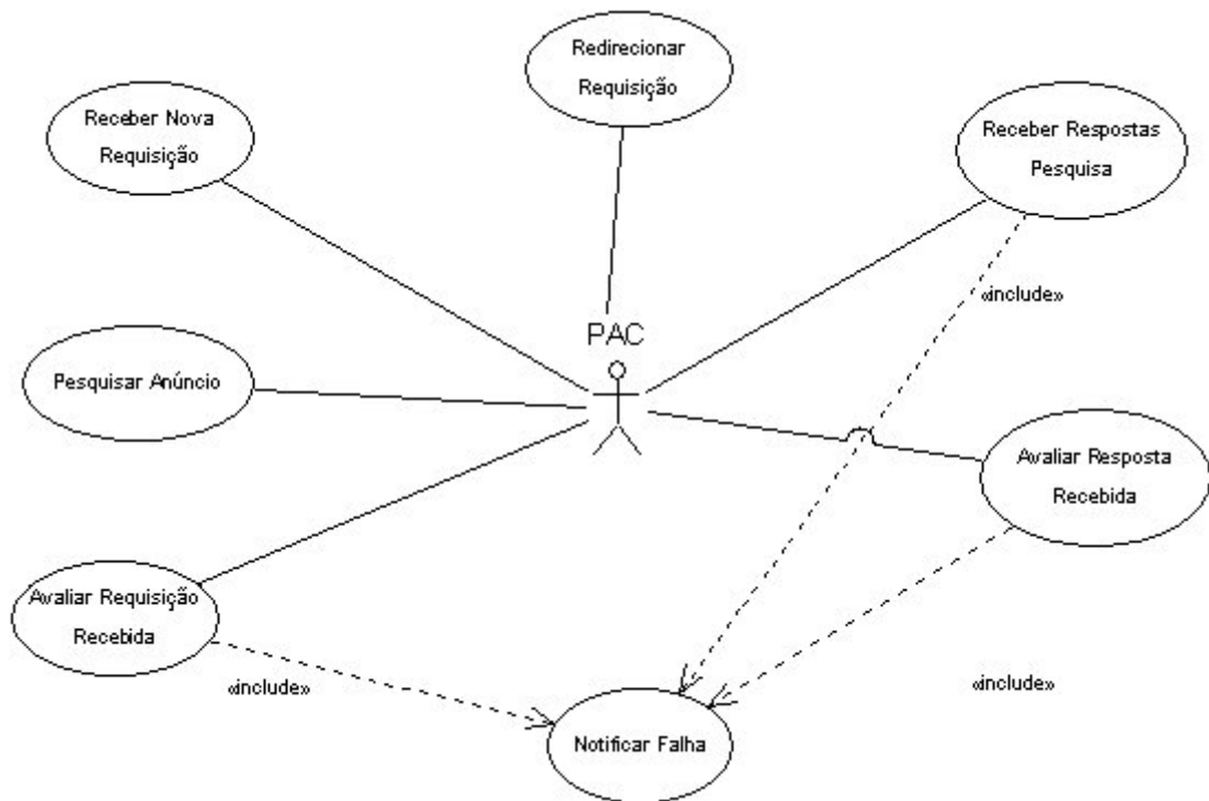
Figura 3.12 – Diagrama de Casos de Uso – PAC
