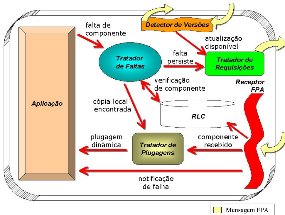
Figura 3.8 – Estrutura do Cliente FPA
