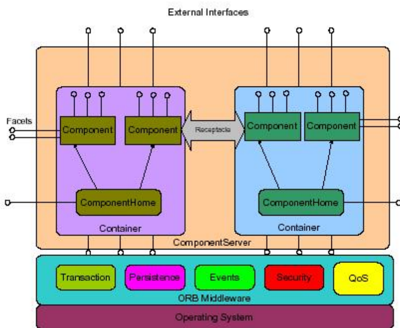
Figura 2.3 – Arquitetura CCM (Balasubramanian, 2002)
