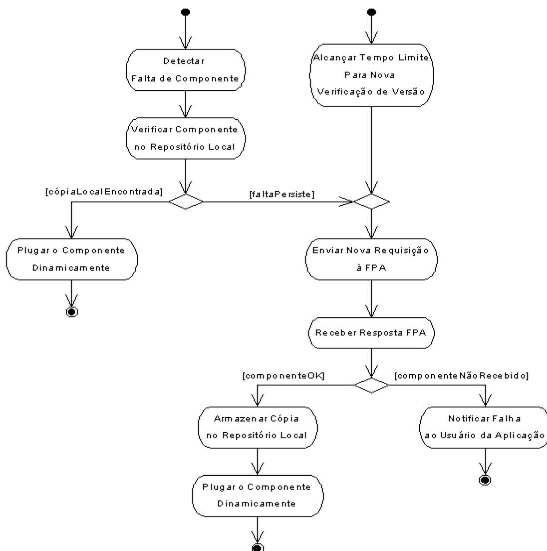
Figura 3.9 – Diagrama de Atividades do Cliente FPA
