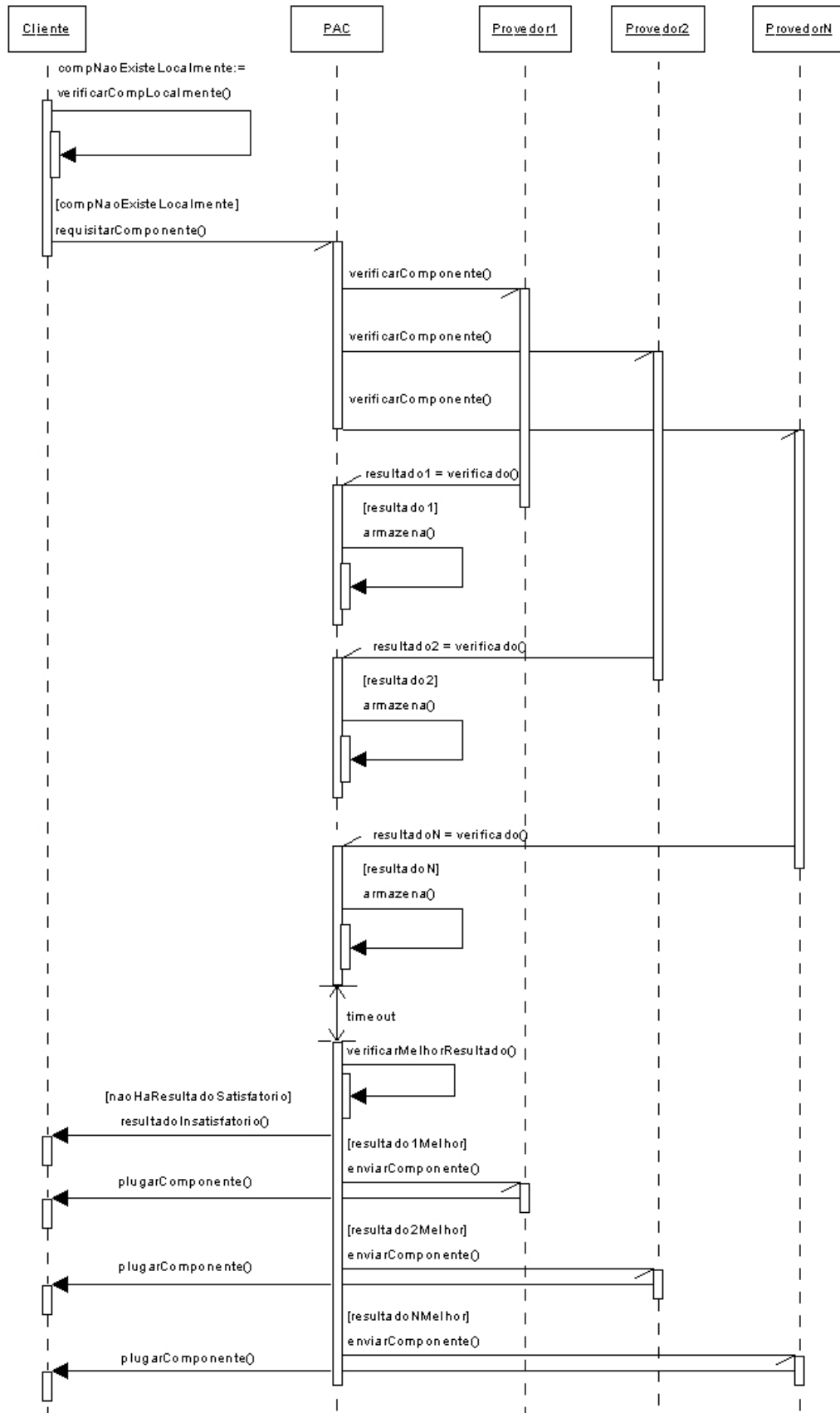
Figura 4.24 – Diagrama de Sequência – Plugagem Dinâmica
