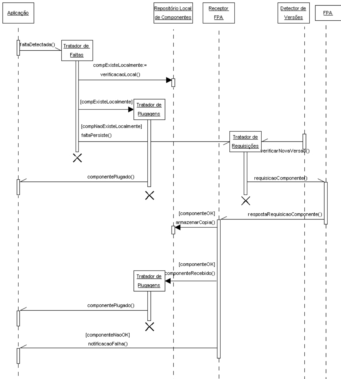
Figura 4.25 – Diagrama de Sequência – Cliente FPA
