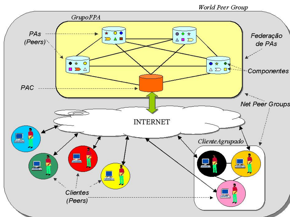
Figura 3.1 – A Federação de Provedores de Aplicação e seus Clientes
