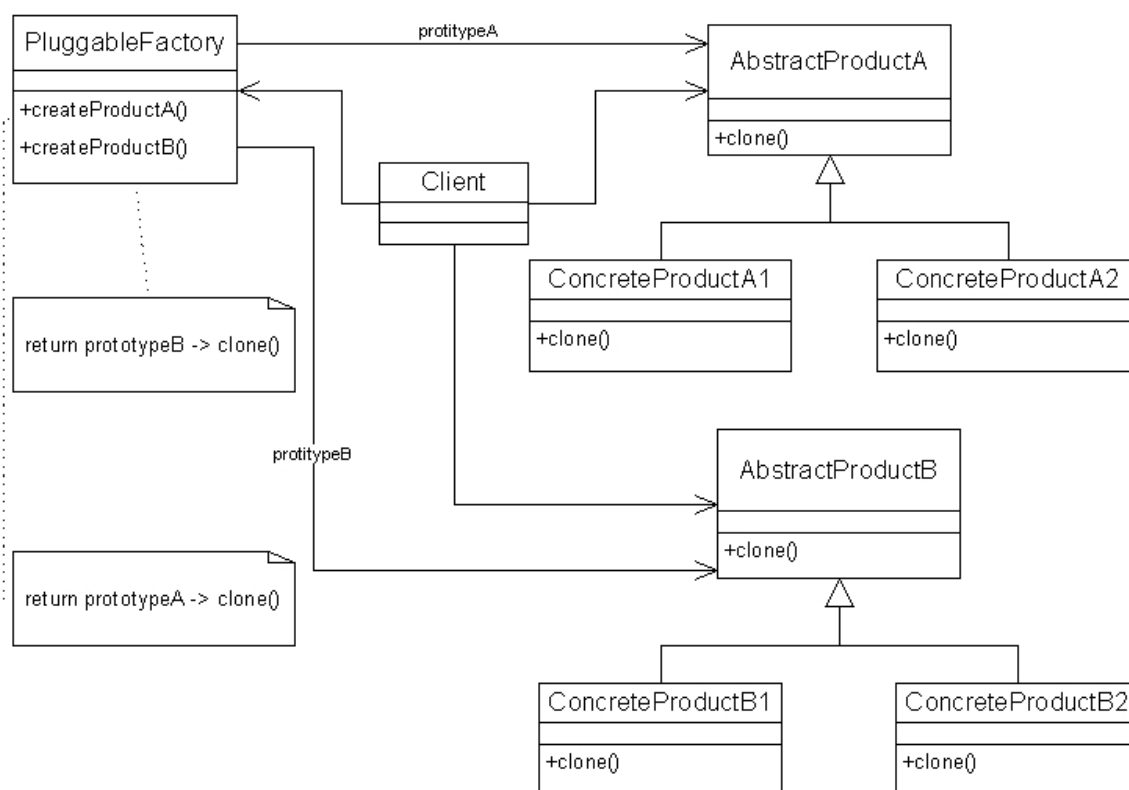
Figura 3.3 – Pluggable Factory em UML (Lauder, 1999)
