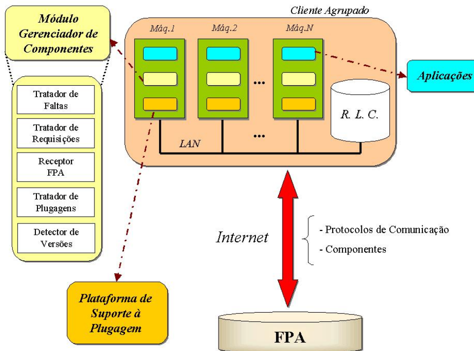
Figura 3.10 – O Cliente Agrupado
