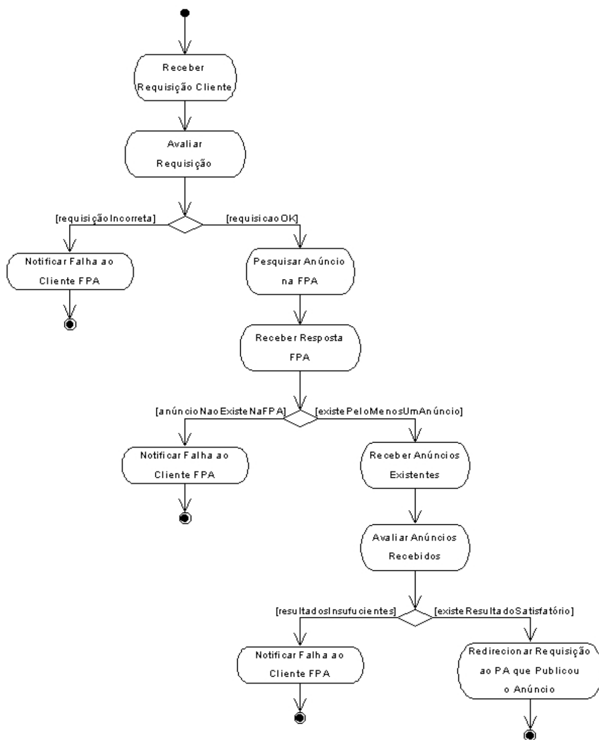
Figura 3.7 – Diagrama de Atividades do Provedor de Aplicação Coordenador
