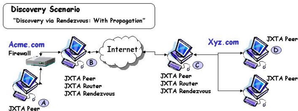
Figura 2.15 – Cenário JXTA – Descoberta com Propagação (JXTA, 2004c)
