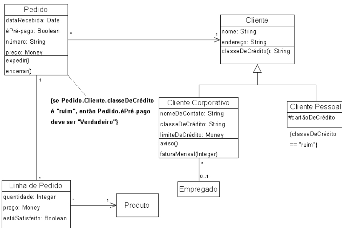
Figura 2.4 – Restrição / Constraint (Fowler et al. , 2000)
