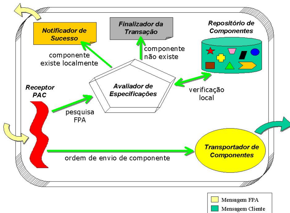
Figura 3.4 – Estrutura do Provedor de Aplicação
