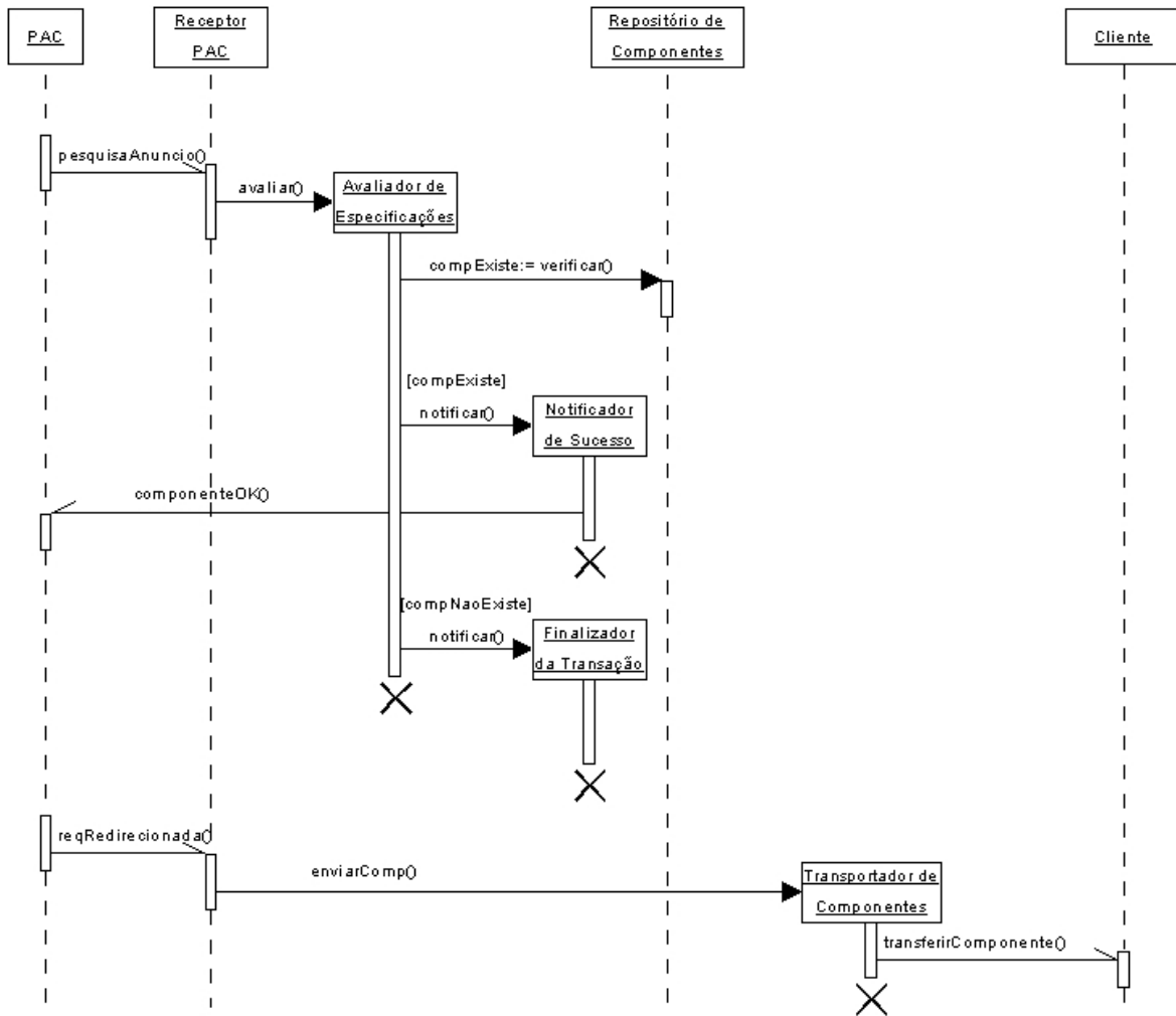
Figura 4.29 – Diagrama de Sequência – PA
