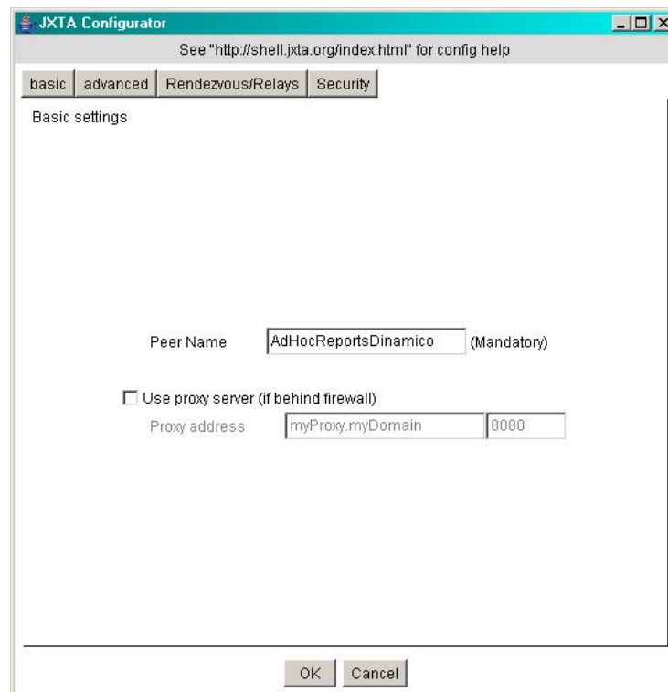
Figura 4.15 – Configuração Peer JXTA – Basic
