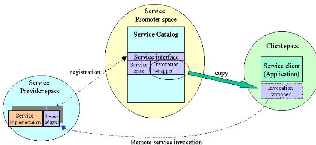
Figura 3.2 – O Catálogo de Serviços da FS (Garita et al. , 2002)
