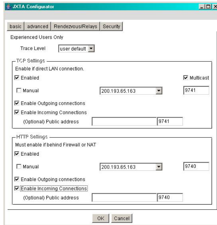
Figura 4.16 – Configuração Peer JXTA – Advanced
