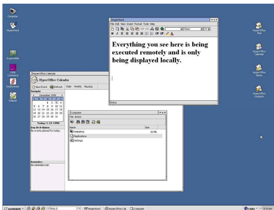
Figura 2.7 – WebOS (WebOS, 1998)
