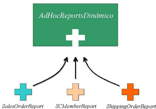
Figura 4.1 – Cenário Base
