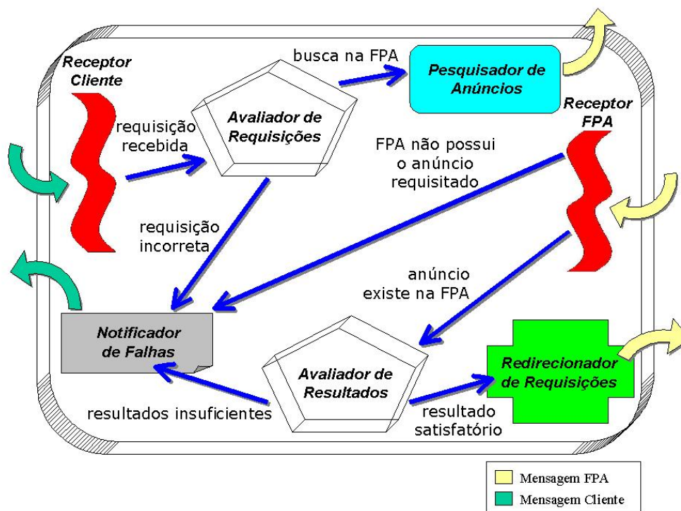
Figura 3.6 – Estrutura do Provedor de Aplicação Coordenador
