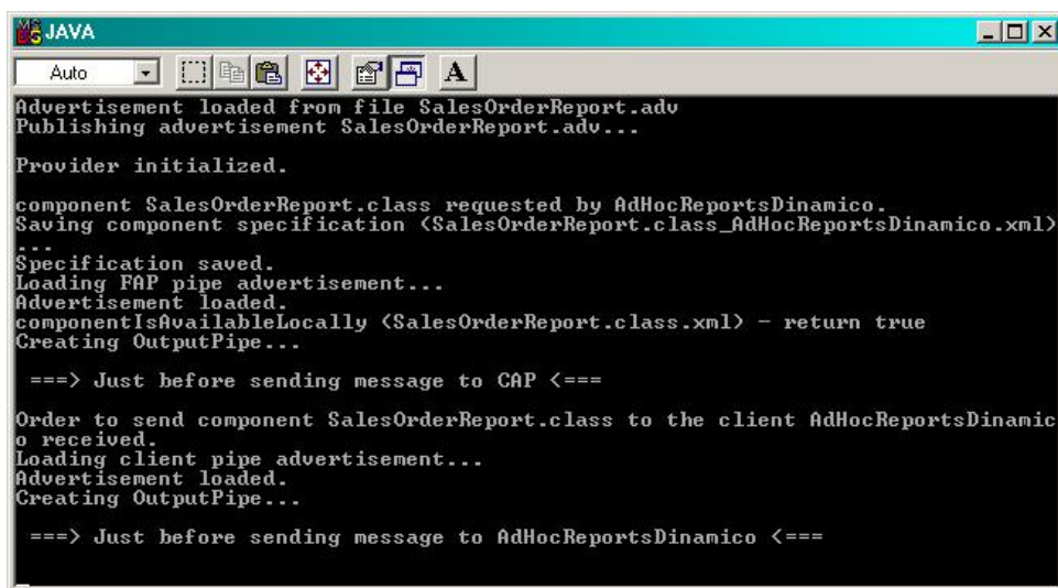
Figura 4.30 – Plugagem Dinâmica no PA
