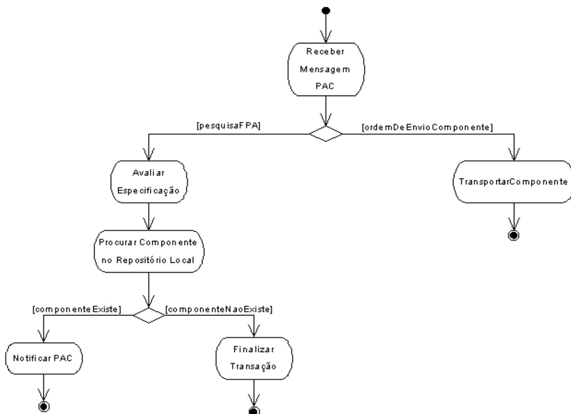
Figura 3.5 – Diagrama de Atividades do Provedor de Aplicação
