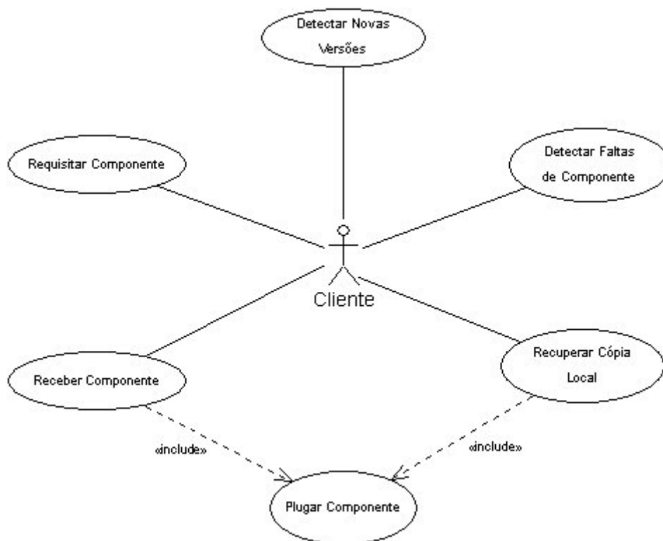
Figura 3.11 – Diagrama de Casos de Uso – Cliente FPA
