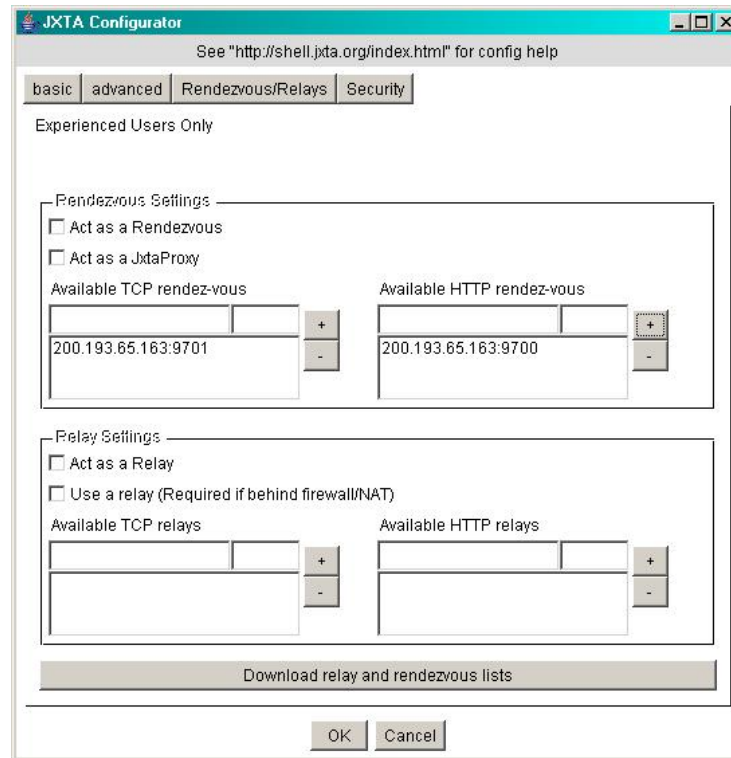
Figura 4.17 – Configuração Peer JXTA – Rendezvous / Relays
