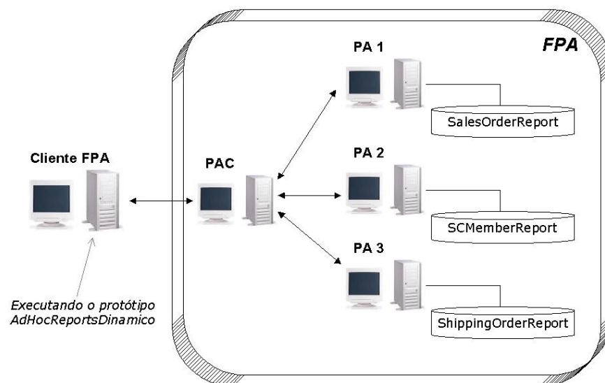
Figura 4.20 – Cenário do Fluxo de Execução
