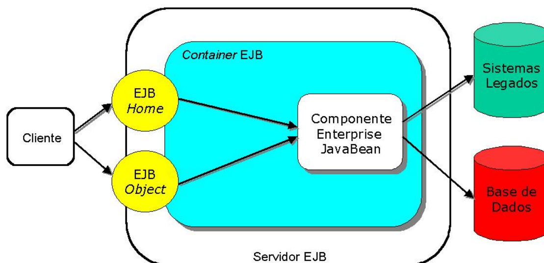
Figura 2.1 – Arquitetura EJB
