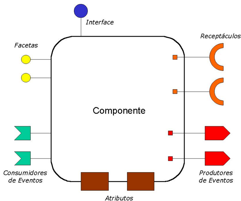
Figura 2.2 – Componente CCM
