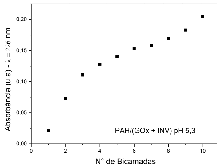
Figura 48: Crescimento do filme PAH/(GOx + INV) preparado em pH 5,3.
