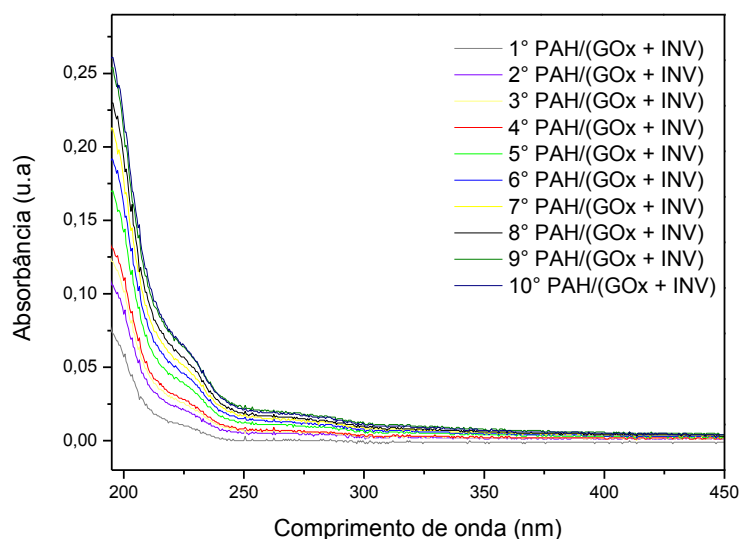
Figura 45: Espectros UV-vis do filme PAH/(GOx + INV) preparado em pH 6,3.
