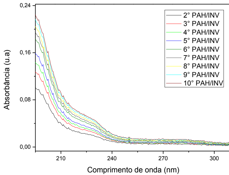
Figura 30: Espectros UV-vis do filme (PAH/INV) 10
