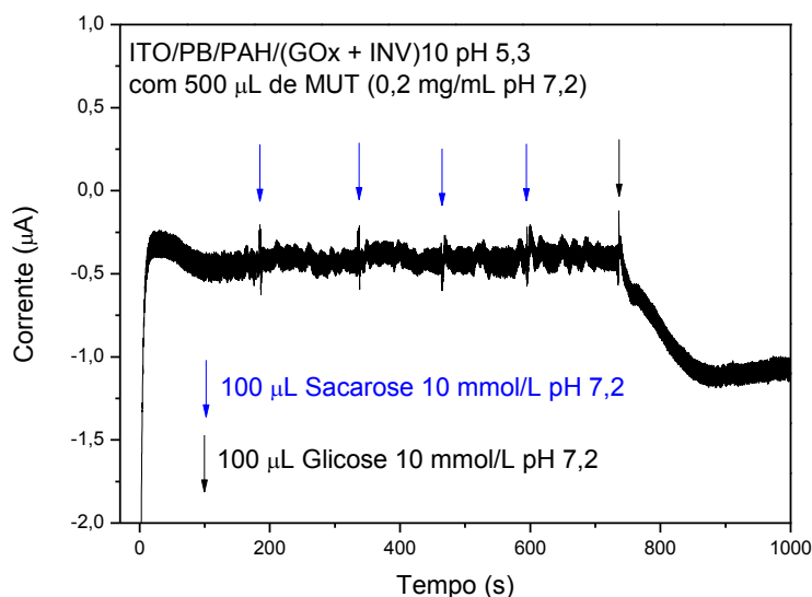
Figura 54: Resposta amperométrica (0,0 V vs ECS) de ITO/PB/PAH/(GOx + INV) 10 pH 5,3 com 500 µL de MUT 0,2 mg/mL pH 7, 2 em solução. Eletrólito: Tampão fosfato 10 mmol/L pH 7,2.
