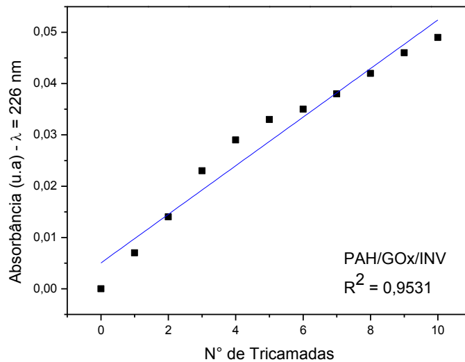
Figura 44: Crescimento do filme PAH/GOx/INV em 226 nm.
