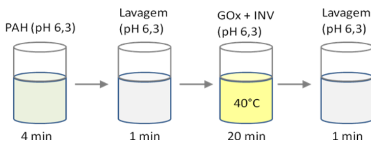
Figura 16: Sequência de deposição do filme PAH/(GOx + INV) pH 6,3.
