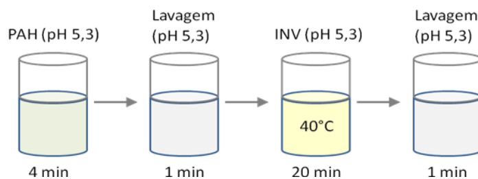
Figura 12: Sequência de deposição do filme PAH/INV.
