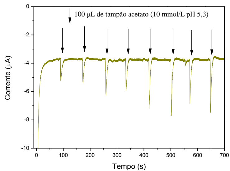
Figura 35: Curva amperométrica de ITO/PB/(PAH/INV) 10 (0,0 V vs ECS) mediante adições de tampão acetato pH 5,3 10 mmol/L
