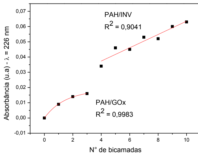
Figura 42: Crescimento do filme (\text{PAH/GOx})_3/(\text{PAH/INV})_7 para \lambda = 226 nm.
