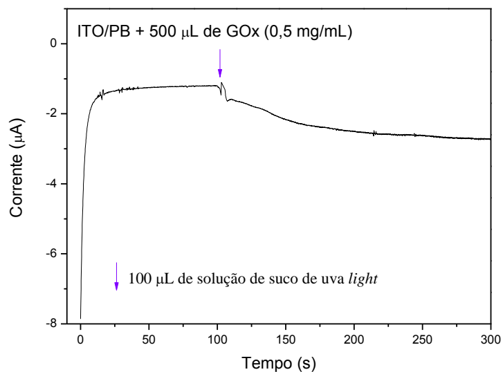
Figura 60: Resposta amperométrica (0,0 V vs ECS) de ITO/PB com 500 µL de GOx 0,5 mg/mL em solução. Adições de solução de suco de uva light .
