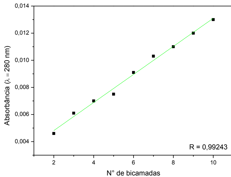
Figura 31: Absorbância em função do número de bicamadas do filme (PAH/INV) 10
