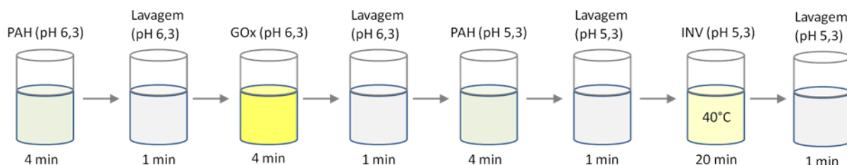
Figura 13: Sequência de deposição do filme PAH/GOx/PAH/INV.
