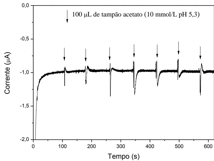
Figura 34: Curva amperométrica de ITO/PB/(PAH/INV) 10 (0,0 V vs ECS) com 500 µL de GOx 0,5 mg/mL pH 5,3 em solução.
