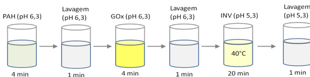
Figura 15: Sequência de deposição do filme PAH/GOx/INV.
