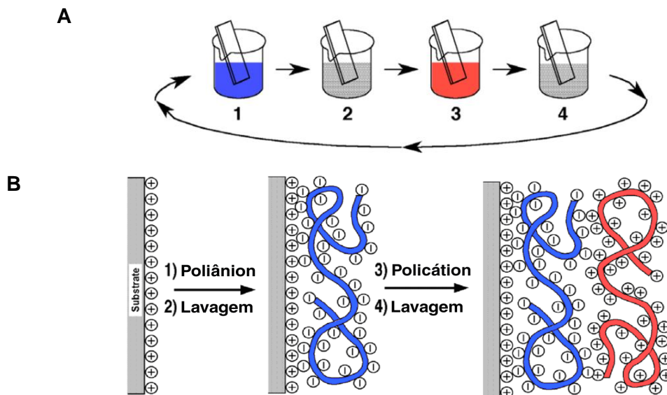
Figura 1: (A) Representação esquemática do processo de deposição do filme LbL sobre um substrato sólido. As etapas 1 e 3 representam a adsorção dos polieletrólitos aniônico e catiônico, respectivamente, e as etapas 2 e 4 são os procedimentos de lavagem. No fim da etapa 4 tem-se a construção de um filme do tipo (A/B) n . (B) Estrutura idealizada do filme LbL contendo as duas primeiras etapas de adsorção dos polieletrólitos. Figura extraída da referência [4].
