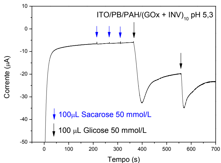
Figura 52: Resposta amperométrica (0,0 V vs ECS) do sistema ITO/PB/PAH/(GOx + INV) 10 em pH 5,3 mediante adições de glicose e sacarose.
