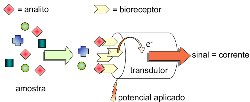
Figura 3: Representação esquemática do funcionamento de um biossensor amperométrico. Figura extraída de [29].
