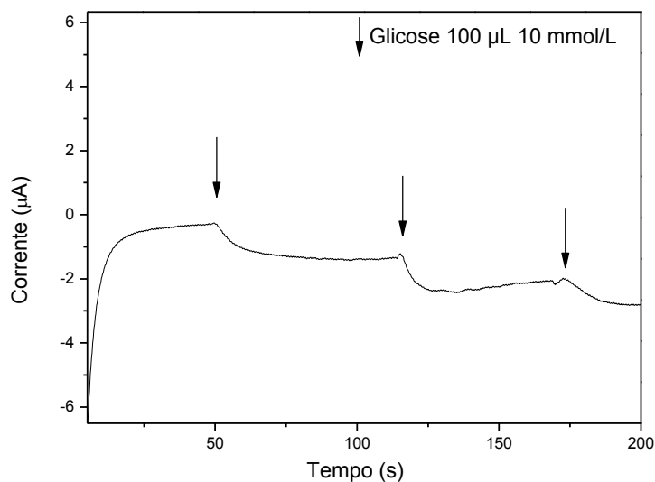
Figura 27: Curva amperométrica de ITO/PB/(PAH/GOx) 10 0,0 V vs ECS mediante adições de glicose.
