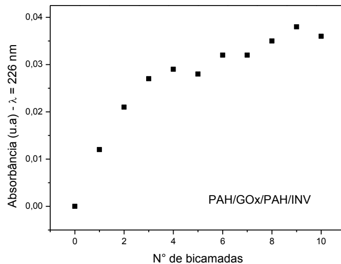
Figura 38: Crescimento do filme (PAH/GOx/PAH/INV) 10 em \lambda = 226 nm.
