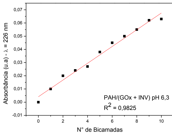
Figura 46: Crescimento do filme PAH/(GOx + INV) preparado em pH 6,3.
