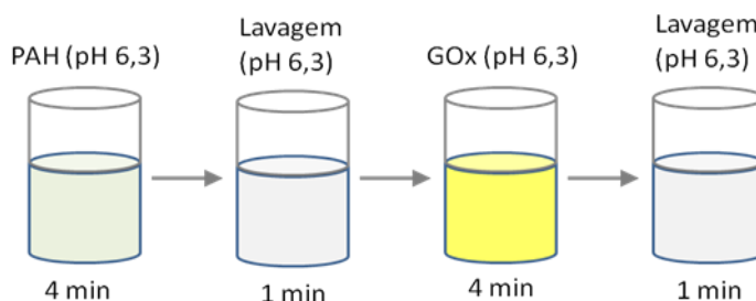
Figura 11: Sequência de deposição do filme PAH/GOx.
