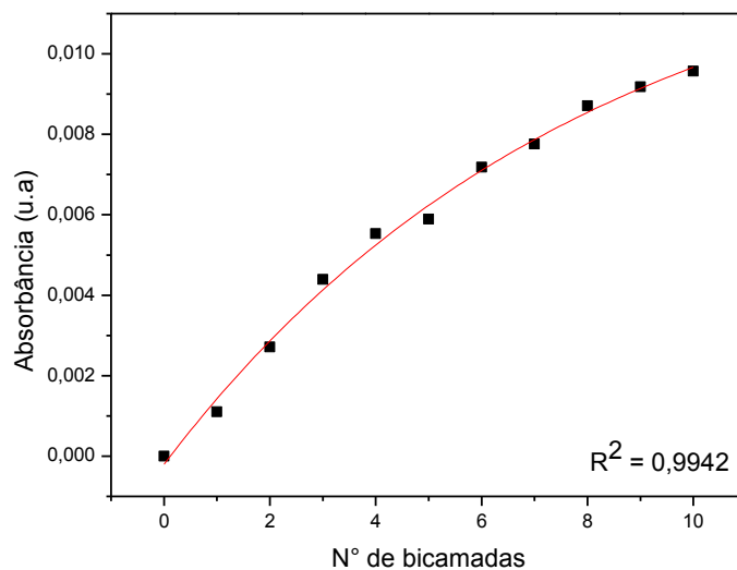
Figura 26: Absorbância em função do número de bicamadas do filme (PAH/GOx) 10 em \lambda = 250 nm.
