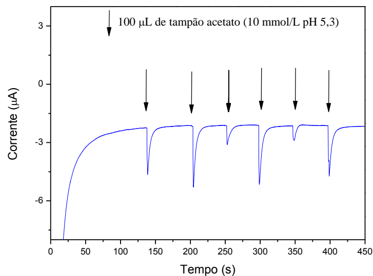
Figura 36: Curva amperométrica de ITO/PB mediante a adição de tampão acetato pH 5,3 10 mmol/L.
