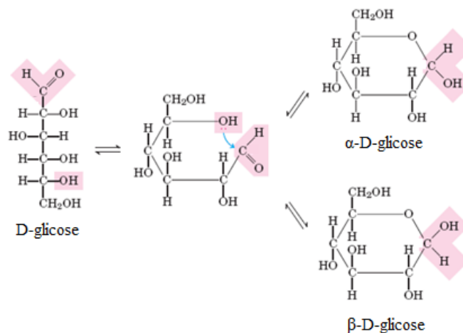
Figura 10: Ilustração das formas cíclicas \alpha e \beta da D-glicose. Figura adaptada da referência [33].
