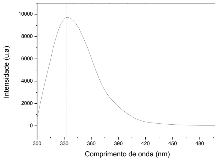
Figura 24: Espectro de fluorescência da solução INV 0,5 mg/mL (pH 5,3). Banda em 333 nm.
