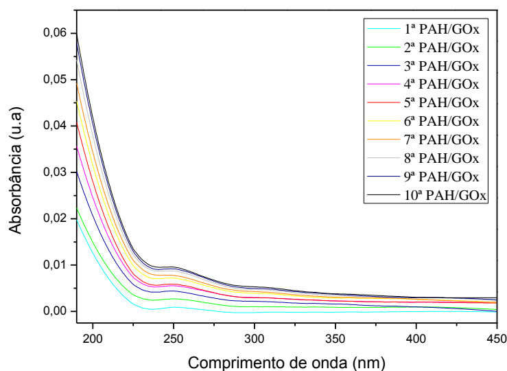
Figura 25: Espectro de absorção por camada do filme (PAH/GOx) 10 .
