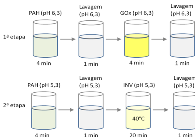
Figura 14: Sequência de deposição do filme (PAH/GOx)/(PAH/INV).
