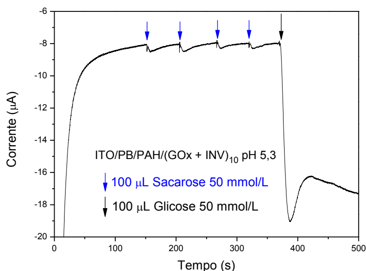
Figura 53: Resposta amperométrica (0,0 V vs ECS) do sistema ITO/PB/PAH/(GOx + INV) 10 em pH 5,3. Solução da mistura: GOx (5 mg/mL) e INV (1 mg/mL).
