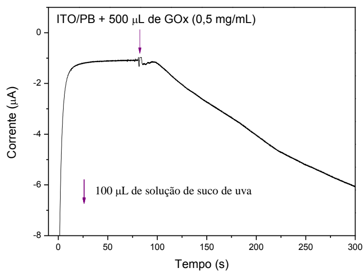
Figura 57: Resposta amperométrica (0,0 V vs ECS) de ITO/PB com 500 μL de GOx 0,5 mg/mL pH 5,3 em solução. Adição de solução de suco de uva.
