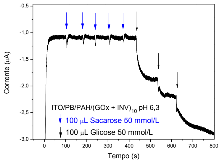
Figura 51: Resposta amperométrica (0,0 V vs ECS) do sistema ITO/PB/PAH/(GOx + INV) 10 em pH 6,3 mediante adições de glicose e sacarose.
