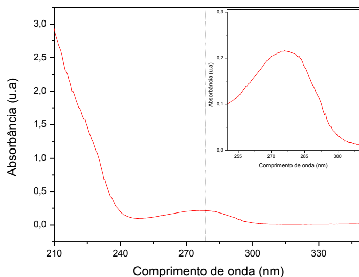
Figura 21: Espectro UV-vis da solução de GOx 2mg/mL (pH 6,3). Inset : Banda em 278 nm.
