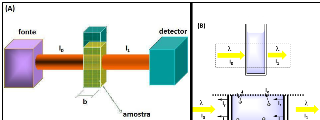
Figura 18: (A) Esquema de um espectrômetro de UV-vis: uma fonte de luz monocromática incide um feixe de intensidade I_0 . O detector recebe um feixe de intensidade I_1 . (B) Esquema de uma cubeta recebendo um feixe de intensidade I_0 , que é espalhada devido à reflexão nas paredes da cubeta e absorvida pelas moléculas, chegando um feixe de intensidade I_1 ao detector.
