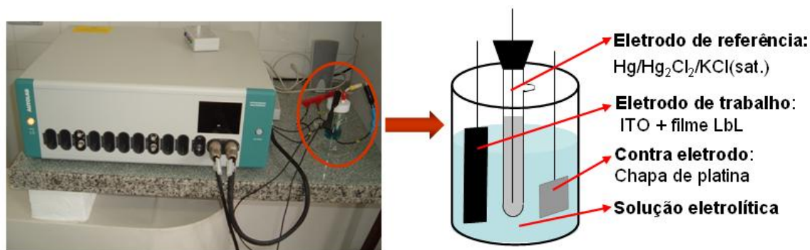
Figura 19: Representação de uma célula eletroquímica acoplada a um potenciostato. Célula convencional de três eletrodos: trabalho, contra-eletrodo e eletrodo de referência.
