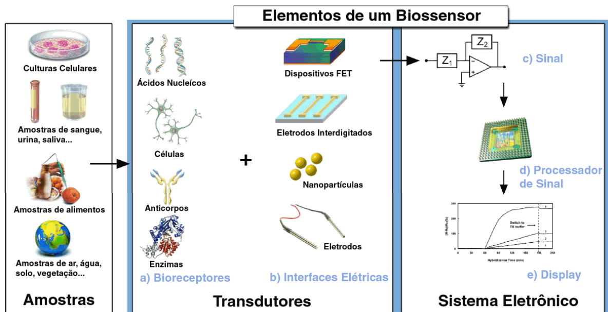
Figura 2: Elementos e componentes de um típico biossensor. Figura adaptada de Grieshaber e colaboradores [6].
