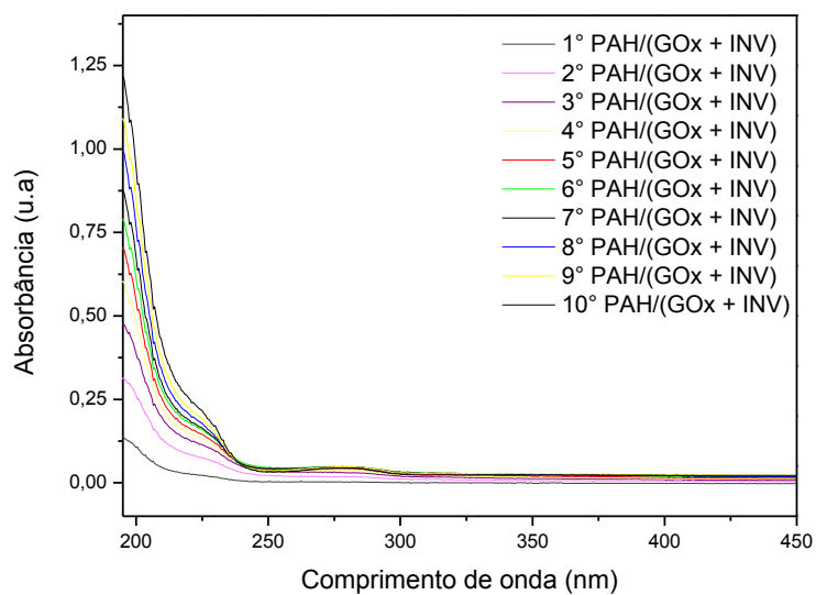
Figura 47: Espectros UV-vis do filme PAH/(GOx + INV) preparado em pH 5,3.
