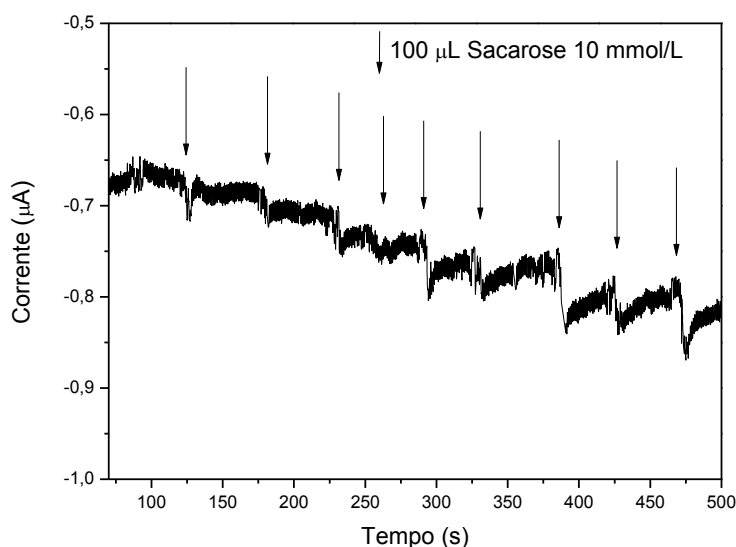
Figura 32: Curva amperométrica de ITO/PB/(PAH/INV) 10 (0,0 V vs ECS) com 500 \mu L de GOx em solução mediante adições sucessivas de sacarose.
