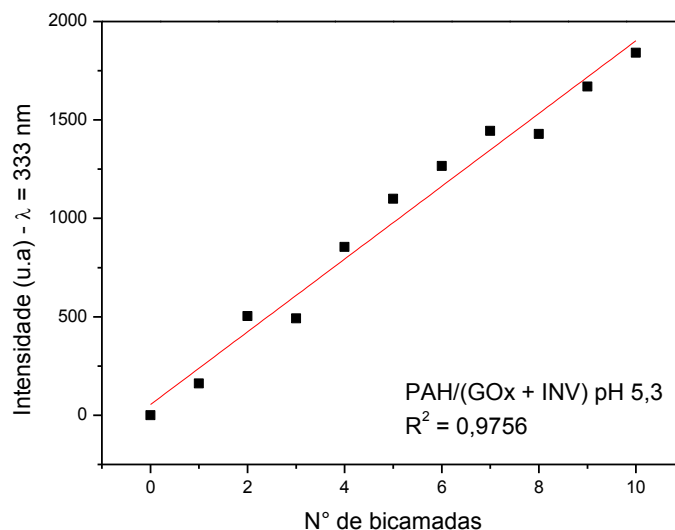
Figura 50: Crescimento por fluorescência do filme PAH/(GOx + INV) preparado em pH 5,3.
