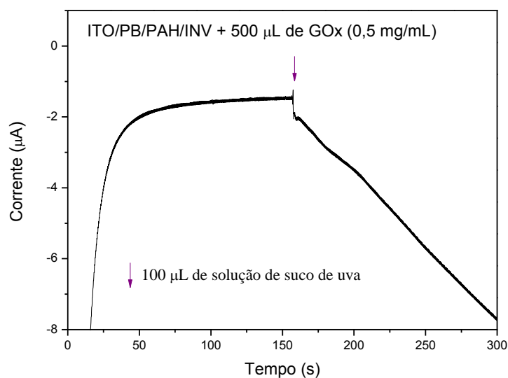
Figura 56: Resposta amperométrica (0,0 V vs ECS) de ITO/PB/(PAH/INV) 10 com 500 \mu\text{L} de GOx 0,5 mg/mL pH 5,3 em solução. Adições de solução de suco de uva.
