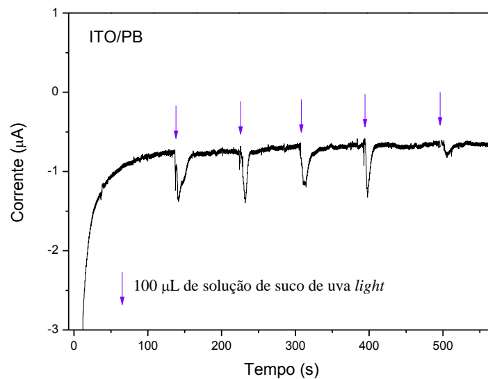
Figura 61: Resposta amperométrica (0,0 V vs ECS) ITO/PB sem GOx. Adições de solução de suco de uva light .
