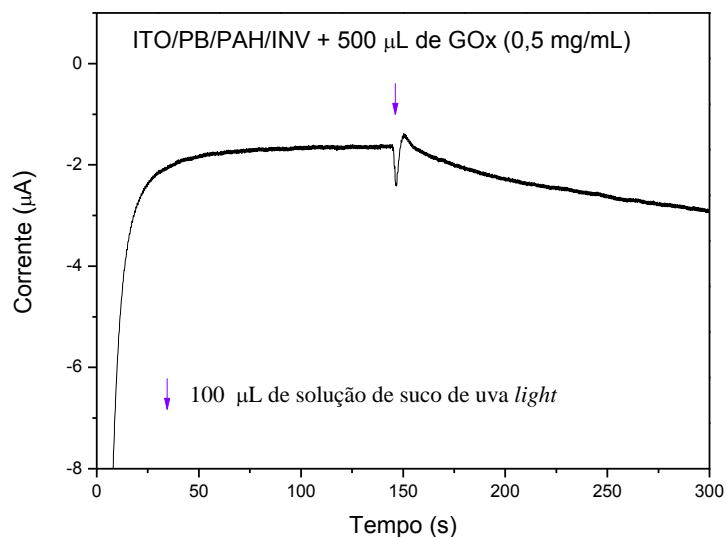
Figura 59: Resposta amperométrica (0,0 V vs ECS) de ITO/PB/(PAH/INV) 10 com 500 µL de GOx 0,5 mg/mL em solução. Adições de solução de suco de uva light .
