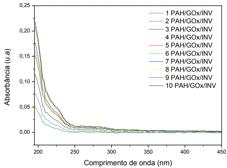
Figura 43: Espectros UV-vis do filme PAH/GOx/INV.
