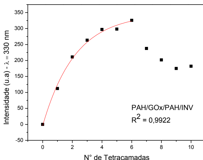
Figura 40: Crescimento do filme PAH/GOx/PAH/INV analisado por espectroscopia de fluorescência.
