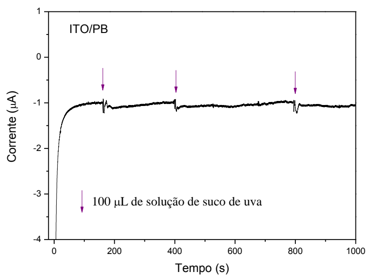
Figura 58: Resposta amperométrica (0,0 V vs ECS) de ITO/PB sem GOx. Adições de solução de suco de uva.
