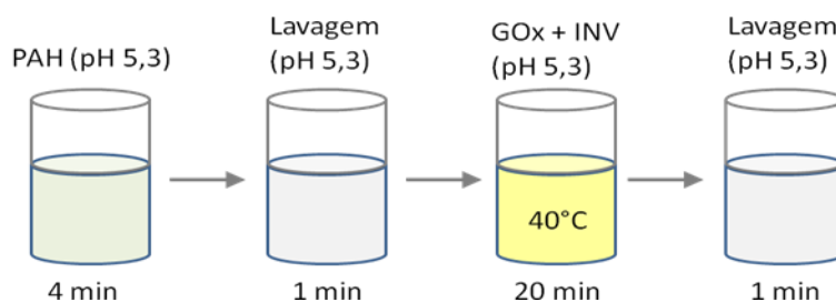
Figura 17: Sequência de deposição do filme PAH/(GOx + INV) pH 5,3.
