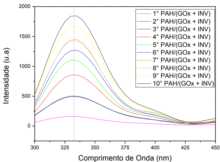
Figura 49: Espectros de emissão do filme PAH/(GOx + INV) preparado em pH 5,3. Excitação em 280 nm e banda de emissão em 333 nm.
