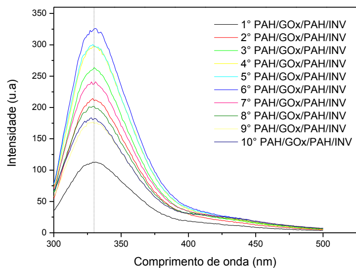
Figura 39: Espectros de fluorescência do filme PAH/GOx/PAH/INV. Banda em 330 nm.
