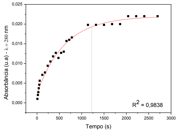
Figura 29: Cinética de crescimento na deposição PAH (3min)/ INV (tempos variáveis), para \lambda = 280 nm. Tempo ideal de deposição a partir de 20 min (1200 s).
