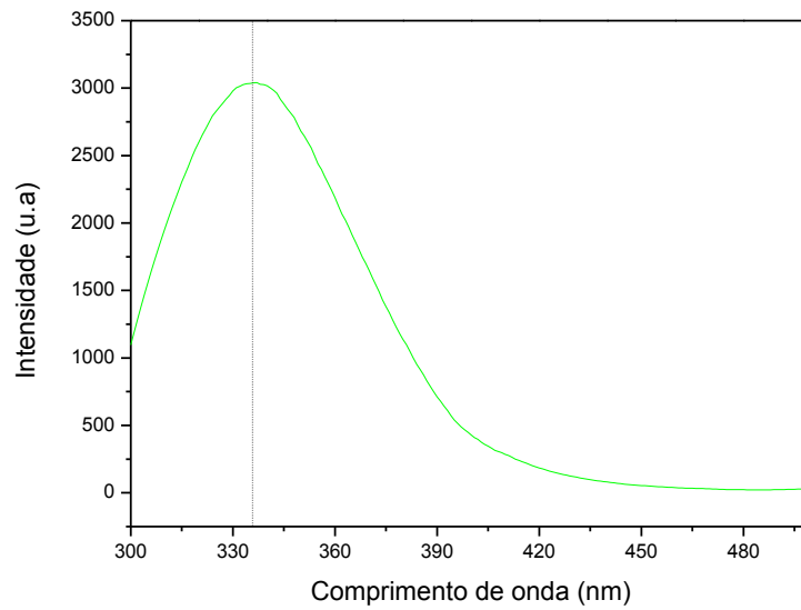
Figura 23: Espectro de fluorescência da solução GOx 2mg/mL (pH 6,3). Banda em 336 nm.
