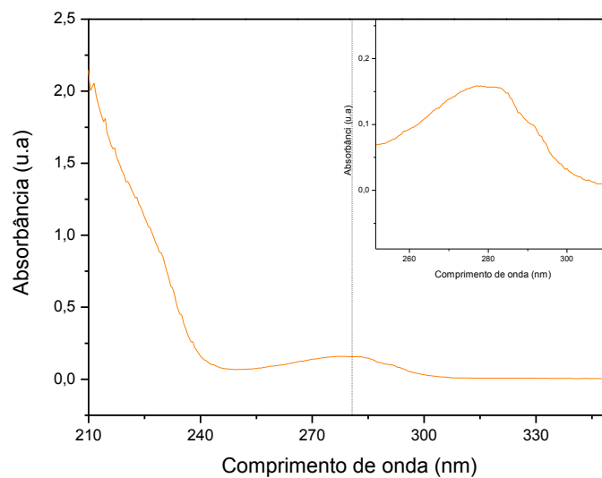
Figura 22: Espectro UV-vis da solução de INV 0,5 mg/mL (pH 5,3). Inset : Banda em 280 nm.
