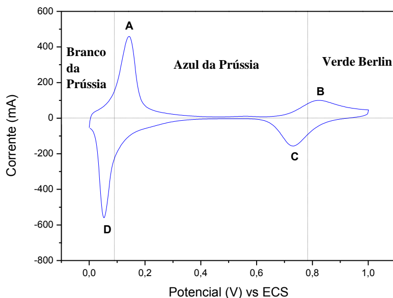
Figura 20: Voltamograma cíclico do eletrodo ITO/PB de 0,0 V a 1,0 V ( vs ECS) – 50 mV/s após 20 ciclos.
