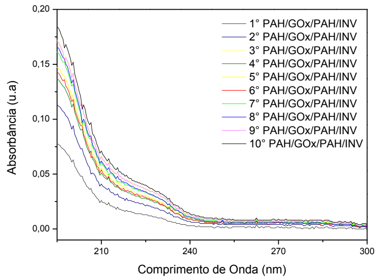
Figura 37: Espectros UV-vis do filme (PAH/GOx/PAH/INV) 10 .
