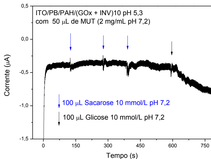
Figura 55: Resposta amperométrica (0,0 V vs ECS) de ITO/PB/PAH/(GOx + INV) 10 pH 5,3 com 50 µL de MUT 2 mg/mL pH 7,2 em solução. Solução eletrolítica: Tampão fosfato 10 mmol/L pH 7,2.
