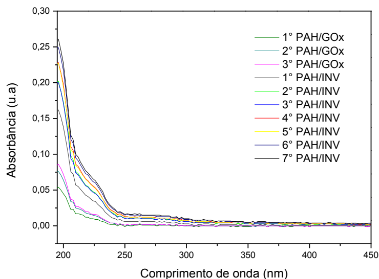
Figura 41: Espectros UV-vis do filme (PAH/GOx) 3 /(PAH/INV) 7 .
