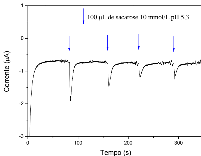
Figura 33: Curva amperométrica de ITO/PB (0,0 V vs ECS) com 500 µL de GOx 0,5 mg/mL em pH 5,3 na solução eletrolítica mediante adições de sacarose.
