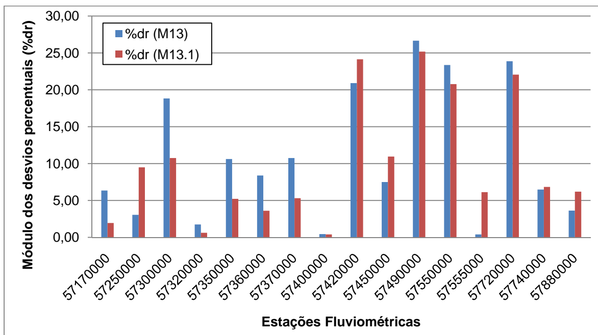
Figura 29 - Gráfico de barras representativo dos módulos dos erros percentuais (%dr) para os modelos M13 e M13.1 da sub-região SR2
