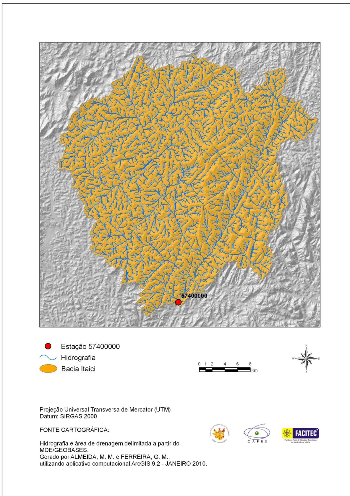
Figura 8 - Delimitação da bacia da estação Itaici, gerada a partir do MDE/GEOPORTAL
