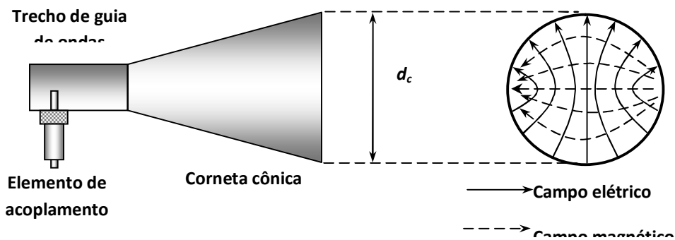
Figura 3.12 6 Ilustração de uma corneta cônica, frequentemente empregada em radares para medição de nível. Estão indicadas também as distribuições de campo elétrico e magnético supondo a posição fixada para o elemento de acoplamento.
