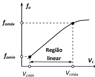
Figura 3.5 6 Comportamento típico dos valores da freqüência de saída de um oscilador controlado por tensão, com destaque para a região linear.
