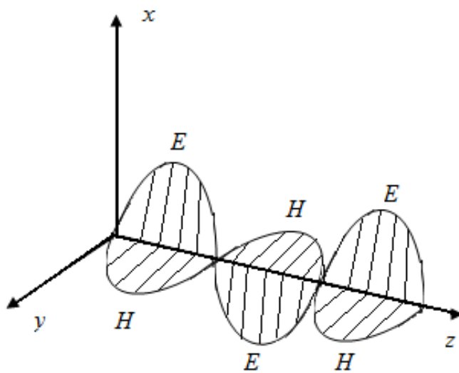
Figura 3.1 o Campo elétrico e campo magnético de uma onda propagando-se na direção z . Suas direções são tais que formam um sistema dextrógiro.
