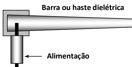
Figura 3.15 Esboço de uma antena de barra ou haste dielétrica para operação em microondas
