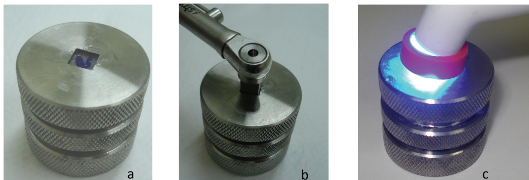
Figura 11 – Cimentação: a) dispositivo metálico com o dente e a cerâmica já cimentada; b) torquímetro aplicando carga equivalente à 750g; c) fotopolimerização.
