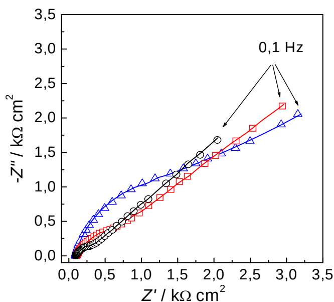
Figura 27. Espectros no plano complexo para os eletrodos de GC ( \Delta ), GC/MWCNT ( \square ) e GC/MWCNT/CoPc ( \circ ), em solução de tampão acetato 0,1 \text{ mol L}^{-1} (pH 4.0) contendo 1,0 \times 10^{-4} \text{ mol L}^{-1} de carbaril.
