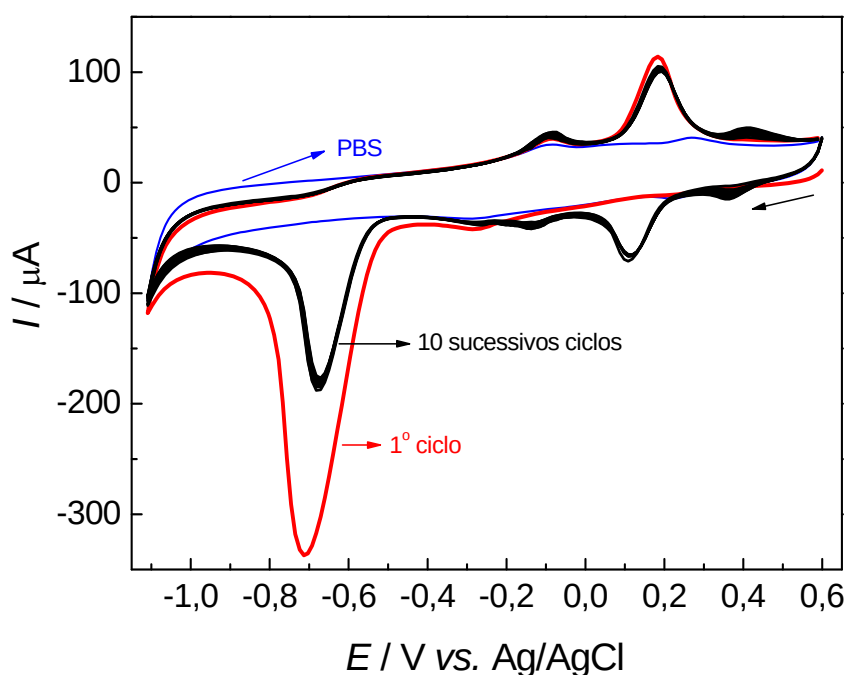
Figura 17. Voltamogramas cíclicos sucessivos na presença de 1,0 \text{ mmol L}^{-1} de 4-NP em meio de PBS ( \text{pH} = 6,0 ). (—) PBS na ausência de 4-NP, (—) primeiro ciclo e (—) nove sucessivos ciclos.
