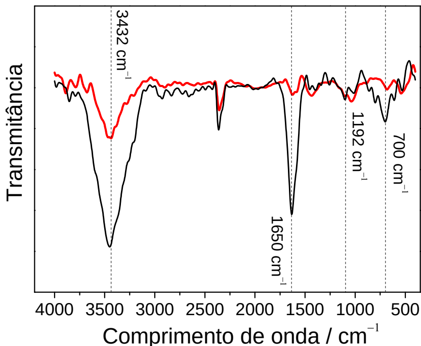
Figura 13. Espectros de FTIR para os CNTs não funcionalizados (—) e CNTs funcionalizados (—).
