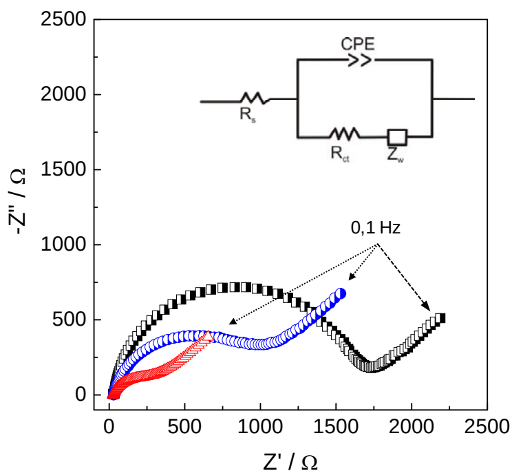
Figura 15. Diagramas de Nyquist para os eletrodos: GC (■), CNTs não funcionalizado (●) e CNTs funcionalizados (▲), na presença de 5,0 \text{ mmol L}^{-1} de \text{K}_3[\text{Fe}(\text{CN})_6] . Detalhe: circuito de Randles modificado.
