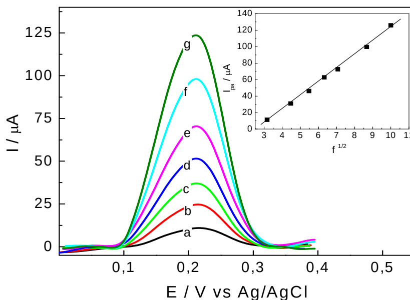
Figura 22. Efeito da frequência nos voltamogramas de SWV na detecção de 4-NP: Frequências: (a) 10; (b) 20; (b) 30; (d) 40; (e) 50; (f) 75 e (g) 100 Hz. Detalhe: dependência linear do pico de corrente com a raiz quadrada da frequência.
