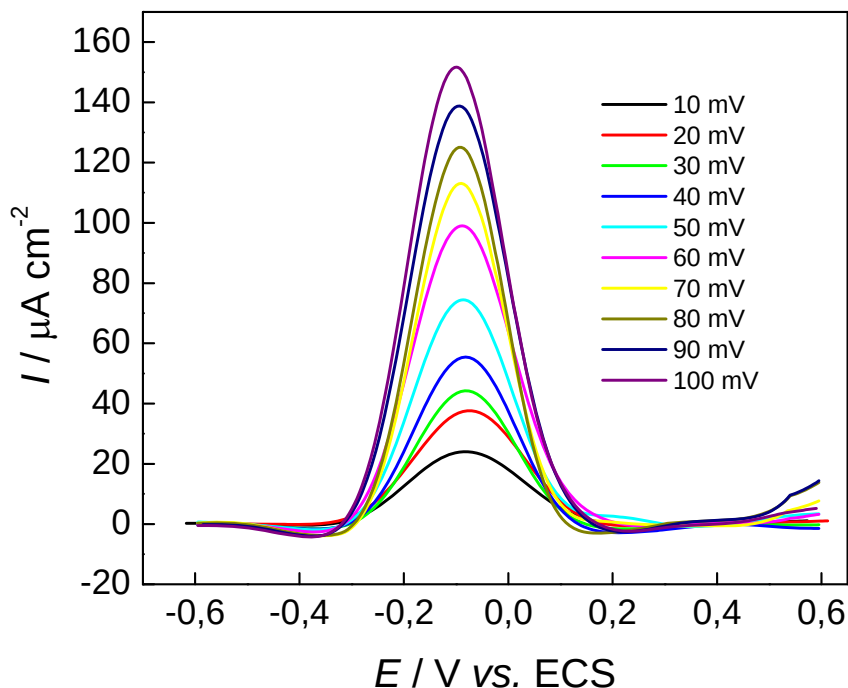
Figura 38. Estudo da amplitude de pulso na técnica de DPV para o eletrodo de GC/MWCNT/CuPc, em solução tampão fosfato 0.1 mol L -1 (pH 7.5) contendo 1.0 mmol L -1 de glifosato, com amplitude de pulso variando no intervalo de 10 a 100 mV.
