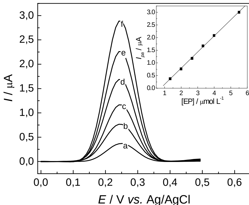
Figura 54. Curva analítica utilizando DPV com eletrodo composto Parafina/MWCNT/CoPc com os parâmetros otimizados para as seguintes concentrações de epinefrina em \mu mol L^{-1} : (a) 1,33; (b) 1,99; (c) 2,66; (d) 3,33; (e) 3,99 e (f) 5,50. Detalhe: dependência linear do pico de corrente com a concentração de epinefrina.
