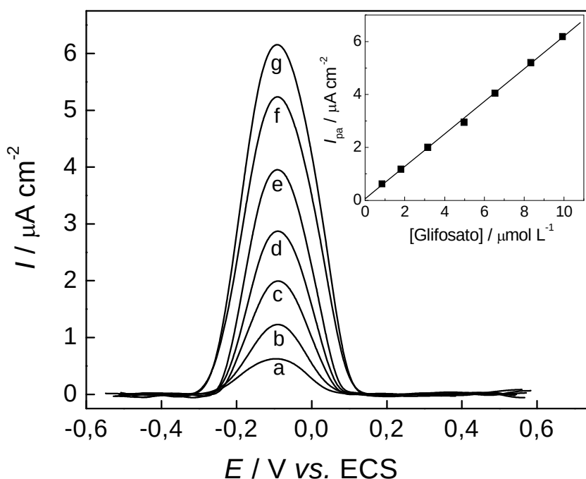
Figura 39. Curva analítica utilizando DPV com eletrodo de GC/MWCNT/CuPc com os parâmetros otimizados para as seguintes concentrações de glifosato em \mu\text{mol L}^{-1} : (a) 0,83; (b) 1,66; (c) 3,32, (d) 4,97; (e) 6,62, (f) 8,26 e (g) 9,90. Detalhe: dependência linear do pico de corrente com a concentração de glifosato.
