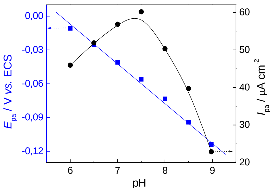
Figura 33. Gráfico da relação linear entre a variação de pH vs. E_{pa} (■) e pH vs. I_{pa} (●), em meio 0,1 mol L -1 PBS contendo 1,0 mmol L -1 de Gli.
