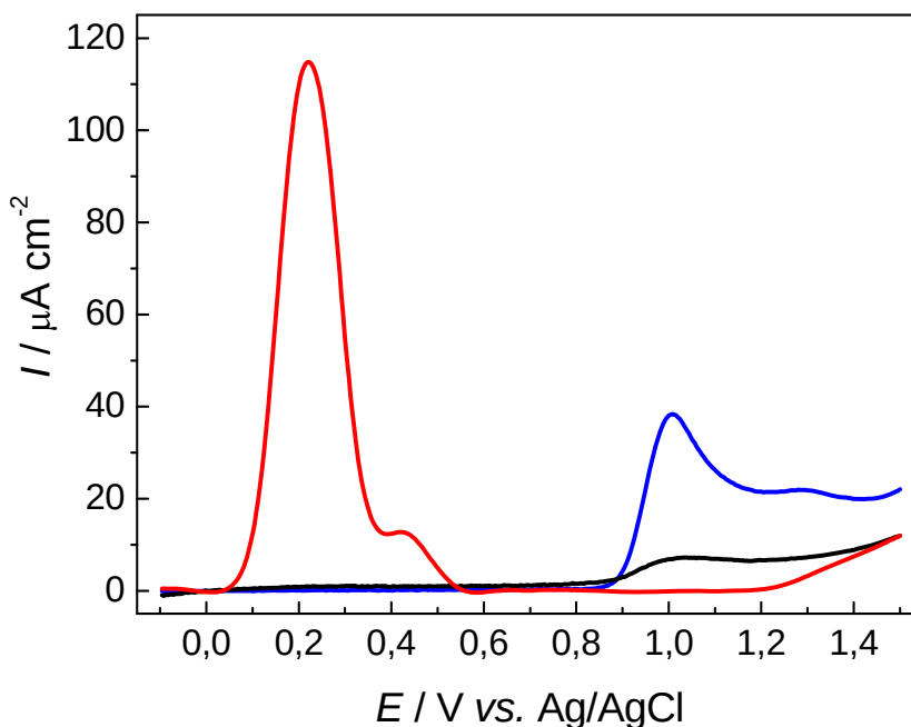
Figura 20. Voltametria de varredura linear para os eletrodos de GC (—), BDD (—) e GC/MWCNT (—) em PBS 0,2 mol L -1 (pH 6,0) contendo de 1.0 mmol L -1 de 4-NP, com \nu = 50 \text{ mV s}^{-1} .
