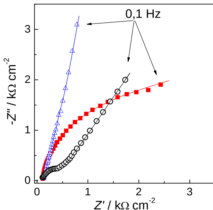
Figura 36. Espectros no plano complexo para os eletrodos de GC/MWCNT/CuPc, nas seguintes situações: a) 0,1 mol L -1 de PBS (pH 7,5) ( \Delta ); b) 0,1 mol L -1 de PBS (pH 7,5) contendo 1,0 mmol L -1 de Gli ( \blacksquare ) e c) 0,1 mol L -1 de PBS (pH 7,5) após dez sucessivos voltamogramas cíclicos em solução contendo 1,0 mmol L -1 de Gli ( \circ ).
