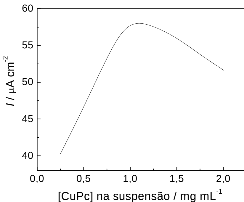
Figura 37. Relação entre a concentração de CuPc na suspensão de MWCNT e o pico de corrente de oxidação de 1,0 mmol L -1 de Gli, em meio PBS pH 7,5.
