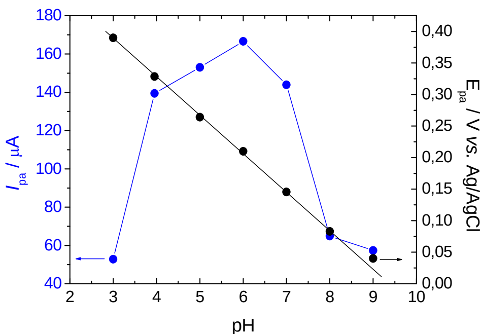
Figura 21. Gráfico da relação linear entre a variação de pH vs. E_{pa} (●) e pH vs. I_{pa} (●), em um meio 0,2 \text{ mol L}^{-1} PBS contendo 1,0 \text{ mmol L}^{-1} de 4-NP.
