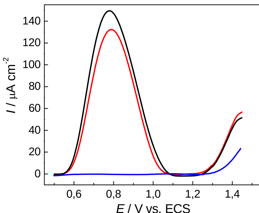
Figura 26. Componentes da corrente da SWV para o eletrodo de GC/MWCNT/CoPc: total (—); direta (—) e reversa (—).
