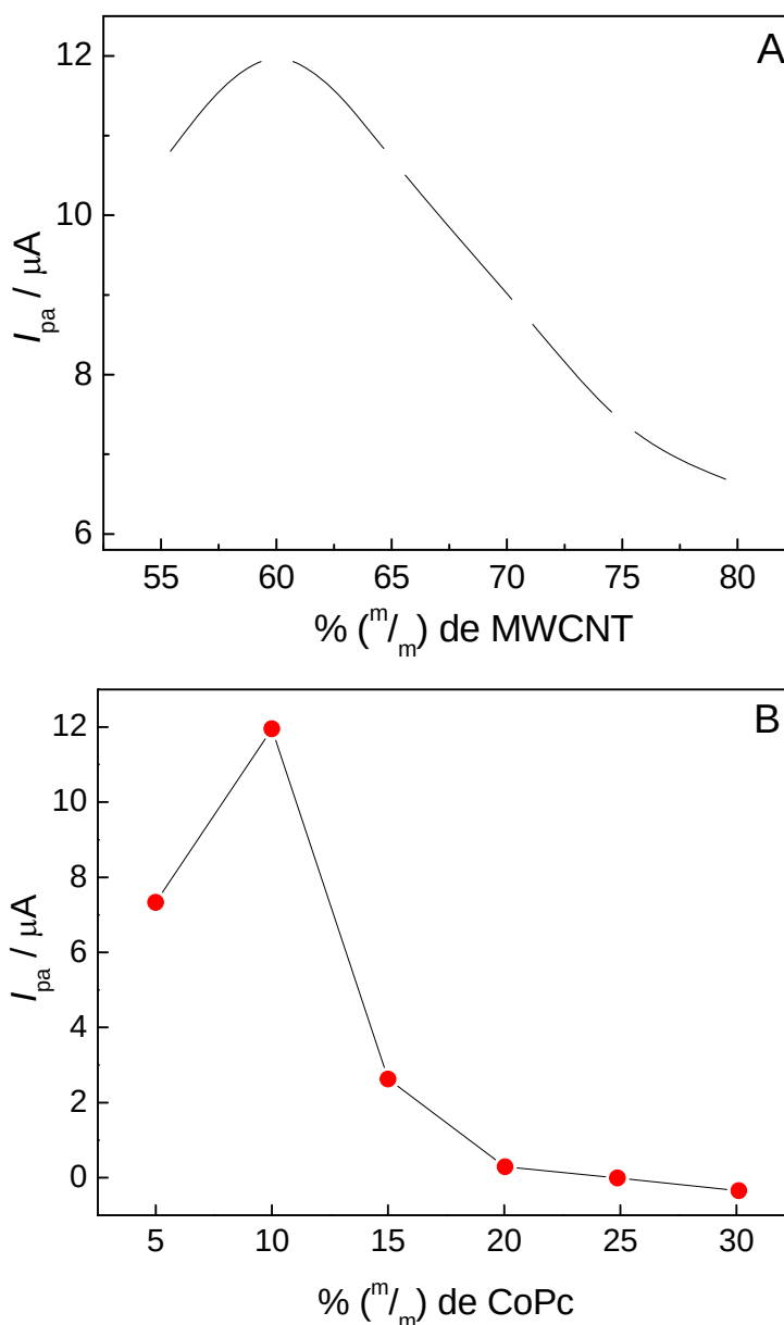
Figura 51. Efeito da composição do eletrodo no pico de oxidação da EP, em 0,2 mol L -1 de PBS (pH 6,0) contendo 1,0 mmol L -1 de EP, com amplitude de pulso de 100 mV e salto de potencial de 2mV. (A) Proporção ( m/m ) de MWCNT e parafina. (B) Proporção ( m/m ) de MWCNT e CoPc, com teor de parafina fixo em 40 %.
