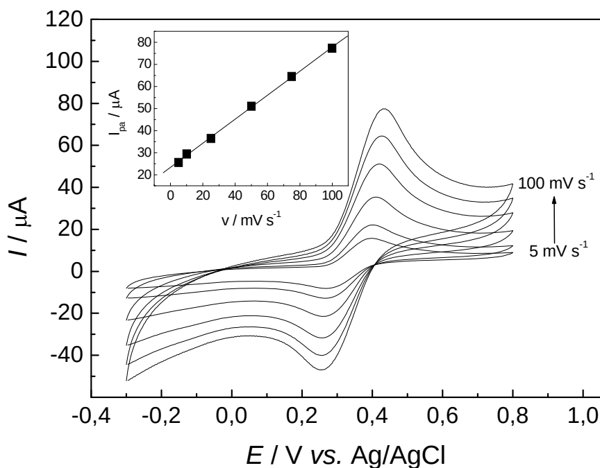
Figura 43. Voltamogramas cíclicos para o eletrodo de GC/MWCNT/CoPc em solução 0,2 \text{ mol L}^{-1} PBS contendo 1,0 \text{ mmol L}^{-1} de dopamina, nas seguintes velocidades de varredura: 5; 10; 25; 50; 75 e 100 \text{ mV s}^{-1} . Detalhe: relação linear entre I_{pa} e a velocidade de varredura.
