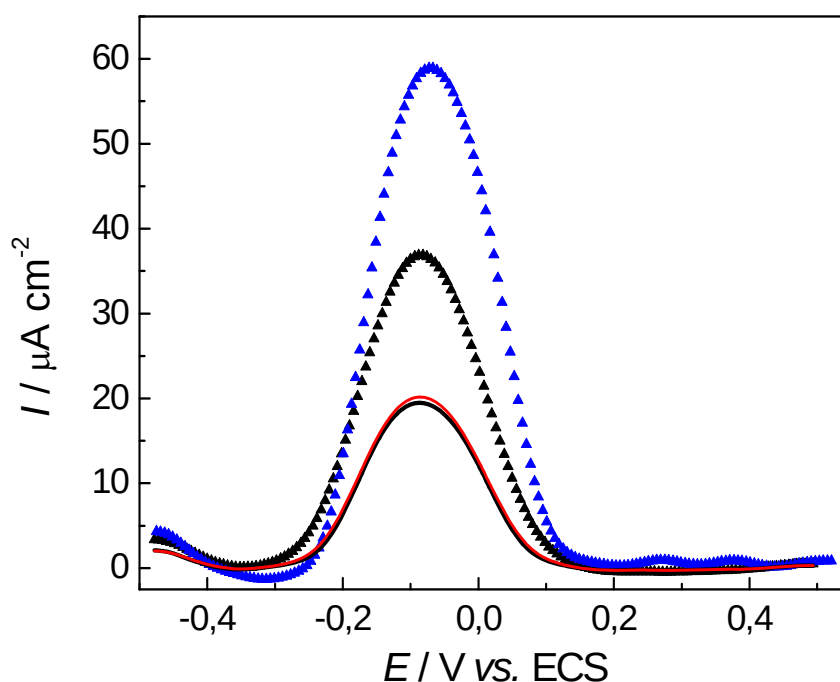
Figura 32. Voltamogramas de DPV, em PBS (pH 7,5) para os eletrodos: GC/MWCNT na ausência (—) e na presença de 1,0 \text{ mmol L}^{-1} de Gli (—) e GC/MWCNT/CuPc na ausência ( \blacktriangle ) e presença de 1,0 \text{ mmol L}^{-1} de Gli ( \blacktriangle ). Os parâmetros de DPV foram amplitude de 100 mV e step de potencial de 2mV.
