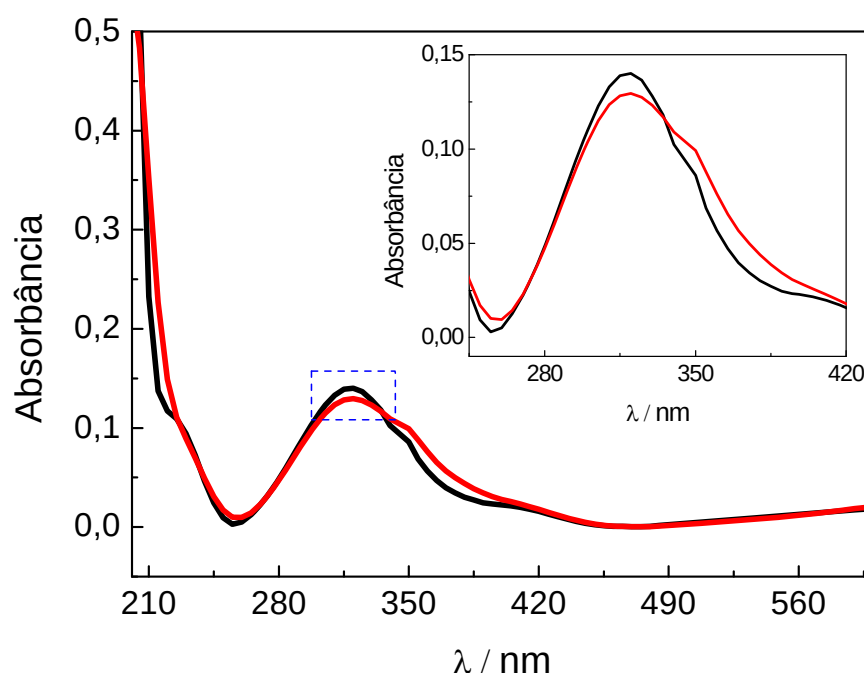
Figura 18. Espectros de UV/Vis para uma solução contendo 1,0 \mu\text{mol L}^{-1} de 4-NP: antes da eletrólise (—) e após uma hora de eletrólise, em potencial fixo de -1,0 V (—). Detalhe: ampliação da região da banda de absorção do 4-NP.
