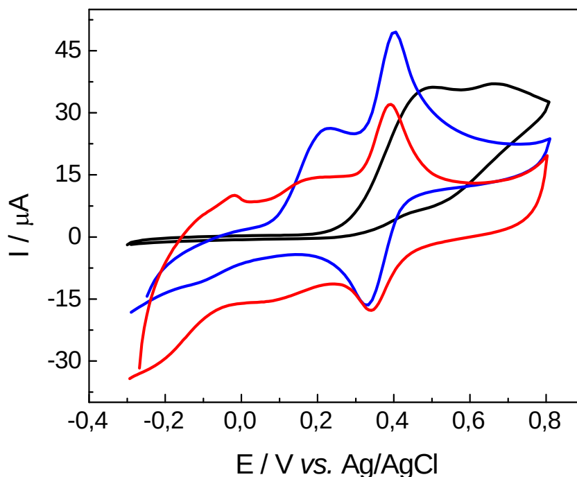
Figura 44. Voltamogramas cíclicos para os eletrodos de GC (—), GC/MWCNT (—) e GC/MWCNT/CoPc (—), em 0,2 \text{ mol L}^{-1} PBS (pH 4.0) contendo 1,0 \text{ mmol L}^{-1} de DA e 2,0 \text{ mmol L}^{-1} de AA, com velocidade de varredura de 50 \text{ mV s}^{-1}
