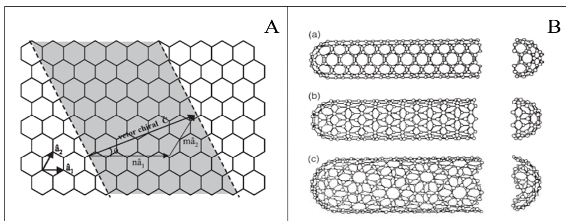
Figura 2 – (A) Diagrama da formação de nanotubos de carbono a partir de uma folha de grafeno e (B) Geometrias dos CNTs: (a) armchair , (b) zig-zag , (c) chiral .
