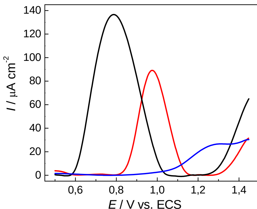
Figura 25. Voltamogramas de SWV para os eletrodos: GC (—), GC/MWCNT (—) e GC/MWCNT/CoPc (—) em solução tampão acetato 0,1 \text{ mol L}^{-1} (pH 4,0) contendo 1,0 \times 10^{-4} \text{ mol L}^{-1} de carbaril, com frequência de 20 Hz, amplitude de 100 mV e salto de potencial de 2 mV.
