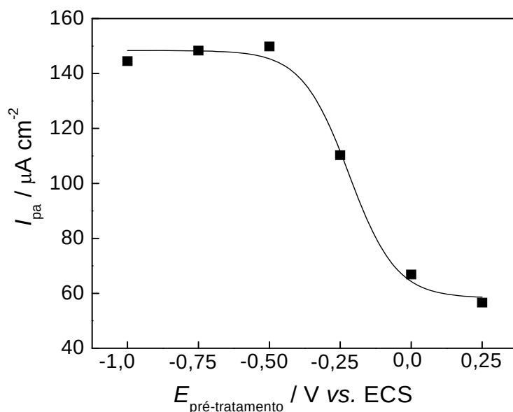
Figura 28. Efeito do potencial de pré-tratamento no pico de oxidação do carbaril em solução tampão acetato 0,1 mol L -1 (pH 4,0) contendo 1,0 \times 10^{-4} mol L -1 de carbaril.
