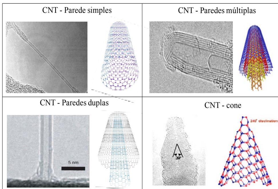
Figura 1 – Diagrama e microscopias dos diferentes tipos de CNTs.
