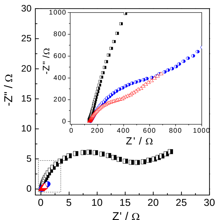
Figura 41. Espectros no plano complexo para os eletrodos de GC (■), GC/MWCNT (●) e GC/MWCNT/CoPc (△), em PBS 0,2 \text{ mol L}^{-1} (pH 4.0) contendo 1.0 \text{ mmol L}^{-1} de DA. Detalhe mostra a ampliação do espectro.
