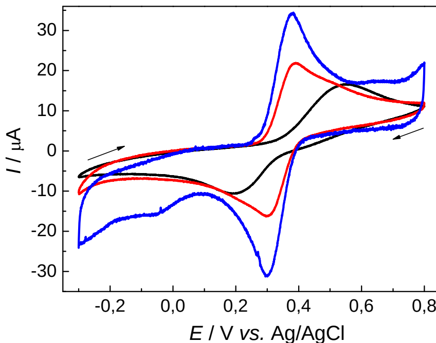
Figura 40. Voltamogramas cíclicos para os eletrodos de GC (—), GC/MWCNT (—) e GC/MWCNT/CoPc (—), em PBS 0,2 \text{ mol L}^{-1} (pH 4.0) contendo 1,0 \text{ mmol L}^{-1} de dopamina, com velocidade de varredura de 50 \text{ mV s}^{-1} .
