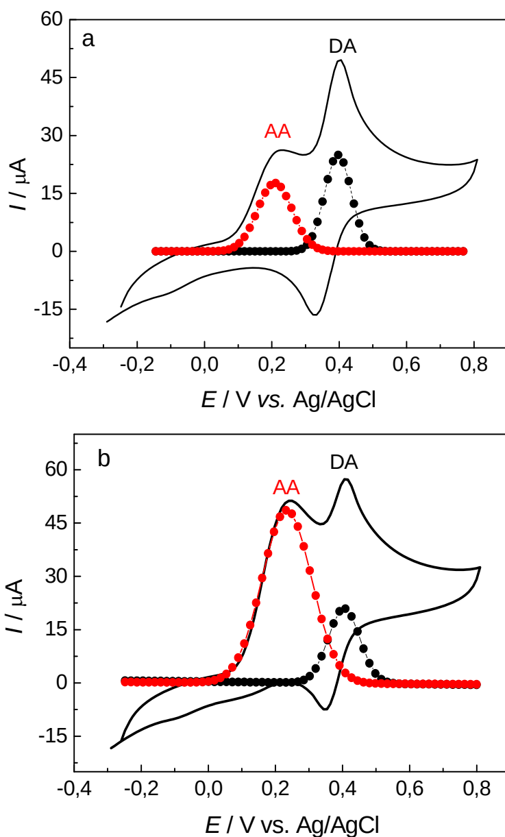
Figura 45. Voltamogramas cíclicos para o eletrodo de GC/MWCNT/CoPc: (a) 1,0 mmol L -1 de DA + 2,0 mmol L -1 de AA e (b) 1,0 mmol L -1 de DA + 100,0 mmol L -1 de AA. Os símbolos correspondem aos processo de deconvolução dos voltamogramas para o AA (●) e para a DA (●).
