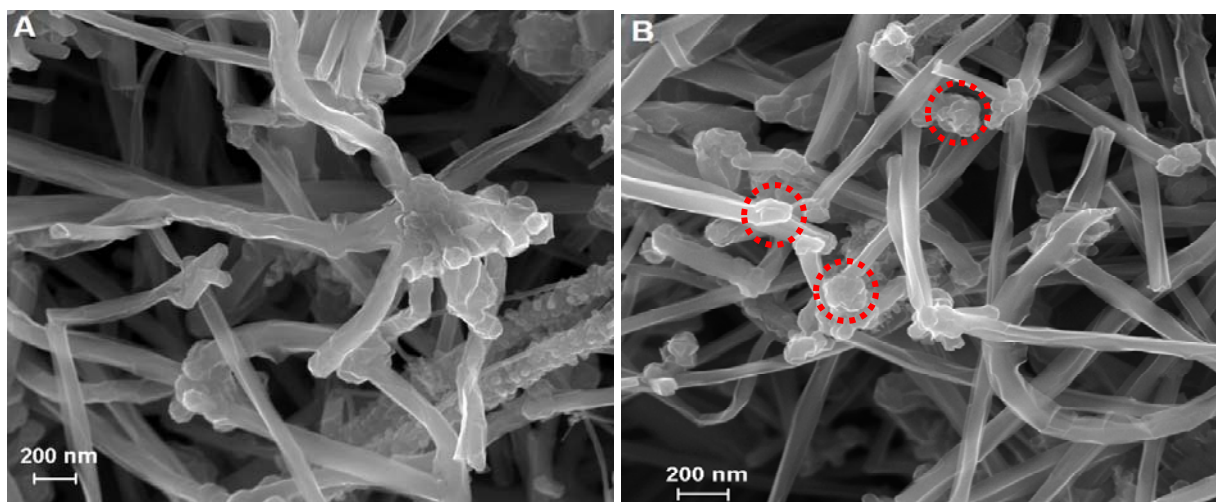
Figura 24 – Micrografias de FEG-SEM para os filmes: (A) MWCNT e (B) MWCNT/CoPc.
