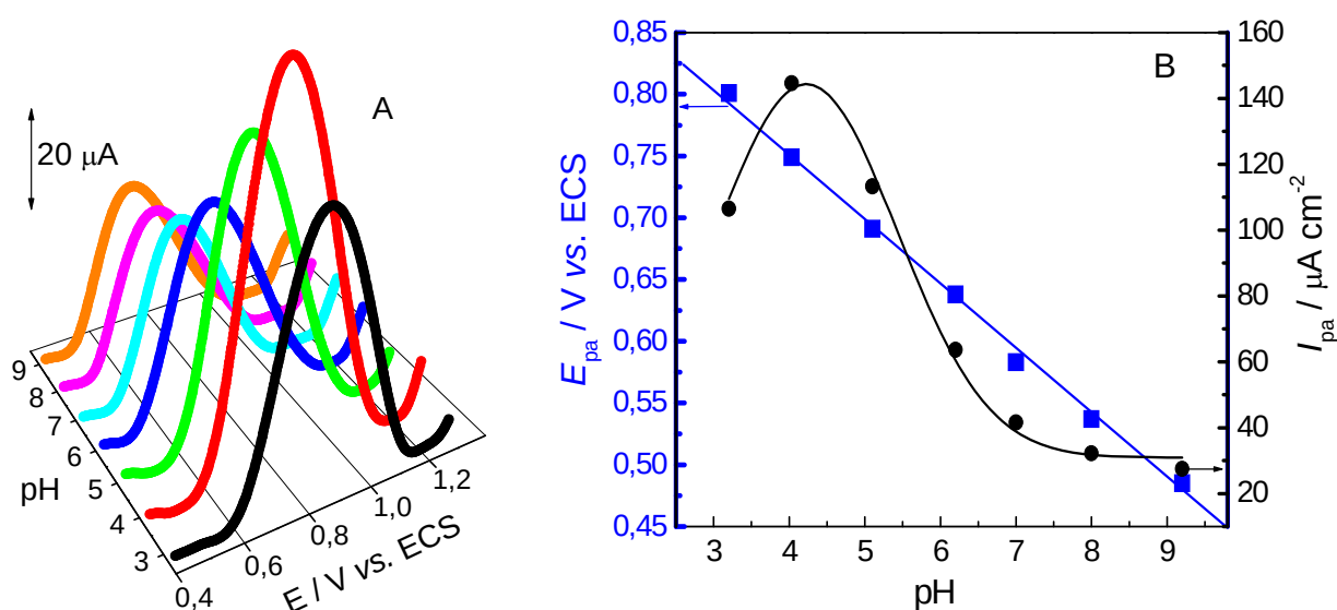
Figura 29. (A) Voltamogramas de SWV para o eletrodo de GC/MWCNT/CoPc em em solução eletrolítica tampão com força iônica de 0.1 mol L -1 em diferentes valores de pH, contendo 1,0 \times 10^{-4} mol L -1 de carbaril. (B) Gráfico de E_{pa} em função do pH (■) e I_{pa} em função do pH (●).
