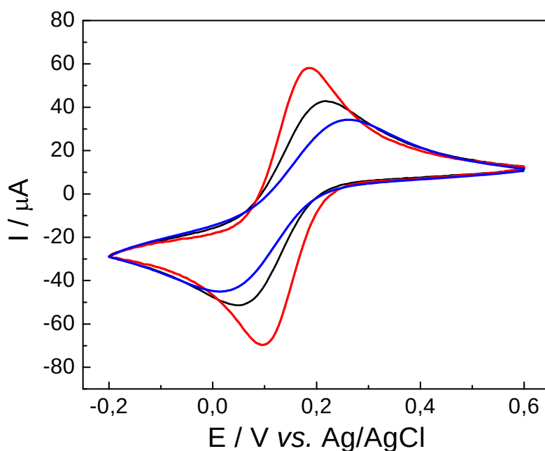
Figura 14. Voltamogramas cíclicos para os eletrodos: GC (—), GC/MWCNT não funcionalizado (—) e GC/MWCNT funcionalizado (—), em meio 0,1 mol L -1 de H 2 SO 4 contendo 5,0 mmol L -1 de K 3 [Fe(CN) 6 ], com velocidade de varredura de potencial de 50 mV s -1 .
