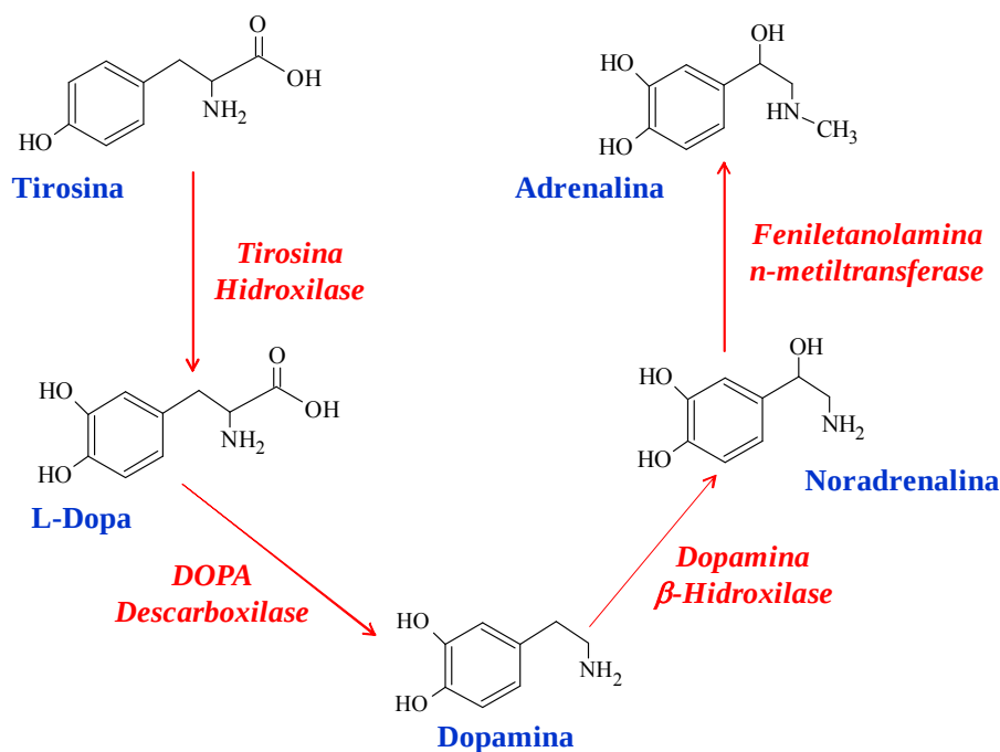
Figura 4. Mecanismo de transformação das catecolaminas no organismo.
