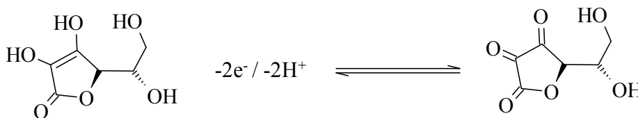
Figura 5. Estruturas moleculares e mecanismos de oxidação eletroquímica para a dopamina e ácido ascórbico.
