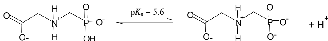
Figura 34. Esquema do equilíbrio e constante de dissociação ácida do glifosato.
