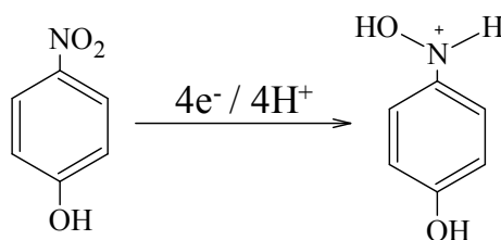
Figura 6. Redução eletroquímica do 4-NP formando hidroxilamina.
