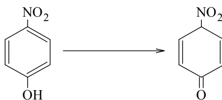
Figura 7. Oxidação eletroquímica do 4-NP formando p -benzoquinona.
