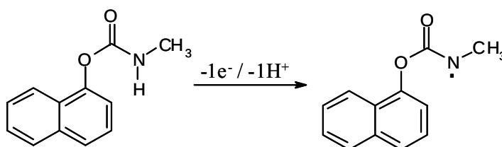
Figura 30. Mecanismo eletroquímico para a reação de oxidação de carbaril.
