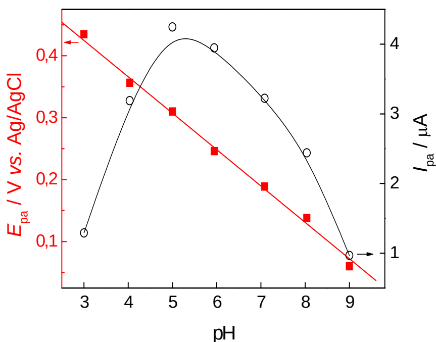
Figura 50. Gráfico da relação linear entre a variação de pH vs. E_{pa} (■) e pH vs. I_{pa} (●), em meio 0,2 mol L -1 PBS contendo 1,0 mmol L -1 EP.
