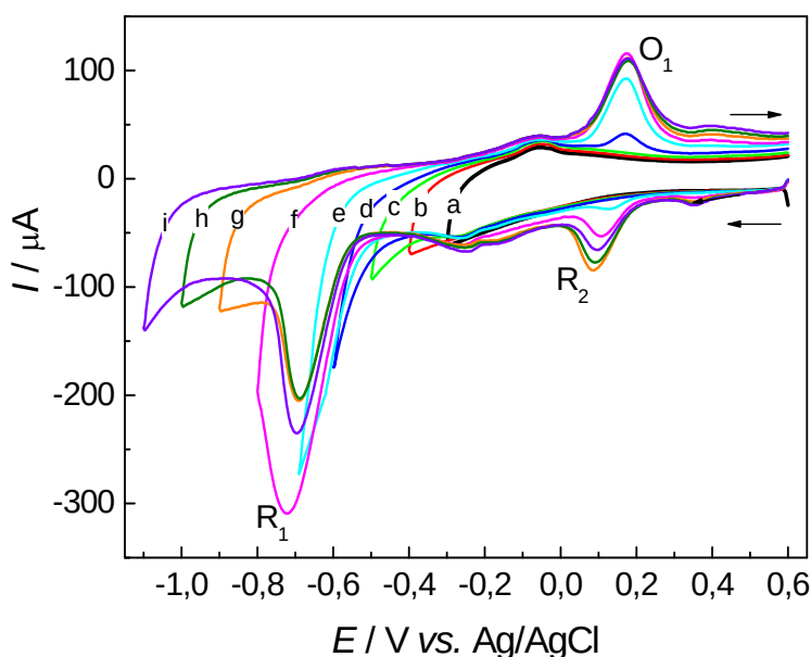
Figura 16. Voltamogramas cíclicos obtidos para 1,0 mmol L -1 de 4-NP em meio de PBS (pH = 6,0), com os seguintes potenciais de inversão: (a) -0,3; (b) -0,4; (c) -0,5; (d) -0,6; (e) -0,7; (f) -0,8; (g) -0,9; (h) -1,0 e (i) -1,1 V.
