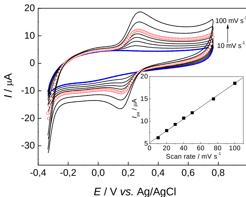
Figura 47. Voltamogramas cíclicos para o eletrodo composto de Parafina/MWCNT/CoPc na ausência de EP (—) e na presença de 1,0 \text{ mmol L}^{-1} de EP (○), com velocidade de varredura de 50 \text{ mV s}^{-1} . Voltamogramas cíclicos com 1,0 \text{ mmol L}^{-1} de EP (—) nas seguintes velocidades de varredura: 10; 20; 30; 40; 75 e 100 \text{ mV s}^{-1} . Detalhe: Relação linear entre I_{pa} e a velocidade de varredura.
