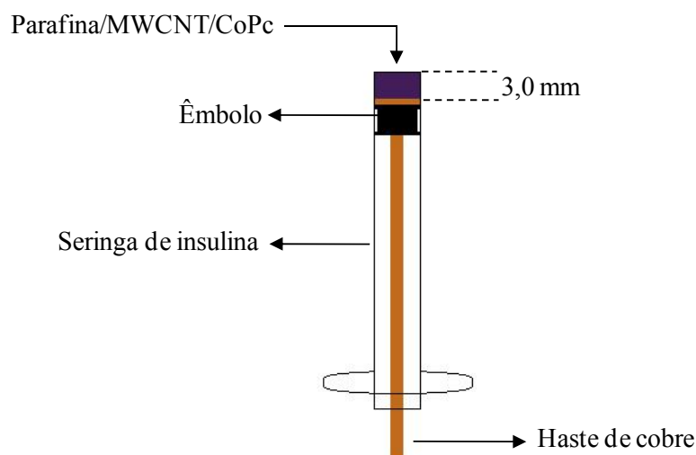
Figura 10. Esquema do eletrodo composto Parafina/MWCMT/CoPc.
