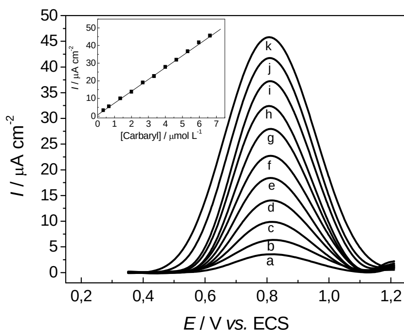
Figura 31. Curva analítica utilizando SWV com o eletrodo de GC/MWCNT/CoPc com os parâmetros otimizados para as seguintes concentrações de carbaril em \mu\text{mol L}^{-1} : (a) 0,33; (b) 0,66; (c) 1,33, (d) 1,99; (e) 2,66, (f) 3,33; (g) 3,99; (h) 4,66; (i) 5,33; (j) 5,99 e (k) 6,62. Detalhe: dependência linear do pico de corrente com a concentração de carbaril.
