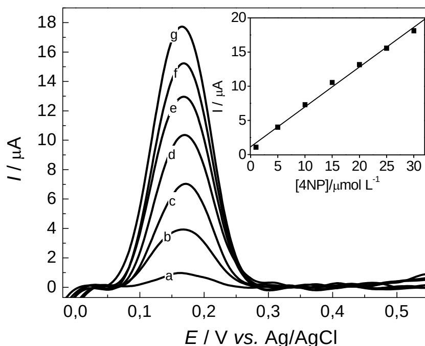
Figura 23. Voltamogramas de SWV para o eletrodo de GC/MWCNT, com os valores otimizados mostrados na Tabela 3. As concentrações de 4-NP em \mu\text{mol L}^{-1} são: (a) 1,0; (b) 5,0; (c) 10,0; (d) 15,0; (e) 20,0; (f) 25,0 e (g) 30,0. Detalhe: dependência linear dependence do pico de corrente com a concentração de 4-NP.
