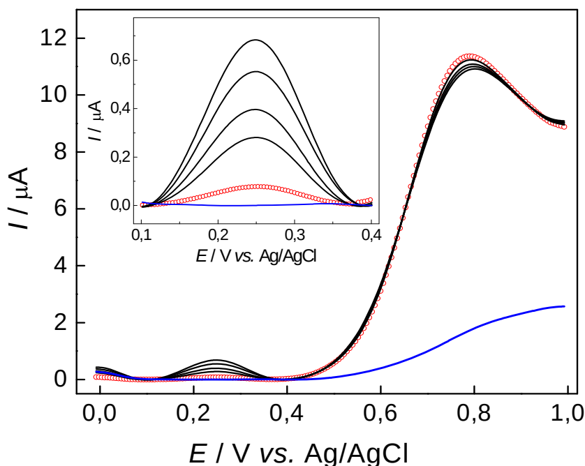
Figura 55. Voltamogramas de DPV para o eletrodo compósito de Parafina/MWCNT/CoPc: PBS na ausência de urina humana (—), PBS contendo urina humana (○) e adições consecutivas de padrão de EP (—) nas seguintes concentrações: 100, 150, 200 e 250 \text{nmol L}^{-1} . Detalhe: ampliação da região de eletro-oxidação da EP.
