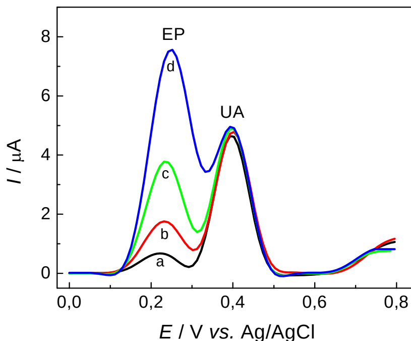
Figura 53. Voltamogramas de DPV para o eletrodo composto de Parafina/MWCNT/CoPc, em 0,2 \text{ mol L}^{-1} de PBS (pH 6,0) contendo 1,0 \times 10^{-4} \text{ mol L}^{-1} de UA e foram adicionadas as seguintes concentrações de EP: (a) 1,0 \times 10^{-5} , (b) 5,0 \times 10^{-5} , (c) 1,0 \times 10^{-4} e (d) 5,0 \times 10^{-4} \text{ mol L}^{-1} .
