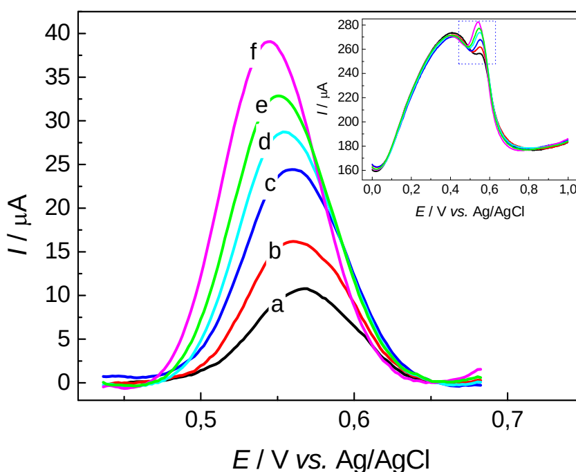
Figura 46. Voltamogramas de DPV para o eletrodo de GC/MWCNT/CoPc, em 0,2 mol L -1 de PBS (pH 4,0) contendo 0,1 mol L -1 de AA. As concentrações de DA em μmol L -1 : (a) 3,1; (b) 13,5; (c) 32,5; (d) 50,5; (e) 62,5 e (f) 90,3. Detalhe: Resposta total dos voltamogramas contendo AA e as adições de DA.
