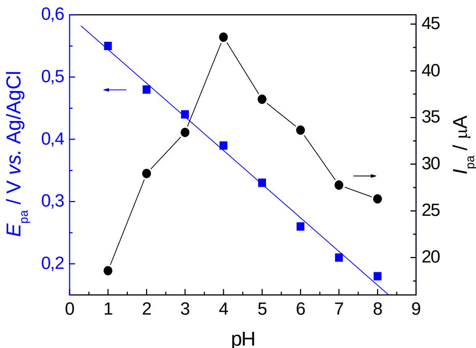
Figura 42. Efeito do pH no E_{pa} (■) e I_{pa} (●) para a oxidação de dopamina sobre o eletrodo de GC/MWCNT/CoPc, em PBS 0,2 mol L -1 contendo 1,0 mmol L -1 de dopamina.
