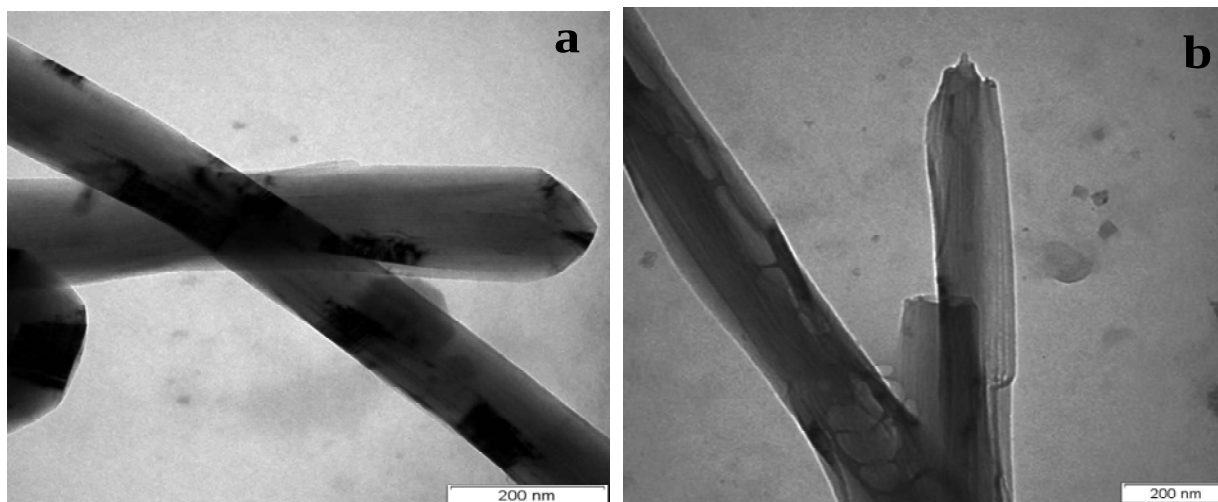
Figura 12. Microscopia TEM: (a) CNTs não funcionalizados e (b) CNTs funcionalizados.
