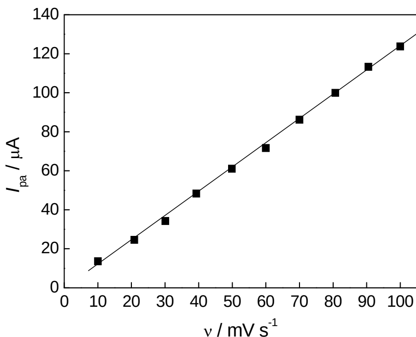
Figura 35. Dependência linear da velocidade de varredura com a I_{pa} .
