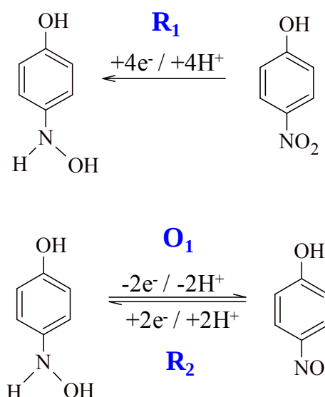
Figura 19. Mecanismo eletroquímico do 4-NP na superfície do eletrodo de GC/MWCNT.
