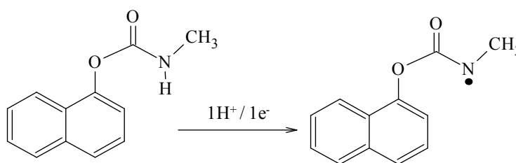
Figura 8. Mecanismo de oxidação eletroquímica do carbaril.
