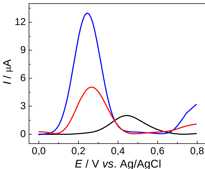
Figura 48. Voltamogramas de DPV para os eletrodos compósitos: Parafina/Grafite (—), Parafina/MWCNT (—) e Parafina/MWCNT/CoPc (—) em 0,2 \text{ mol L}^{-1} PBS (pH 6,0) contendo 1,0 \text{ mmol L}^{-1} de EP, amplitude de 100 mV e salto de potencial de 2 mV.
