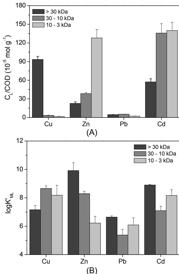
FIGURA 9.3 Capacidade de complexação, C_L (A) e \log K'_{ML} (B) dos excretados da cianobactéria: fração > 30 kDa (cinza escuro); fração entre 30 kDa - 10 kDa (cinza médio); fração entre 10 kDa - 3 kDa (cinza claro) frente aos metais cobre, zinco, cádmio e chumbo.
