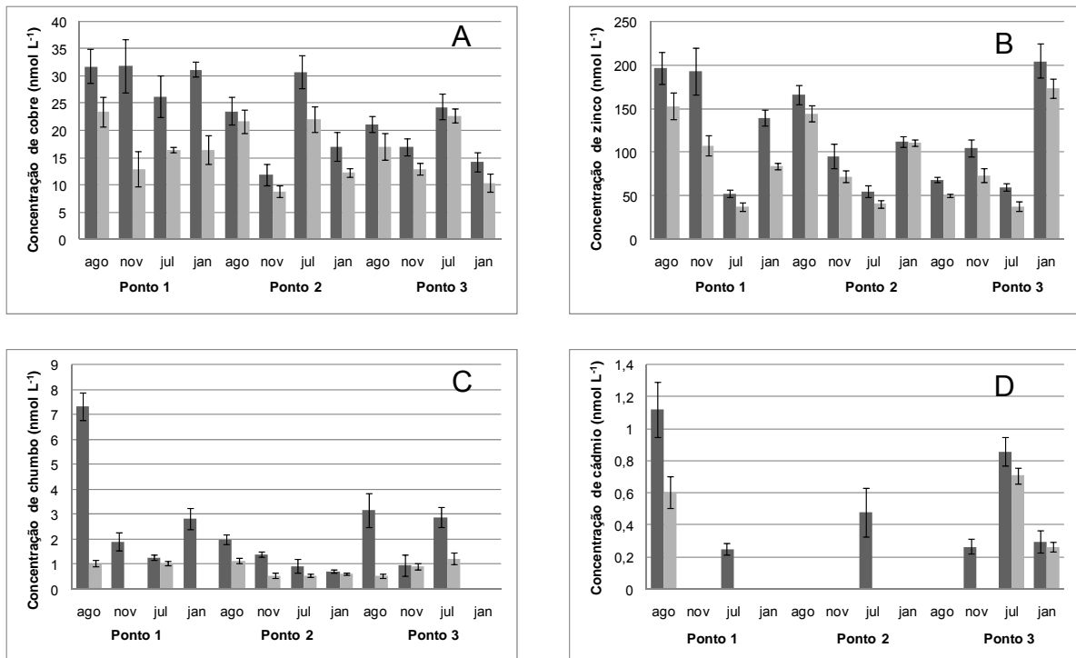
FIGURA 4.6 Concentração total (cinza escuro) e total dissolvida (cinza claro) (nmol L -1 ) de cobre (A), zinco (B), chumbo (C) e cádmio (D) nas amostras de água do Reservatório de Barra Bonita.
