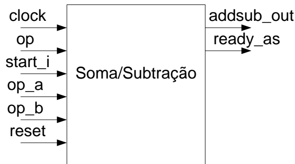
Figura 4.2. entradas/saídas para o bloco soma/subtração
