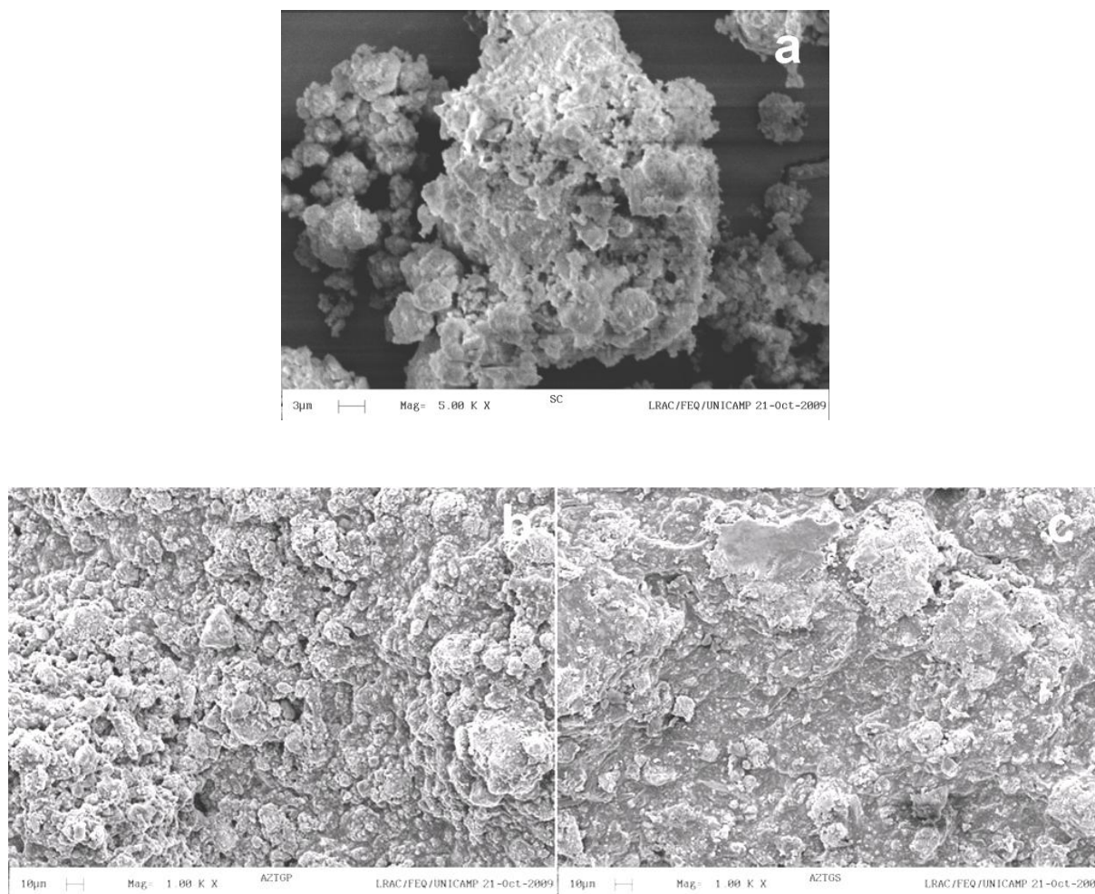
Figura 31: Microscopia eletrônica de varredura: (a) partículas de silicato de cálcio, (b) AZTGP e (c) AZTGS.
