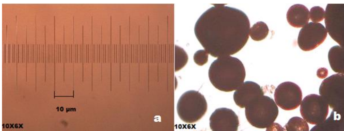
Figura 25: Fotografia obtida em microscópio óptico (aumento no microscópio 10X e aumento na máquina fotográfica 6X) da lâmina com régua de 100 µm (a) e dos microballoons obtidos pelo método MODIFICADO de difusão e evaporação dos solventes da emulsão (b).
