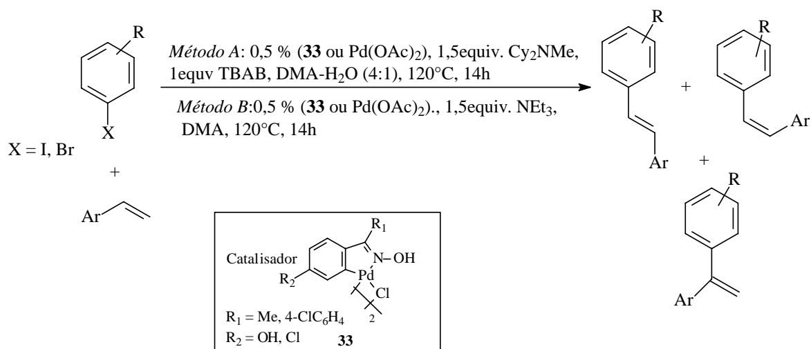
Esquema 37 – Acoplamento entre haleto de arila e estirenos catalisado por paladaciclo ou Pd(OAc) 2 . 98
