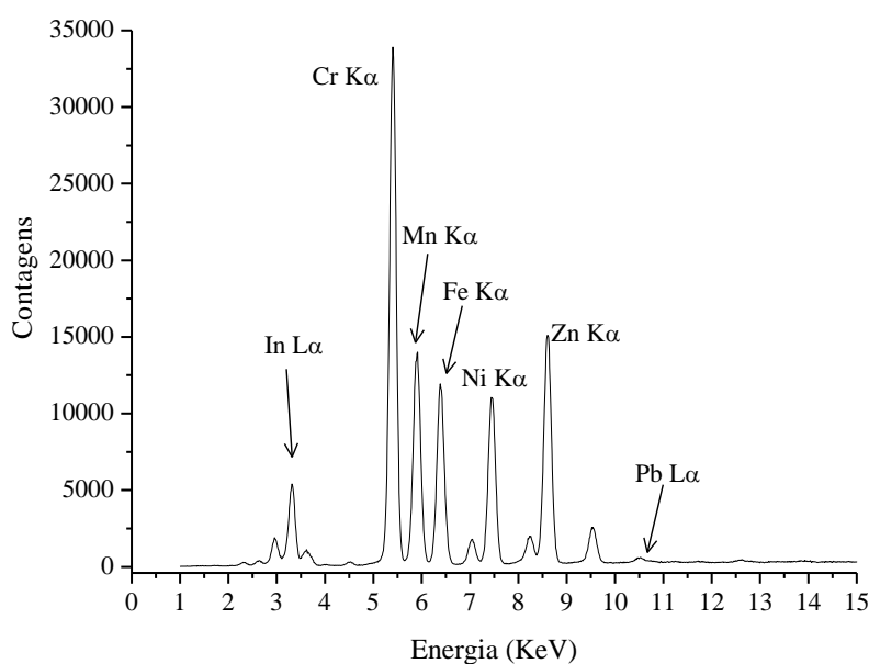
Figura 5. Espectro de TXRF típico de solução de padrões.
