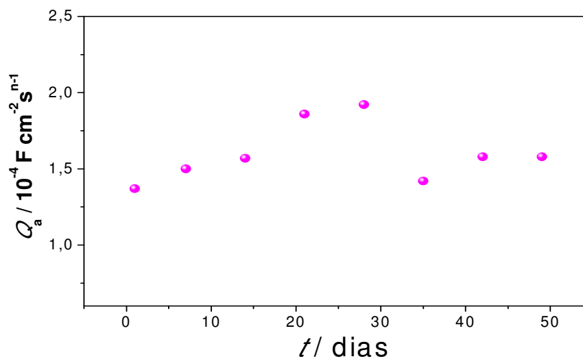
FIGURA 3.67: Valores de Q_a obtidos por EIE para a liga Ti-13Nb-13Zr recoberta por seu óxido natural e HA, em função do tempo de imersão em solução PBS. Sistemas: (a) liga/ox. natural/ \text{HA}_{\text{bio}} e (b) liga/ox. natural/ \text{HA}_{\text{eletro}} .
