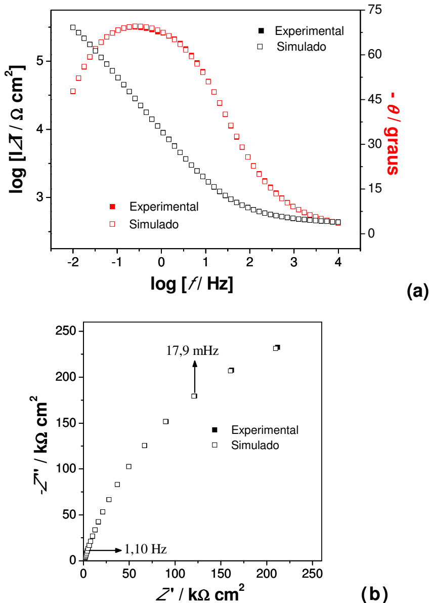
FIGURA 3.84: Espectros de EIE para a liga Ti-13Nb-13Zr com óxido crescido por MAO a 300 V, após 35 dias a circuito aberto em solução PBS. Diagramas: (a) Bode; (b) Nyquist.
