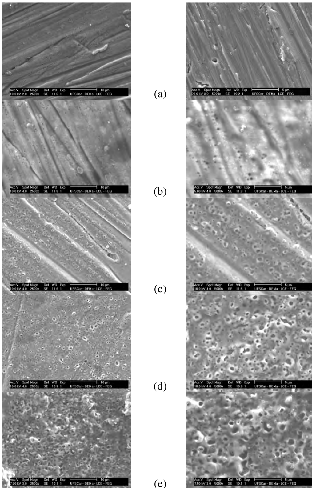
FIGURA 3.16: Micrografias de MEV dos óxidos crescidos a diferentes potenciais sobre a liga Ti-13Nb-13Zr em solução de tampão fosfato, durante 60 s: (a) 180 V; (b) 210 V; (c) 240 V; (d) 270 V e (e) 300 V.
