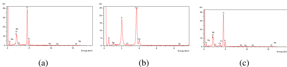
FIGURA 3.97: Espectros de EDS da liga Ti-13Nb-13Zr recoberta por óxido crescido a 300 V e HA obtidas pelo método biomimético e por eletrodeposição, após 49 dias de imersão em solução PBS. Sistemas: (a) liga/ox. 300 V; (b) liga/ox. 300 V/HA bio e (c) liga/ox. 300 V/HA eletro .
