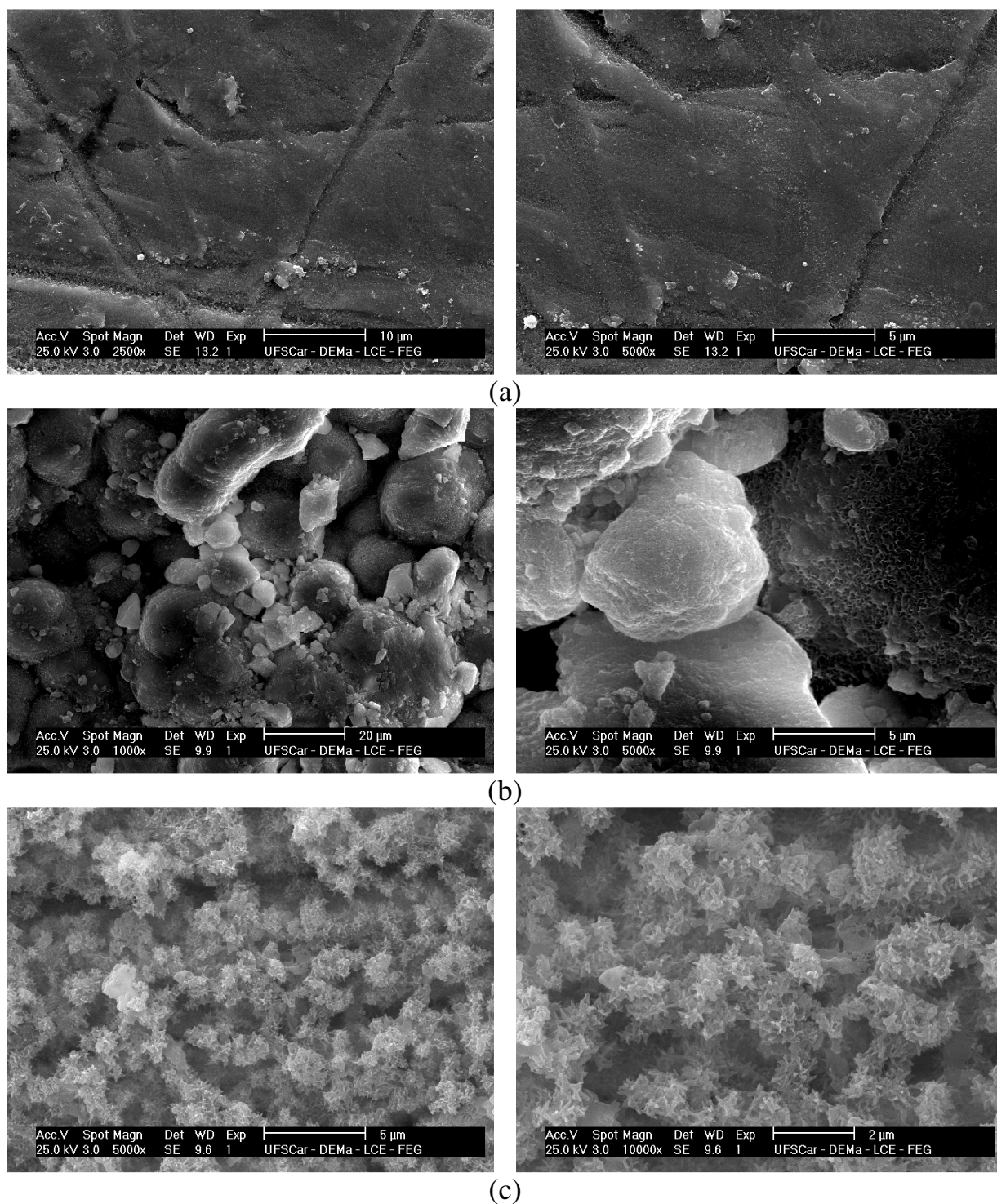
FIGURA 3.80: Micrografias de MEV da liga Ti-13Nb-13Zr recoberta por óxido crescido até 8 V e HA, após 49 dias de imersão em solução PBS. Sistemas: (a) liga/ox. 8 V; (b) liga/ox. 8 V/HA bio e (c) liga/ox. 8 V/HA eletro .
