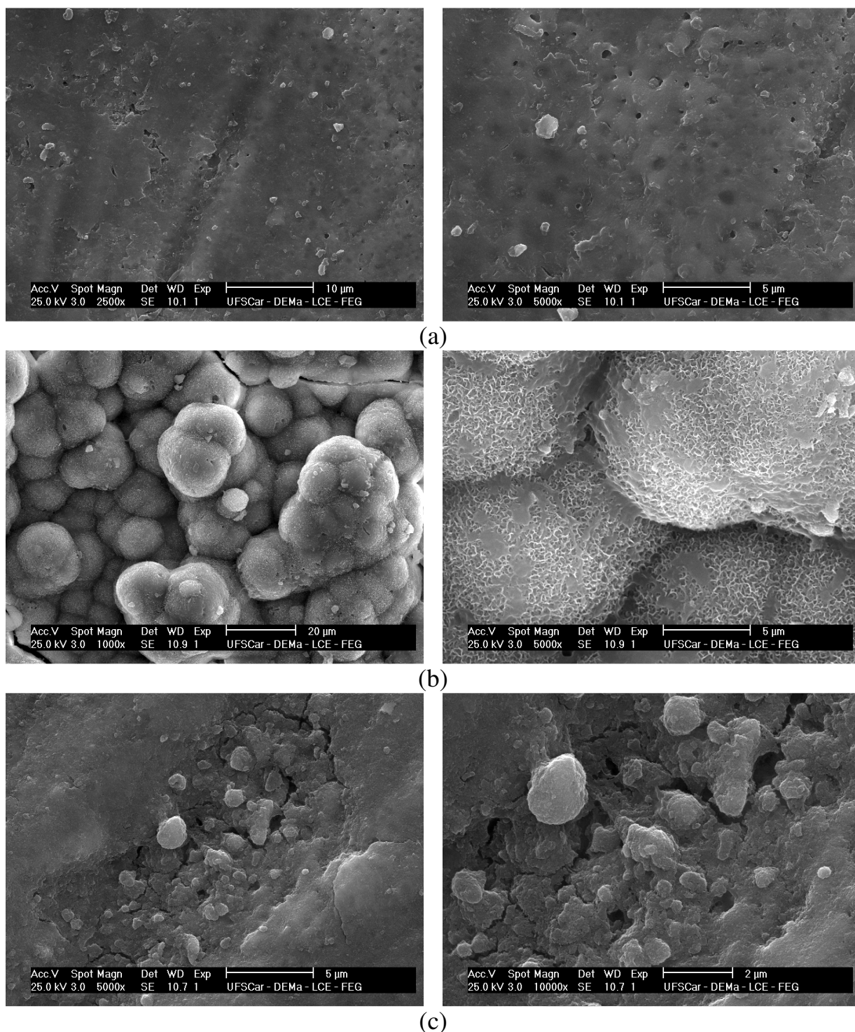
FIGURA 3.96: Micrografias de MEV da liga Ti-13Nb-13Zr recoberta por óxido crescido a 300 V, após 49 dias de imersão em solução PBS. Sistemas: (a) liga/ox. 300 V; (b) liga/ox. 300 V/HA bio e (c) liga/ox. 300 V/HA eletrô .
