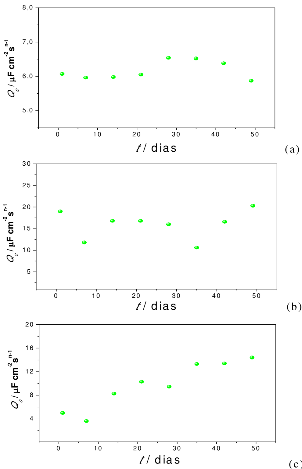
FIGURA 3.77: Valores de Q_c obtidos por EIE para a liga Ti-13Nb-13Zr recoberta por óxido crescido até 8 V, em função do tempo de imersão em solução PBS. Sistemas: (a) liga/ox. 8 V; (b) liga/ox. 8 V/HA bio e (c) liga/ox. 8 V/HA eletro .
