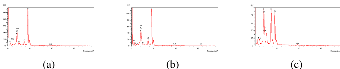
FIGURA 3.47: Espectros de EDS dos filmes de HA eletrodepositadas a -13 \text{ mA cm}^{-2} a várias temperaturas sobre óxidos crescidos por micro-arco a 270 V sobre a liga Ti-13Nb-13Zr em solução tampão fosfato: (a) temperatura ambiente, (b) 40 \text{ }^\circ\text{C} e (c) 60 \text{ }^\circ\text{C} .
