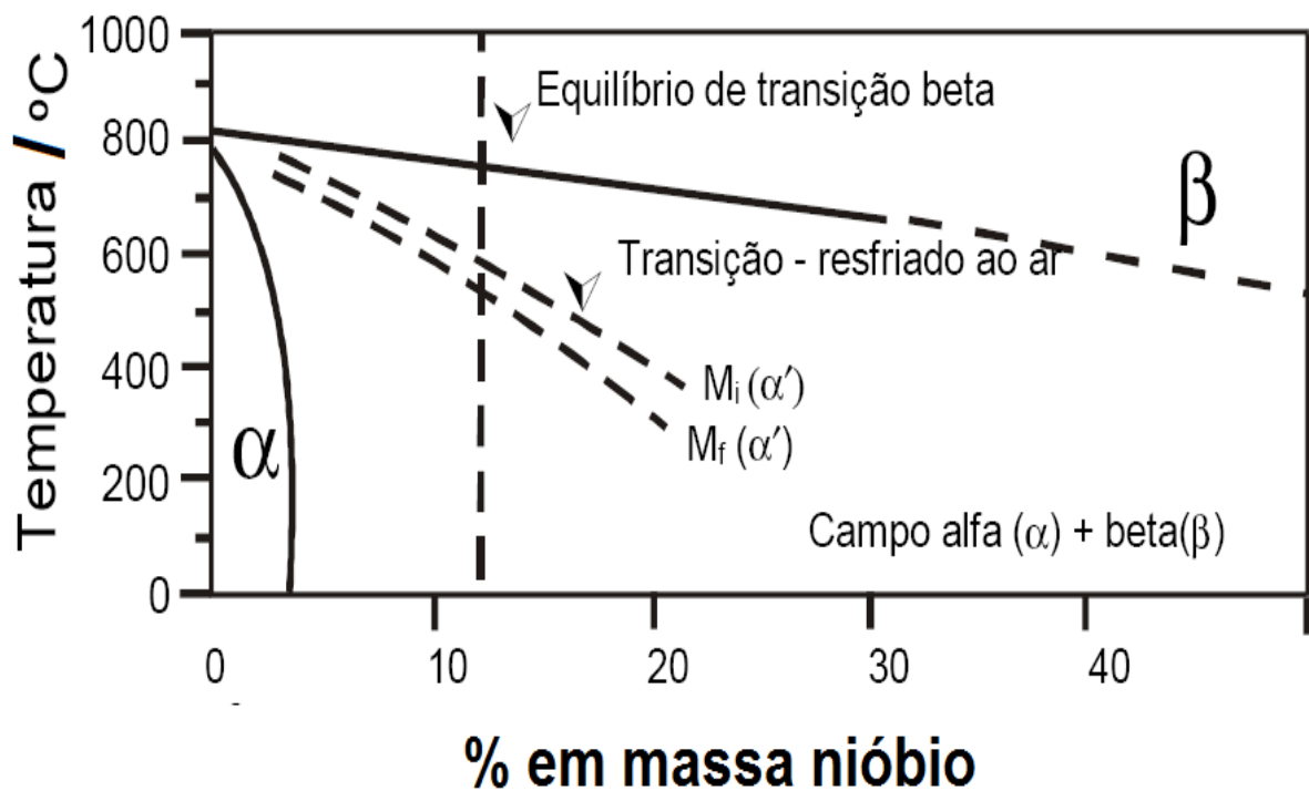
FIGURA 1.2: Diagrama de fase estimado da liga Ti-Nb para 13% em massa de Zr a partir do diagrama de fase ternário Ti-Nb-Zr (DAVIDSON et al. , 1994).
