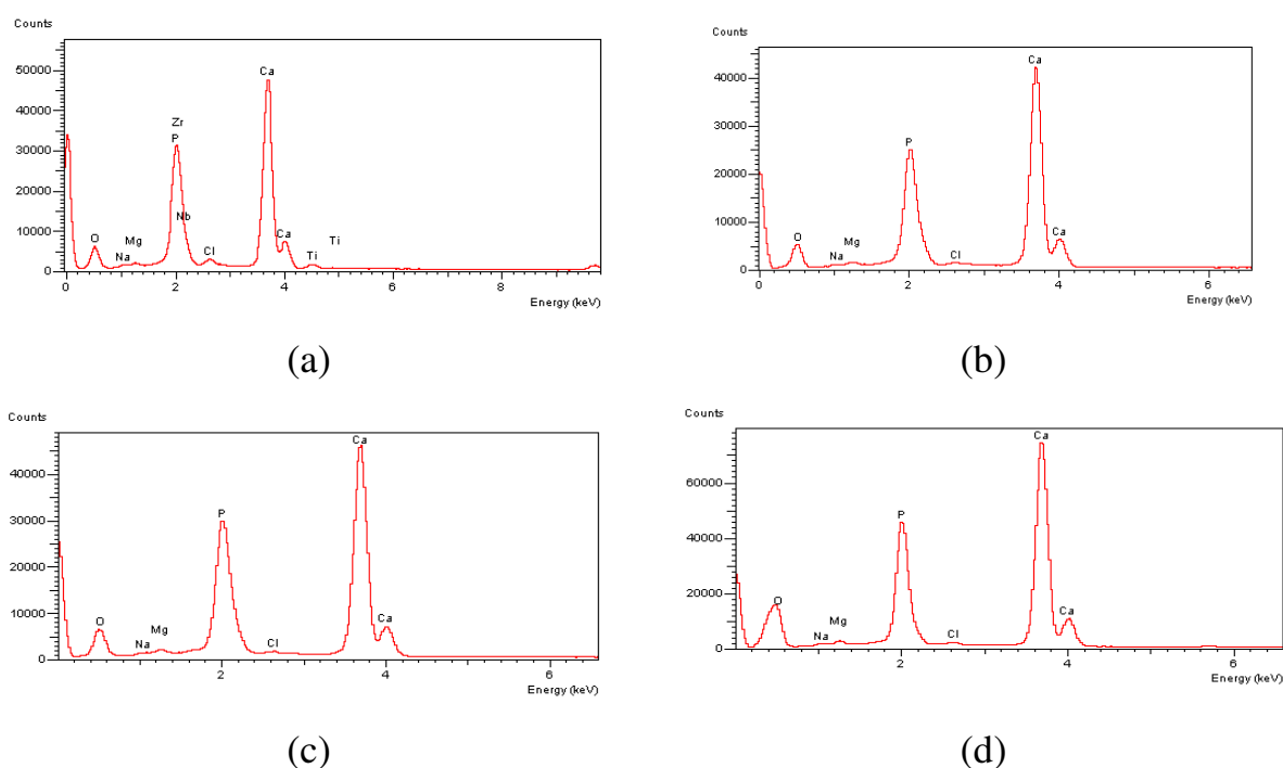
Figura 3.29: Espectros de EDS de HA formada biomimeticamente a diferentes tempos de imersão sobre óxidos crescidos por micro-arco a 240 V sobre a liga Ti-13Nb-13Zr em solução de tampão fosfato: (a) 7, (b) 14, (c) 21 e (d) 28 dias.
