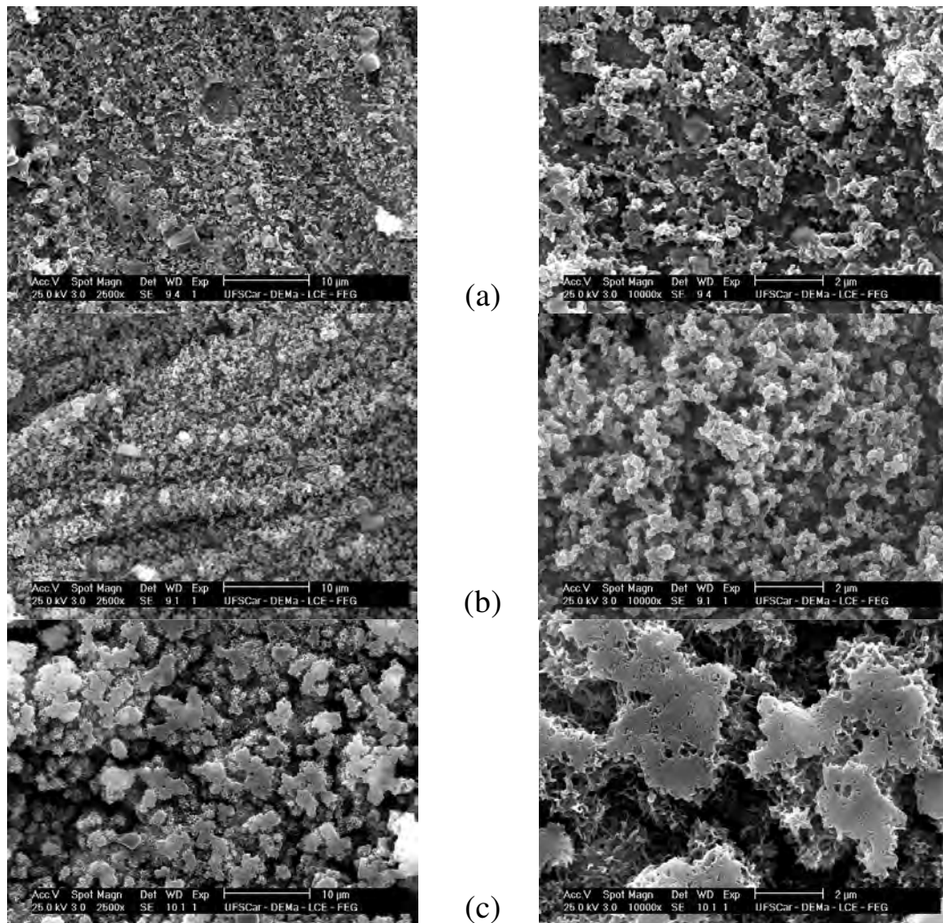
FIGURA 3.40: Micrografias de MEV dos filmes de HA eletrodepositadas a -15 \text{ mA cm}^{-2} a várias temperaturas sobre óxidos crescidos por micro-arco a 270 V sobre a liga Ti-13Nb-13Zr em solução tampão fosfato: (a) temperatura ambiente, (b) 40 °C e (c) 60 °C.
