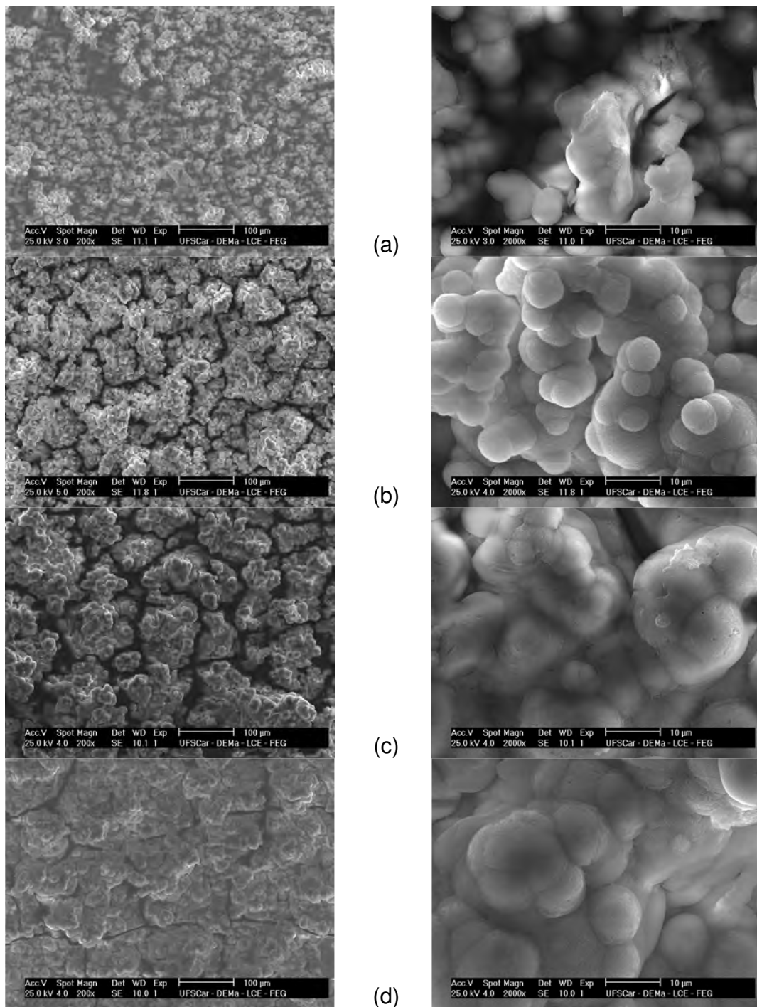
FIGURA 3.26: Micrografias de MEV dos óxidos crescidos por micro-arco a 270 V sobre a liga Ti-13Nb-13Zr em solução de tampão fosfato e cobertos com HA formada biomimeticamente a diferentes tempos de imersão: (a) 7, (b) 14, (c) 21 e (d) 28 dias.
