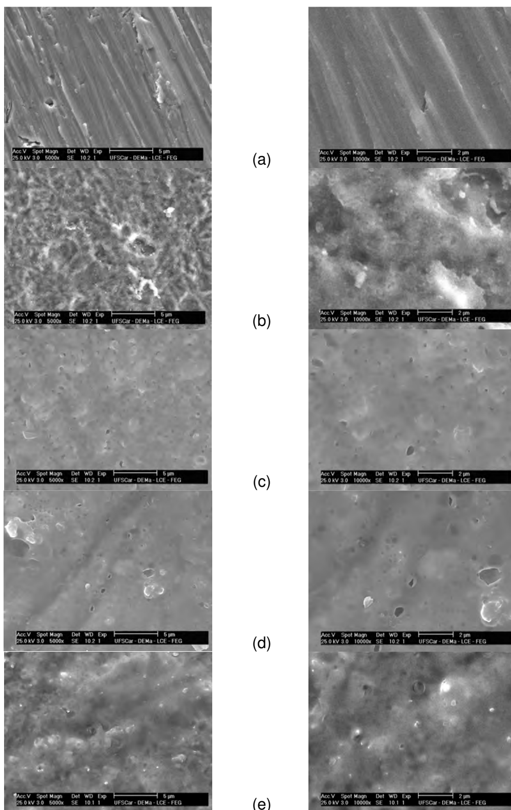
FIGURA 3.20: Micrografias de MEV dos óxidos crescidos a diferentes potenciais sobre a liga Ti-13Nb-13Zr em solução de tampão fosfato após o tratamento químico com HF 5 % por 180 s: (a) 180 V; (b) 210 V; (c) 240 V; (d) 270 V e (e) 300 V.
