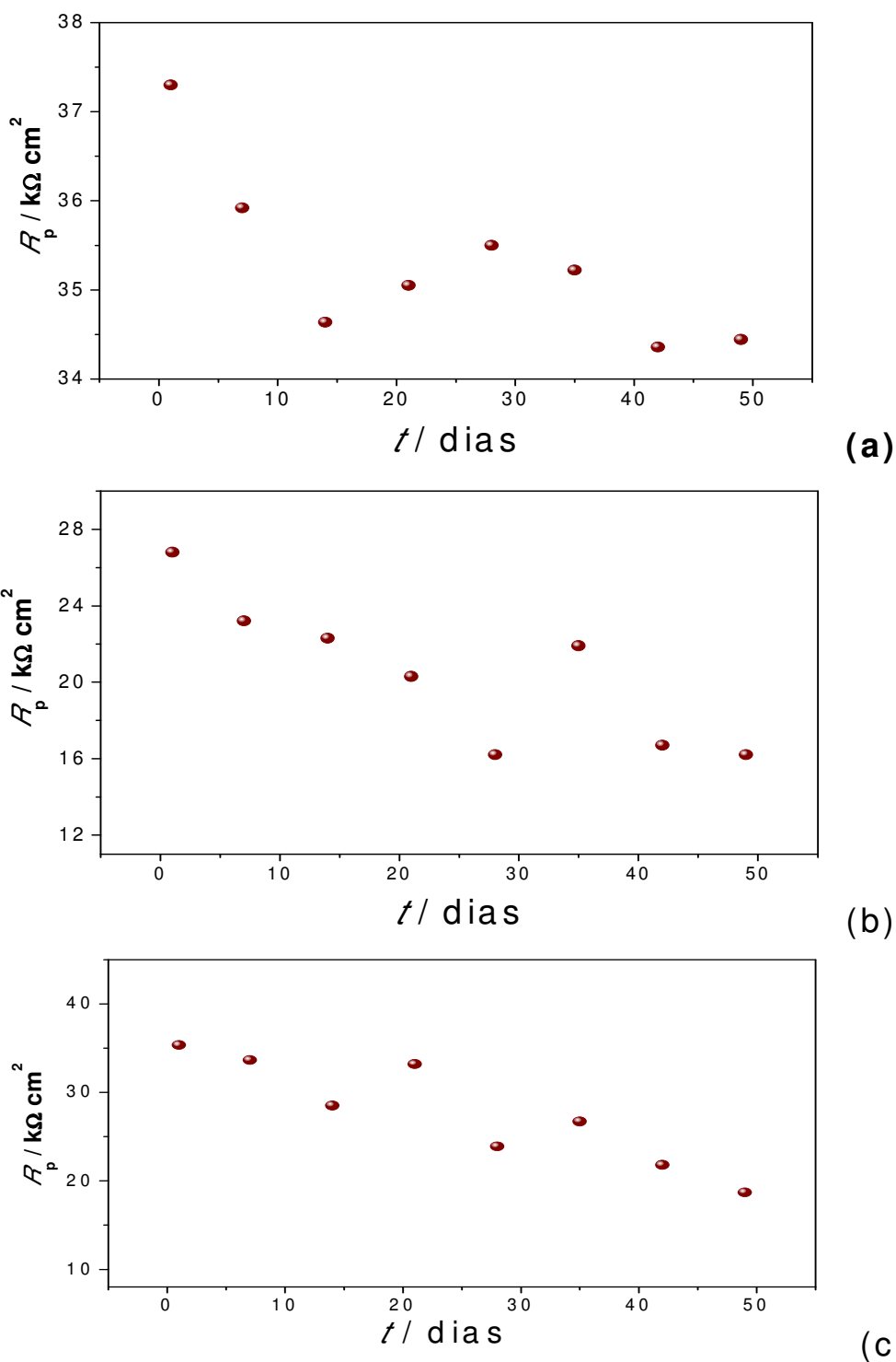
FIGURA 3.92: Valores de R_p obtidos por EIE para a liga Ti-13Nb-13Zr recoberta por óxido crescido a 300 V, em função do tempo de imersão em solução PBS. Sistemas: (a) liga/ox. 300 V; (b) liga/ox. 300 V/ \text{HA}_{\text{bio}} e (c) liga/ox. 300 V/ \text{HA}_{\text{eletro}} .
