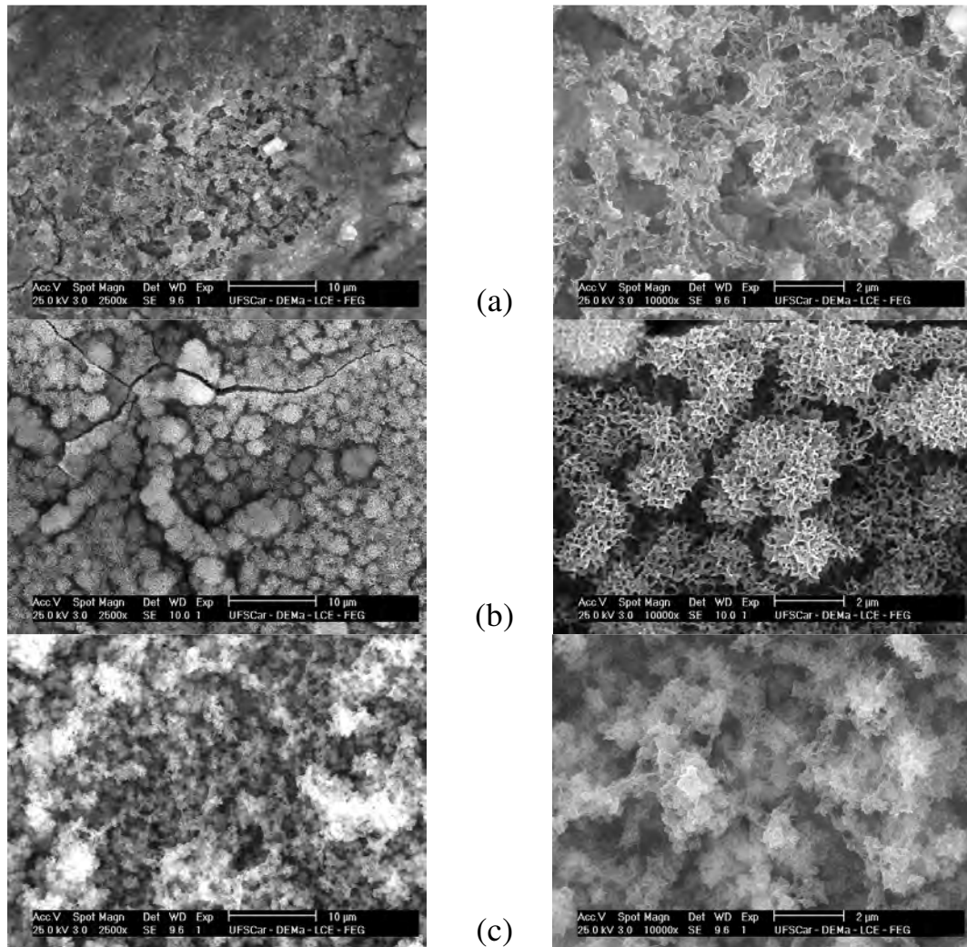
FIGURA 3.44: Micrografias de MEV dos filmes de HA eletrodepositadas a -15 \text{ mA cm}^{-2} a várias temperaturas sobre óxidos crescidos potenciodynamicamente até 8 V sobre a liga Ti-13Nb-13Zr em solução tampão fosfato: (a) temperatura ambiente, (b) 40 \text{ }^\circ\text{C} e (c) 60 \text{ }^\circ\text{C} .
