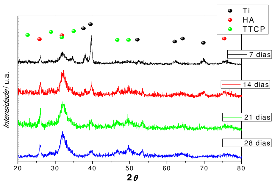
FIGURA 3.34: Difratomogramas de raios X das apatitas obtidas pelo método biomimético a diferentes tempos de imersão, sobre o óxido crescido por micro-arco a 270 V.
