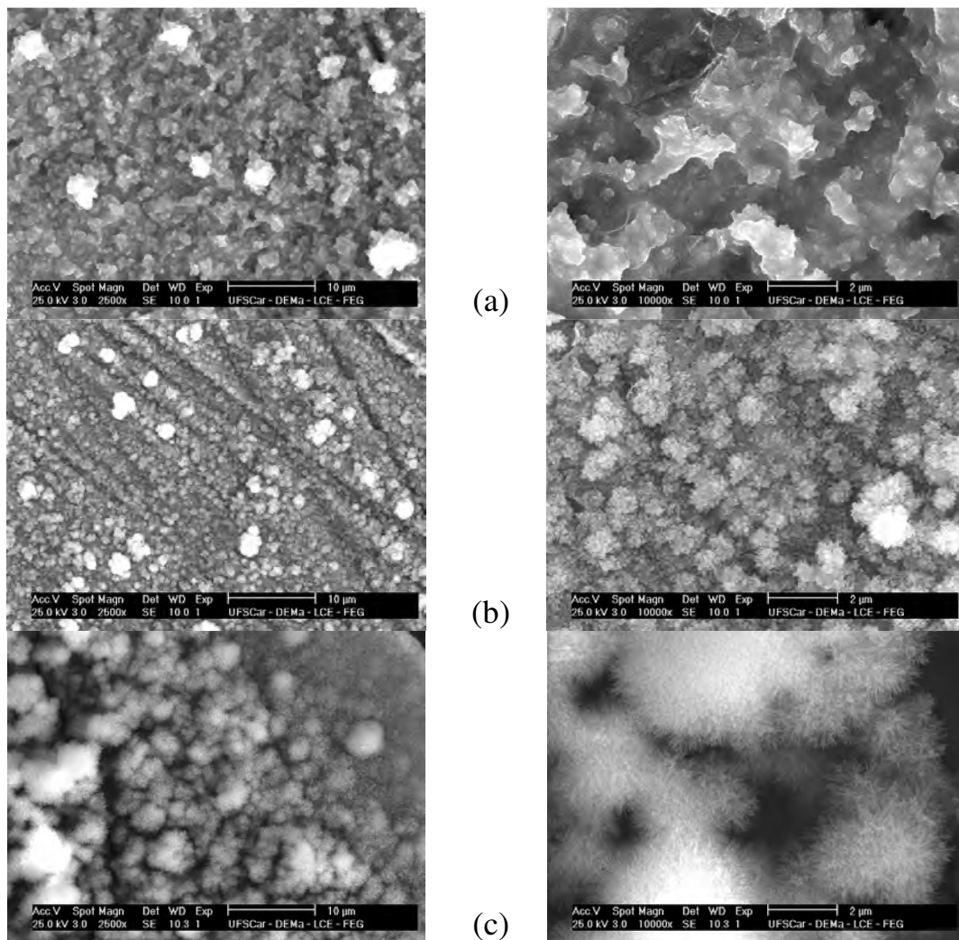
FIGURA 3.43: Micrografias de MEV dos filmes de HA eletrodepositadas a -13 \text{ mA cm}^{-2} a várias temperaturas sobre óxidos crescidos potenciodinamicamente até 8 V sobre a liga Ti-13Nb-13Zr em solução tampão fosfato: (a) temperatura ambiente, (b) 40 \text{ }^{\circ}\text{C} e (c) 60 \text{ }^{\circ}\text{C} .
