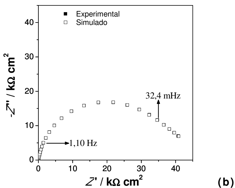
FIGURA 3.61: Espectros de EIE para a liga Ti-13Nb-13Zr com óxido natural e HA obtida por eletrodeposição, após 49 dias a circuito aberto em solução PBS.
