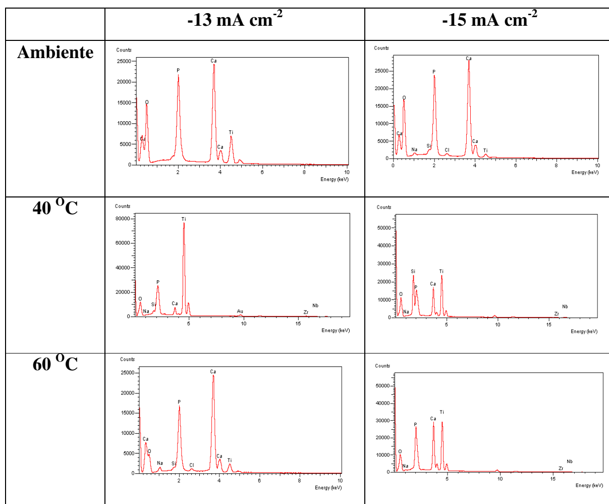
FIGURA 3.3: Espectros de EDS da superfície da liga Ti-13Nb-13Zr recoberta com apatita por eletrodeposição, obtidos em diferentes condições.
