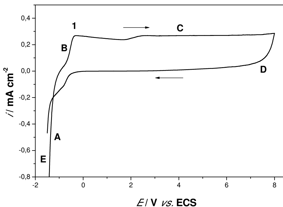
FIGURA 3.22: Voltametria cíclica para a liga Ti-13Nb-13Zr em solução de tampão fosfato (pH 5), a \nu = 50 \text{ mV s}^{-1} .
