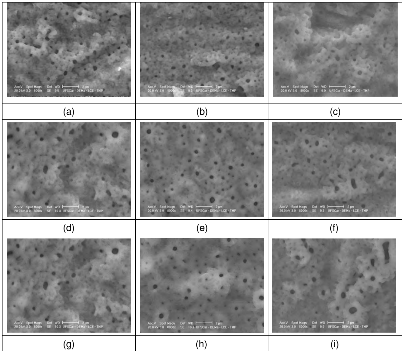
FIGURA 3. 21: Micrografias de MEV dos óxidos crescidos por micro-arco sobre a liga Ti-13Nb-13Zr em solução de tampão fosfato, a diferentes tempos de anodização e potenciais. a 240 V: (a) 60 s, (b) 300 s, (c) 600 s; a 270 V: (d) 60 s, (e) 300 s, (f) 600 s; a 300 V: (g) 60 s, (h) 300 s, (i) 600 s.
