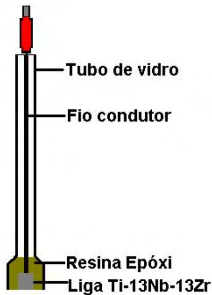
FIGURA 2.5 – Desenho esquemático do eletrodo de trabalho.
