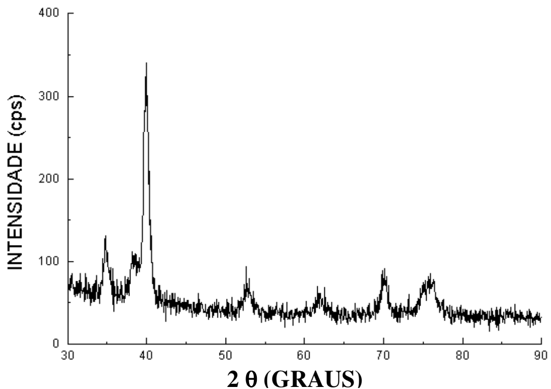
FIGURA A1 – Difratograma de raios X da liga Ti-13Nb-13Zr.
