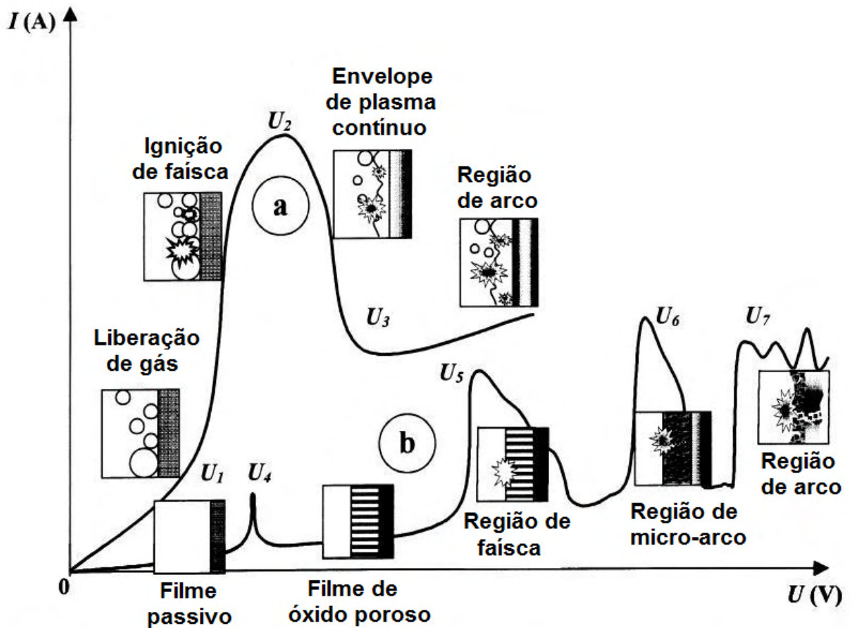
FIGURA 1.4: Diagramas de corrente-voltagem para dois tipos de processo de oxidação por micro-arco: fenômenos de descarga ocorrem (a) próximo ao eletrodo e (b) no filme formado sobre o eletrodo (YEROKHIN et al. , 1999).
