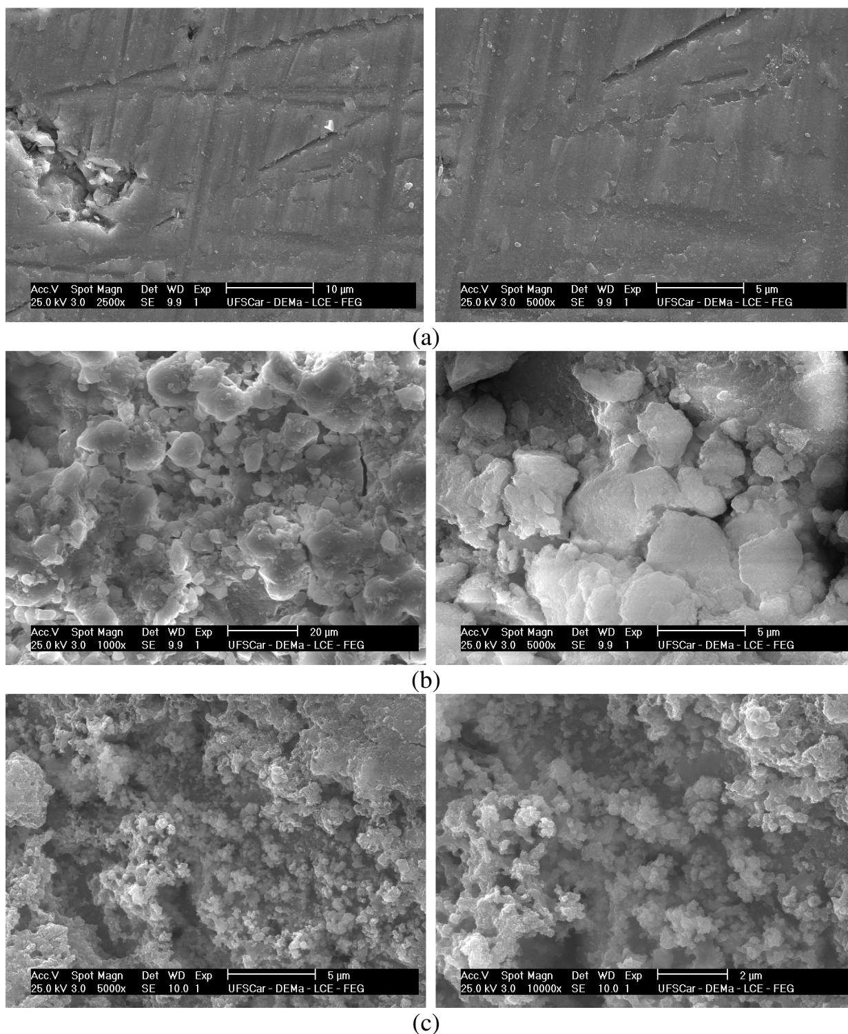
FIGURA 3.68: Micrografias de MEV da liga Ti-13Nb-13Zr recoberta por seu óxido natural e HA, após 49 dias de imersão em solução PBS. Sistemas: (a) liga/ox. natural; (b) liga/ox. natural/HA bio e (c) liga/ox. natural/HA eletro .
