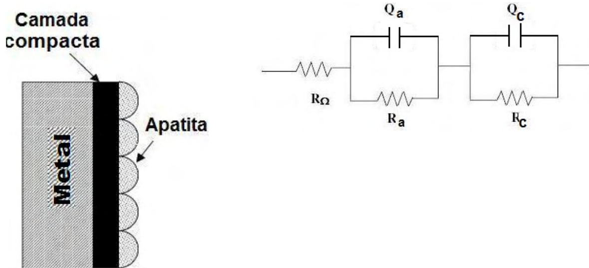
FIGURA 3.62: Representação esquemática das interfaces liga biocompatível/óxido natural/HA/solução, e circuito elétrico equivalente que representa estas interfaces.
