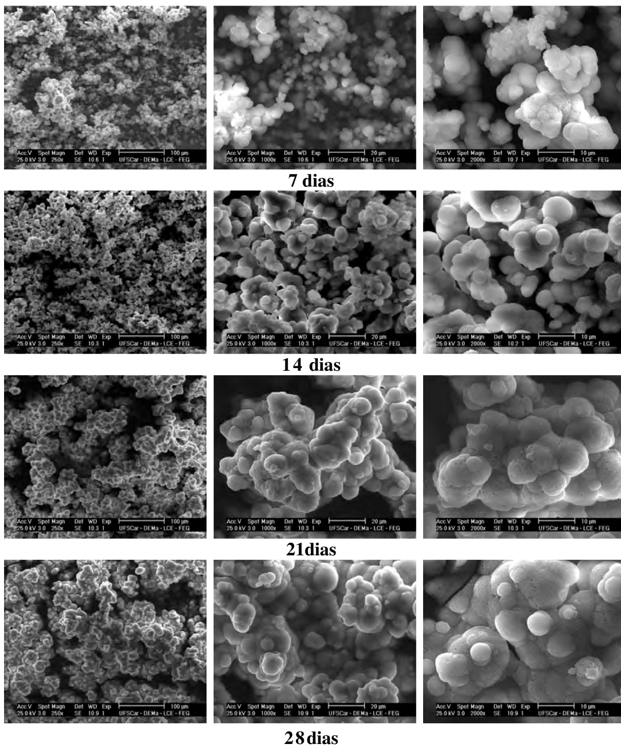
FIGURA 3.9: Micrografias de MEV da apatita depositada pelo método biomimético sobre a liga Ti-13Nb-13Zr por 7, 14, 21 e 28 dias, após o tratamento químico alcalino. Aumentos: 250, 1000 e 2000 x.
