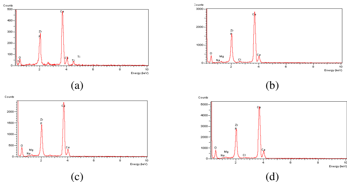
FIGURA 3.31: Espectros de EDS de HA formada biomimeticamente a diferentes tempos de imersão sobre óxidos crescidos por micro-arco a 300 V sobre a liga Ti-13Nb-13Zr em solução de tampão fosfato: (a) 7, (b) 14, (c) 21 e (d) 28 dias.
