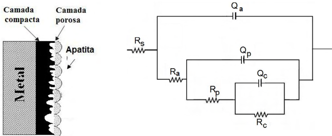
FIGURA 3.88: Representação esquemática das interfaces liga biocompatível/camada compacta/camada porosa/HA/solução, e circuito elétrico equivalente que representa estas interfaces.
