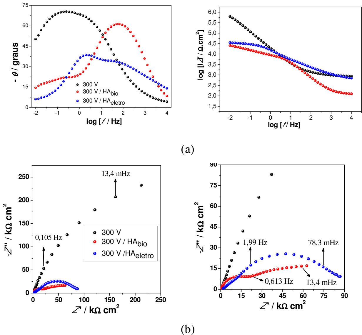
FIGURA 3.89: Comparação entre os espectros de EIE para a liga Ti-13Nb-13Zr recoberta por óxido crescido a 300 V com e sem recobrimento de HA, após 35 dias a circuito aberto em solução PBS. Diagramas: (a) Bode; (b) Nyquist.
