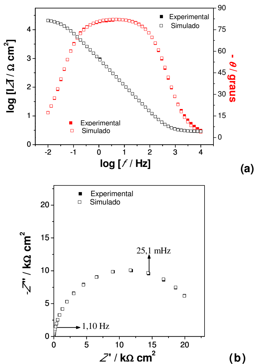
FIGURA 3.58: Espectros de EIE para a liga Ti-13Nb-13Zr com óxido natural, após 42 dias a circuito aberto em solução PBS. Diagramas: (a) Bode; (b) Nyquist.
