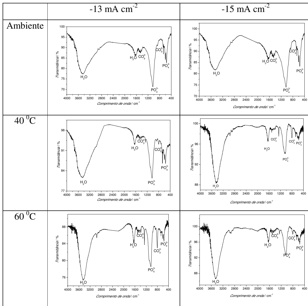
FIGURA 3.5: Espectros no infravermelho por transformada de Fourier dos revestimentos de apatita obtidos por eletrodeposição.
