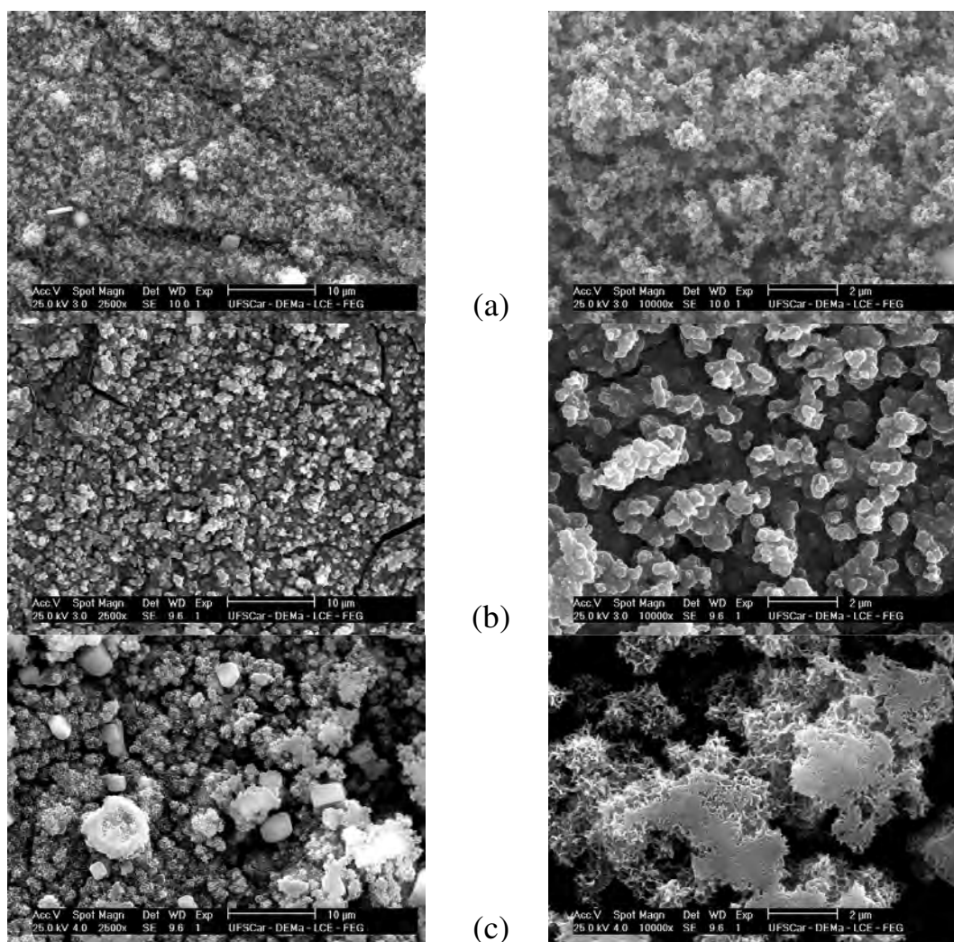
FIGURA 3.39: Micrografias de MEV dos filmes de HA eletrodepositadas a -13 \text{ mA cm}^{-2} a várias temperaturas sobre óxidos crescidos por micro-arco a 270 V sobre a liga Ti-13Nb-13Zr em solução tampão fosfato: (a) temperatura ambiente, (b) 40 °C e (c) 60 °C.
