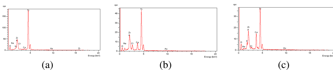
FIGURA 3.46: Espectros de EDS dos filmes de HA eletrodepositadas a -15 \text{ mA cm}^{-2} a várias temperaturas sobre óxidos crescidos por micro-arco a 240 V sobre a liga Ti-13Nb-13Zr em solução tampão fosfato: (a) temperatura ambiente, (b) 40 \text{ }^\circ\text{C} e (c) 60 \text{ }^\circ\text{C} .
