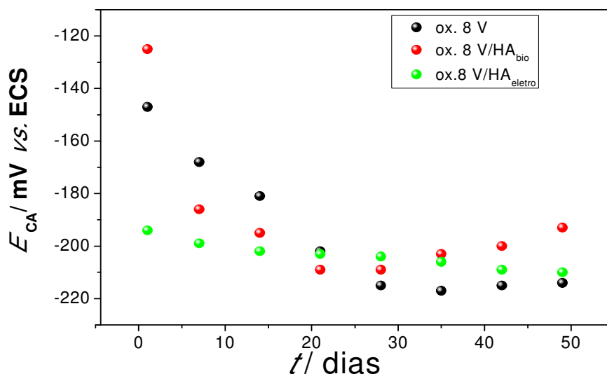
FIGURA 3.71: Potencial de circuito aberto para a liga Ti-13Nb-13Zr recoberta com óxido crescido até 8 V, com e sem recobrimento de fosfato de cálcio, em solução PBS.
