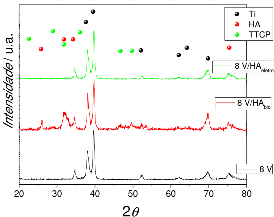
FIGURA 3.82: Difratoogramas de raios X da liga Ti-13Nb-13Zr após 49 dias de imersão em solução PBS. Sistemas: liga/ox. 8 V; liga/ox. 8 V/HA bio e liga/ox. 8 V/HA eleto .
