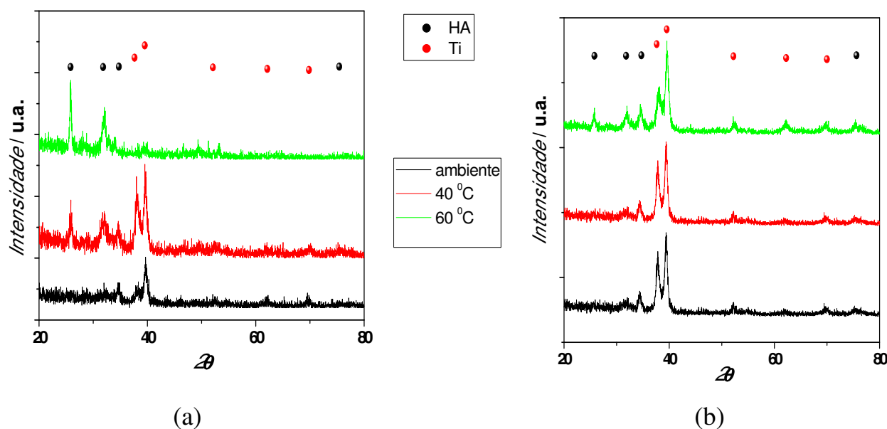
FIGURA 3.4: Difratogramas de raios X das apatitas formadas sobre Ti-13Nb-13Zr por eletrodeposição: (a) -13 \text{ mA cm}^{-2} e (b) -15 \text{ mA cm}^{-2} .
