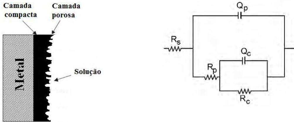
FIGURA 3.87: Representação esquemática das interfaces liga biocompatível/camada compacta/camada porosa/solução, e circuito elétrico equivalente que representa estas interfaces.
