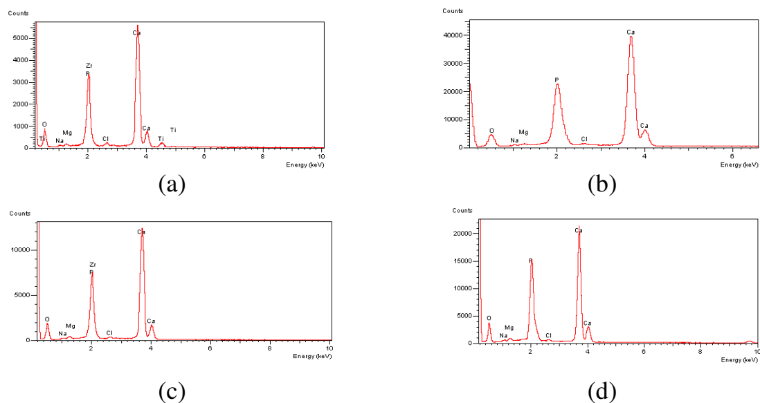
FIGURA 3.30: Espectros de EDS de HA formada biomimeticamente a diferentes tempos de imersão sobre óxidos crescidos por micro-arco a 270 V sobre a liga Ti-13Nb-13Zr em solução de tampão fosfato: (a) 7, (b) 14, (c) 21 e (d) 28 dias.
