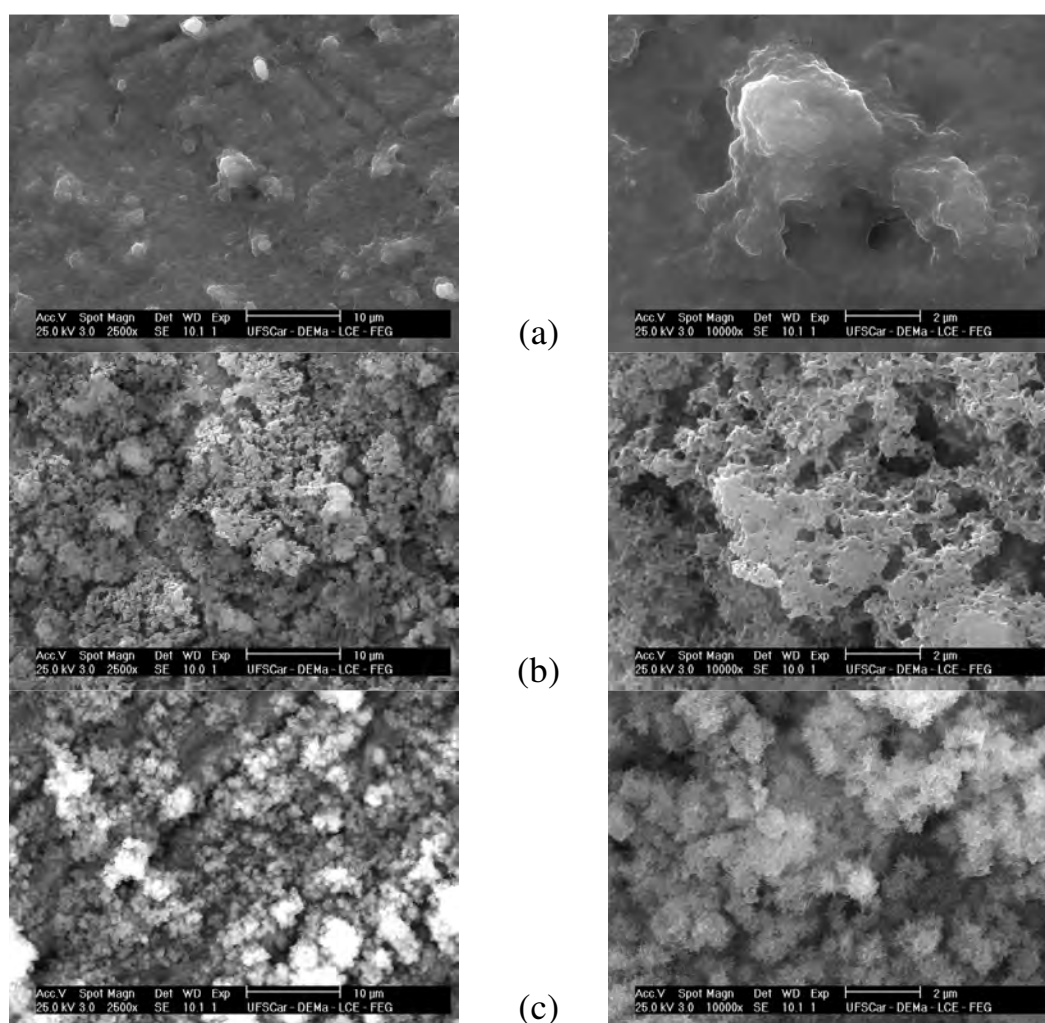
FIGURA 3.38: Micrografias de MEV dos filmes de HA eletrodepositadas a -15 \text{ mA cm}^{-2} a várias temperaturas sobre óxidos crescidos por micro-arco a 240 V sobre a liga Ti-13Nb-13Zr em solução tampão fosfato: (a) temperatura ambiente, (b) 40 \text{ }^\circ\text{C} e (c) 60 \text{ }^\circ\text{C} .
