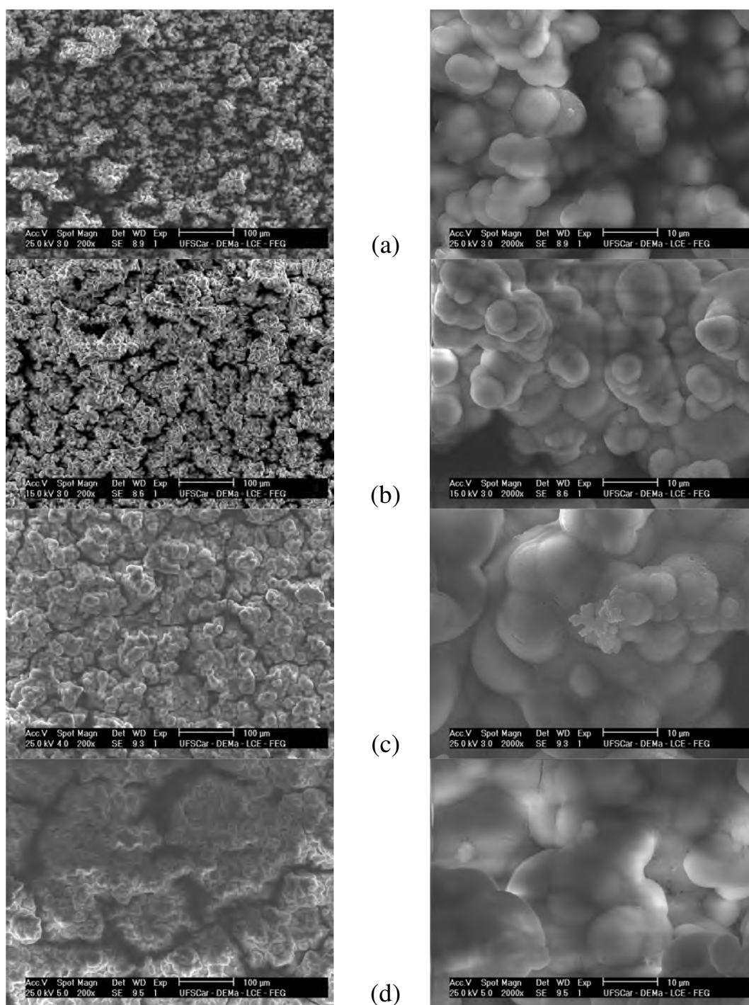
FIGURA 3.27: Micrografias de MEV dos óxidos crescidos por micro-arco a 300 V sobre a liga Ti-13Nb-13Zr em solução de tampão fosfato e cobertos com HA formada biomimeticamente a diferentes tempos de imersão: (a) 7, (b) 14, (c) 21 e (d) 28 dias.
