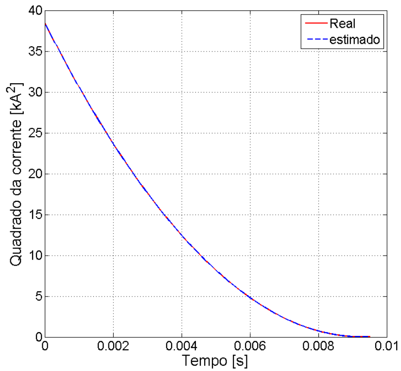
Figura 4.52: Quadrado da Corrente do arco dentro do Disjuntor-Thiel Modificado
