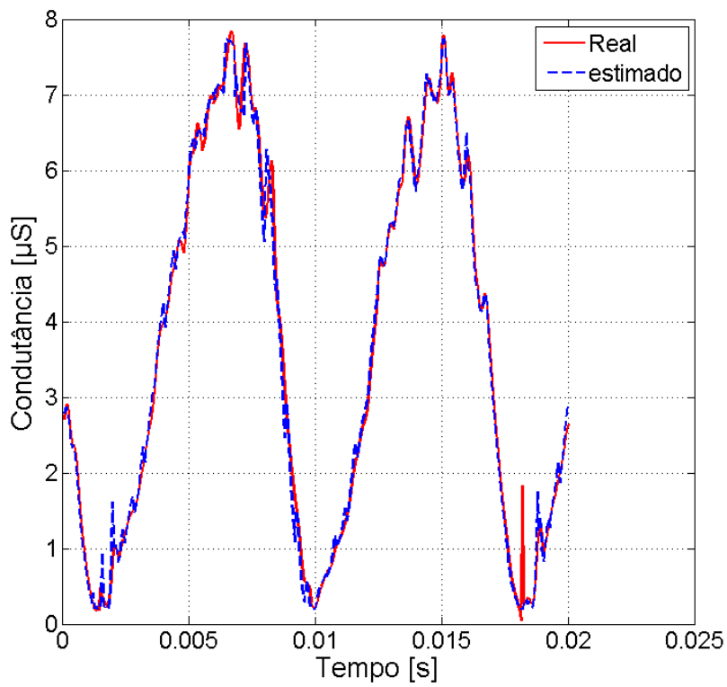
Figura 4.69: Condutância do arco no ar–Mayr-Portela
