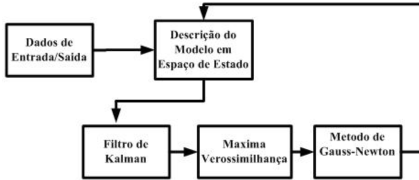
Figura 2.4: Diagrama geral da rotina de Estimação dual
