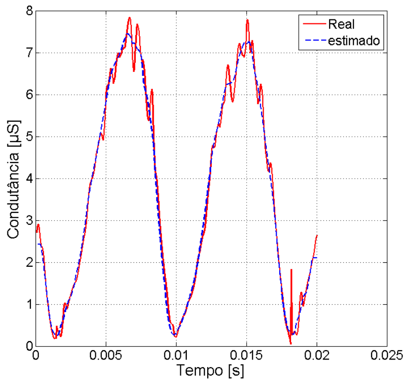
Figura 4.63: Condutância do arco no ar-Schwarz
