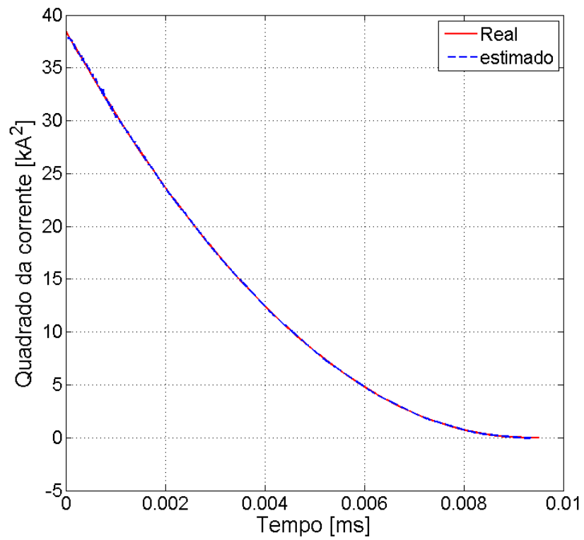
Figura 4.55: Quadrado da Corrente do arco no Disjuntor Mayr-Portela
