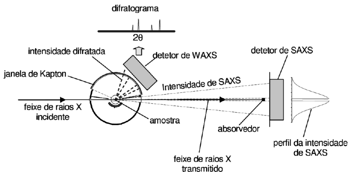
Esquema 3.2: Configuração experimental das análises simultâneas de SAXS e WAXS [62].
