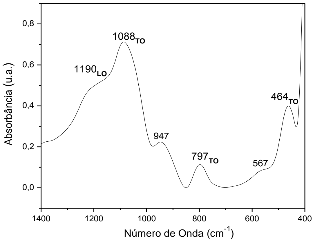
Figura 4.5: Bandas características das vibrações Si-O-Si para a amostra de sílica obtida por RA. Espectros adquiridos com 4 cm -1 de resolução. LO: modo óptico longitudinal; TO: modo óptico transversal.
