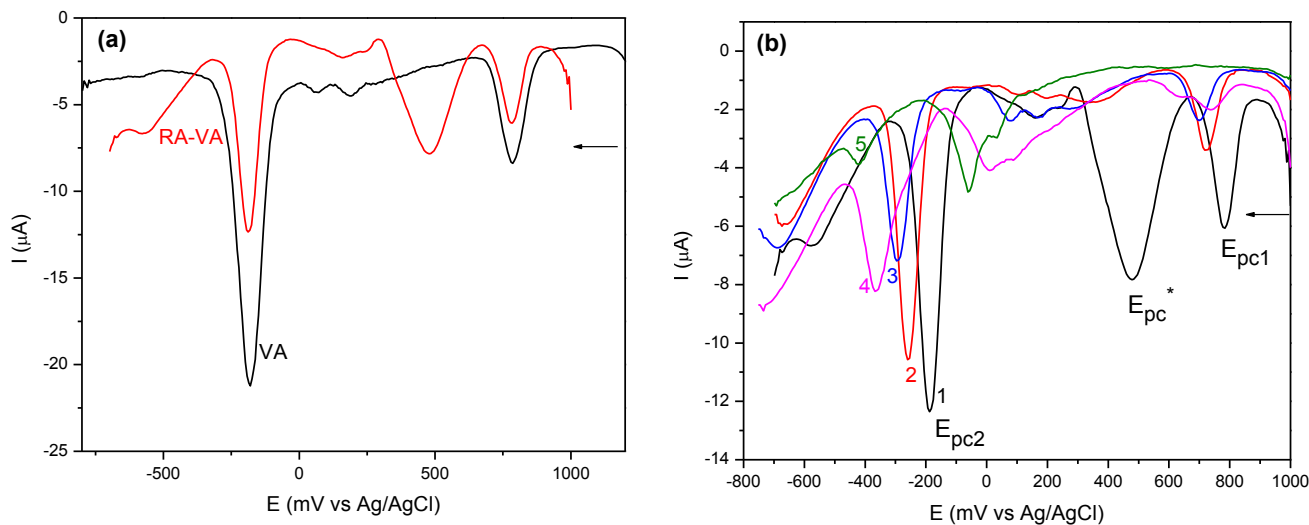
Figura 4.13: VPD do vermelho de alizarina 1 \times 10^{-3} \text{ mol L}^{-1} e eletrodo com a pasta de RAVA em solução aquosa de tampão BR. v = 100 \text{ mV s}^{-1} e varredura catódica. (a) pH = 1 (VA e RAVA) e (b) pH = 1 a 5.
