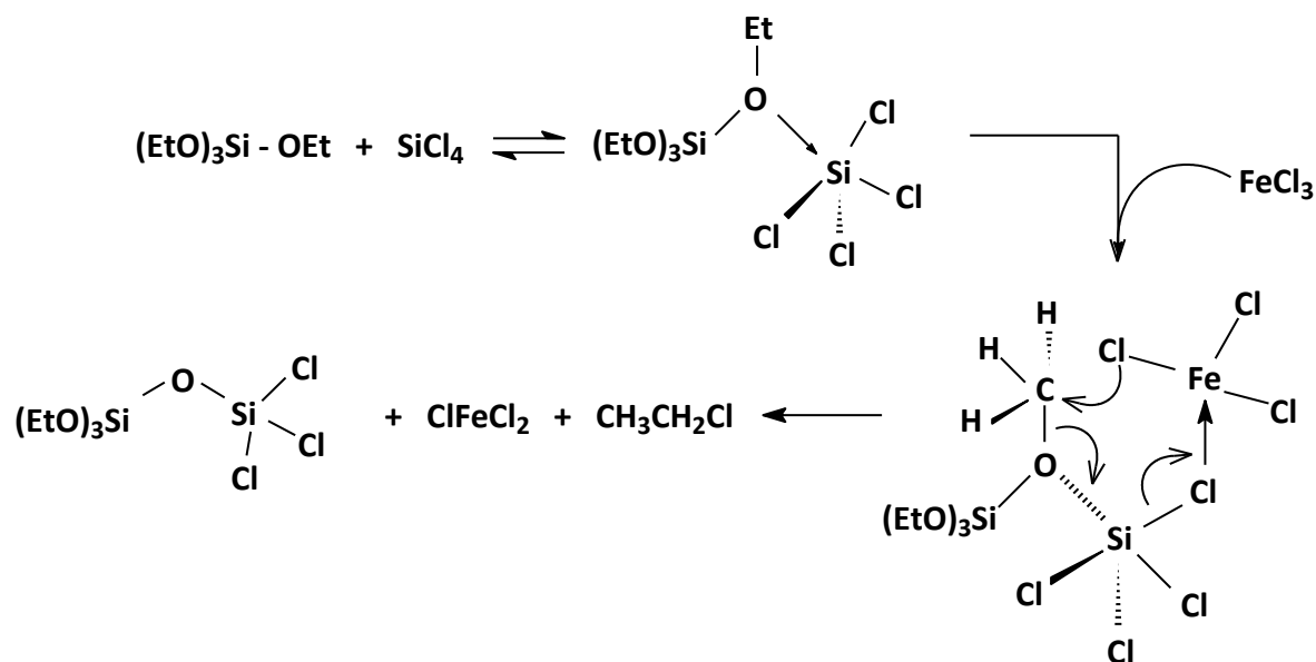
Esquema 1.5: Mecanismo proposto para a rota não-hidrolítica [15].
