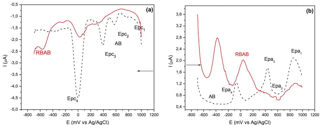
Figura 4.22: VPD do AB livre (---) e do eletrodo com a pasta de RBAB (—) (a) varredura catódica (b) varredura anódica em solução aquosa tampão BR (pH=2). v = 100 \text{ mV s}^{-1} .
