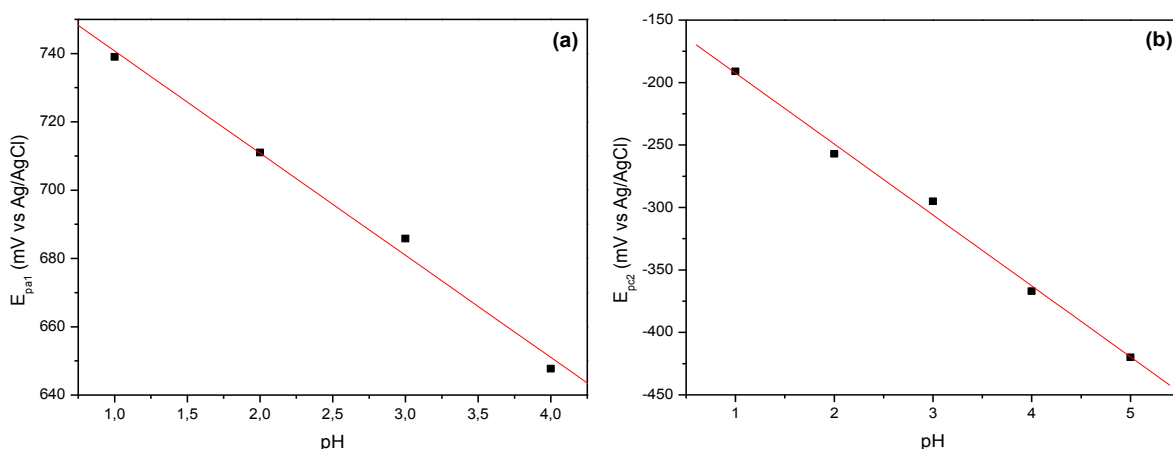
Figura 4.14: Correlação entre (a) E_{pa1} e (b) E_{pc2} versus pH 1 a 5 para RAVA.
