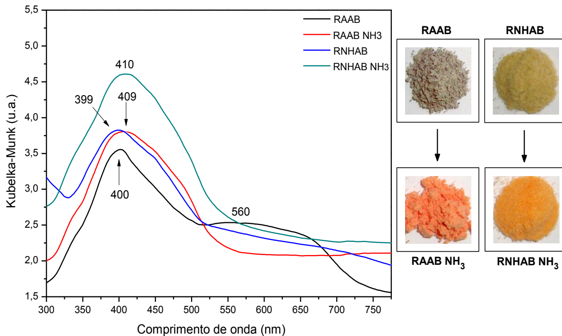
Figura 4.36: Espectros de DRS para as amostras RAAB e RNHAB e a coloração destas antes e após reação com gás amônia.
