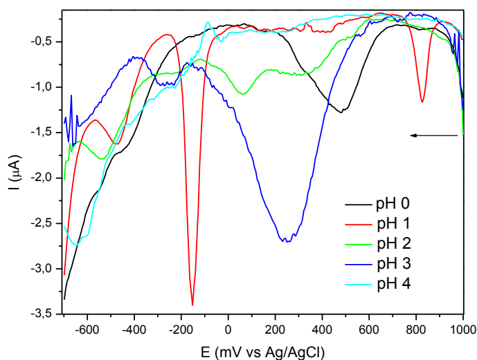
Figura 4.26: VPD do eletrodo contendo a pasta com RBAC em solução aquosa HCl/KCl (pH=0), NaBF 4 (pH=1) e de tampão BR (pH=2-4) ( v= 100 \text{ mV s}^{-1} ). Varredura catódica.
