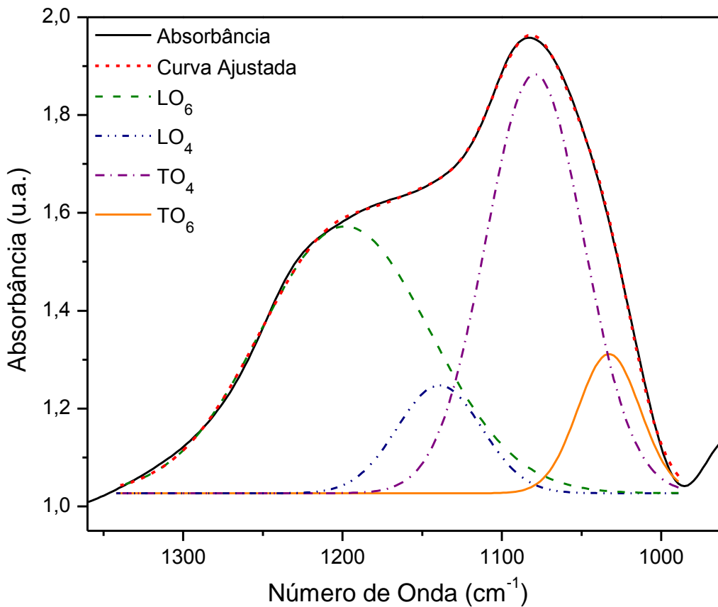
Figura 4.7: Deconvolução para a banda correspondente ao estiramento assimétrico da ligação Si-O-Si no espectro de FTIR da amostra RAAB.
