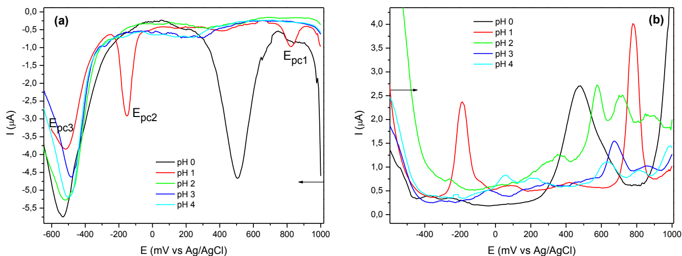
Figura 4.25: VPD do eletrodo com a pasta contendo RAAC (a) varredura catódica (b) varredura anódica em solução aquosa HCl/KCl (pH=0), NaBF 4 (pH=1) e de tampão BR (pH=2-4) ( v= 100 \text{ mV s}^{-1} ).
