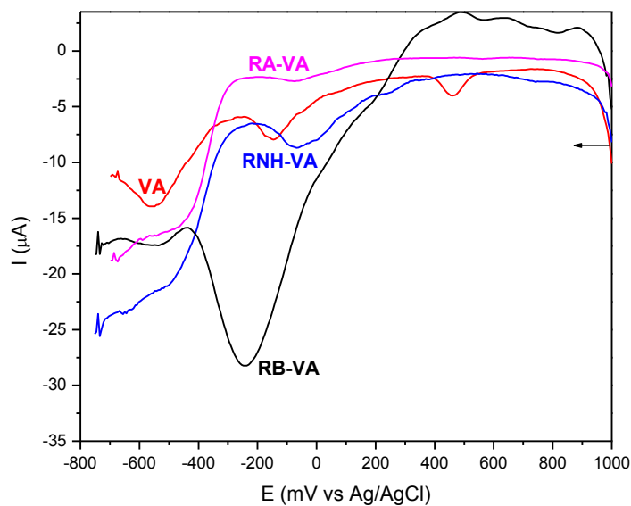
Figura 4.19: VPD do VA do eletrodo com a pasta dos sensores RA-VA, RNH-VA e RB-VA em solução aquosa de tampão BR pH= 7. v= 100 \text{ mV s}^{-1} e varredura catódica.
