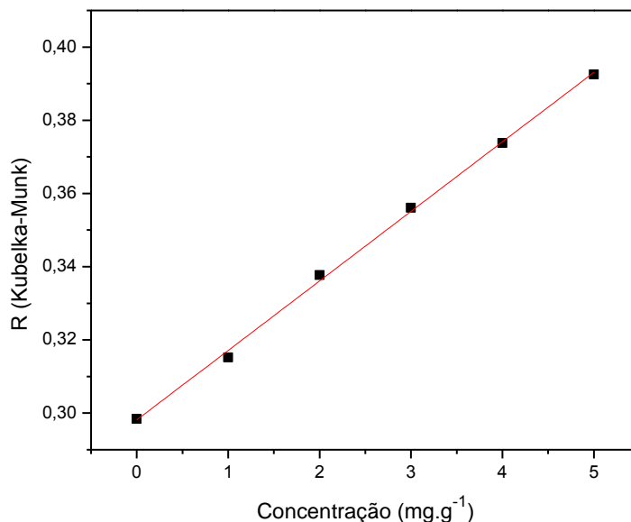
Figura 4.1: Curva de calibração obtida pelo método de adição de padrão para a amostra RNHAC.
