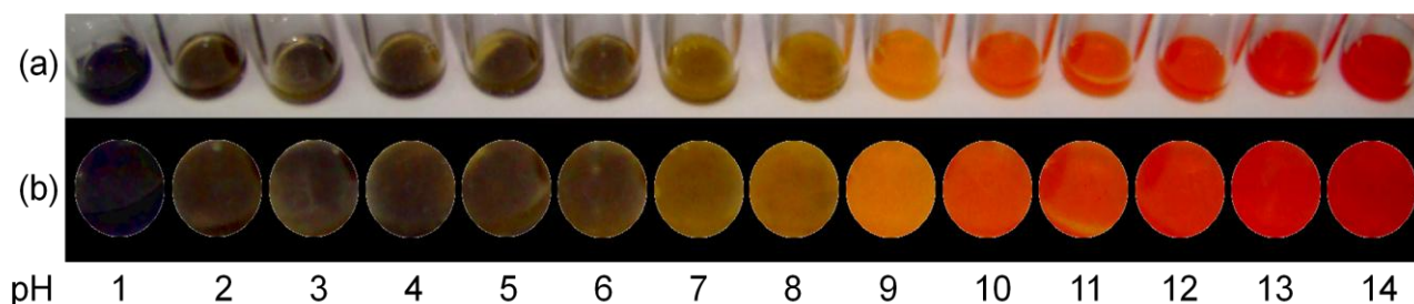
Figura 4.41: Resposta do sensor RAAB às soluções aquosas em pH de 1 a 14. (a) Fotografia do ensaio e (b) detalhe da série de cores obtida.
