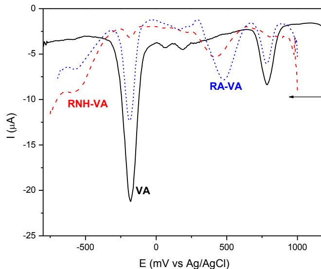
Figura 4.17: VPD do VA (—), do eletrodo contendo a pasta com RAVA (···) e RNHVA (---) em solução aquosa pH= 1. v = 100 \text{ mV s}^{-1} e varredura catódica.
