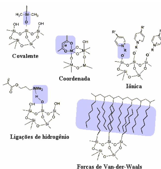
Esquema 1.8: Possíveis interações encontradas em materiais híbridos. Adaptado da referência [16].
