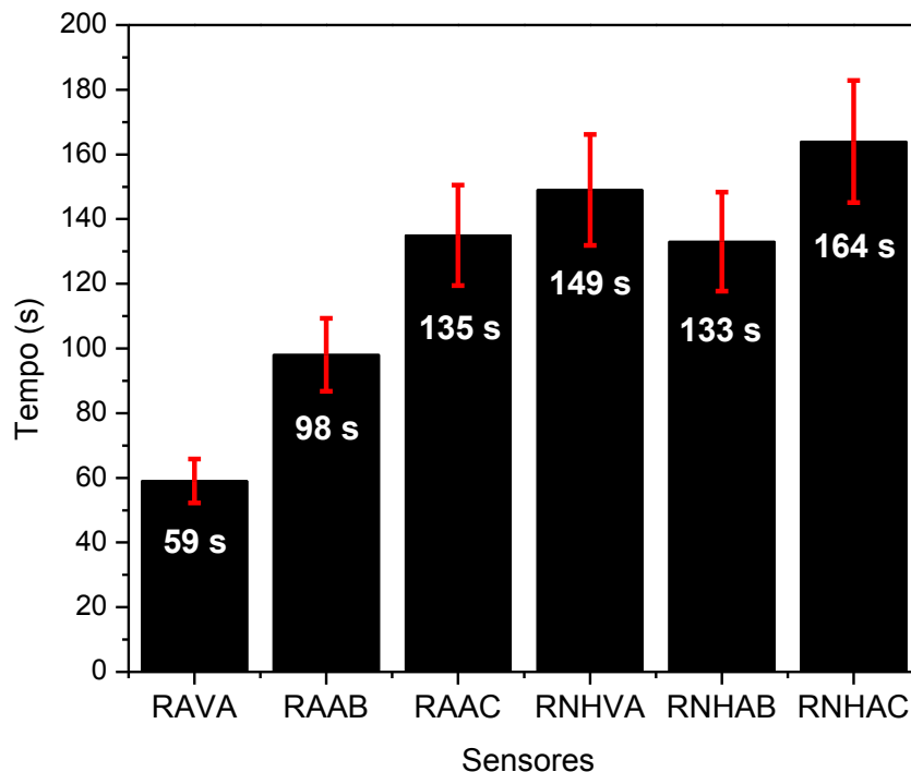
Figura 4.38: Tempo de resposta ao gás \text{NH}_3 dos sensores preparados pelas rotas RA e RNH. Desvio padrão de \pm 11.5\% .
