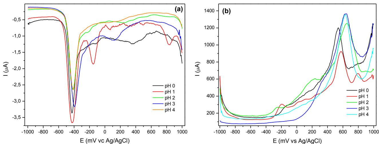
Figura 4.24: VPD da acridina 1 \times 10^{-3} \text{ mol L}^{-1} em solução aquosa de HCl/KCl pH =0, NaBF 4 pH=1 e de tampão BR pH 2 a 4 ( v= 100 \text{ mV s}^{-1} ) (a) varredura catódica e (b) varredura anódica.
