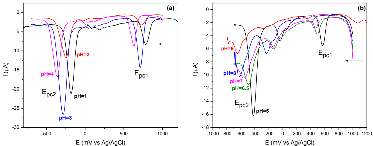
Figura 4.11: VPD do vermelho de alizarina 1 \times 10^{-3} \text{ mol L}^{-1} em solução aquosa de tampão BR. v = 100 \text{ mV s}^{-1} e varredura catódica. (a) \text{pH} = 1 a 4 e (b) \text{pH} = 5 a 9.
