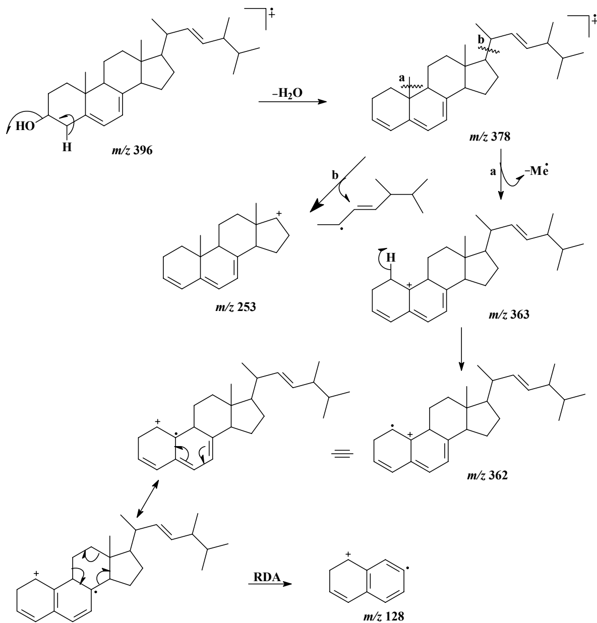
ESQUEMA 4.20: PROPOSTA DE FRAGMENTAÇÃO PARA S9
