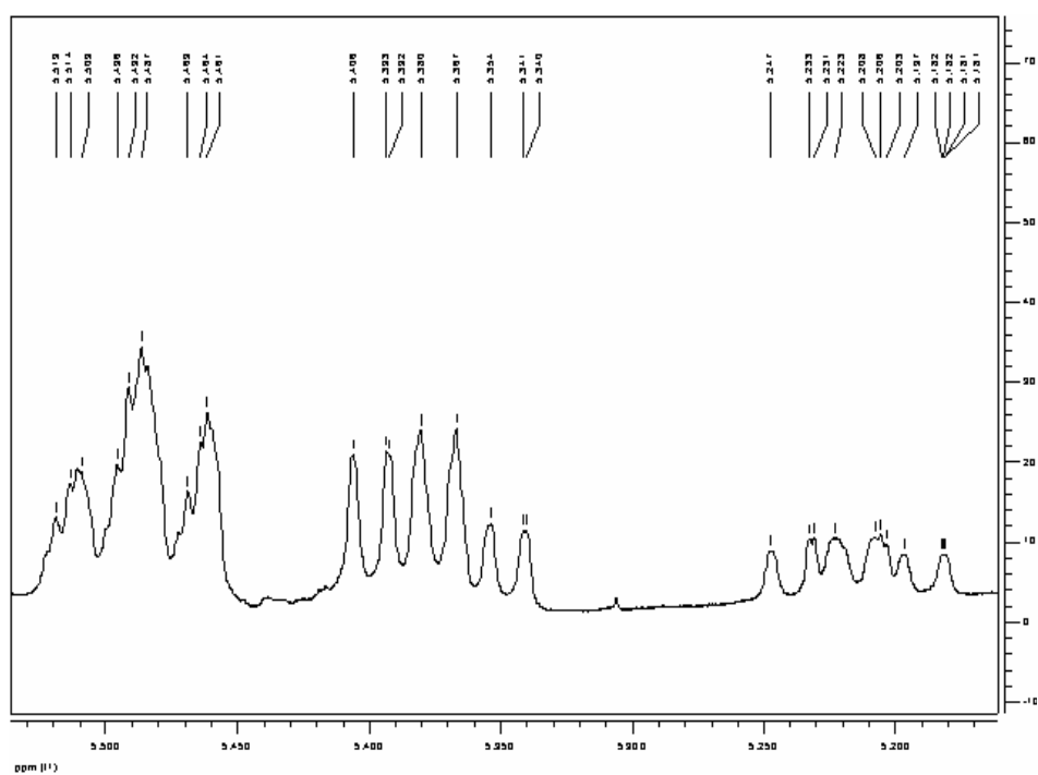
FIGURA 4.52: Expansão do espectro de RMN ^1\text{H} de S6 (400 MHz, \text{CDCl}_3 )
