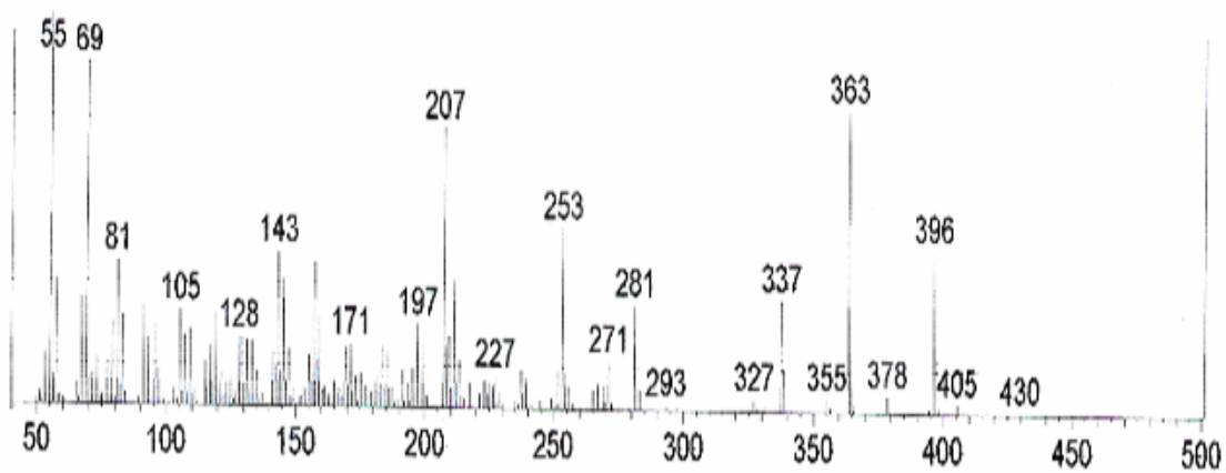
FIGURA 4.72: Espectro de CG/MS de S9
