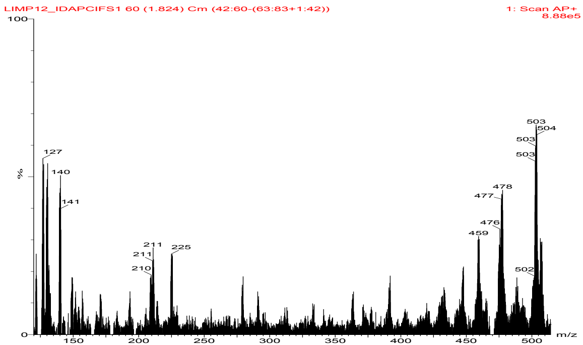
FIGURA 4.120: Espectro de massas (APCI + ) 23-hidroxi-20(22)-em-21,23-γ-lactona-angolensato de metila (P11)
