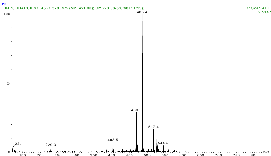
FIGURA 4.105: Espectro de massas (APCI + ) do 8β-hidroxicarapina 3,8-hemiacetal (P6)
