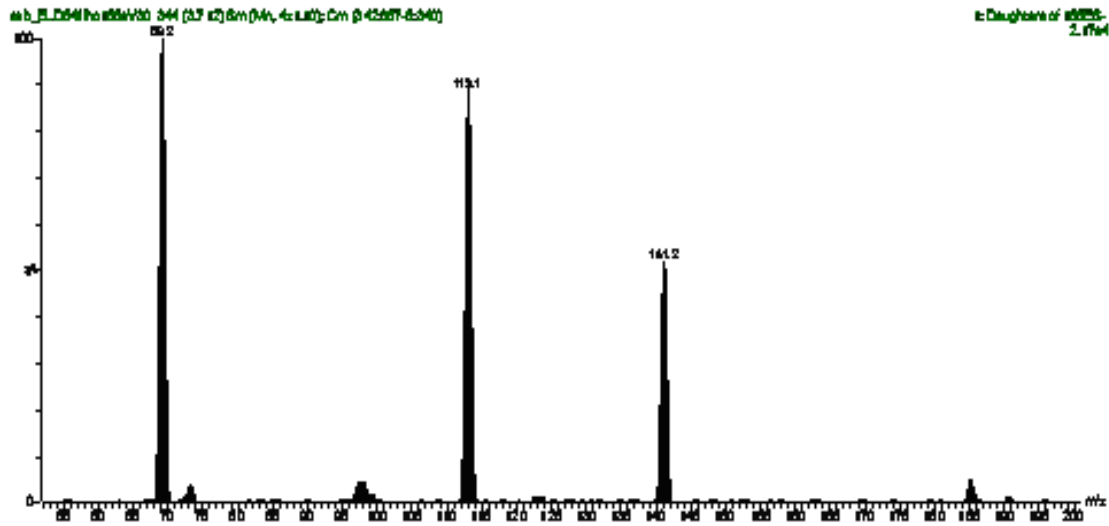
FIGURA 4.40: Espectro de massas Filhos do m/z 185,2 ( \text{ES}^- )
