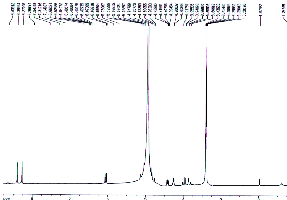
FIGURA 4.75: Espectro de RMN 1 H de S12 (200 MHz, MeOD)
