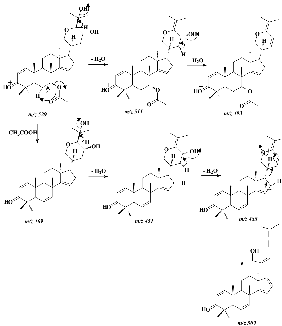
FIGURA 4.125: Proposta de fragmentação para o Grandifoliolenona (P12)
