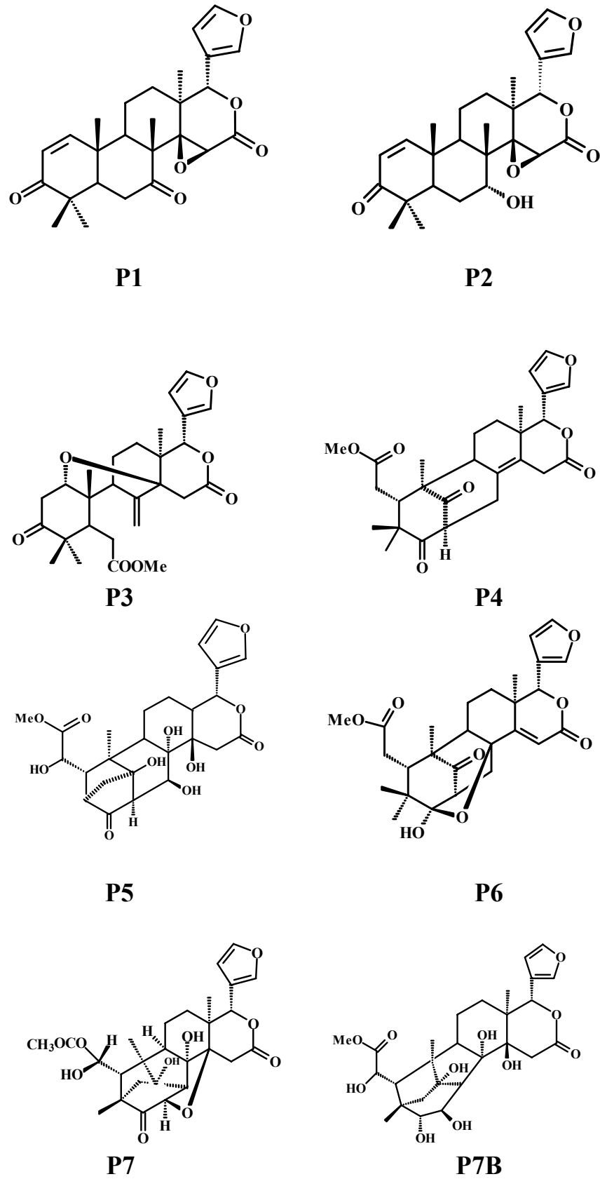
FIGURA 4.89: Limonóides utilizados como padrões para análise de seus espectros de massas
