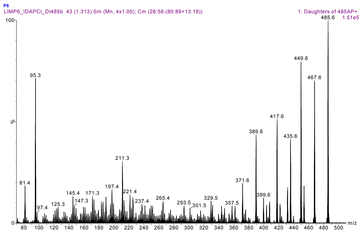
FIGURA 4.106: Espectro de massas (APCI + ), íons filhos de m/z 485 do 8β-hidroxicarapina 3,8-hemiacetal (P6)
