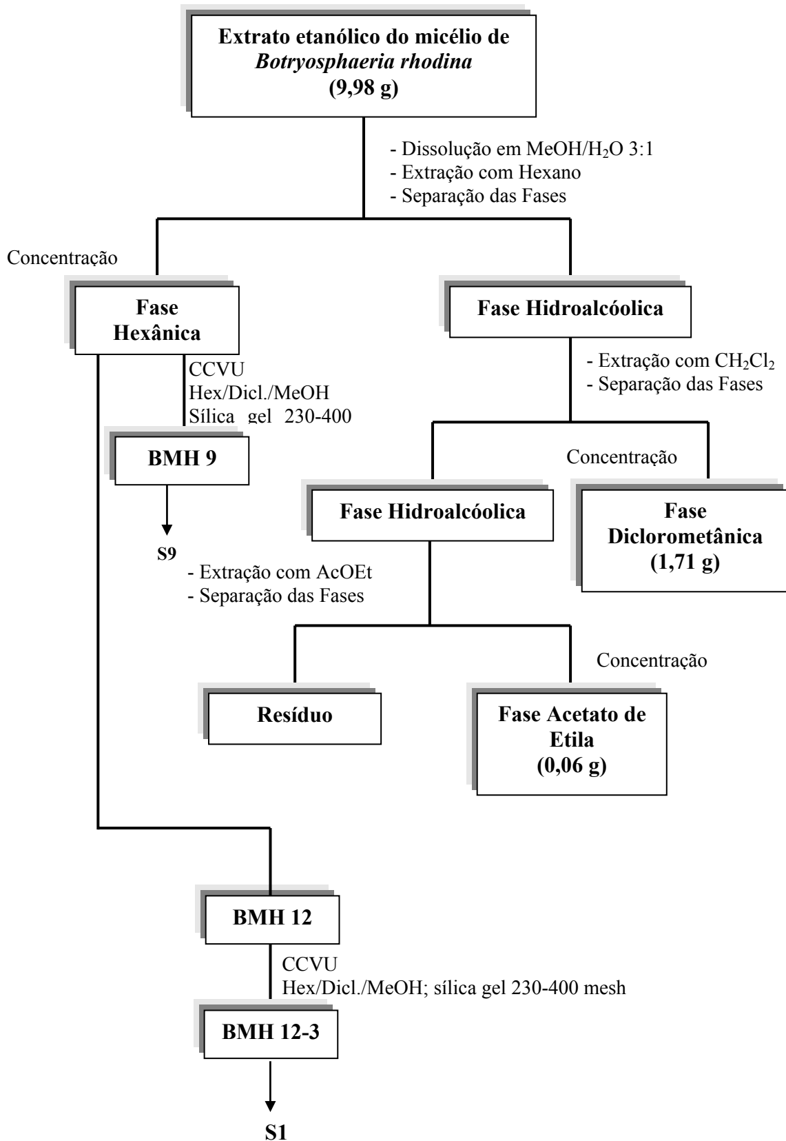
FLUXOGRAMA 3.6: Partição líquido-líquido do extrato etanólico do micélio
