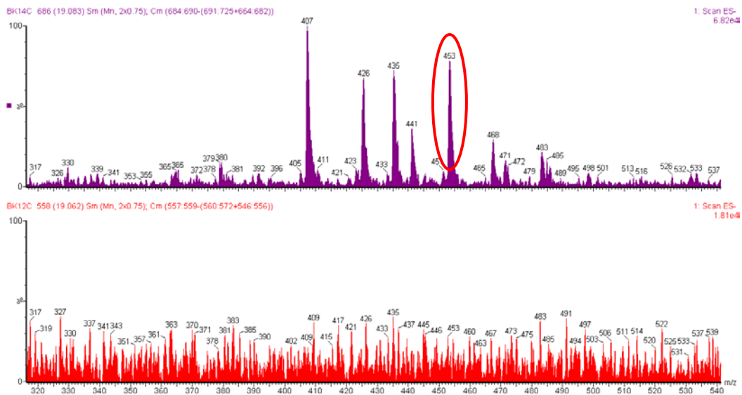
FIGURA 4.146: Espectro de massas ( ES^- ) Meio + Botryosphaeria rhodina + angolesato de metila (BK14C) e Meio + Botryosphaeria rhodina (BK12C)
