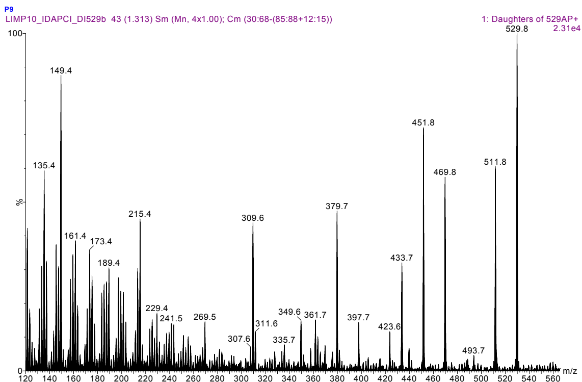
FIGURA 4.118: Espectro de massas ( APCI^+ ), íons filhos de m/z 529 do acetato de sapelina E (P9)
