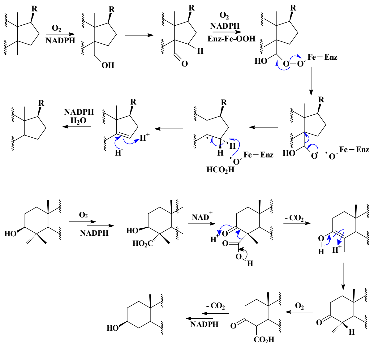
ESQUEMA 4.24: Perda de três grupos metílicos em esteróides (DEWICK 2004)
