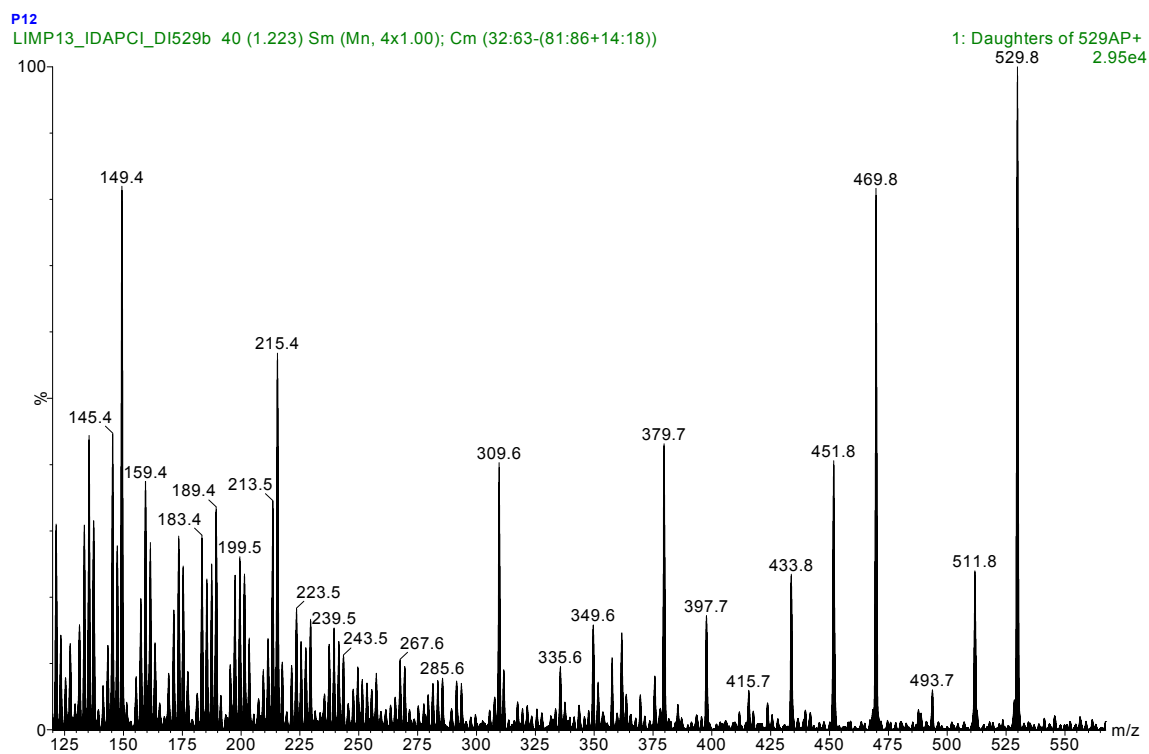
FIGURA 4.124: Espectro de massas ( APCI^+ ), íons filhos de m/z 529 do Grandifoliolenona (P12)
