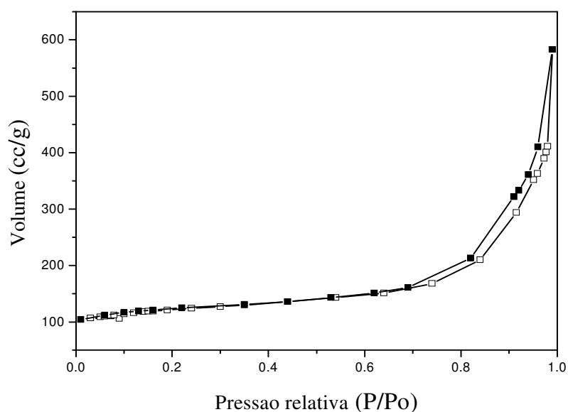
Figura 50. Isotherma de adsorção de N_2 da zeólita beta sintetizada em 7 dias.
