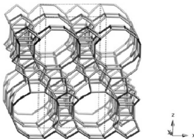
Figura 49. Estrutura da zeólita Beta.
