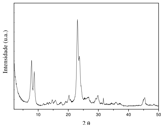
Figura 52. Difratoograma de raios-X da zeólitas beta sintetizada com a utilização de semente.
