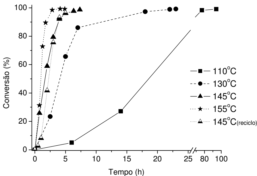
Figura 65. Variação da conversão do epóxido de alil-glicidila com o tempo de reação com CO 2 a 50 atm, temperaturas de 110 a 155 °C empregando 0,250 gramas de zeólita beta e 40mmols de AGE.
