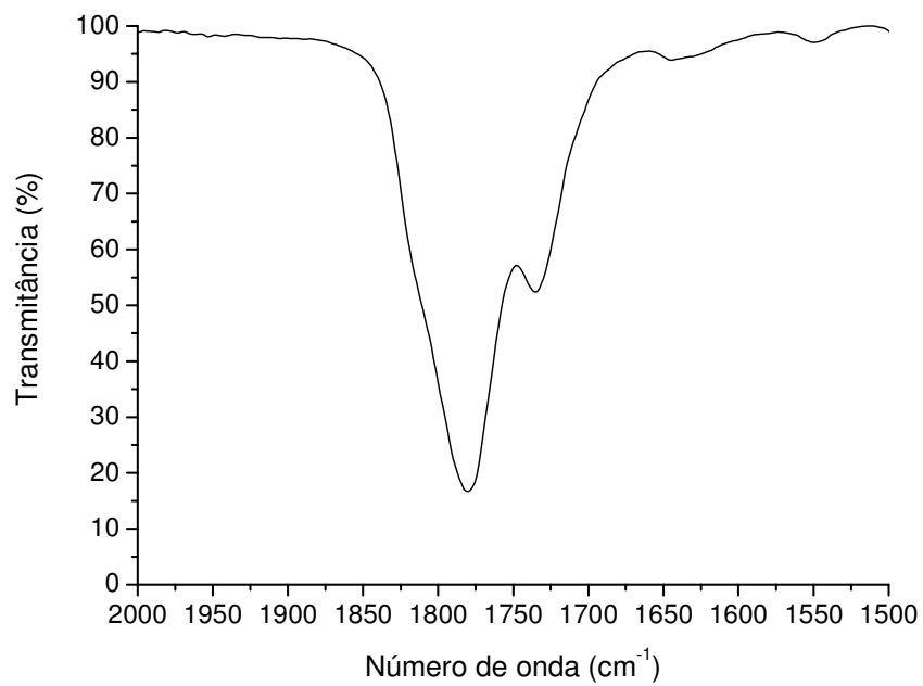
Figura 74. Espectrograma na região do infravermelho do APC.
