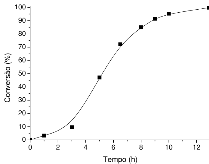
Figura 67. Variação da conversão do epóxido de alil-glicidila com o tempo de reação com CO 2 a 50 atm e 145 °C.
