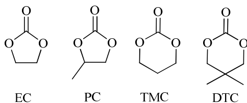
Figura 33: Carbonatos destaque para polimerização por abertura de anel.
