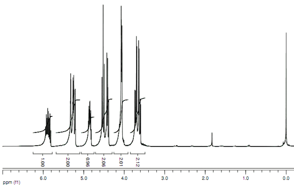
Figura 43. Espectro de ressonância magnética nuclear ^1\text{H} a 300 MHz em \text{CDCl}_3 do carbonato de alil glicidila.
