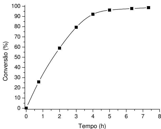
Figura 59. Variação da conversão do epóxido de alil-glicidila com o tempo de reação com CO 2 a 50 atm e a 145 °C.
