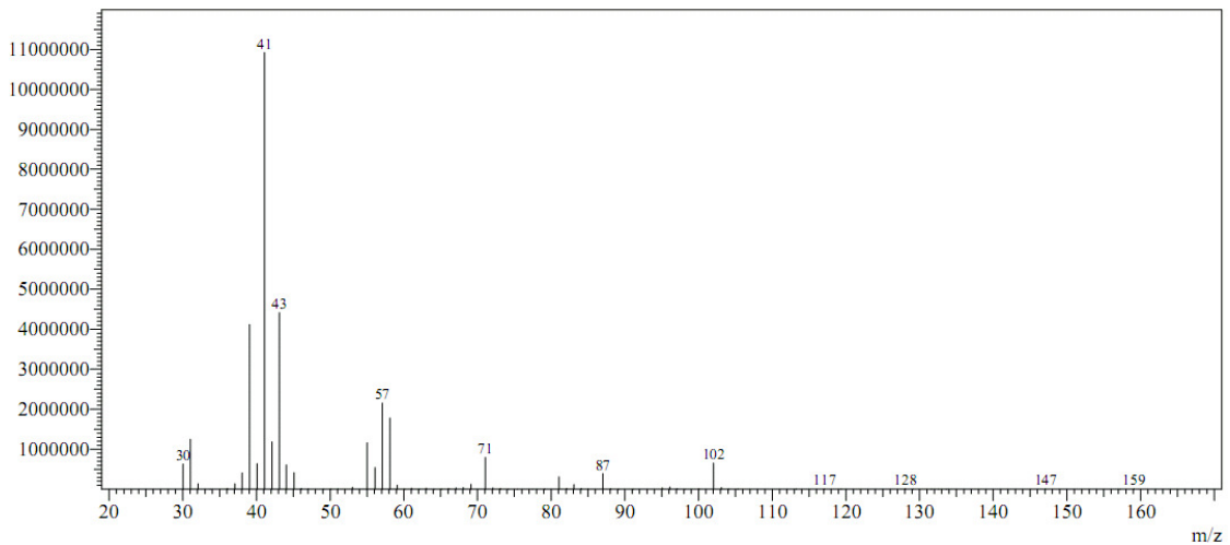
Figura 44. Análise de espectrometria de massas do carbonato de alil glidila.
