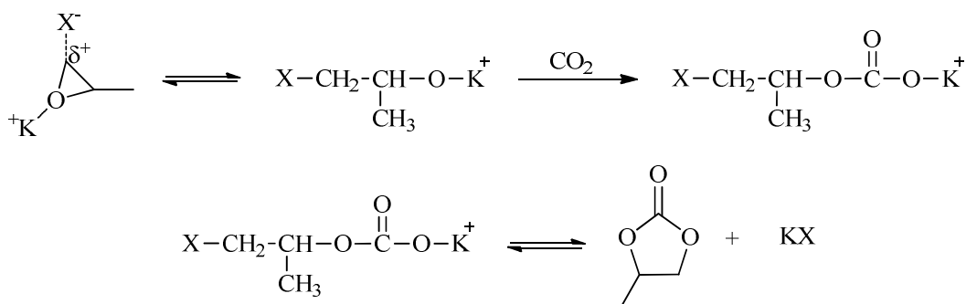
Figura 12. Mecanismo de formação de carbonatos cíclicos usando metais alcalinos.
