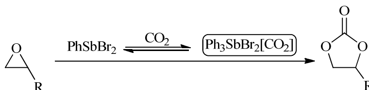
Figura 15: Síntese de carbonatos cíclicos usando catalisadores de antimônio.
