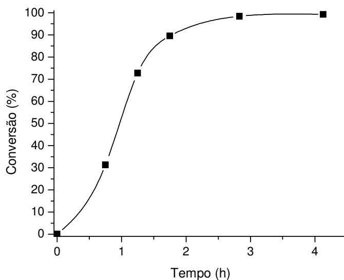
Figura 60. Variação da conversão do epóxido de alil-glicidila com o tempo de reação com CO 2 a 50 atm e 155 °C.
