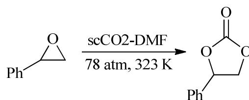
Figura 21: Síntese de carbonatos cíclicos empregando dióxido de carbono supercrítico.
