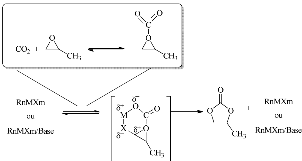
Figura 16: Formação de estado hexacoordenado na formação de carbonatos cíclicos empregando catalisadores de estanho 59 .
