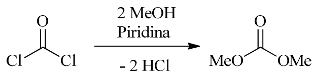
Figura 8: Síntese de dimetilcarbonato usando fosgênio.
