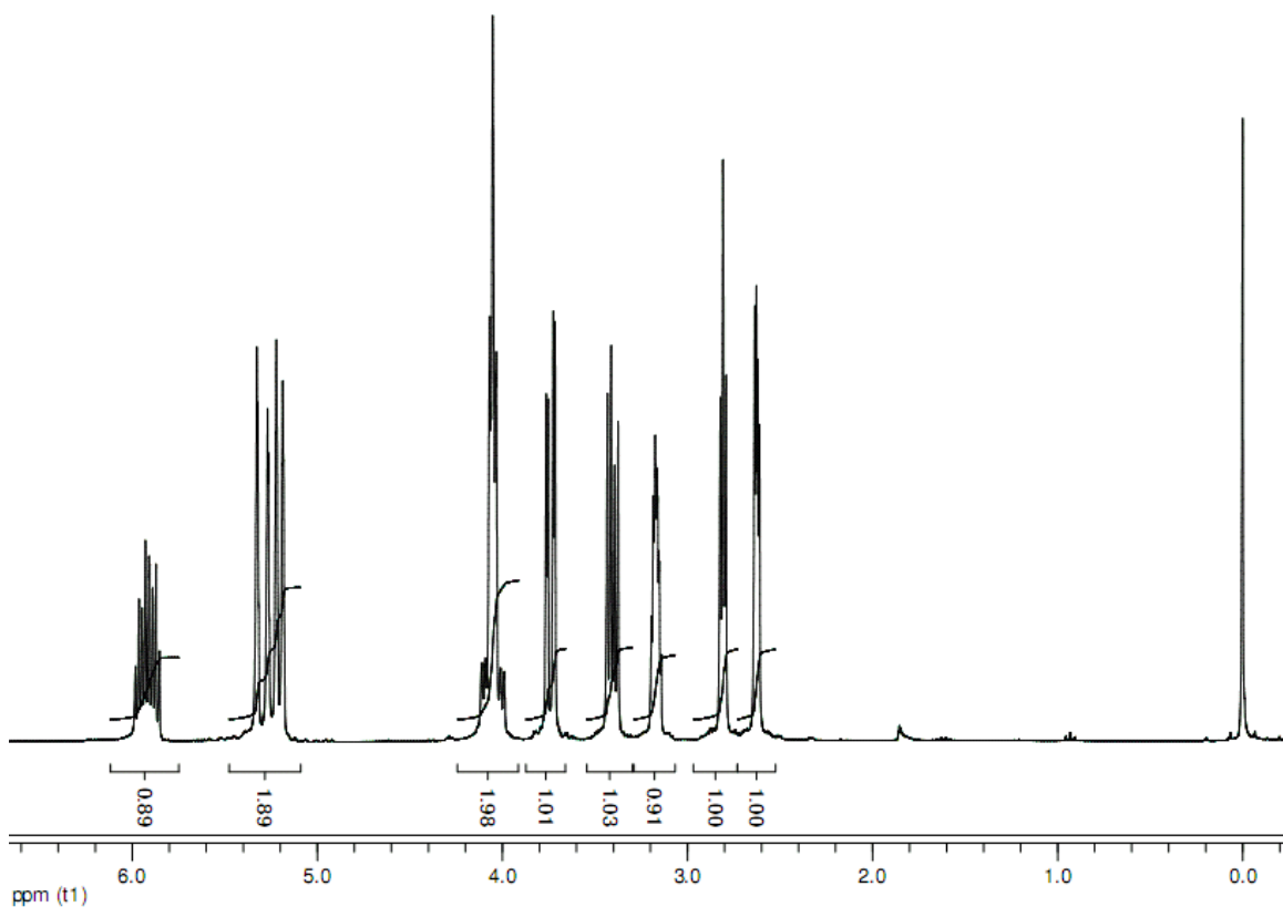
Figura 40. Espectro de ressonância magnética nuclear 1 H a 300 MHz em CDCl 3 do epóxido de alil-glicidila.
