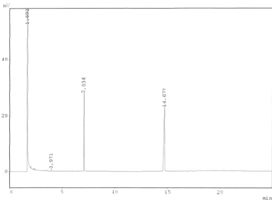
Figura 45. Cromatograma gasoso típico de análise de conversão nos testes catalíticos realizados.
