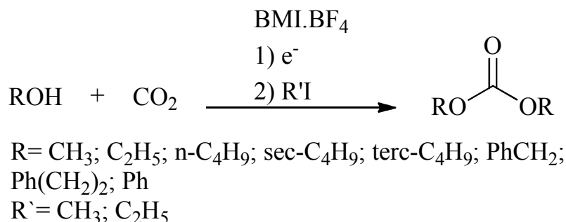
Figura 9: Síntese eletroquímica de alquil carbonatos.
