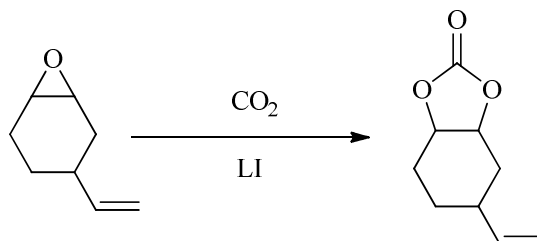
Figura 20. Síntese do carbonato de vinilciclohexeno.
