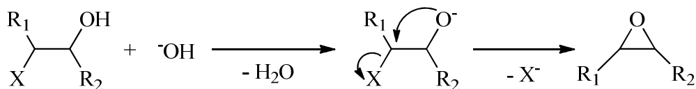
Figura 6: Formação epóxido via 1,2 haloidrina.
