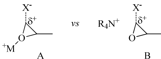
Figura 11: Interações de epóxidos com metais e sais de amônio quaternários.
