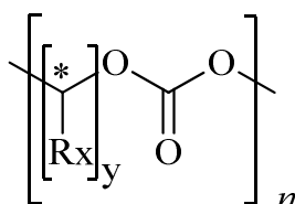
Figura 32: Estrutura geral de policarbonatos alifáticos.
