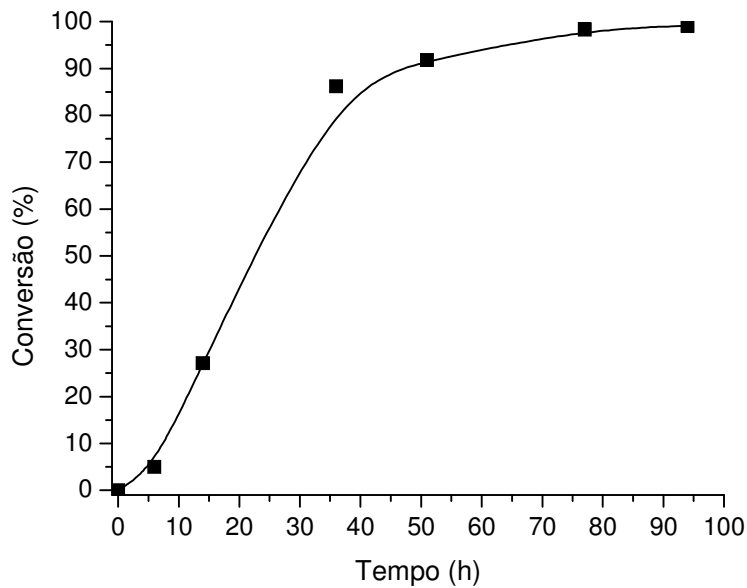
Figura 57. Variação da conversão do epóxido de alil-glicidila com o tempo de reação com CO 2 a 50 atm e a 110 °C.
