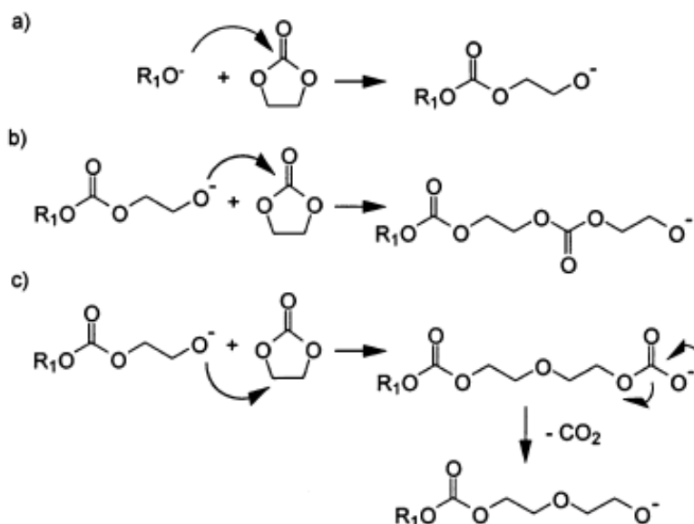
Figura 34: (a) Abertura do EC por espécie aniônica. (b) Propagação via ataque a carbonila, formando ligação carbonato. (c) Propagação via ataque alquilênico formando uma ligação éter e perda de CO 2 .
