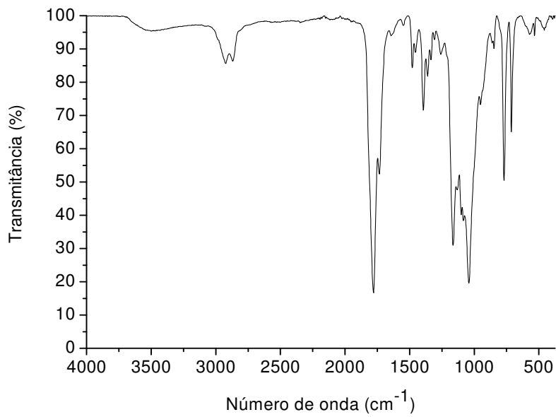
Figura 73. Espectrograma na região do infravermelho do APC.
