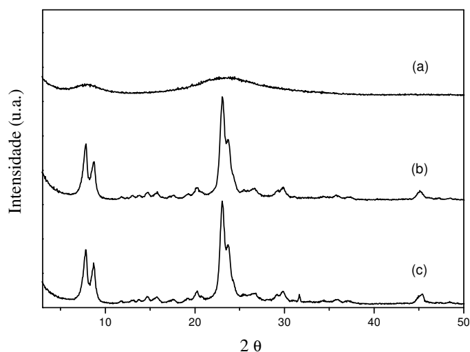
Figura 48. Difratoogramas de raios-X do material sintetizado utilizando [C4MIm.Cl], 150°C, Si/Al = 20 e agitação mecânica; (a) 3 dias, (b) 7 dias e (c) 14 dias de síntese.
