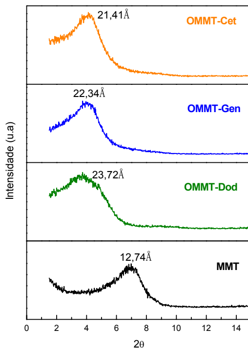
Figura 18: Difratogramas da argila sem tratamento (MMT) e da argila tratada com os sais Dodigen (OMMT-Dod), Genamin (OMMT-Gen) e Cetremide (OMMT-Cet).
