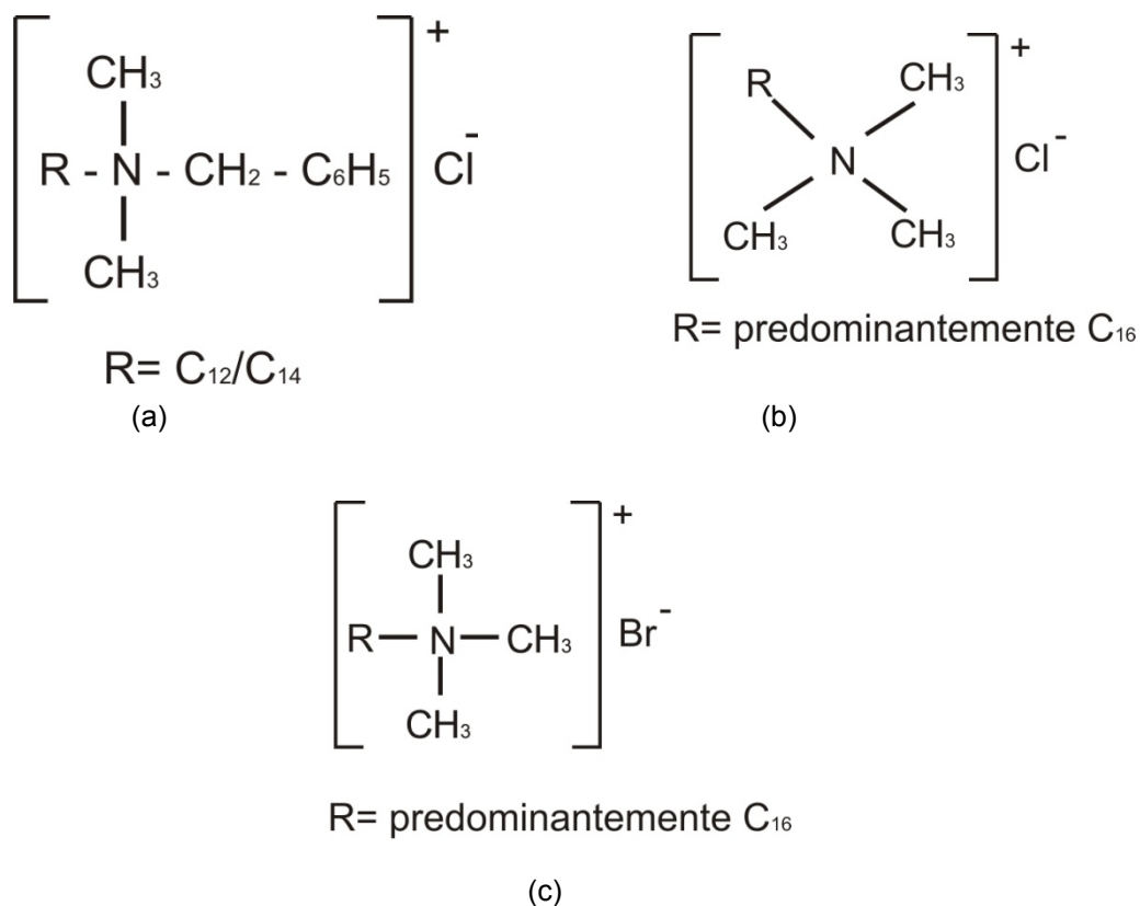
Figura 13: Estrutura molecular dos sais quaternários de amônio: (a) Dodigen, (b) Genamin e (c) Cetremide.
