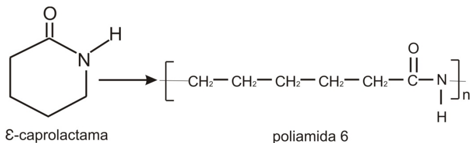
Figura 2: Representação esquemática da polimerização do nylon 6 pela abertura do anel.
