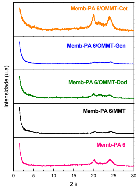
Figura 30: Difratomogramas das membranas de poliamida 6 e das membranas obtidas a partir de seus nanocompósitos, com maior teor de ácido.
