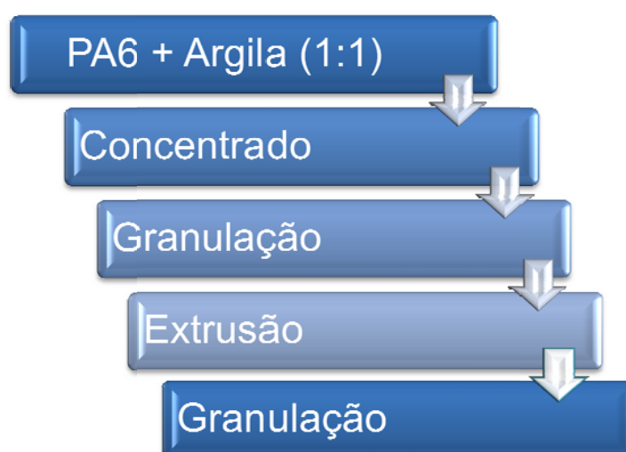
Figura 15: Fluxograma da preparação dos nanocompósitos de poliamida 6/argila.
