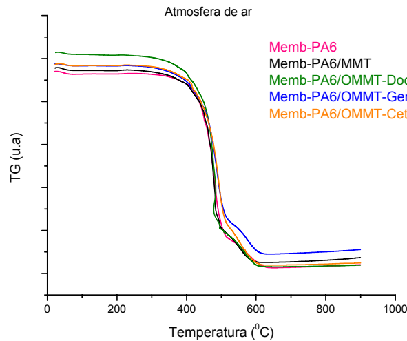
Figura 34: Curvas de TG das membranas obtidas a partir da poliamida 6 e de seus nanocompósitos, com maior teor de ácido.
