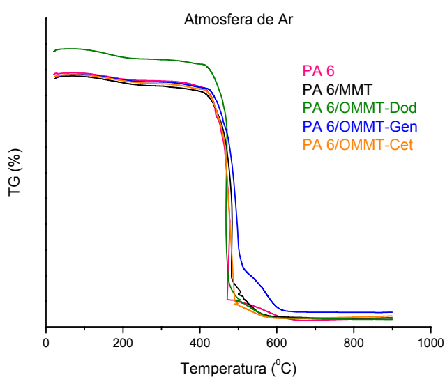
Figura 27: Curvas de TG da poliamida 6 e de seus nanocompósitos.
