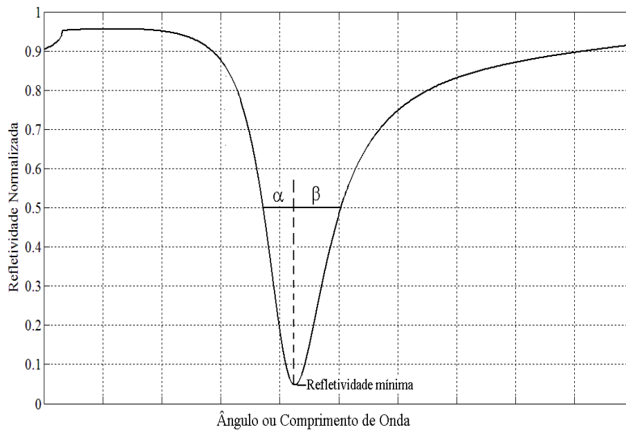
Figura 2.3: Curva de refletividade, com o mínimo de refletividade na condição de ressonância SPR e parâmetros característicos da curva.
