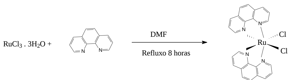
ESQUEMA 1. Rota sintética para obtenção do complexo cis - \text{RuCl}_2(\text{phen})_2 .
