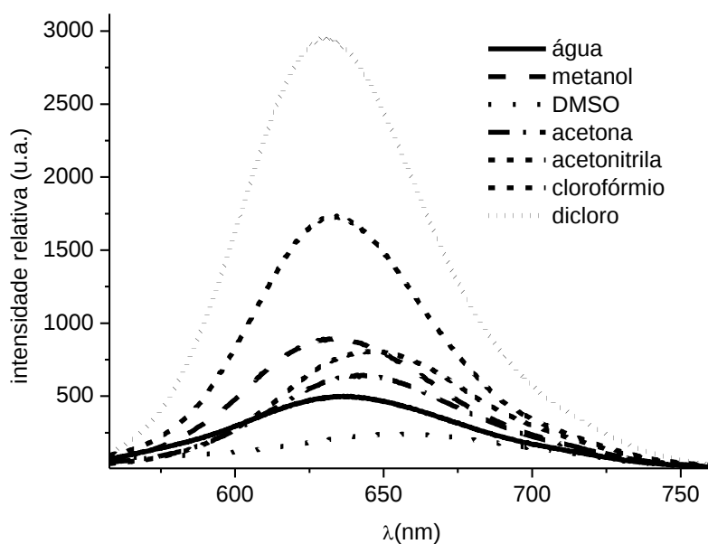
FIGURA 14. Emissão do complexo cis - [\text{Ru}(\text{phen})_2(\text{him})_2](\text{PF}_6)_2 em vários solventes na concentração de 5 \times 10^{-5} \text{ mol} \cdot \text{L}^{-1} com \lambda_{\text{exc}} = 480\text{nm} .
