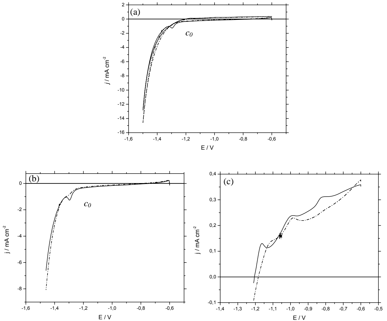
FIGURA 6.6: Curvas voltamétricas obtidas de uma solução de NaOH 2,0 mol L -1 , na ausência (—) ou presença (---) de manitol 0,20 mol L -1 , sobre eletrodo de aço 1010, em 10,0 mV s -1 . (a) varredura catódica e anódica, (b) varredura catódica e (c) varredura anódica.
