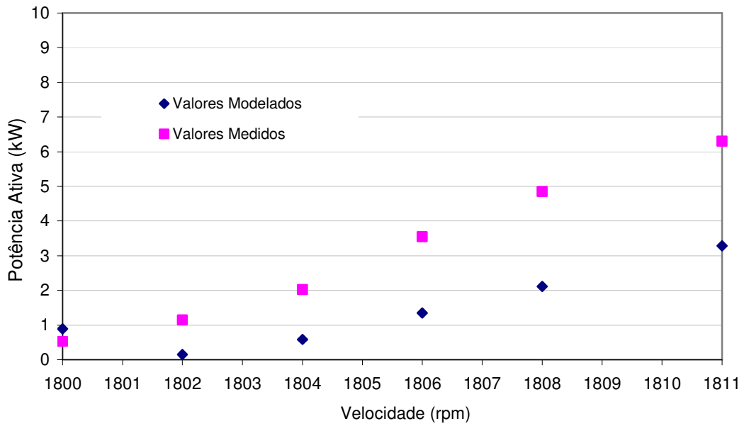
Figura 72 – Comparação entre valores modelados e experimentais da potência ativa do gerador de indução interligado à rede de distribuição com banco de capacitores de 60µF.
