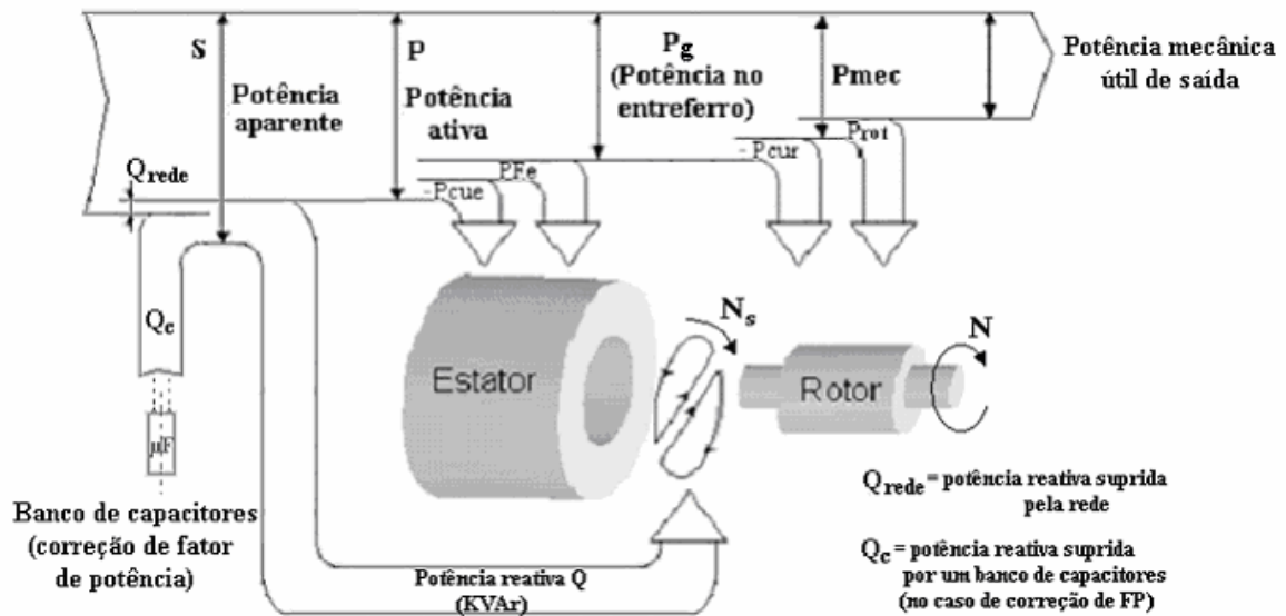
Figura 9 – Fluxo de potência no motor de indução (CHAPALLAZ, 1992).
