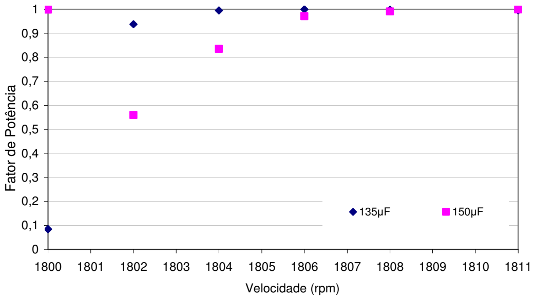
Figura 52 – Fator de potência dos valores medidos para banco de capacitores com capacitâncias de 135µF e 150µF ligados em paralelo ao gerador de indução.
