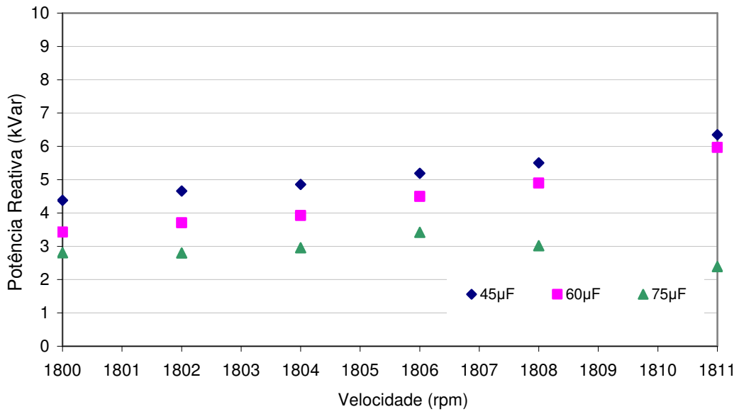
Figura 58 – Potência reativa trifásica dos valores medidos para banco de capacitores com capacitâncias de 45 μF, 60 μF e 75 μF ligados em paralelo ao gerador de indução.
