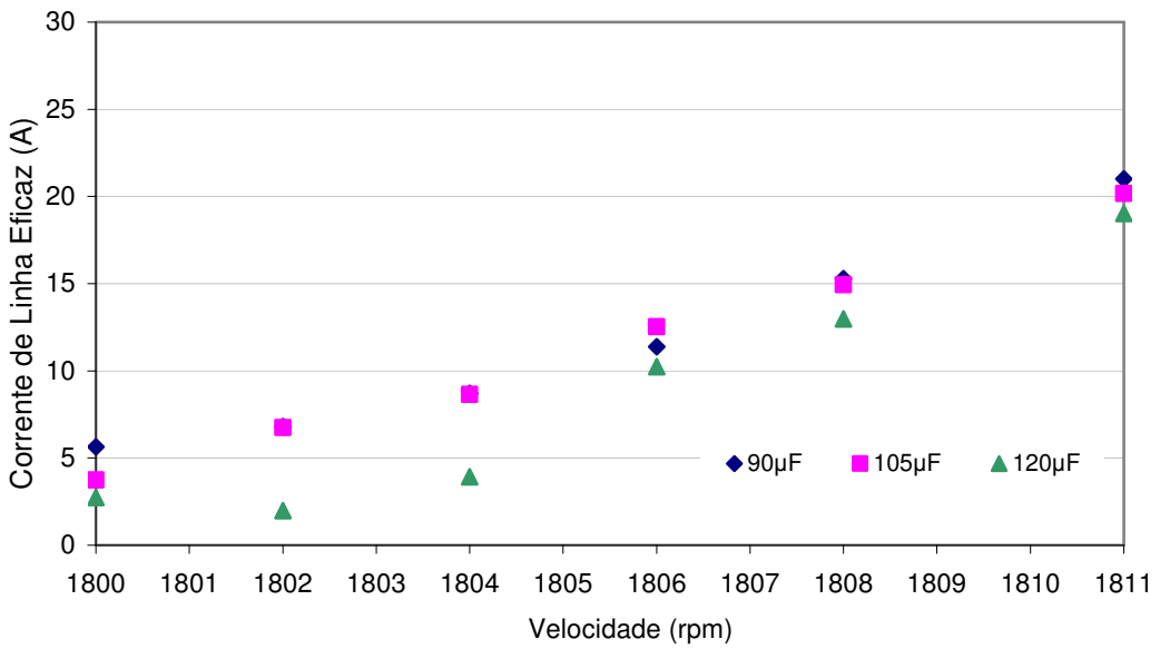
Figura 46 – Valores de corrente de linha medidos para banco de capacitores com capacitâncias de 90µF, 105µF e 120µF ligados em paralelo ao gerador de indução.
