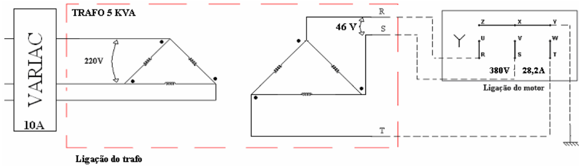
Figura 22 – Topologia para ensaio a rotor bloqueado.
