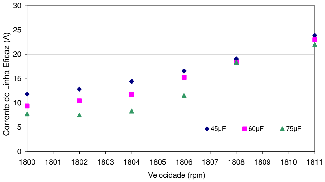
Figura 45 – Valores de corrente de linha medidos para banco de capacitores com capacitâncias de 45µF, 60µF e 75µF ligados em paralelo ao gerador de indução.
