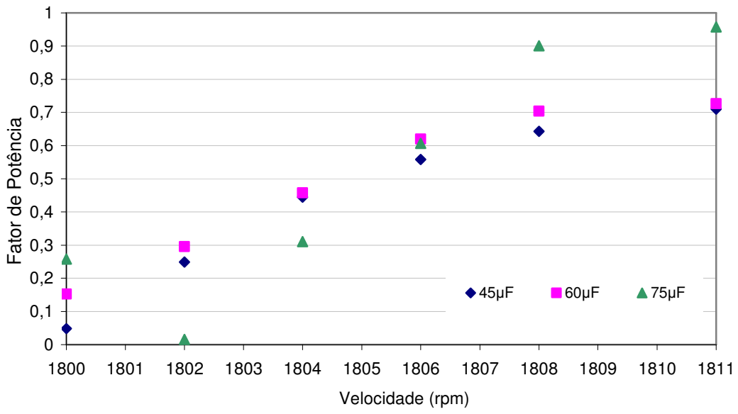
Figura 50 – Fator de potência dos valores medidos para banco de capacitores com capacitâncias de 45µF, 60µF e 75µF ligados em paralelo ao gerador de indução.
