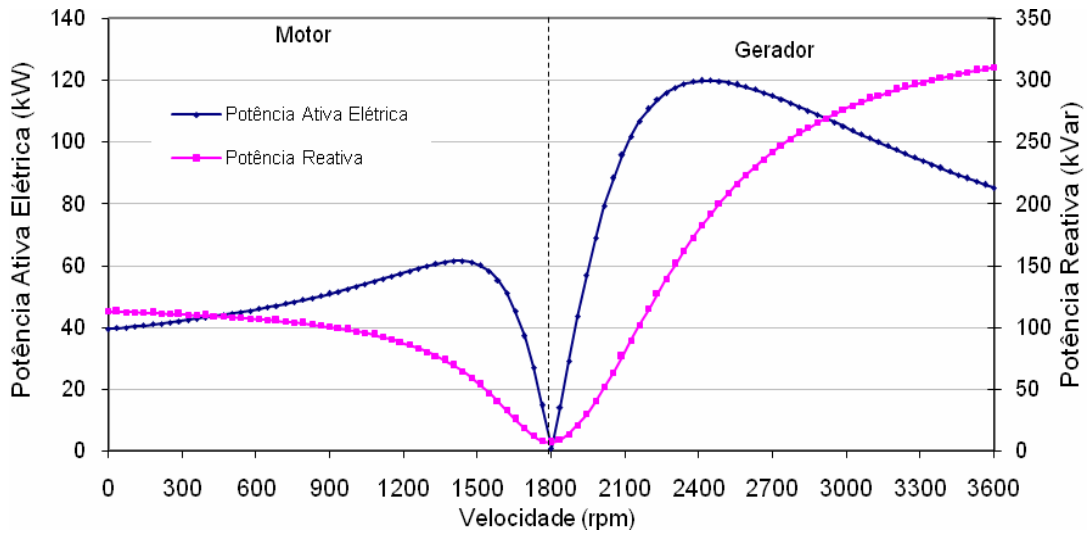
Figura 29 – Resultados teóricos para o gerador de indução – Potência ativa elétrica e potência reativa para escorregamento no intervalo [1,-1].
