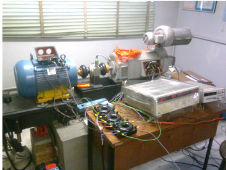
Figura 20 – Bancada de ensaios do gerador de indução.
