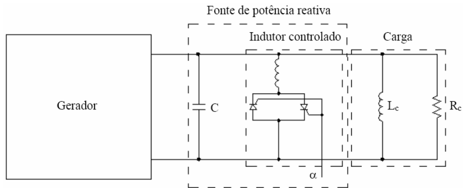
Figura 83 – Método do indutor controlado (CHAPALLAZ, 1992).
