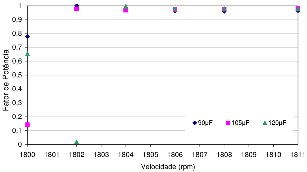
Figura 51 – Fator de potência dos valores medidos para banco de capacitores com capacitâncias de 90µF, 105µF e 120µF ligados em paralelo ao gerador de indução.
