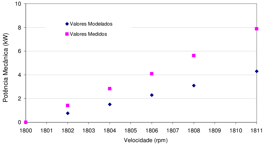
Figura 62 – Comparação entre valores modelados e experimentais da potência mecânica para o gerador de indução interligado à rede de distribuição.
