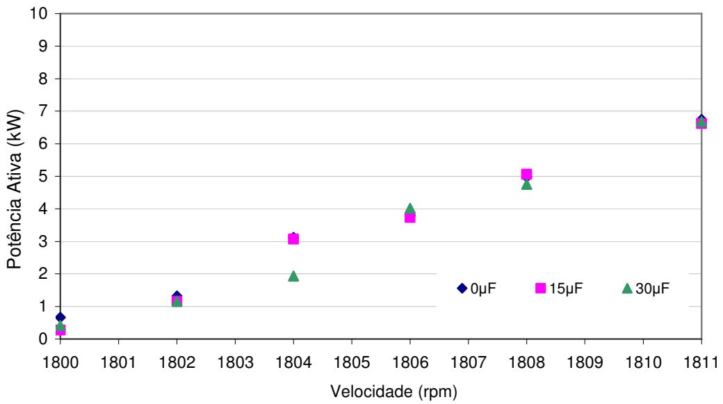
Figura 53 – Potência ativa trifásica dos valores medidos para banco de capacitores com capacitâncias de 0µF, 15µF e 30µF ligados em paralelo ao gerador de indução.
