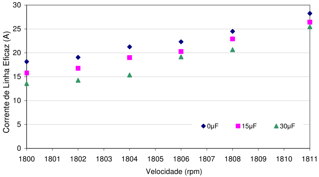
Figura 44 – Valores de corrente de linha medidos para banco de capacitores com capacitâncias de 0 \mu F, 15 \mu F e 30 \mu F ligados em paralelo ao gerador de indução.
