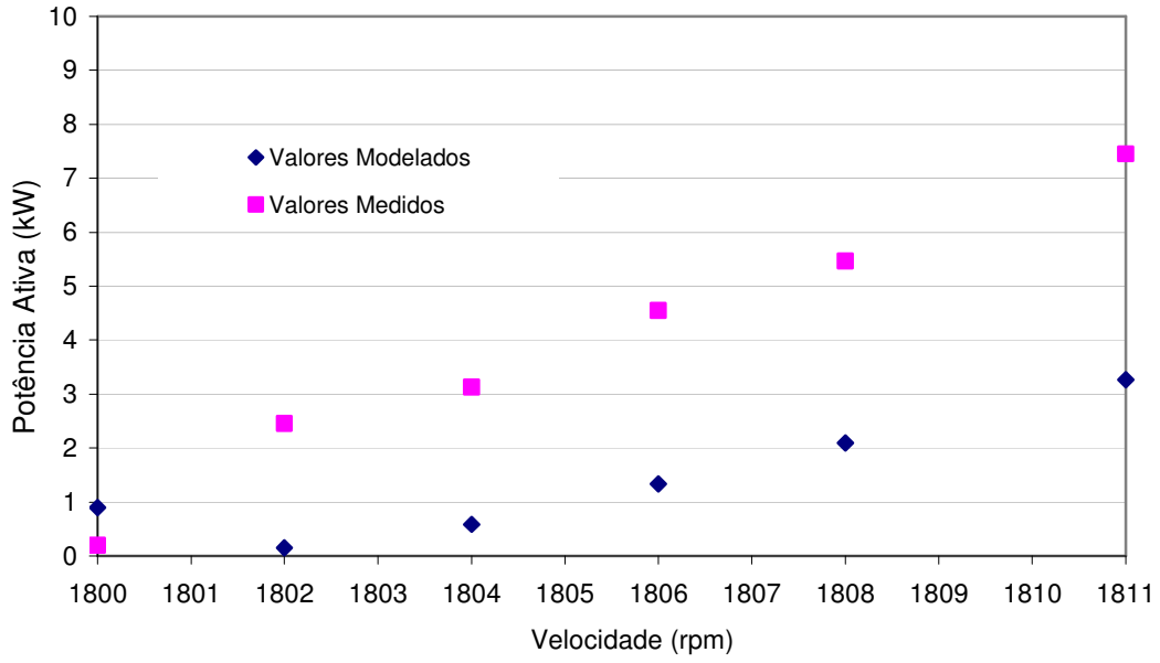
Figura 73 – Comparação entre valores modelados e experimentais da potência ativa do gerador de indução interligado à rede de distribuição com banco de capacitores de 105µF.
