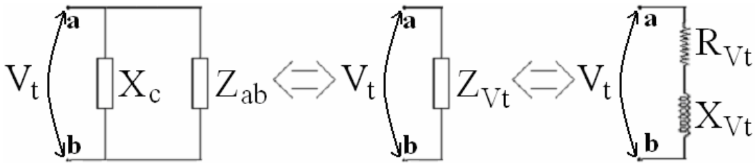
Figura 18 – Reatância capacitiva X_c em paralelo a impedância Z_{ab} .
