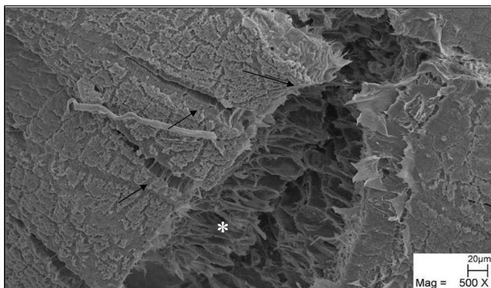
FIGURA 13. Eletromicrografia de varredura da testa de sementes de garapa apresentando rachadura na testa (→), atingindo a camada de macroesclereídes em paliçada (*), ocasionada pelo ácido sulfúrico 98% por 3 minutos. UFV, Viçosa, MG, 2009.
