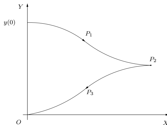
Figura 29: Possível trajetória para um robô móvel atingir a origem com condições iniciais do tipo [0 \ y(0) \ 0]^T .
