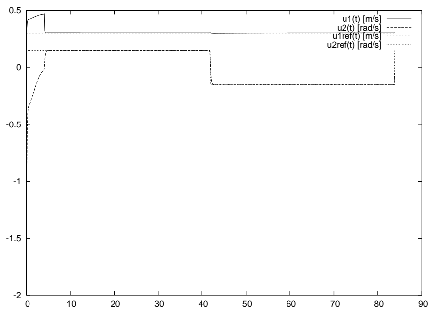
Figura 20: Sinal de controle para rastreamento de uma trajetória em “oito” com NMPC com função custo de (KÜHNE, 2005).
