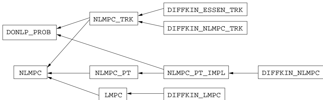
Figura 40: Diagrama de classes dos controladores implementados.
