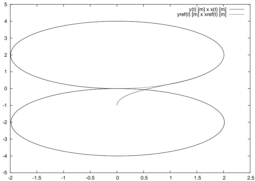
Figura 23: Trajetórias real e de referência para NMPC com função-custo de (ESSEN; NIJMEIJER, 2001) seguindo uma trajetória em “oito”.
