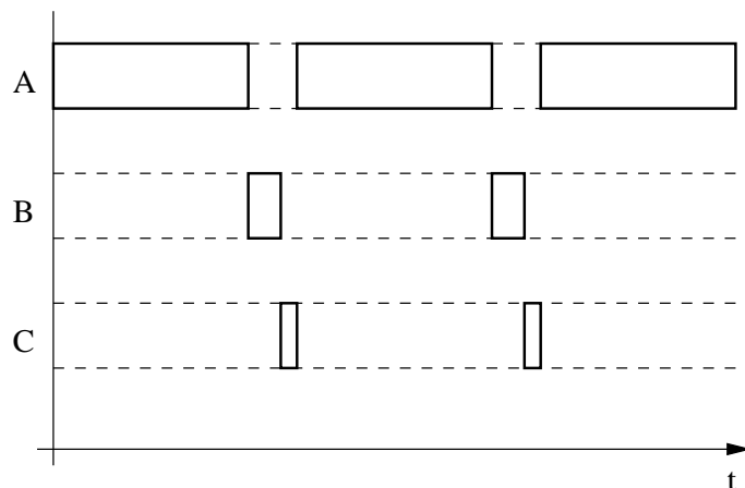
Figura 11: Escalonamento de tarefas com tempos de execução ilimitados em sistemas operacionais não de tempo real. Tarefa A: maior prioridade. Tarefa C: menor prioridade.
