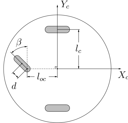
Figura 6: Parâmetros do robô móvel.
