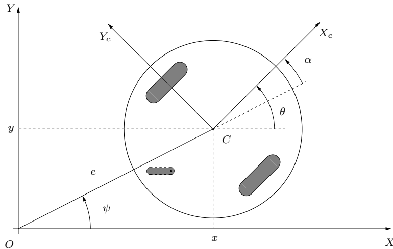
Figura 7: Relação entre coordenadas polares e cartesianas para um robô móvel com acionamento diferencial.
