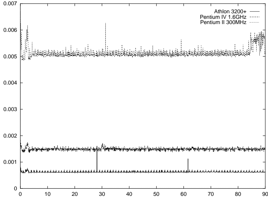
Figura 18: Tempo de computação do sinal de controle para o LMPC.
