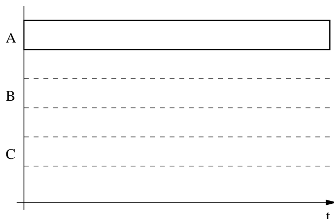
Figura 12: Escalonamento de tarefas com tempo de execução ilimitado em sistemas operacionais de tempo real. Tarefa A: maior prioridade. Tarefa C: menor prioridade.
