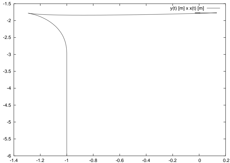
Figura 26: Trajetória do robô móvel no plano XY para NMPC com coordenadas cartesianas e \mathbf{x}(0) = [-1 \quad -6 \quad \pi/2] .
