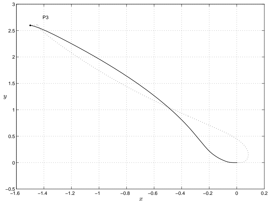
Figura 32: Comparação entre NMPC em coordenadas polares de (KÜHNE, 2005) (linha tracejada) e NMPC em coordenadas polares alteradas (linha contínua).
