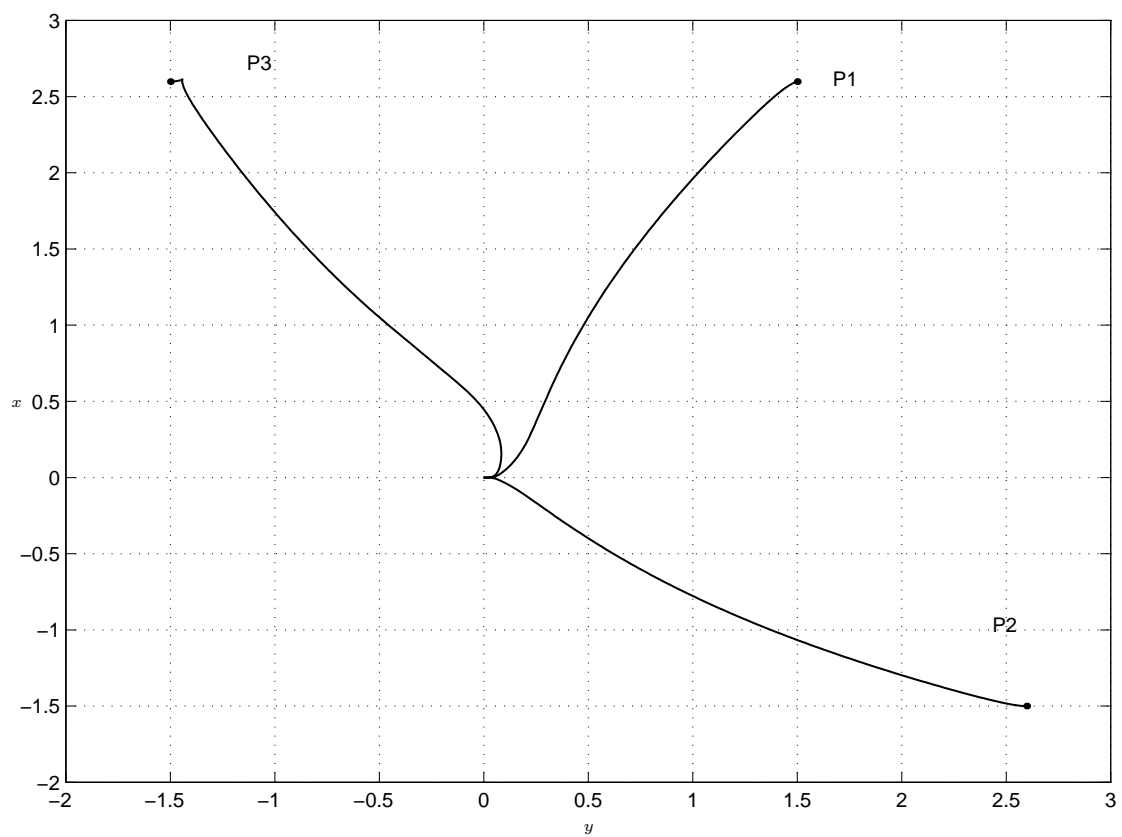
Figura 30: Trajetórias para diferentes condições iniciais, NMPC em coordenadas polares de (KÜHNE, 2005).
