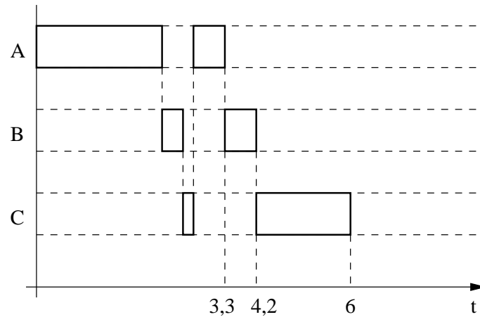
Figura 13: Escalonamento de tarefas com tempos de execução limitados em sistemas operacionais não de tempo real. Tarefa A: maior prioridade. Tarefa C: menor prioridade.
