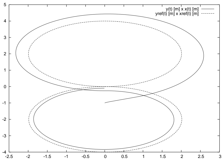
Figura 22: Trajetórias real e de referência para NMPC com função custo de (KÜHNE, 2005) seguindo uma trajetória em “oito” para \mathbf{Q} = \text{diag}(1, 1, 0, 5) .
