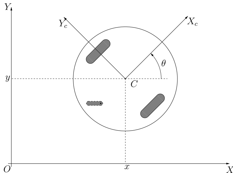
Figura 3: Sistema de coordenadas do robô móvel.
