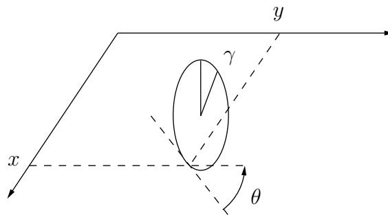
Figura 2: Moeda rolando sobre um plano horizontal.
