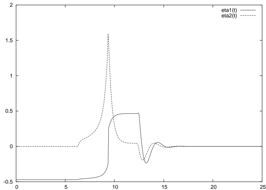
Figura 27: Sinal de controle para NMPC com coordenadas cartesianas e \mathbf{x}(0) = [-1 \ -6 \ \pi/2] .
