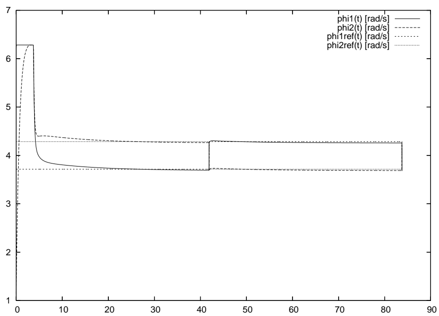
Figura 17: Velocidades das rodas para LMPC seguindo uma trajetória em “oito”.
