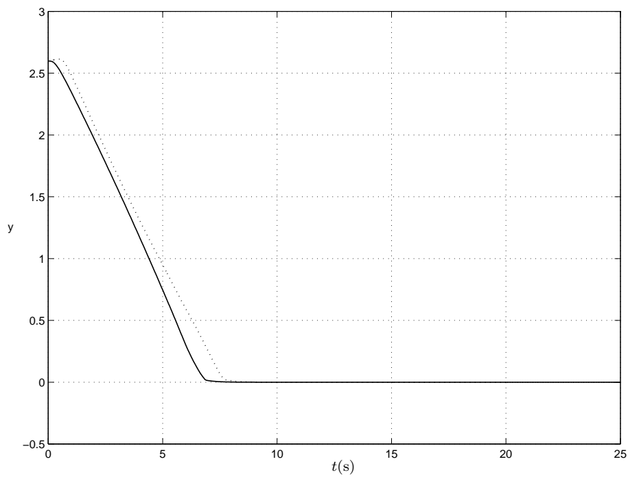
Figura 35: y em função do tempo. Linha tracejada: NMPC em coordenadas polares de (KÜHNE, 2005). Linha contínua: NMPC em coordenadas polares alteradas.
