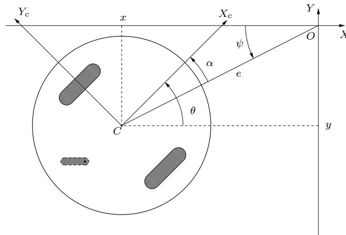
Figura 31: Conjunto de coordenadas alternativo para um robô móvel com acionamento diferencial.
