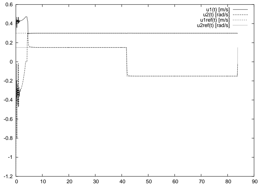
Figura 24: Sinal de controle para rastreamento de uma trajetória em “oito” com NMPC com função custo de (ESSEN; NIJMEIJER, 2001).
