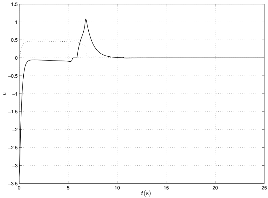
Figura 38: Entradas do sistema para NMPC em coordenadas polares alteradas. Linha contínua: v(t) . Linha tracejada: w(t) .
