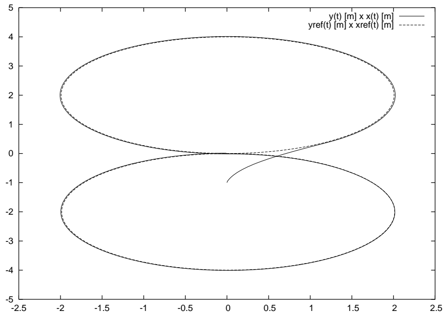
Figura 19: Trajetórias real e de referência para NMPC com função custo de (KÜHNE, 2005) seguindo uma trajetória em “oito”.
