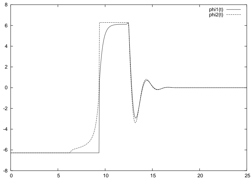
Figura 28: Velocidades das rodas para NMPC com coordenadas cartesianas e \mathbf{x}(0) = [-1 \ -6 \ \pi/2]^T .
