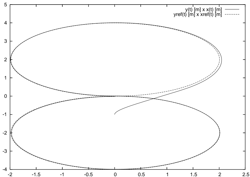
Figura 15: Trajetórias real e de referência para LMPC seguindo uma trajetória em “oito”.
