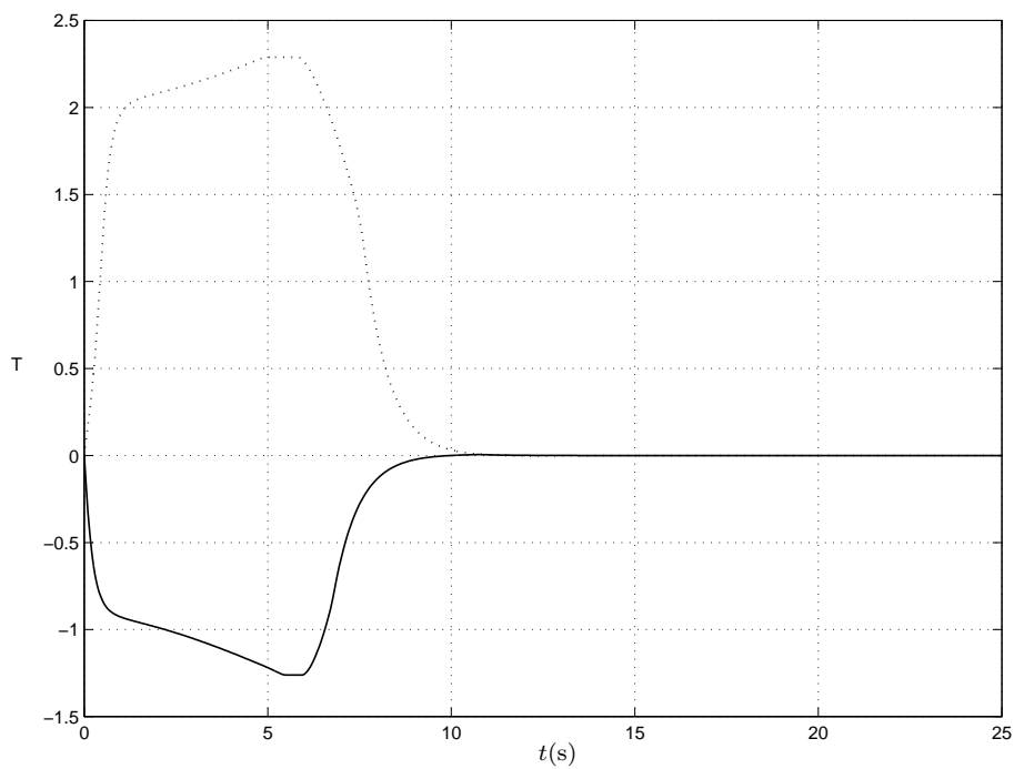
Figura 36: \theta em função do tempo. Linha tracejada: NMPC em coordenadas polares de (KÜHNE, 2005). Linha contínua: NMPC em coordenadas polares alteradas.
