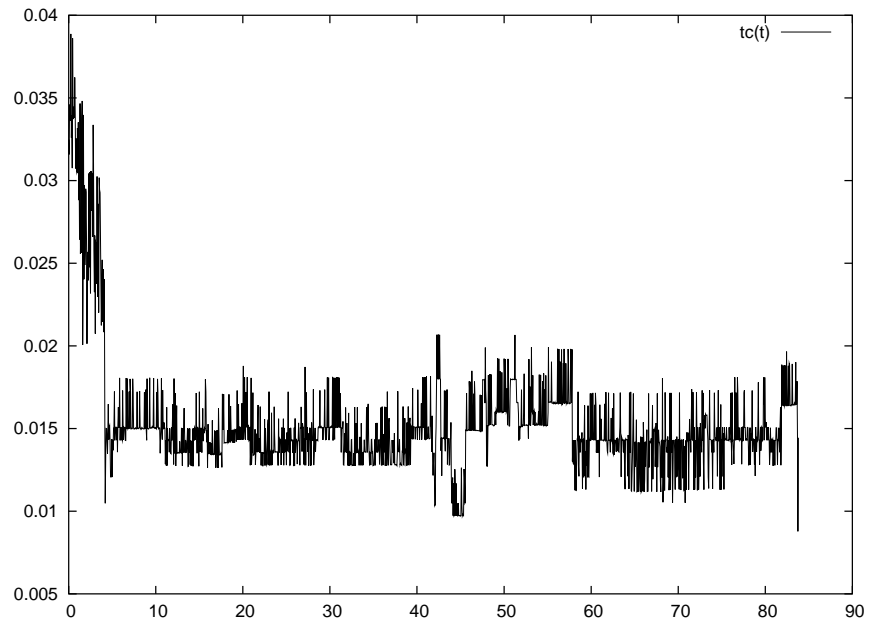
Figura 21: Tempo de computação do sinal de controle para rastreamento de uma trajetória em “oito” com NMPC com função custo de (KÜHNE, 2005).
