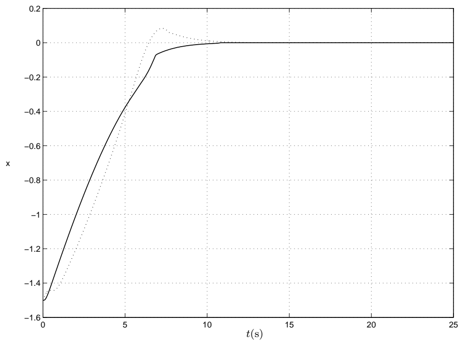
Figura 34: x em função do tempo. Linha tracejada: NMPC em coordenadas polares de (KÜHNE, 2005). Linha contínua: NMPC em coordenadas polares alteradas.
