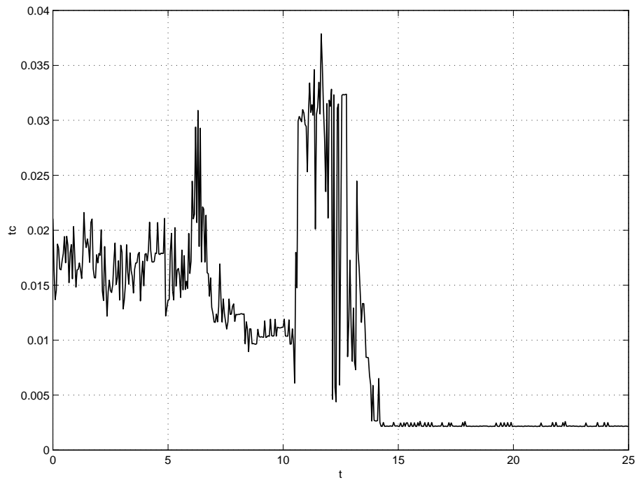
Figura 39: Tempo de computação do sinal de controle para NMPC em coordenadas polares alteradas.
