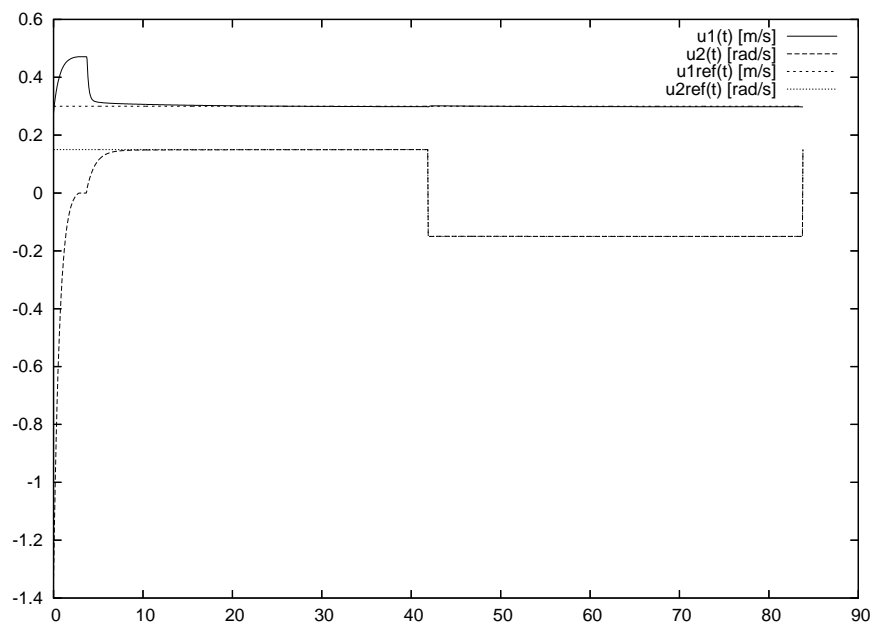
Figura 16: Entradas de controle para LMPC seguindo uma trajetória em “oito”.
