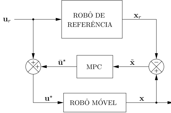
Figura 9: Diagrama de blocos do LMPC.
