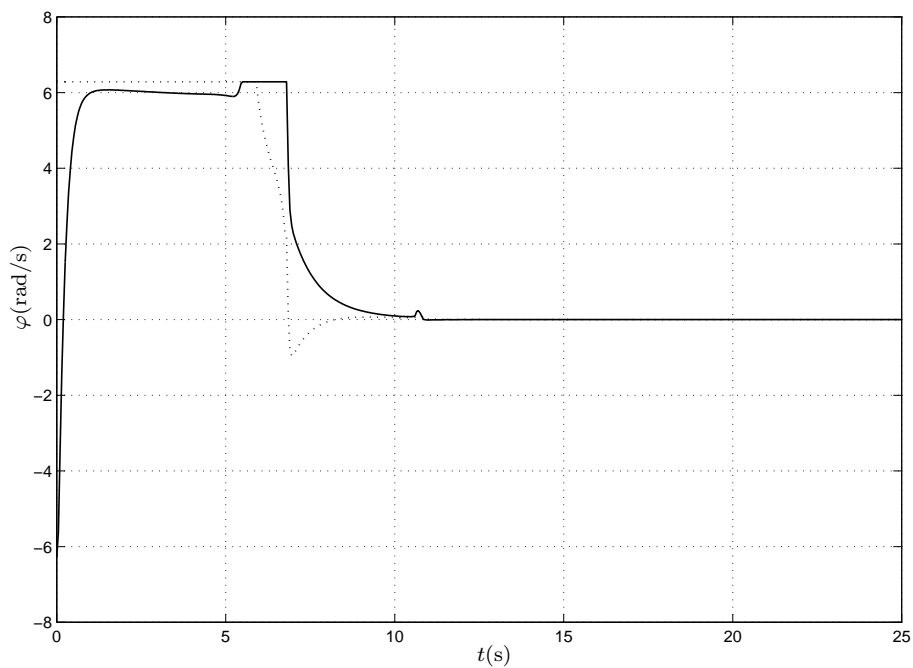
Figura 37: Velocidades das rodas para NMPC em coordenadas polares alteradas. Linha contínua: \varphi_r(t) . Linha tracejada: \varphi_l(t) .
