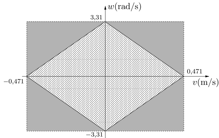
Figura 10: Restrições nas rodas: regiões que satisfazem as restrições nas entradas considerando-se limitações em \dot{\varphi}_{min} e \dot{\varphi}_{max} (região hachurada) e limitações em v_{max} e w_{max} (região em cinza).
