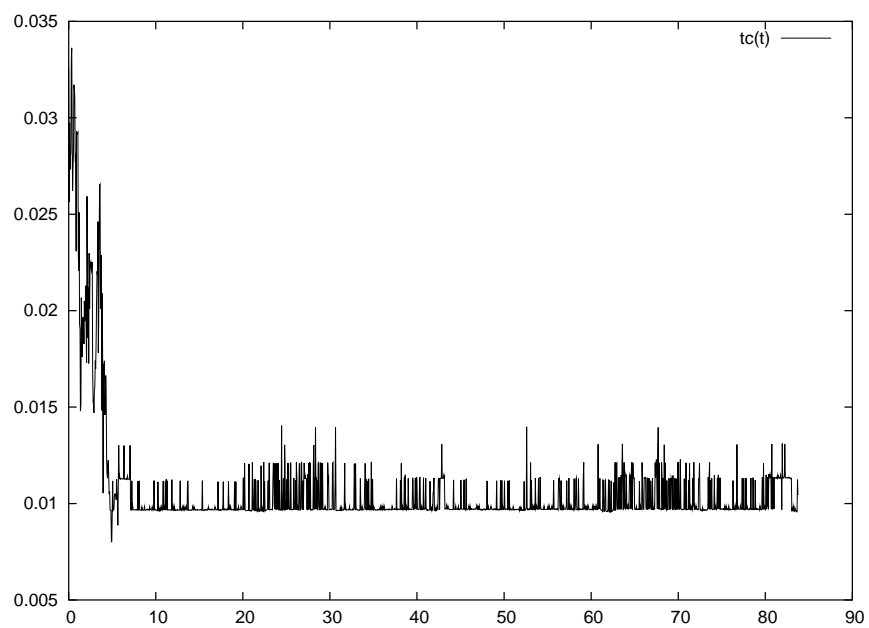
Figura 25: Tempo de computação do sinal de controle para rastreamento de uma trajetória em “oito” com NMPC com função custo de (ESSEN; NIJMEIJER, 2001).
