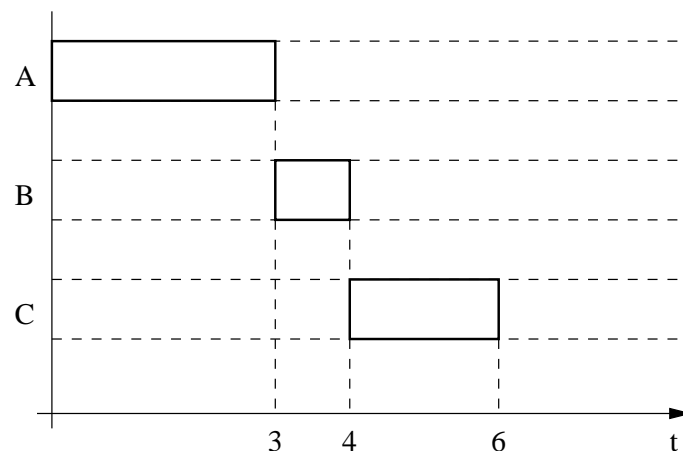
Figura 14: Escalonamento de tarefas com tempo de execução limitado em sistemas operacionais de tempo real. Tarefa A: maior prioridade. Tarefa C: menor prioridade.
