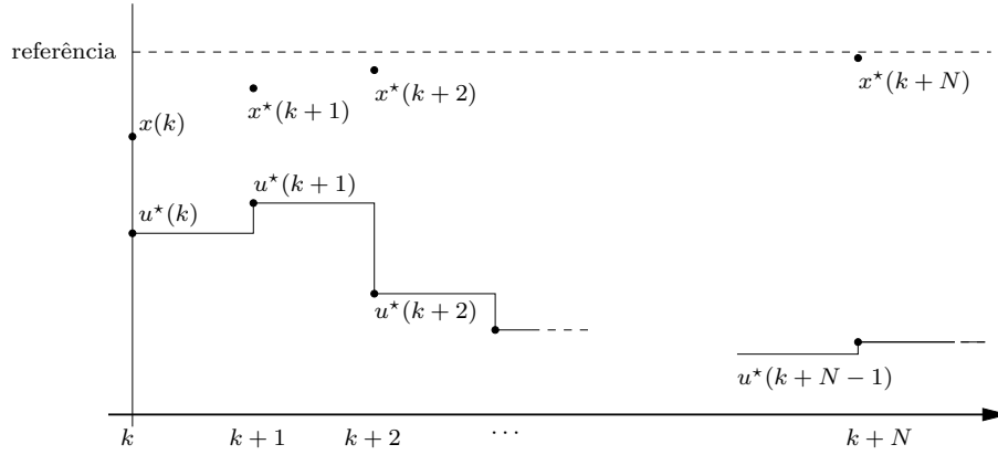
Figura 8: Esquema do MPC.
