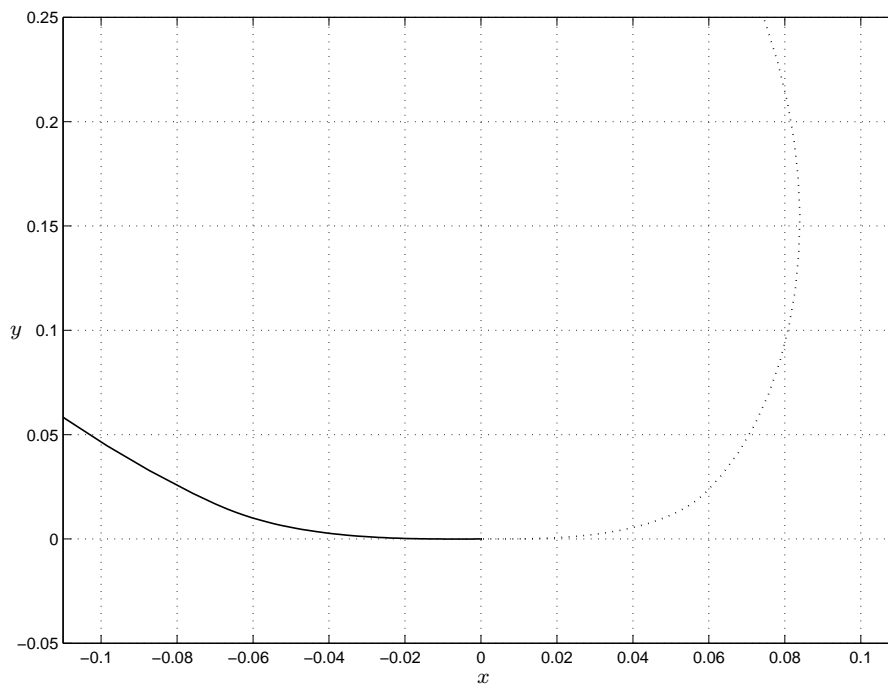
Figura 33: Detalhe da Figura 32 em torno da origem. Linha tracejada: NMPC em coordenadas polares de (KÜHNE, 2005). Linha contínua: NMPC em coordenadas polares alteradas.
