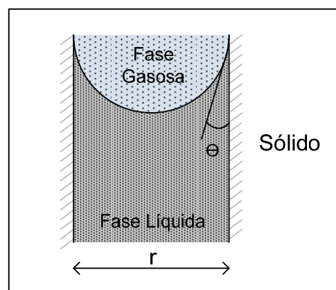
Figura 9: representação esquemática de um capilar não saturado (adaptado de HUA; ACKER; EHRLACHER, 1995)
