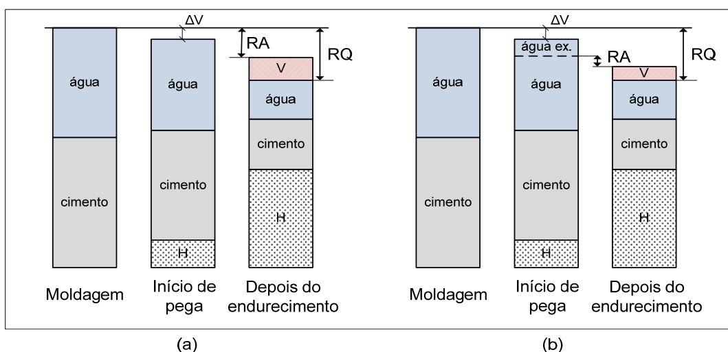
Figura 4: representação esquemática da relação entre a retração química e a retração autógena. (a) sem exsudação. (b) com exsudação (adaptado de Tazawa 6 , 1998 apud Lam, 2005)
