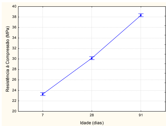
Figura 47: efeito isolado da idade na resistência à compressão uniaxial do concreto
