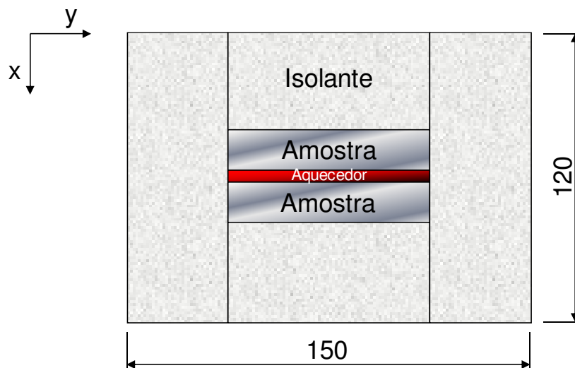
Figura 4.14 – Esquema da montagem (corte vista lateral esquerda).
