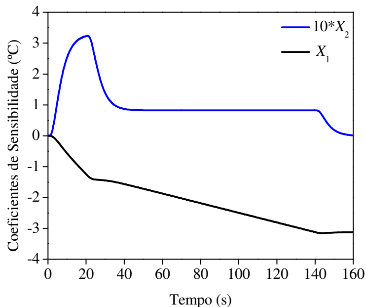
Figura 5.1 – Coeficientes de Sensibilidade do Aço Inox AISI 304.
