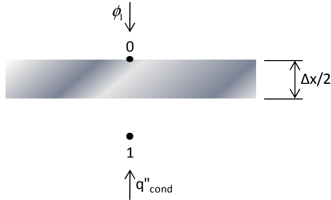
Figura 3.3 – Nó 0 (zero) na superfície onde o fluxo de calor é imposto e nó adjacente 1.
