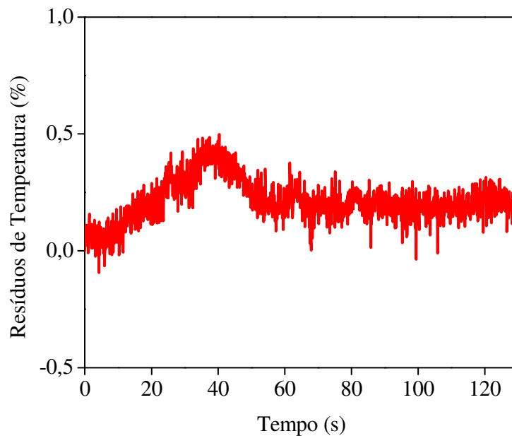
Figura 5.12 – Resíduos de Temperatura para o Aço Inox AISI 316.
