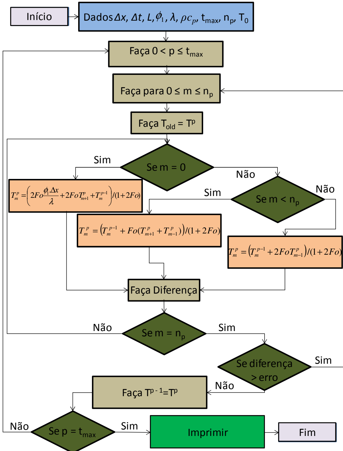
Figura 3.6 – Algoritmo utilizado para calcular a distribuição de temperatura na amostra.
