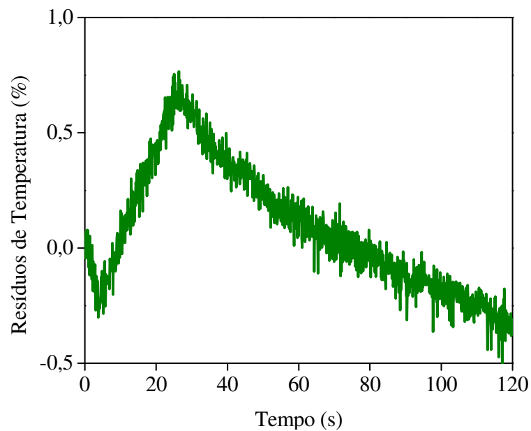
Figura 5.17 – Resíduos de Temperatura para o Titânio.
