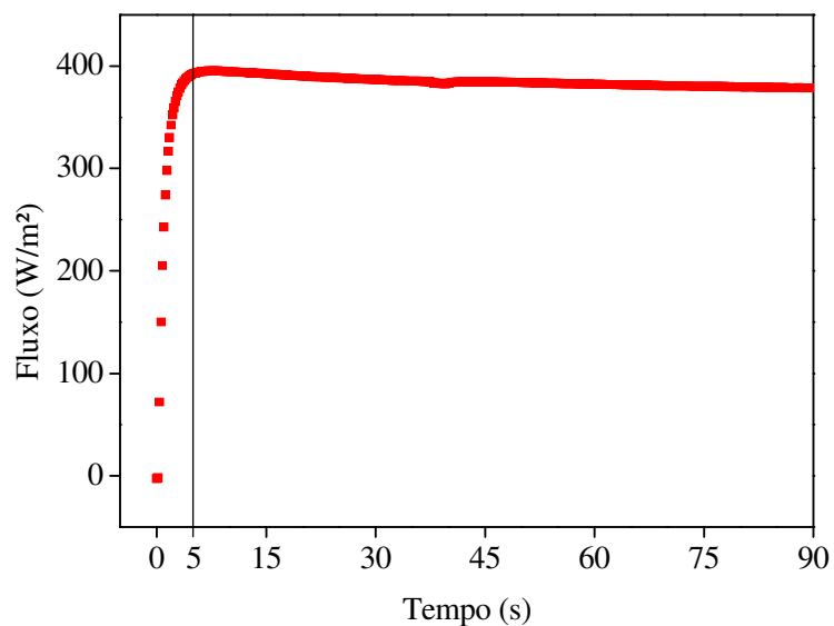
Figura B.2 – Fluxo de calor de 380 \text{ W/m}^2 .
