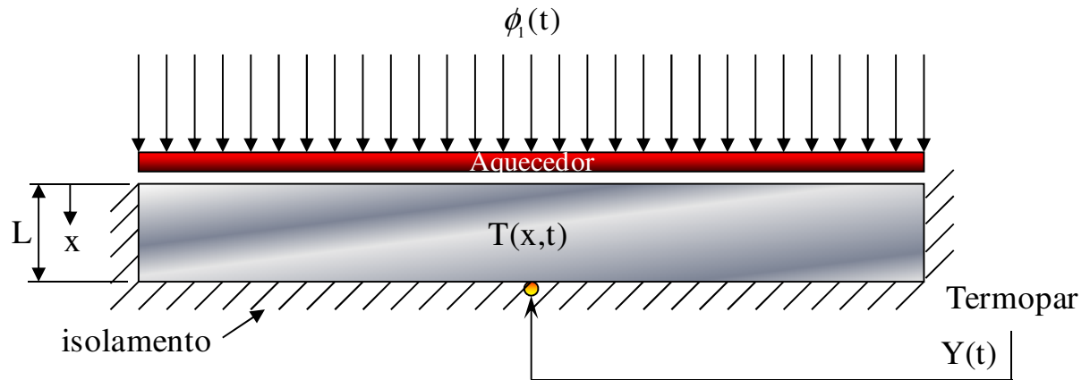
Figura 3.1 – Modelo térmico unidimensional.
