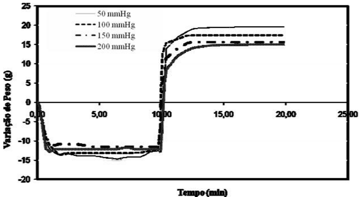
Figura 15 – Cinética da impregnação a vácuo de maçã ( var. fuji ) nas pressões de vácuo de 50 mmHg, 100 mmHg, 150 mmHg e 200 mmHg.
