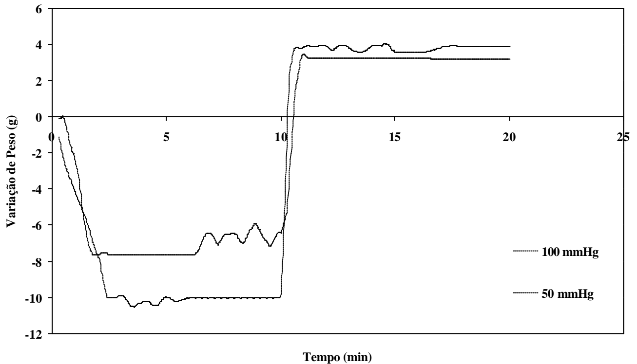
Figura 19 - Cinética da impregnação a vácuo de pêra ( var. d'anjou ) nas pressões de vácuo de 50 mmHg e 100 mmHg.
