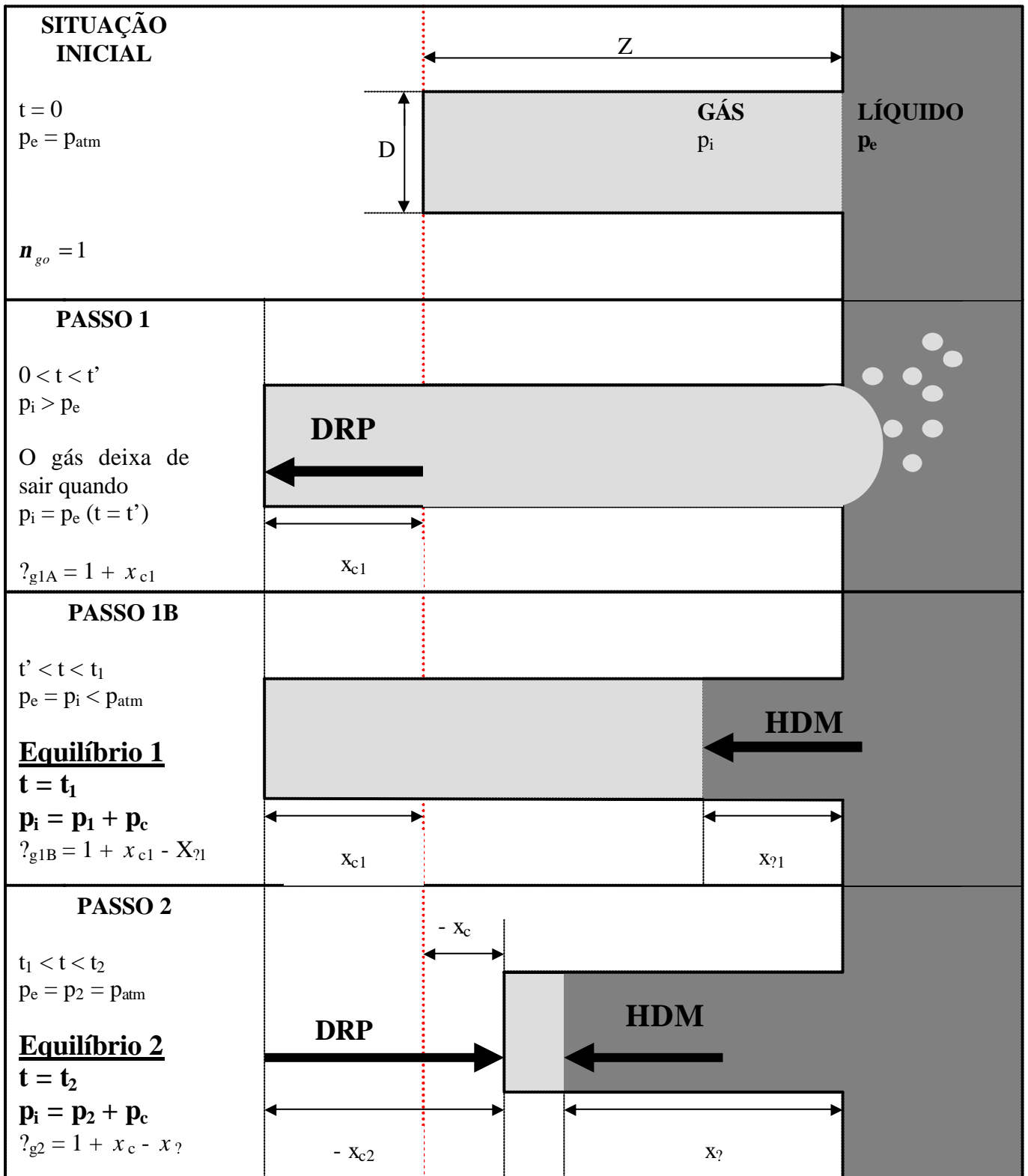
Figura 7 – Sistema sólido-líquido, HDM acoplado ao fenômeno de deformação-relaxação em um poro ideal. (FITO et al, 1996).
