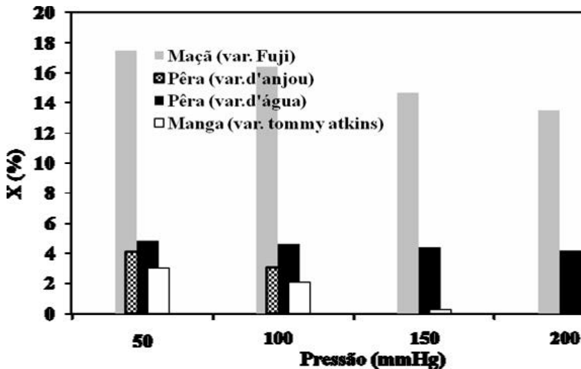
Figura 23 – Influência da pressão de vácuo na fração da amostra impregnada X(%).
