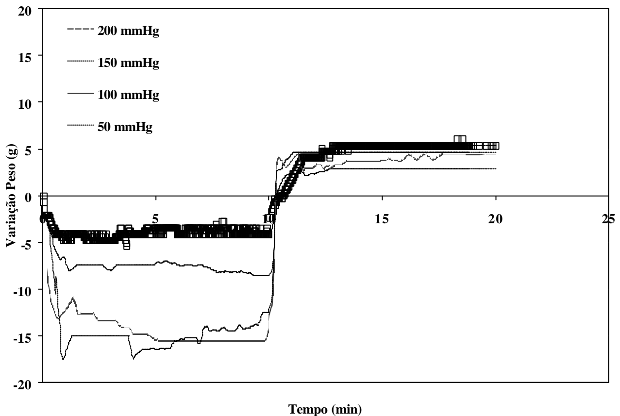
Figura 21 - Cinética da impregnação a vácuo de manga ( var. tommy atkins ) nas pressões de vácuo de 50 mmHg, 100 mmHg, 150 mmHg e 200 mmHg.
