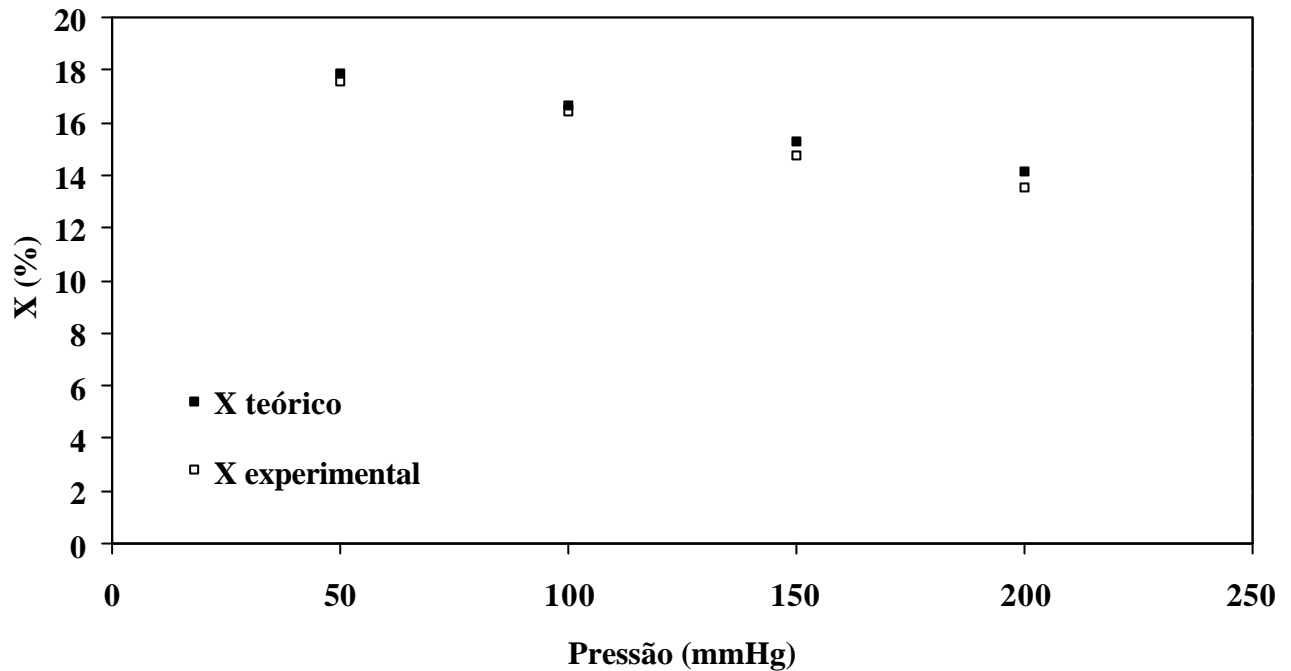
Figura 16 – Fração da amostra de maçã ( var. fuji ) impregnada pela solução em diferentes pressões de vácuo.
