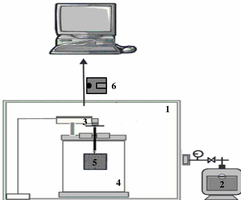
Figura 8 – Representação esquemática do dispositivo experimental para os ensaios de impregnação a vácuo.
