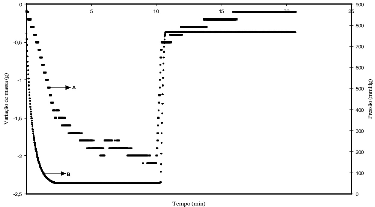
Figura 12 – A: Curva padrão para suco de maçã desaerado com 12,6°BRIX a pressão de 50 mmHg. B: Curva de pressão.
