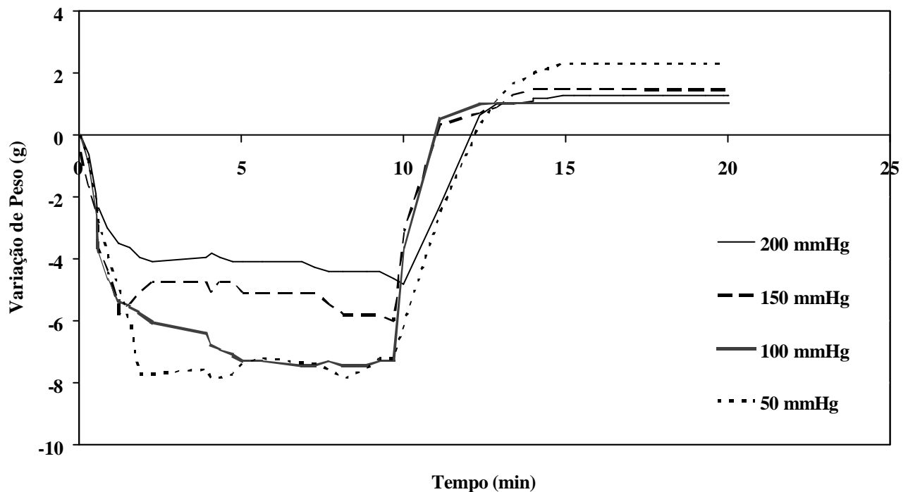
Figura 17 - Cinética da impregnação a vácuo de pêra ( var. d'água ) nas pressões de vácuo de 50 mmHg, 100 mmHg, 150 mmHg e 200 mmHg.
