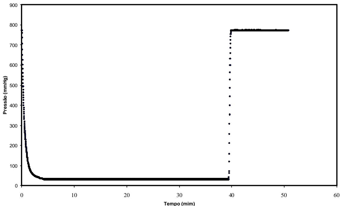
Figura 10 – Curva de pressão obtida para câmara de vácuo com 50 L de volume interno.
