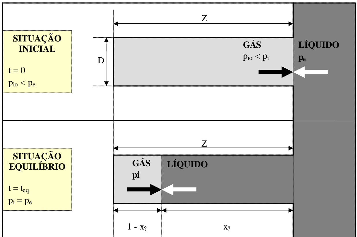
Figura 6 - Mecanismo Hidrodinâmico em um poro ideal (FITO, 1994).
