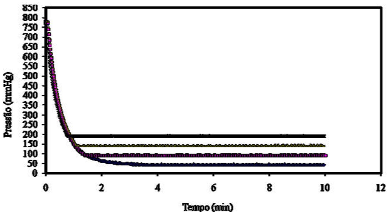
Figura 11 – Curvas de vácuo mantendo-se constante as pressões de 50, 100, 150 e 200 mmHg.
