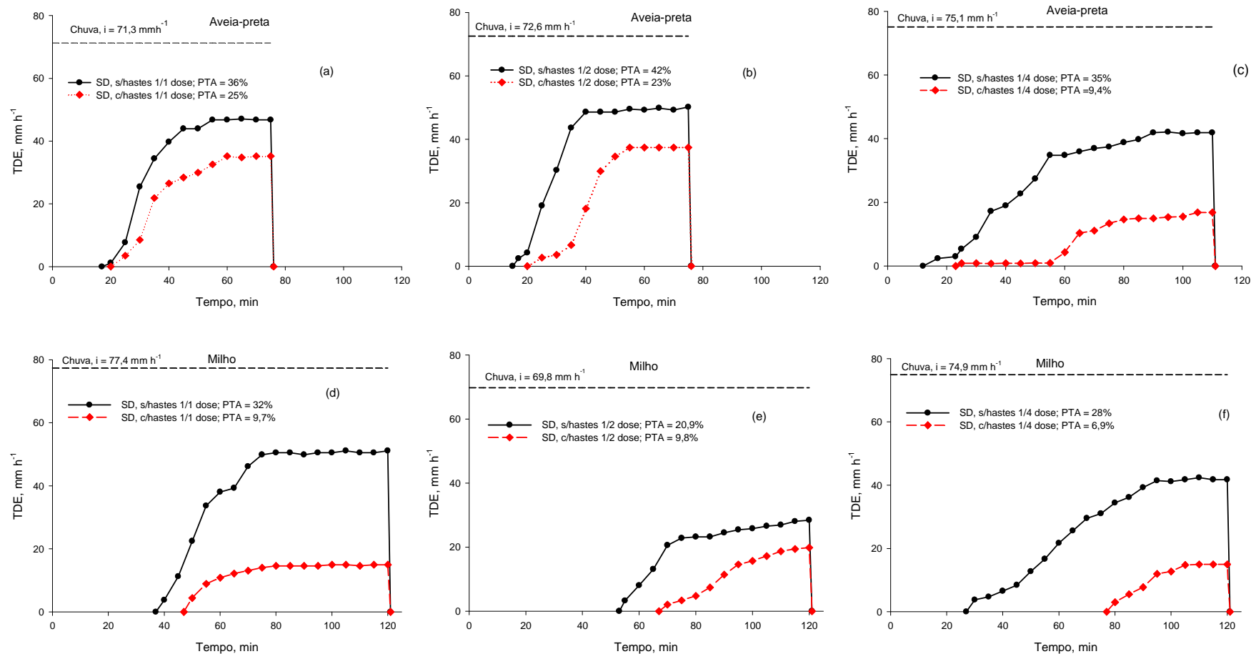
FIGURA 7. Distribuição temporal das taxas de descarga enxurrada (TDE) e correspondentes perdas totais de água (PTA) em relação às quantidades totais de chuva aplicadas, sob as intensidades e durações reais das chuvas simuladas, com os resíduos culturais de aveia preta e de milho, nos tratamentos estudados.
