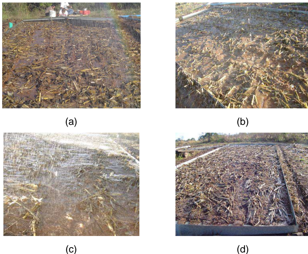
FIGURA 20. Vista da superfície do solo na parcela experimental do tratamento semeadura direta sem hastes sulcadoras e metade da dose integral do resíduo cultural de milho (SD s/hastes, 1/2 dose ou 4,0 \text{ Mg ha}^{-1} ), em diferentes momentos do correspondente teste de erosão: (a) durante a aplicação somente da chuva simulada, (b) durante a adição do terceiro nível de fluxo extra, evidenciando a movimentação inicial do resíduo cultural, no modo de peça por peça, (c) durante a adição do quarto nível de fluxo extra, evidenciando a remoção efetiva do resíduo cultural, predominantemente no modo em massa, mas com alguma remoção no modo de peça por peça, e (d) após o término da chuva simulada e da adição do último nível de fluxo extra, evidenciando de modo mais claro a remoção do resíduo cultural.
