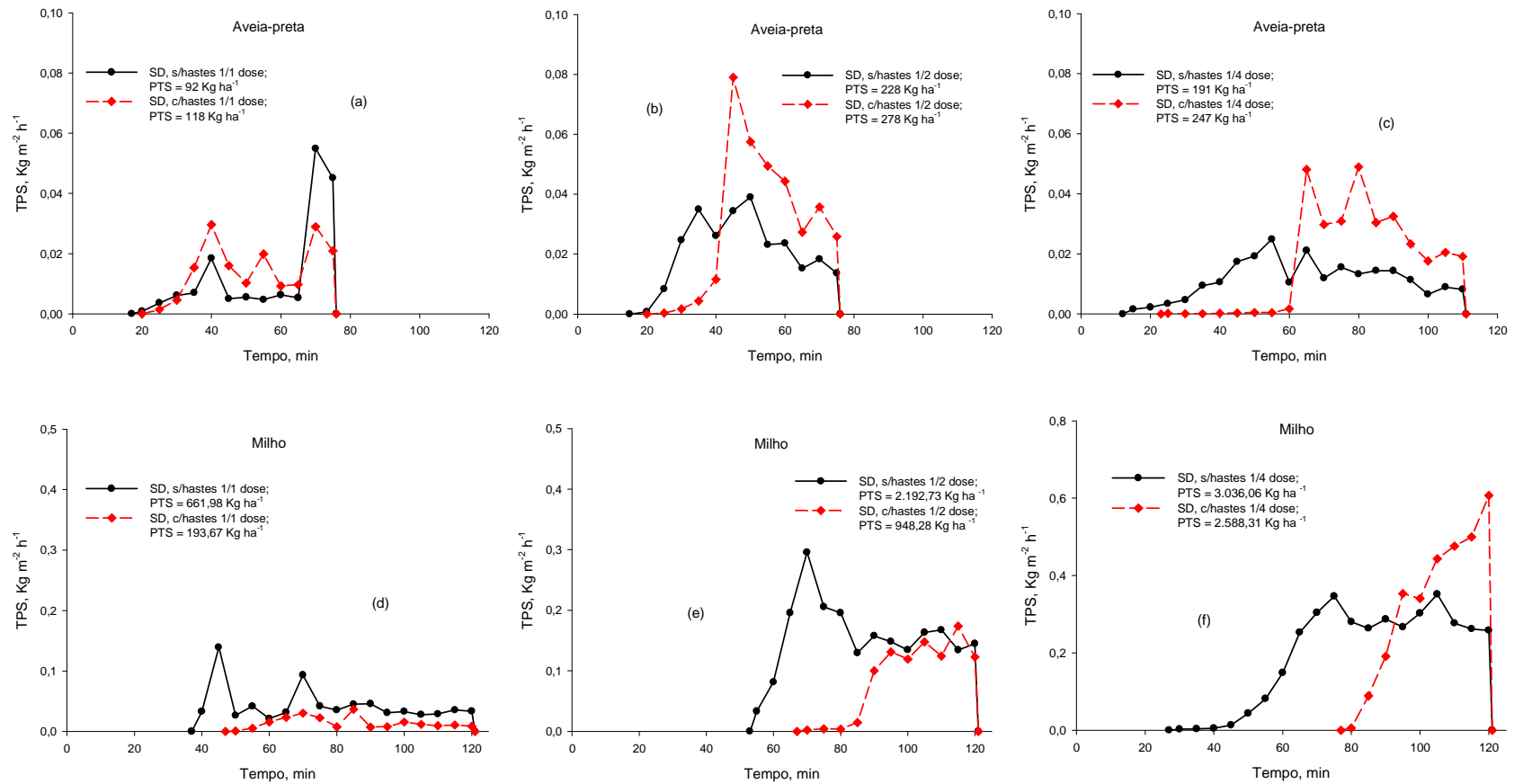
FIGURA 9. Distribuição temporal das taxas de perda de solo (TPS) e correspondentes perdas totais da mesma (PTS), sob as intensidades e durações observadas das chuvas aplicadas, nas condições com o resíduo cultural de aveia-preta e de milho, nos tratamentos estudados.
