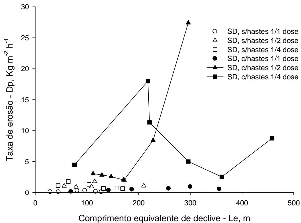
FIGURA 18. Taxas de erosão ou perda de solo ( D_p ) em função dos comprimentos equivalentes de declive simulados na pesquisa ( L_e ), nos tratamentos estudados.
