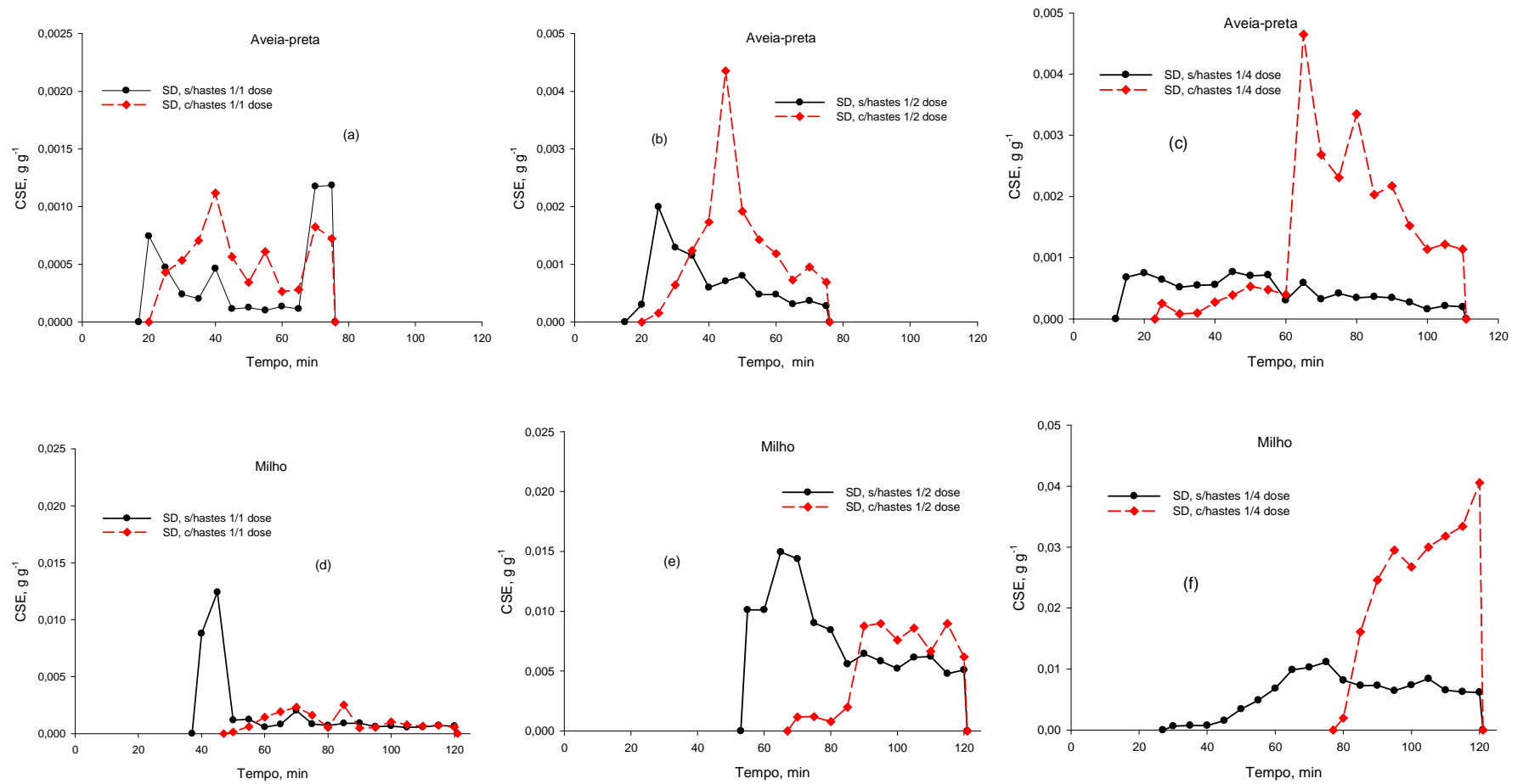
FIGURA 8. Distribuição temporal das concentrações de sedimento na enxurrada (CSE), sob as intensidades e durações reais das chuvas simuladas, com os resíduos culturais de aveia preta e de milho, nos tratamentos estudados.
