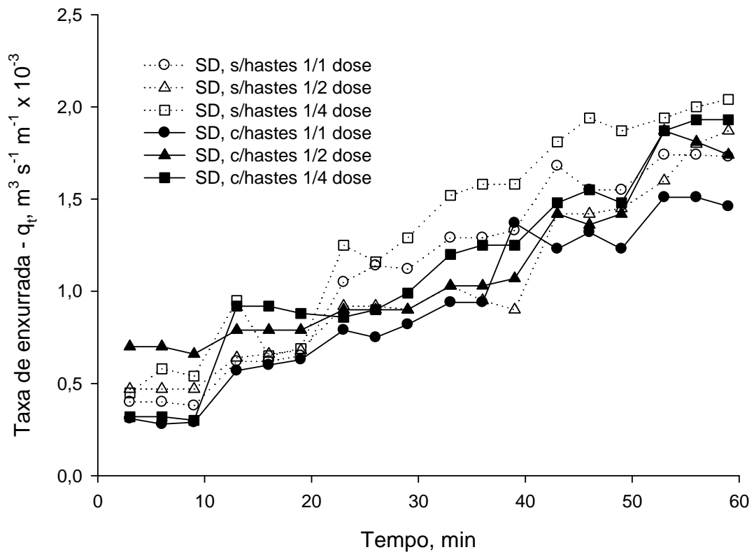
FIGURA 14. Distribuição temporal das taxas de descarga da enxurrada ( q_t ) a partir da adição dos níveis de fluxo extra de água nas parcelas experimentais, sobre o resíduo cultural de milho, nos tratamentos estudados.
