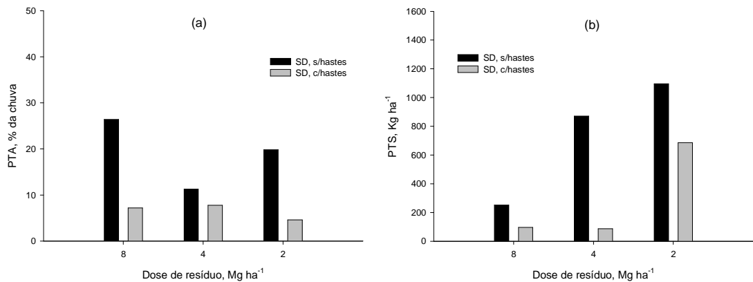
FIGURA 11. Perda total de água (PTA - a) e perda total de solo (PTS - b) na condição com o resíduo cultural de milho, nos tratamentos estudados.
