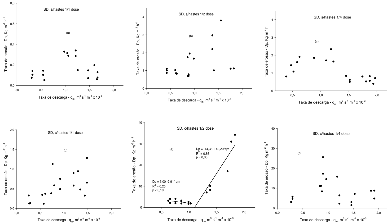
FIGURA 27. Relação da taxa de erosão ou perda de solo ( D_p ) com a taxa de descarga da enxurrada no ponto médio das parcelas experimentais ( q_m ), nos tratamentos estudados.
