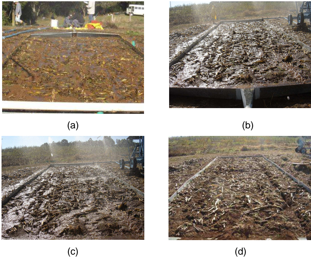
FIGURA 24. Vista da superfície do solo na parcela experimental do tratamento semeadura direta com hastes sulcadoras e um quarto da dose integral do resíduo cultural de milho (SD c/hastes, 1/4 dose ou 2,0 \text{ Mg ha}^{-1} ), em diferentes momentos do correspondente teste de erosão: (a) durante a aplicação somente da chuva simulada, (b) durante a adição do quinto nível de fluxo extra, evidenciando a movimentação inicial do resíduo cultural, no modo de peça por peça, e (c) durante a adição do sexto nível de fluxo extra, evidenciando a remoção efetiva do resíduo cultural, nos modos de peça por peça e em massa, e (d) após o término da chuva simulada e da adição do último nível de fluxo extra, evidenciando de modo mais claro a remoção do resíduo cultural.
