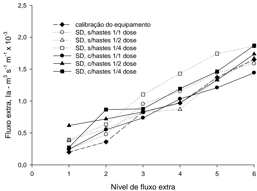
FIGURA 12. Taxas dos fluxos extras de água adicionados nas parcelas experimentais (Ia), em cada um dos seus níveis, sobre o resíduo cultural de milho, nos tratamentos estudados.
