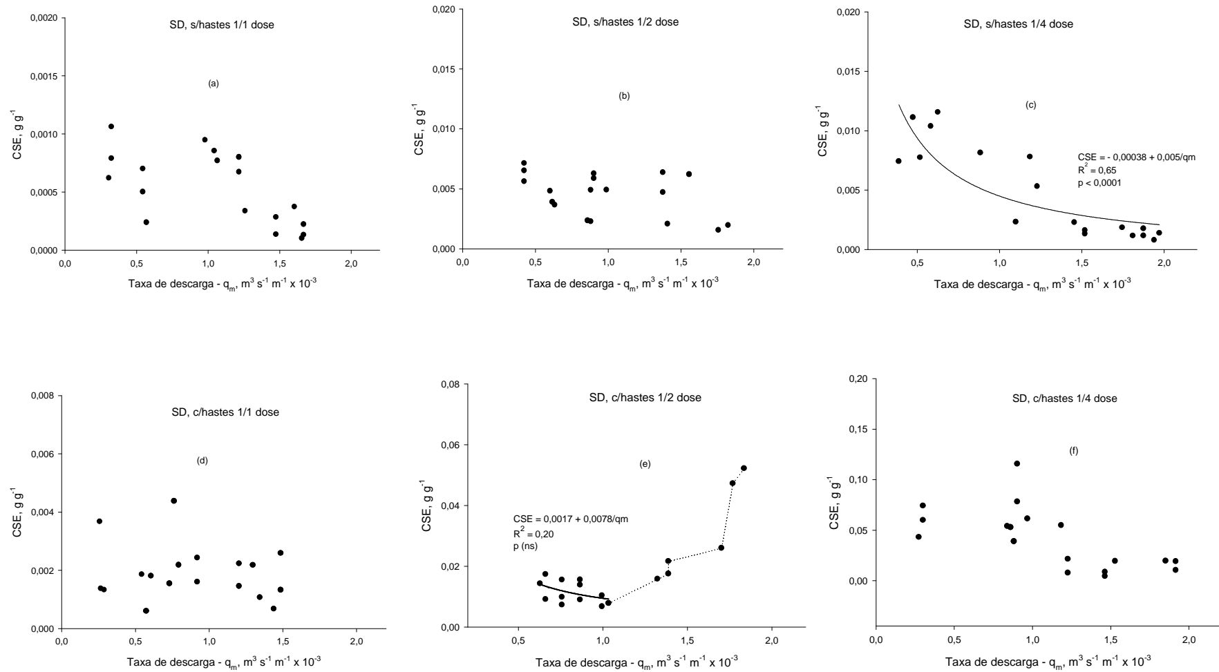
FIGURA 26. Relação da concentração de sedimentos na enxurrada (CSE) com a sua taxa de descarga no ponto médio das parcelas experimentais ( q_m ), nos tratamentos estudados.
