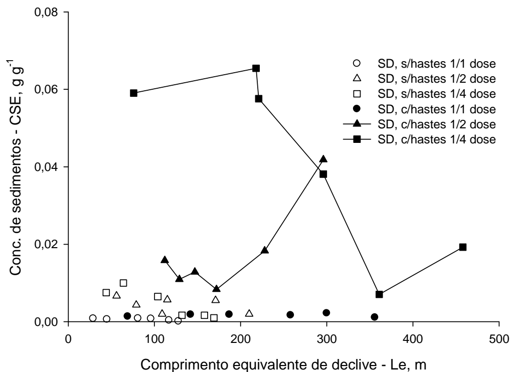
FIGURA 17. Concentração de sedimento na enxurrada (CSE) em função dos comprimentos equivalentes de declive simulados na pesquisa ( L_e ), nos tratamentos estudados.
