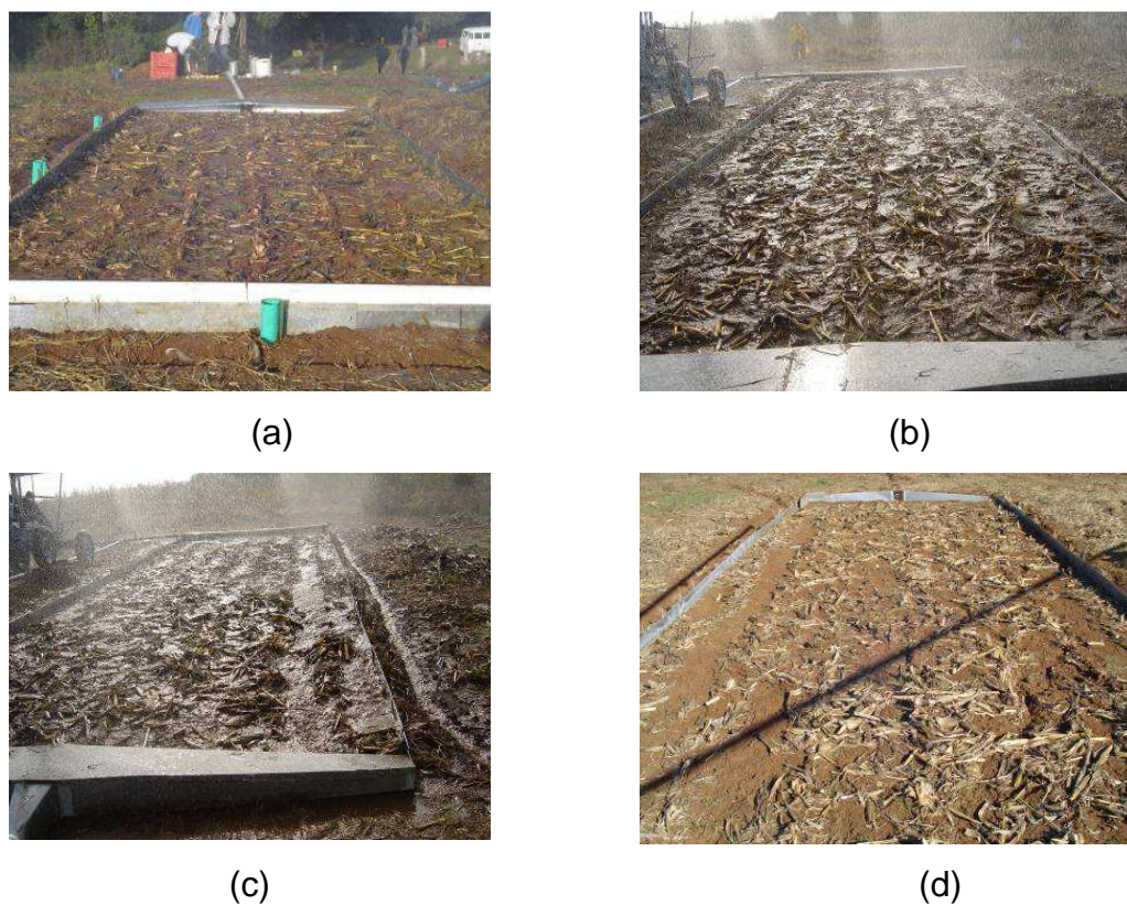
FIGURA 21. Vista da superfície do solo na parcela experimental do tratamento semeadura direta sem hastes sulcadoras e um quarto da dose integral do resíduo cultural de milho (SD s/hastes, 1/4 dose ou 2,0 \text{ Mg ha}^{-1} ), em diferentes momentos do correspondente teste de erosão: (a) durante a aplicação somente da chuva simulada, (b) durante a adição do segundo nível de fluxo extra, evidenciando a movimentação inicial do resíduo cultural, no modo de peça por peça, (c) durante a adição do terceiro nível de fluxo extra, evidenciando a remoção efetiva do resíduo cultural, nos modos de peça por peça e em massa, e (d) após o término da chuva simulada e da adição do último nível de fluxo extra, evidenciando de modo mais claro a remoção do resíduo cultural.
