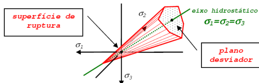
Figura 4.8: Representação geométrica da superfície de ruptura do critério de Mohr-Coulomb no espaço das tensões principais (Fonte: FAGLIONI, 2006 p.86)
