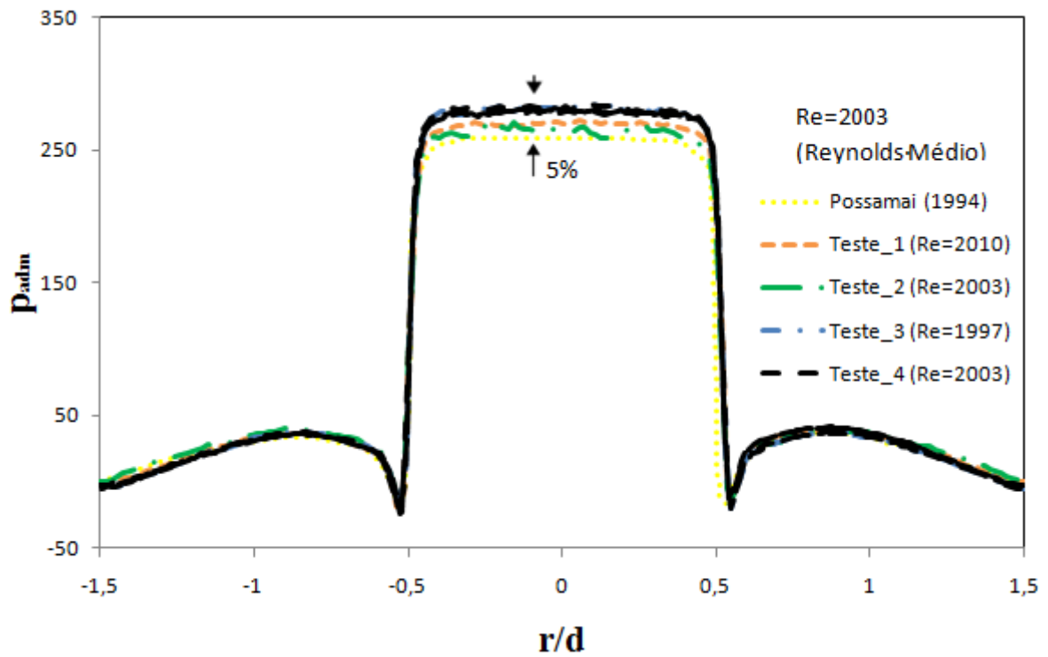
Figura 3.16 - Perfis adimensionais experimental para Re=2003 e s=0,705mm .
