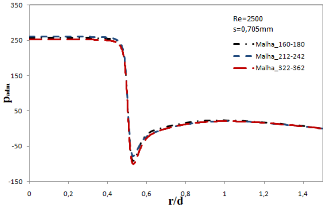
Figura 4.2 - Teste de malha para Re=2500 e s=0,705mm .
