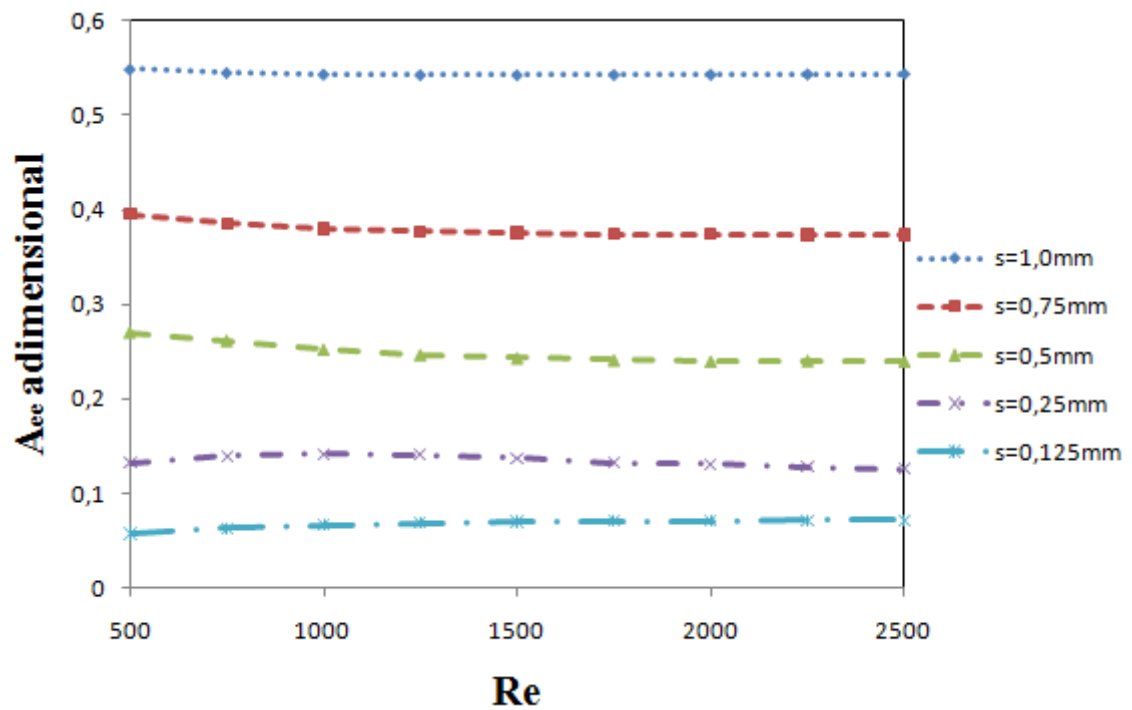
Figura 4.36 – Área efetiva de escoamento adimensional em função do número de Reynolds.
