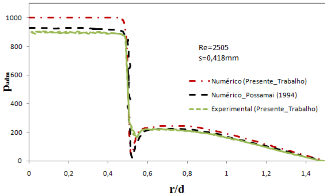
Figura 4.7 - Comparação entre os perfis adimensionais para Re=2505 e s=0,418\text{mm} .
