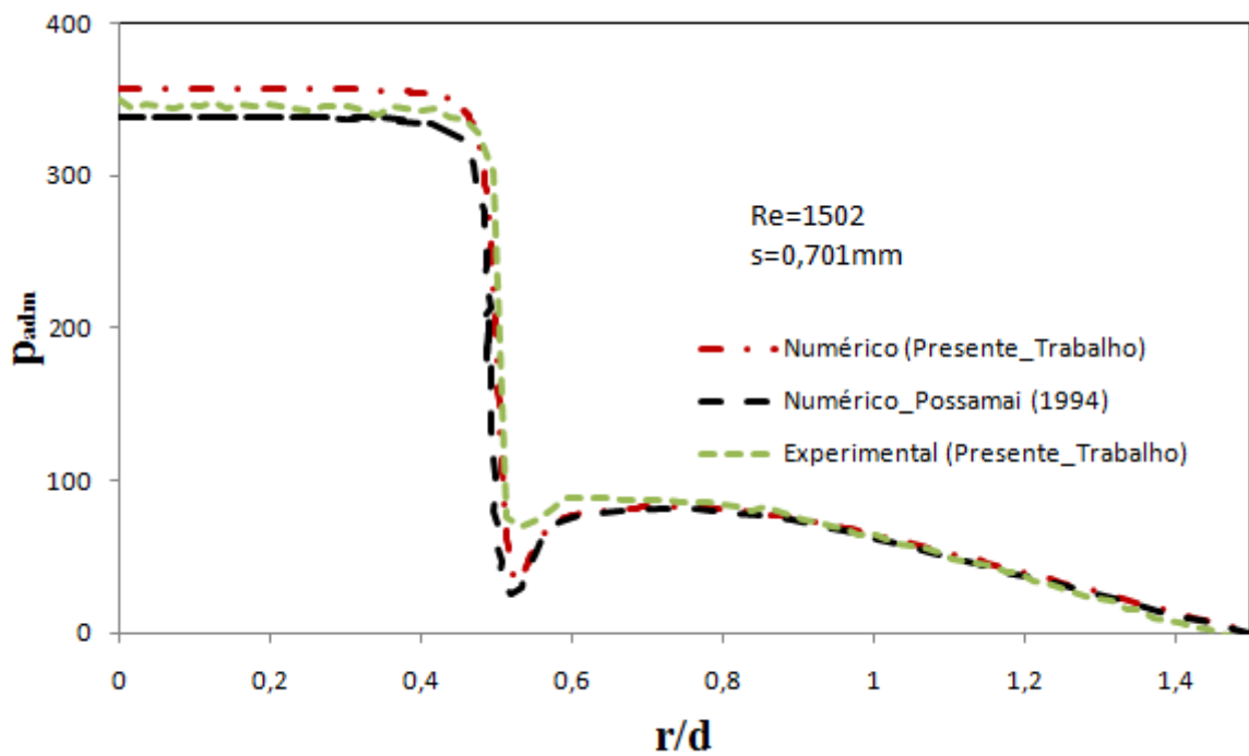
Figura 4.8 - Comparação entre os perfis adimensionais para Re=1502 e s=0,701\text{mm} .
