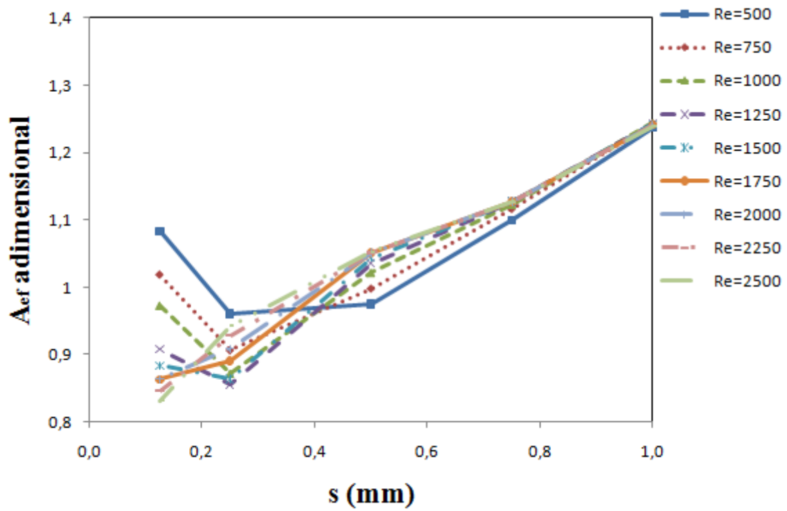
Figura 4.35 – Área efetiva de força adimensional em função do afastamento.
