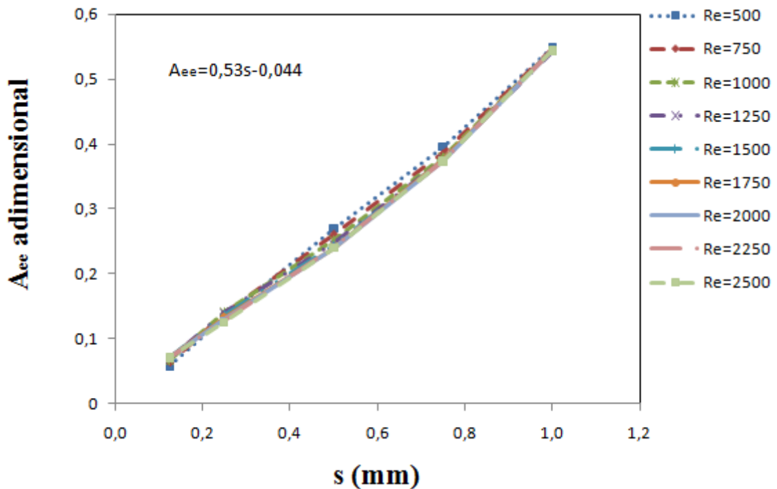
Figura 4.37 – Área efetiva de escoamento adimensional em função do afastamento
