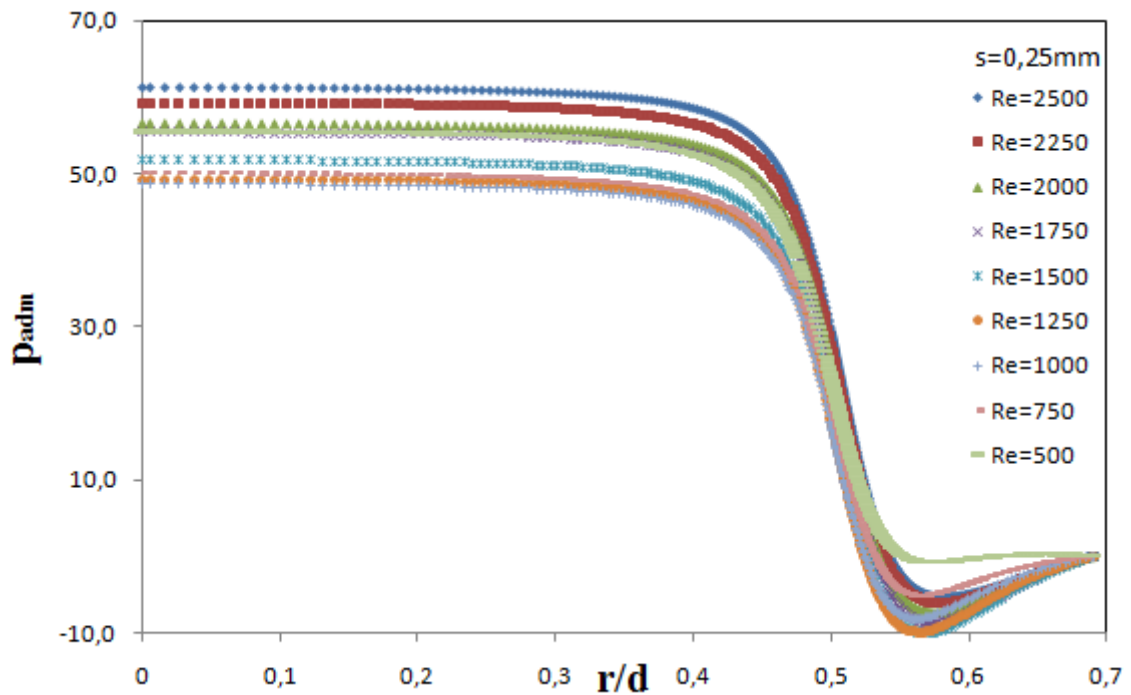
Figura 4.15 - Perfis adimensionais de pressão para s=0,25\text{mm}
