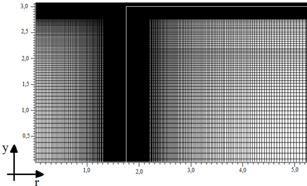
Figura 4.4 - Malha computacional de 212x242 usada para analisar o escoamento.
