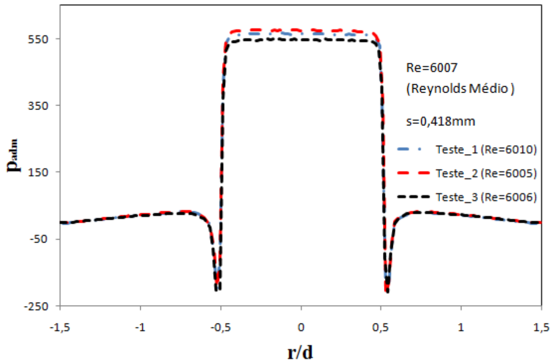
Figura 3.21 - Perfis adimensionais experimental para Re=6007 e s=0,418mm.
