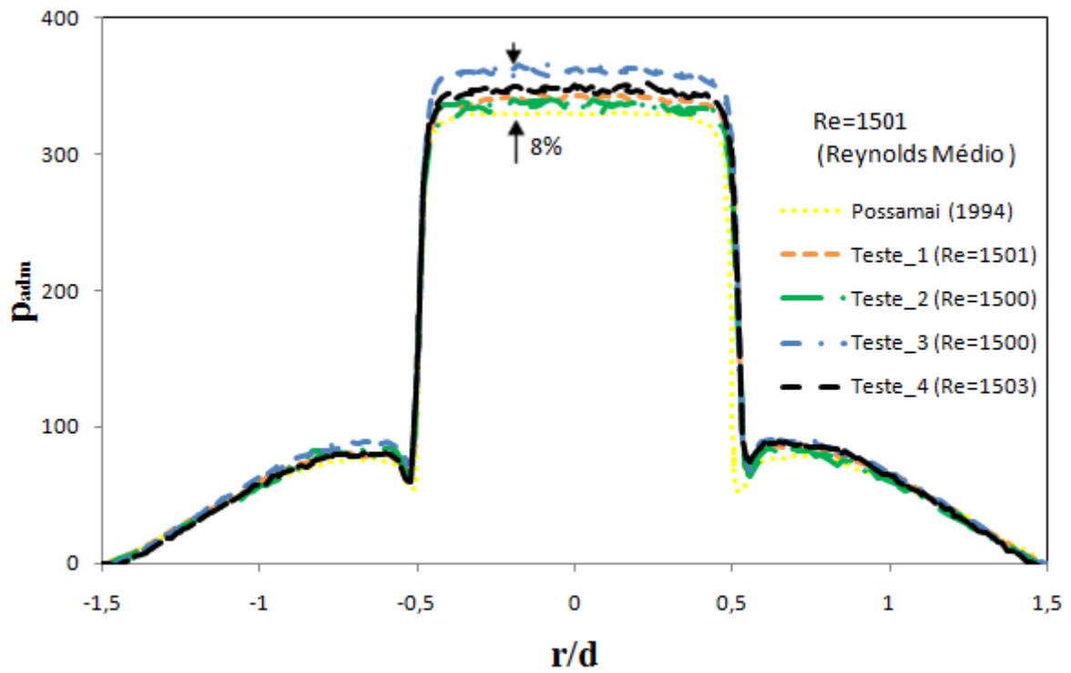
Figura 3.15 - Perfis adimensionais experimental para Re=1501 e s=0,701\text{mm} .
