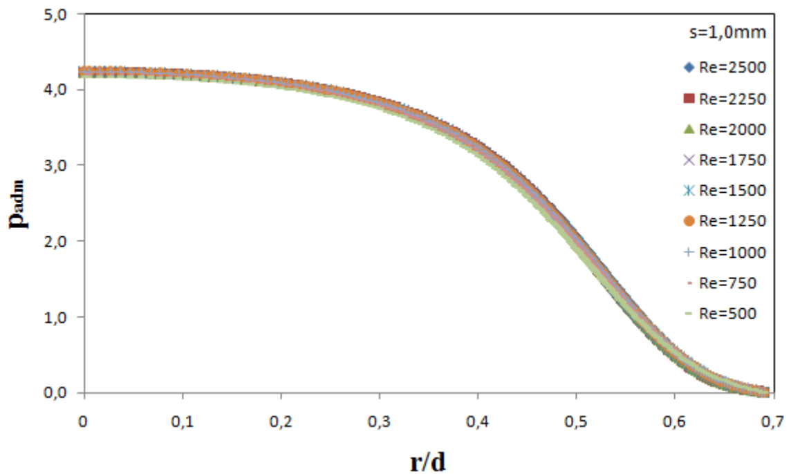
Figura 4.12 - Perfis adimensionais de pressão para s=1,0\text{mm}
