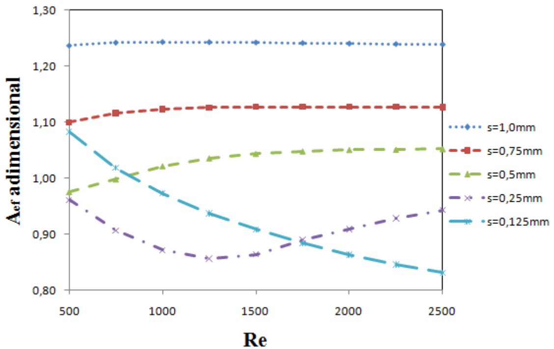
Figura 4.34 – Área efetiva de força adimensional em função do número de Reynolds.
