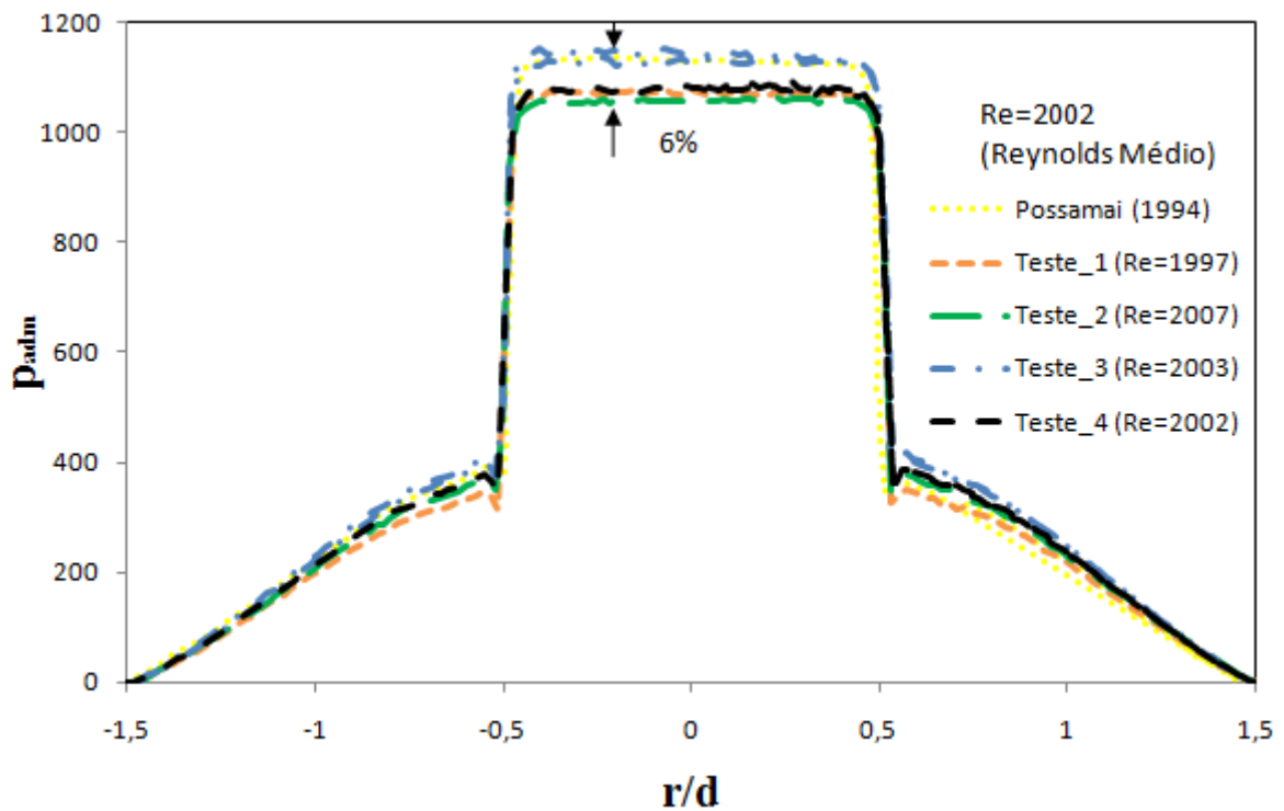
Figura 3.13 - Perfis adimensionais experimental para Re=2002 e s=0,415mm .
