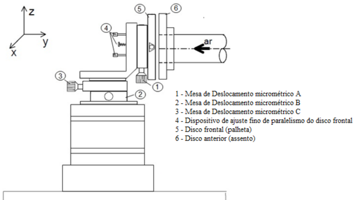
Figura 3.4 – Vista geral da secção de testes.
