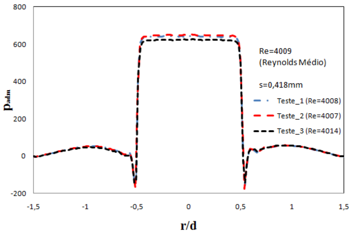
Figura 3.19 - Perfis adimensionais experimental para Re=4009 e s=0,418mm.
