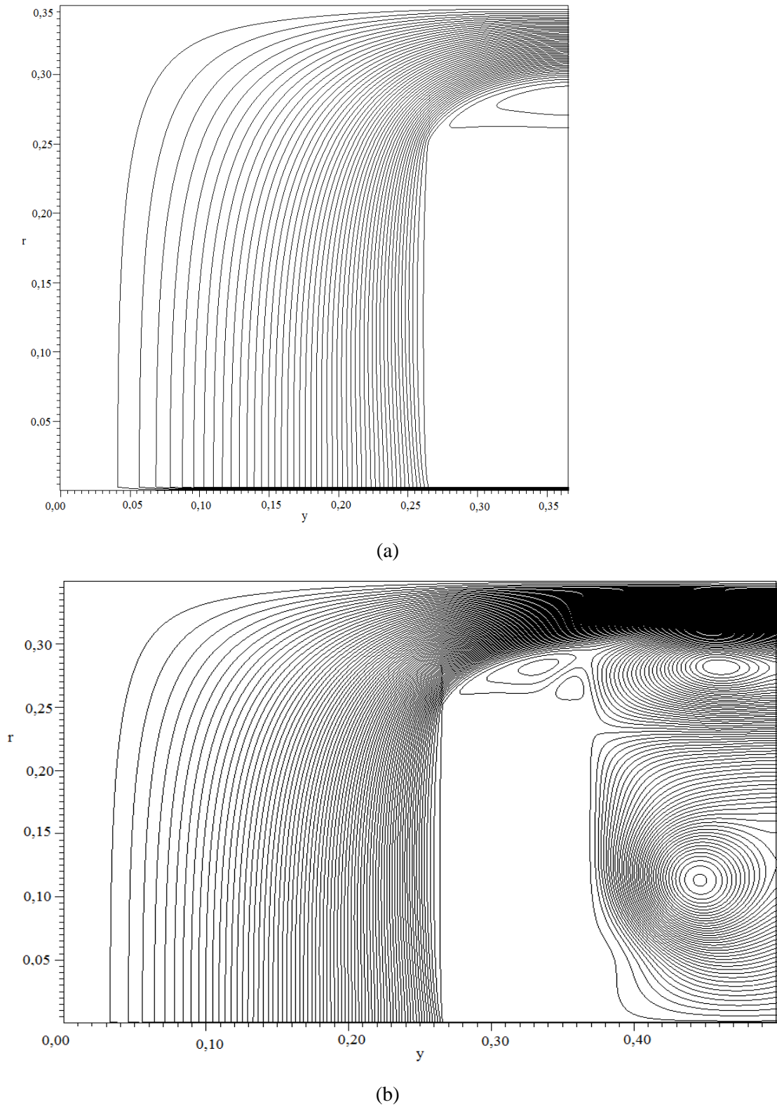
Figura 4.28 - Linhas de corrente considerando Re=1500 e s=1,0\text{mm} para a) domínio original e b) domínio estendido.
