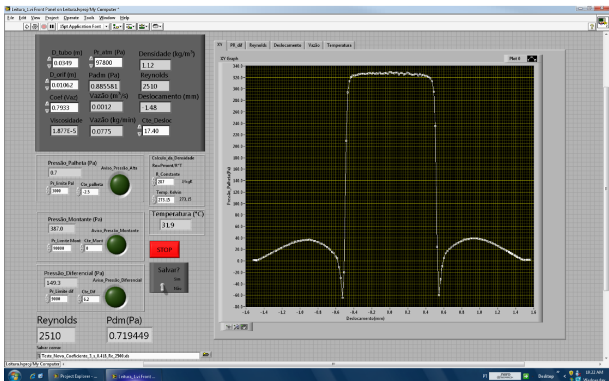
Figura 3.8 – Tela principal do programa de monitoramento e aquisição.
