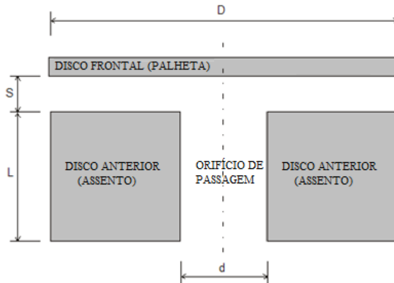
Figura 3.1 - Difusor radial
