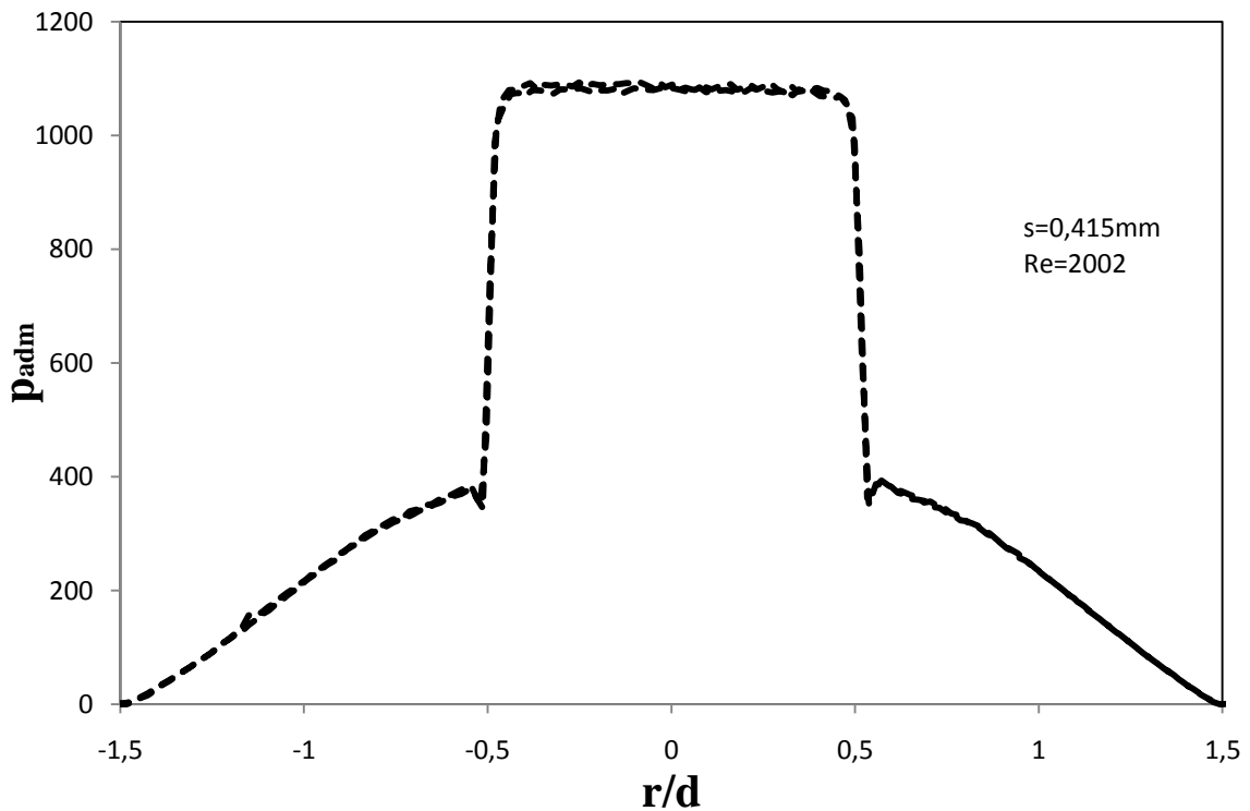
Figura 3.10 – Perfis adimensionais de pressão para Re=2002 e s=0,415\text{mm} .
