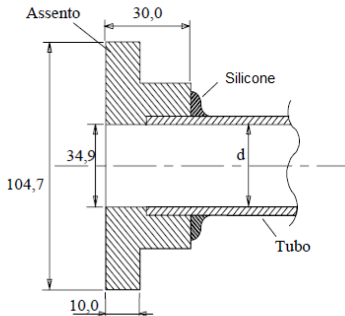
Figura 3.5 – Disco anterior representando o assento do sistema de válvula.
