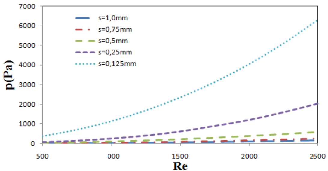
Figura 4.17 - Comportamento da pressão dimensional máxima ( r/d=0 ) em função do número de Reynolds e do afastamento.
