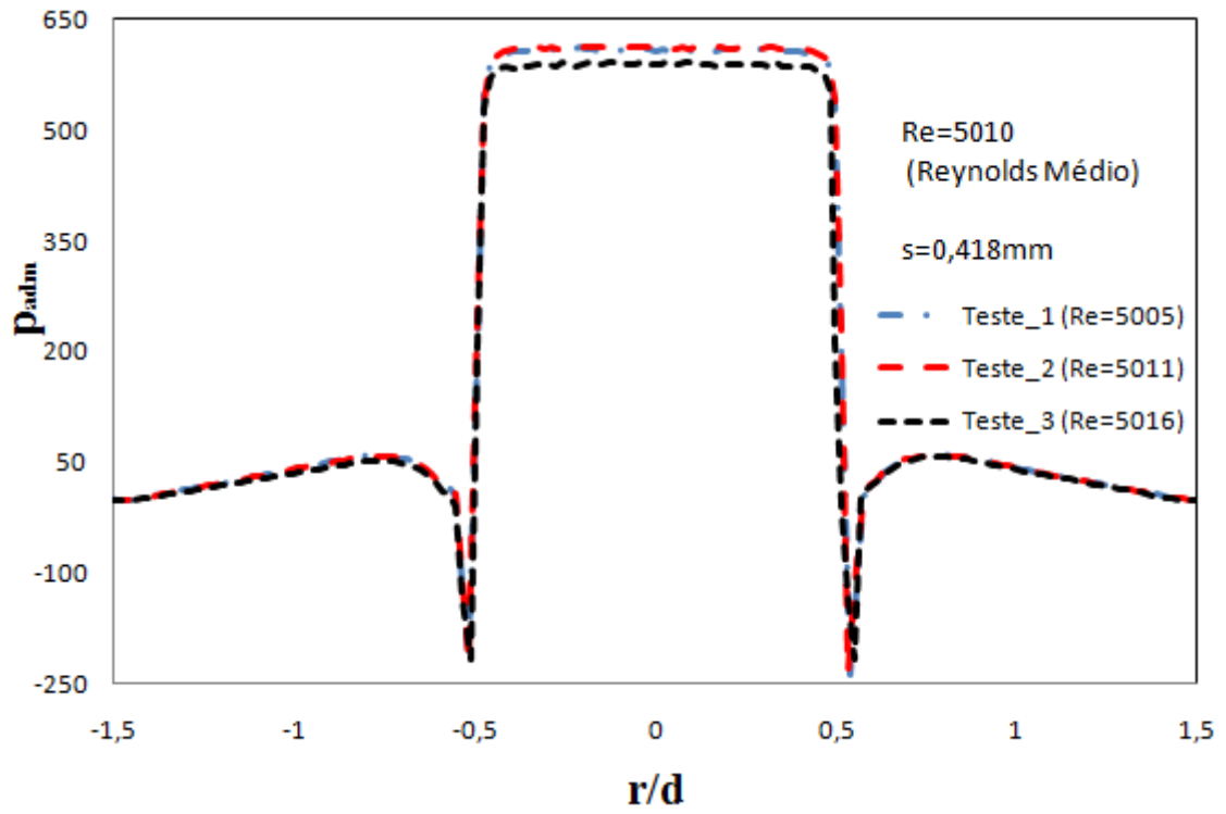
Figura 3.20 - Perfis adimensionais experimental para Re=5010 e s=0,418mm.
