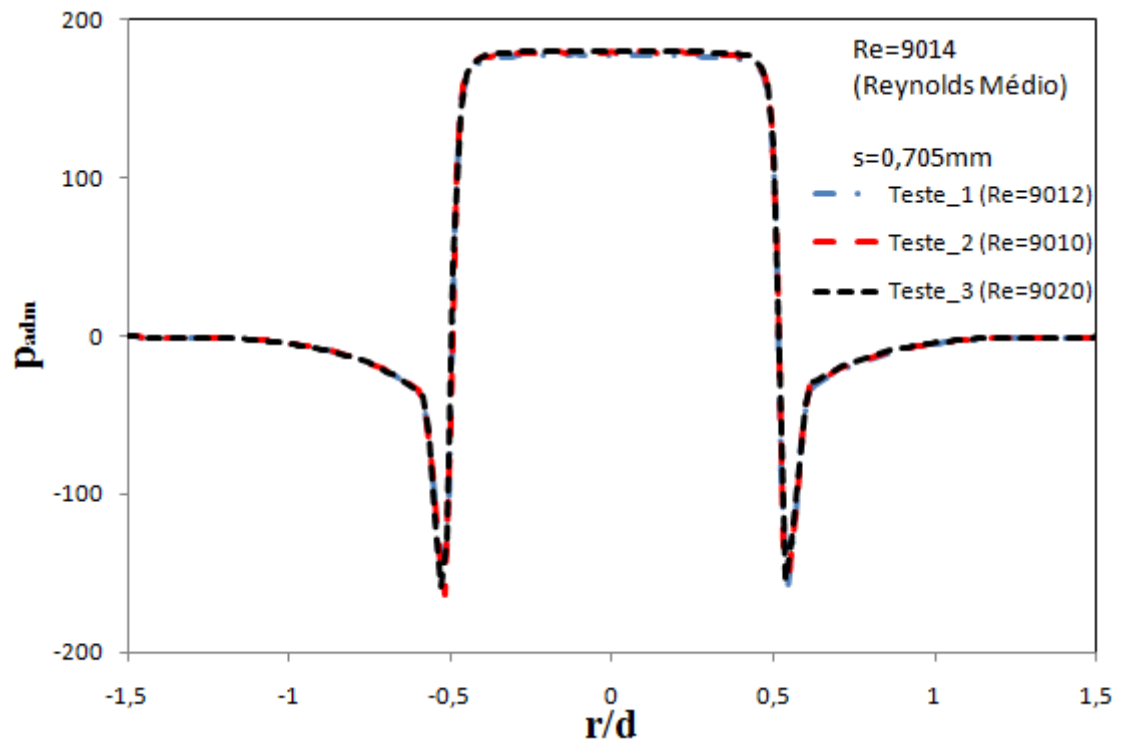
Figura 3.25 - Perfil adimensional experimental para Re=9014 e s=0,705\text{mm} .
