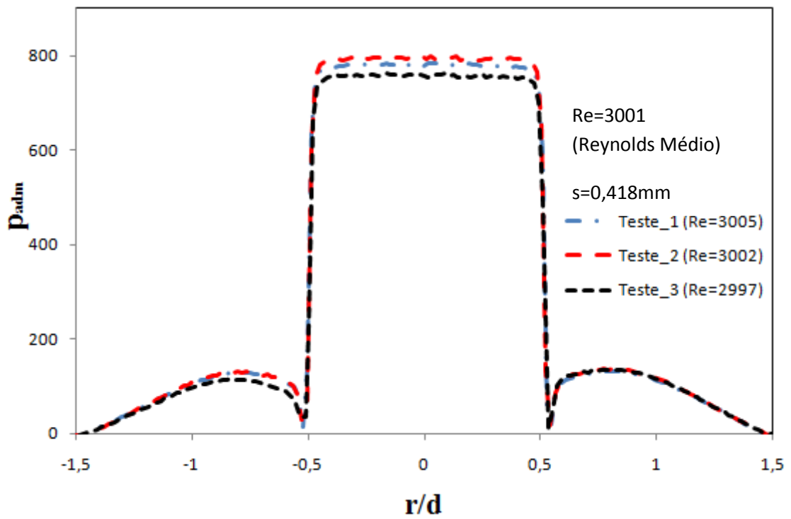
Figura 3.18 - Perfis adimensionais experimental para Re=3001 e s=0,418mm.
