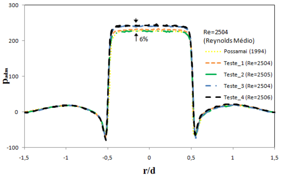
Figura 3.17 - Perfis adimensionais experimental para Re=2504 e s=0,705mm .
