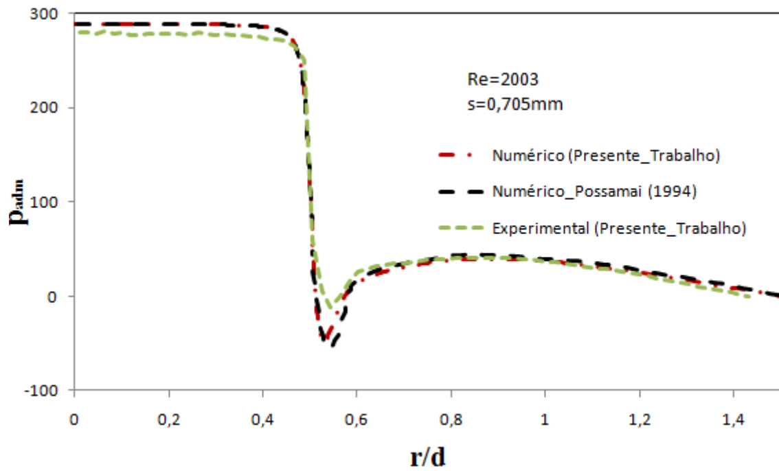
Figura 4.9 - Comparação entre os perfis adimensionais para Re=2003 e s=0,705mm .
