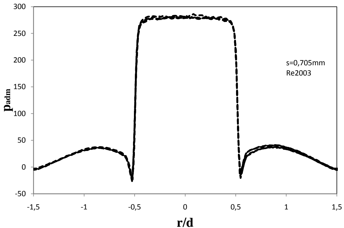
Figura 3.11 – Perfis adimensionais de pressão para Re=2003 e s=0,705\text{mm} .
