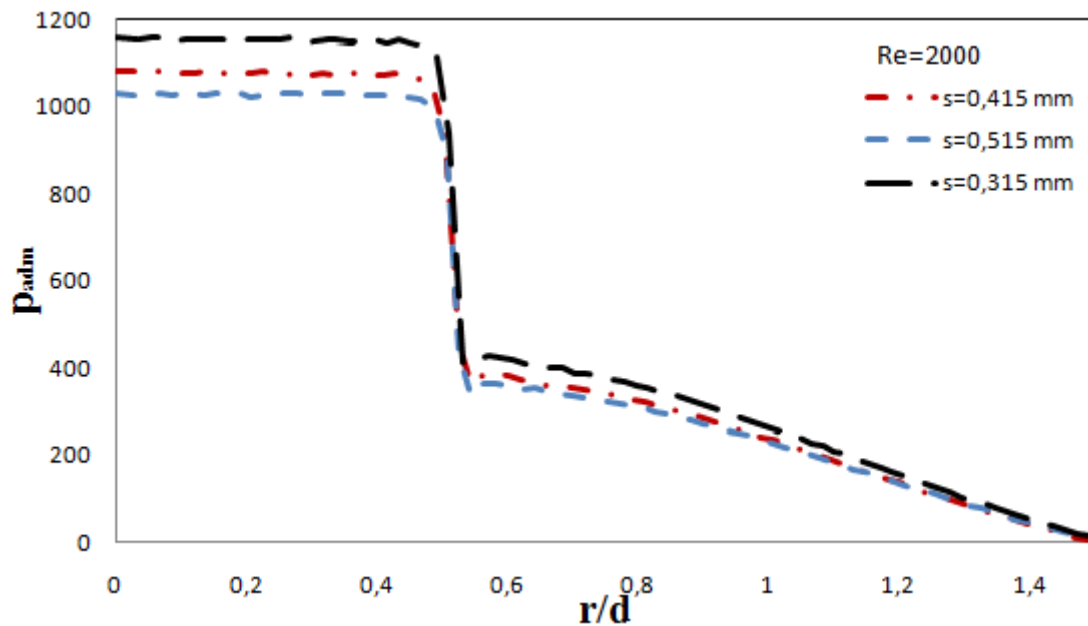
Figura 3.9 - Sensibilidade da pressão sobre o disco frontal com o afastamento entre os discos.
