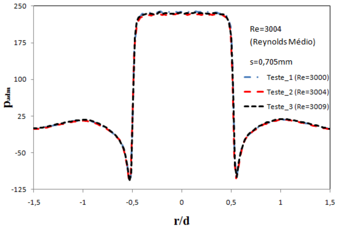
Figura 3.22 - Perfis adimensionais experimental para Re=3004 e s=0,705mm.
