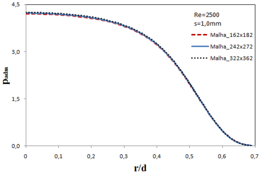
Figura 4.11 - Perfil de pressão para diferentes malhas
