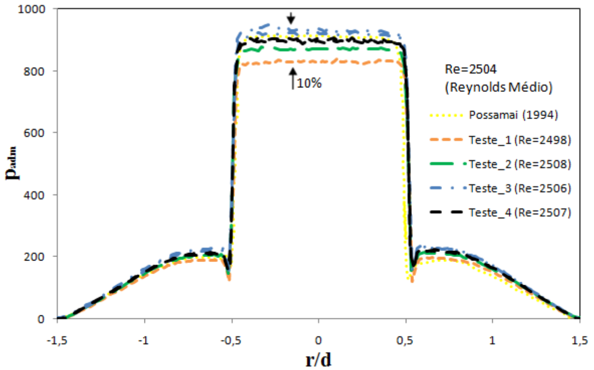
Figura 3.14 - Perfis adimensionais experimental para Re=2504 e s=0,418\text{mm} .
