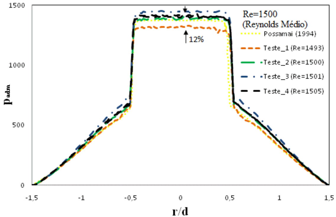
Figura 3.12 - Perfis adimensionais experimental para Re=1500 e s=0,415mm .
