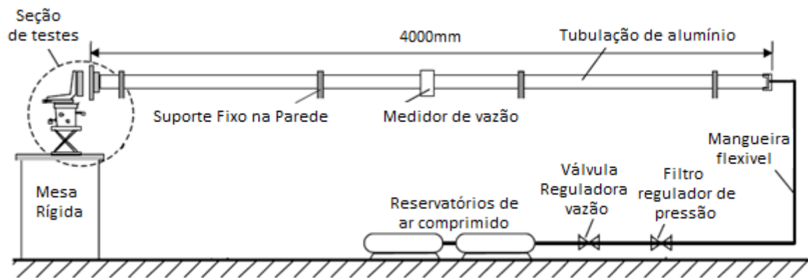
Figura 3.2 – Bancada Experimental.
