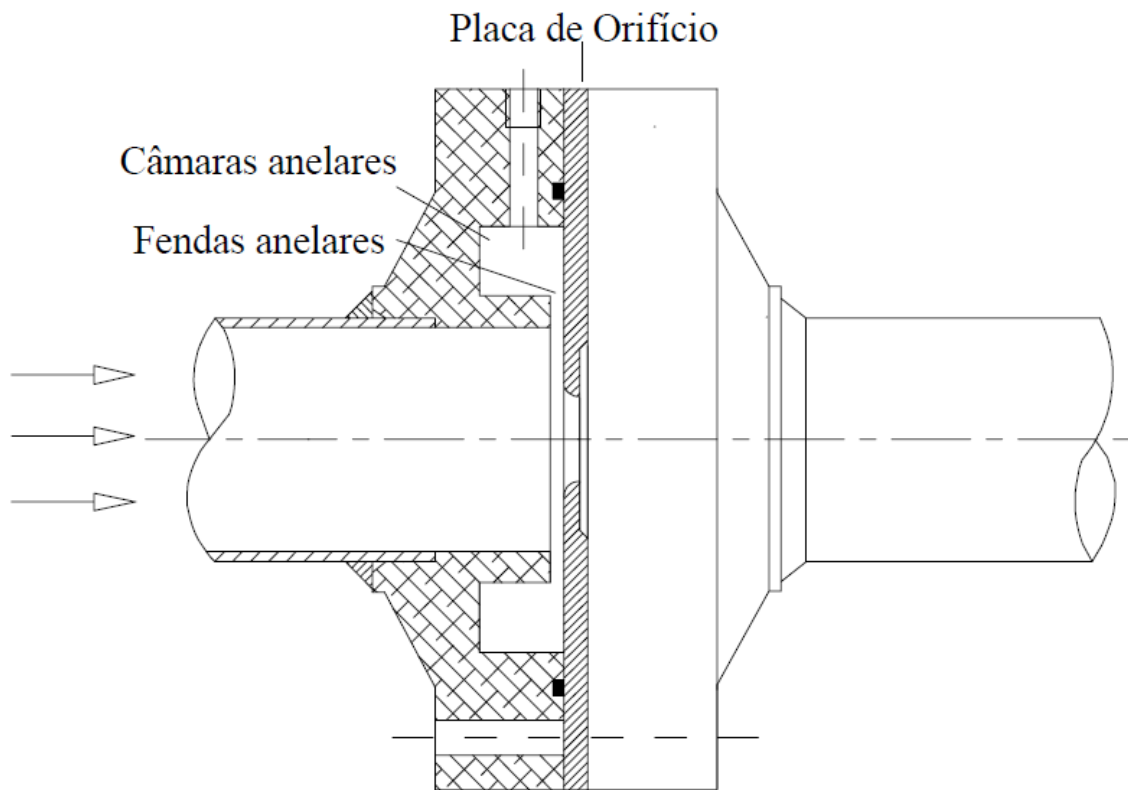
Figura A.2 – Tomada de pressão
