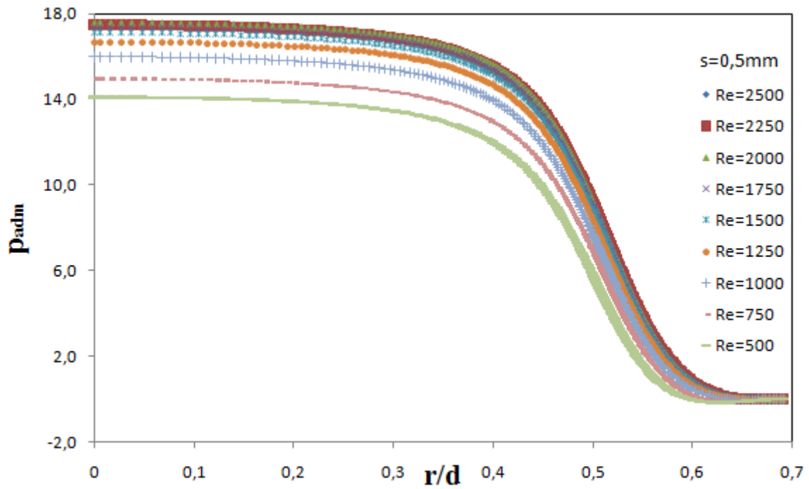
Figura 4.14 - Perfis adimensionais de pressão para s=0,5\text{mm}
