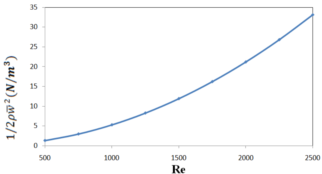
Figura 4.18 - Comportamento da energia cinética por unidade de volume em função do número de Reynolds.
