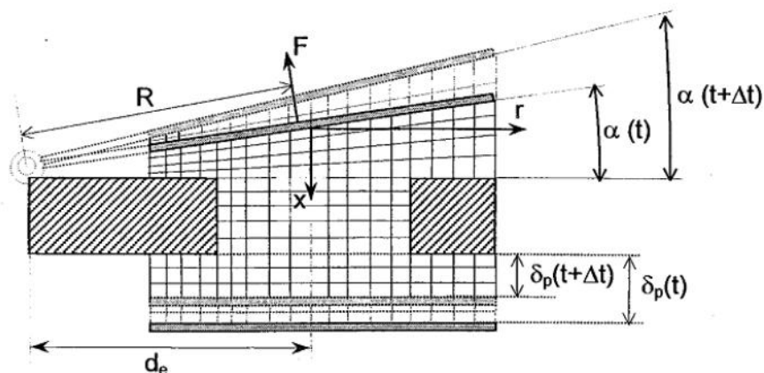
Figura 2.1 – Domínio computacional usado por Matos, Prata e Deschamps (2000).
