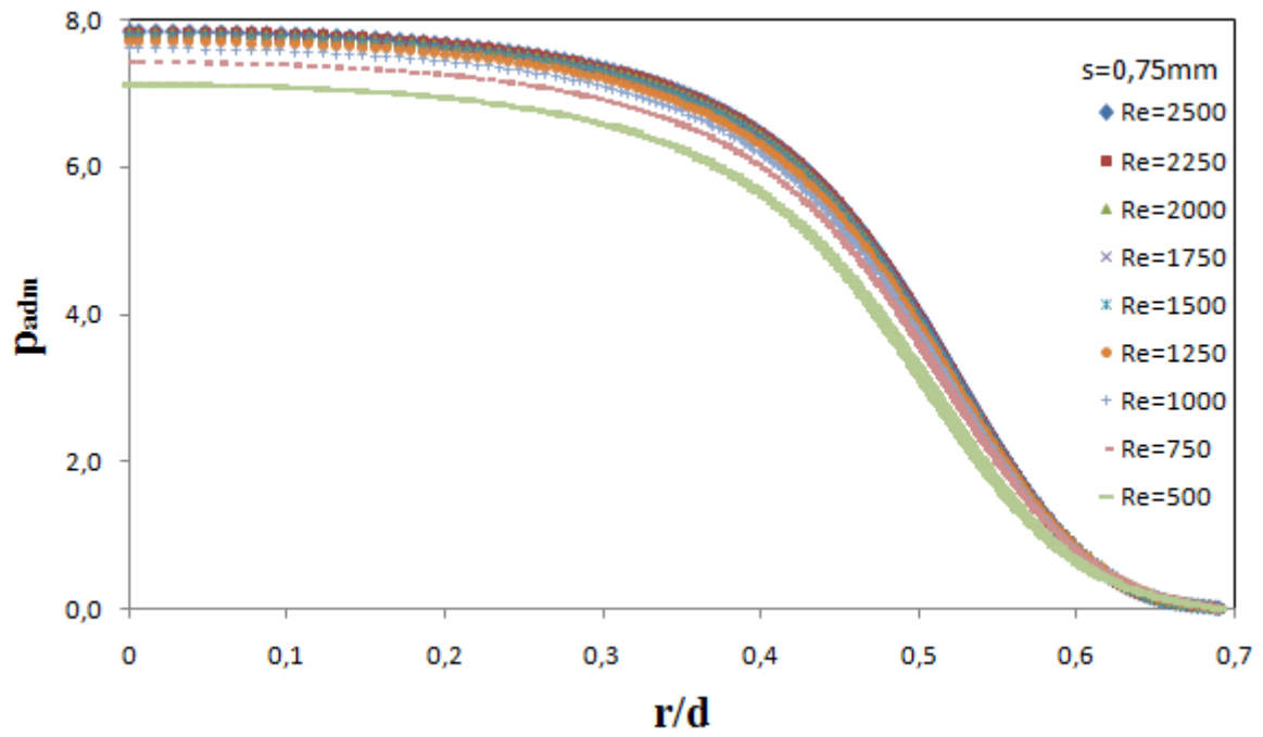
Figura 4.13 - Perfis adimensionais de pressão para s=0,75\text{mm}
