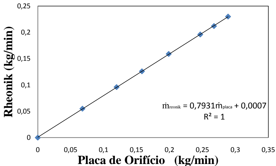
Figura B.1 Calibração da placa de orifício.
