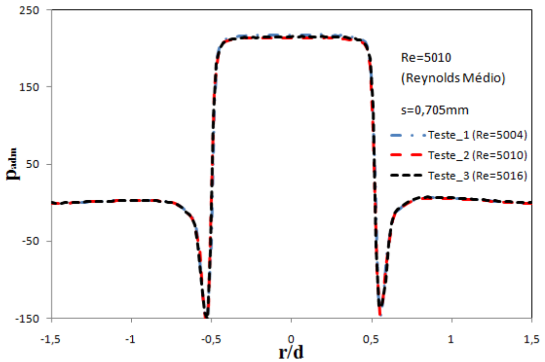
Figura 3.23 - Perfis adimensionais experimental para Re=5010 e s=0,705mm.
