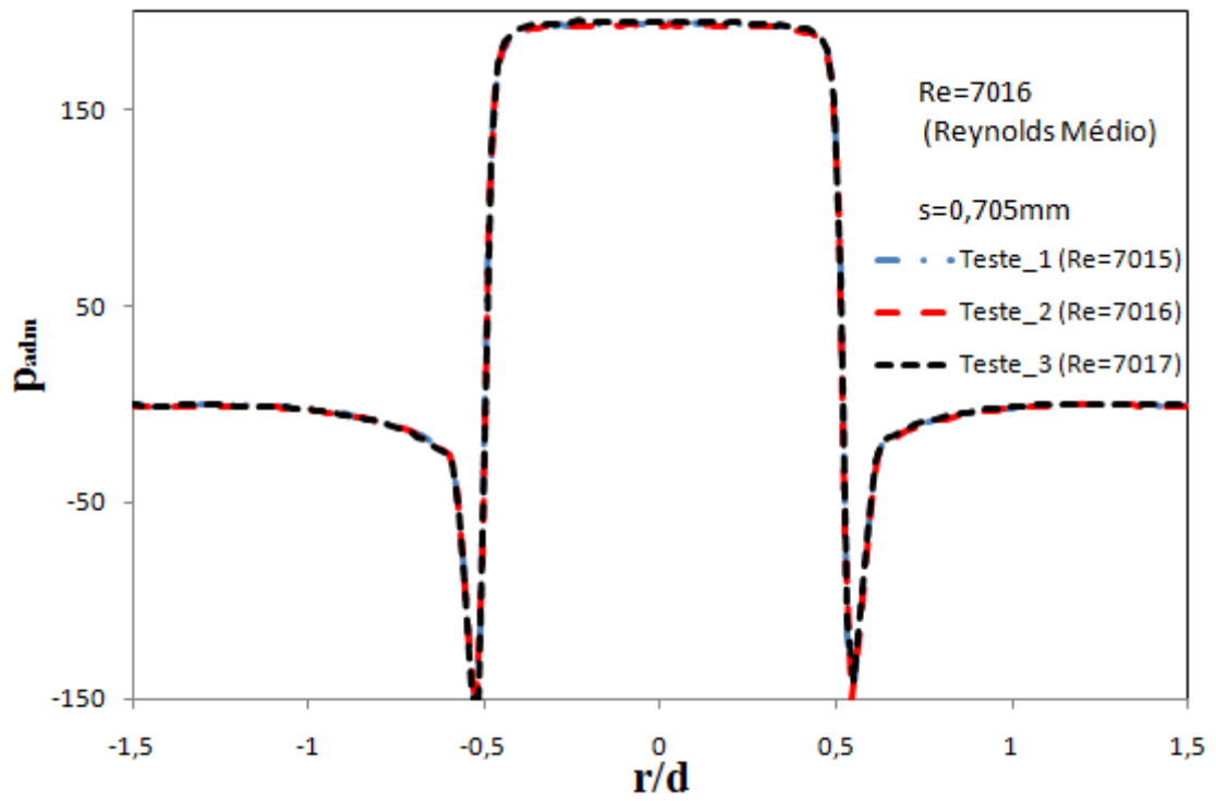
Figura 3.24 - Perfil adimensional experimental para Re=7016 e s=0,705\text{mm} .
