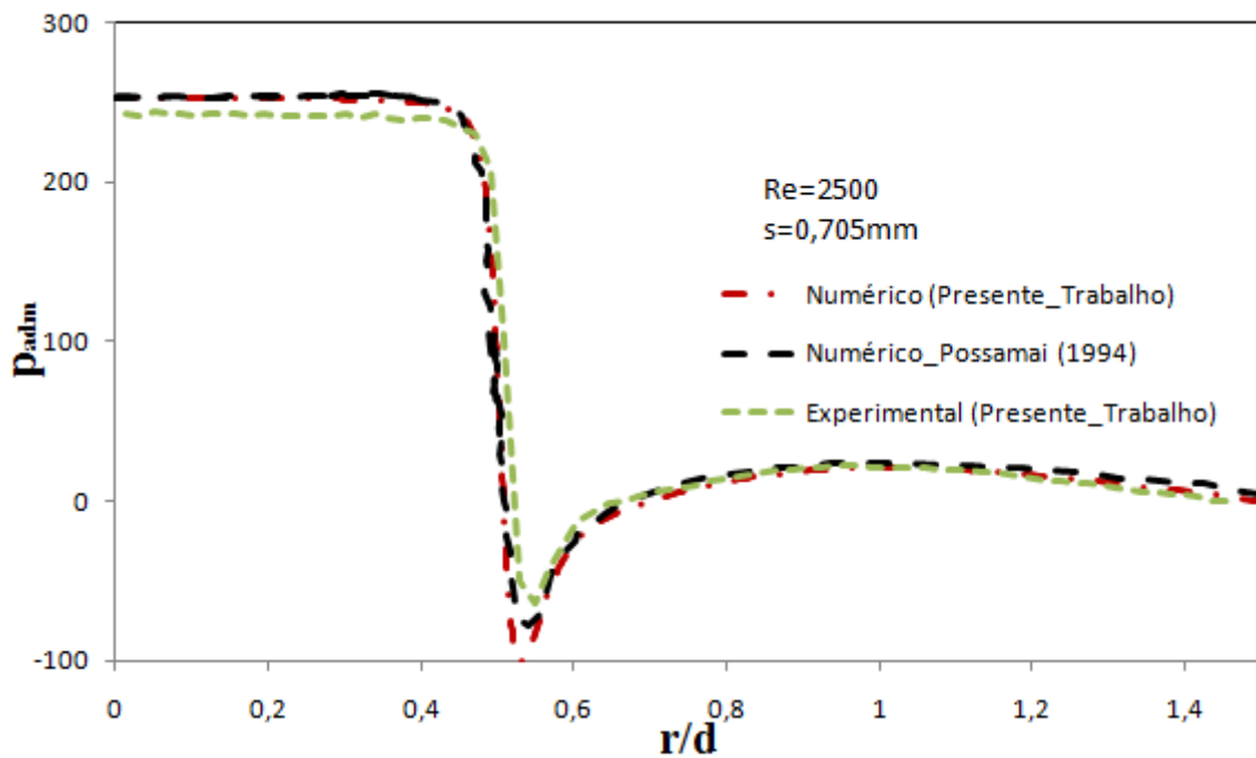
Figura 4.10 - Comparação entre os perfis adimensionais para Re=2500 e s=0,705mm .
