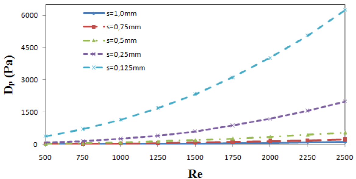
Figura 4.33 – Diferencial total de pressão do escoamento.
