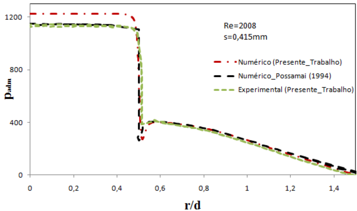
Figura 4.6 Comparação entre os perfis adimensionais para Re=2008 e s=0,415\text{mm} .
