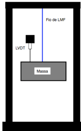
Figura A1.1. Desenho esquemático do aparato experimental de simulação
