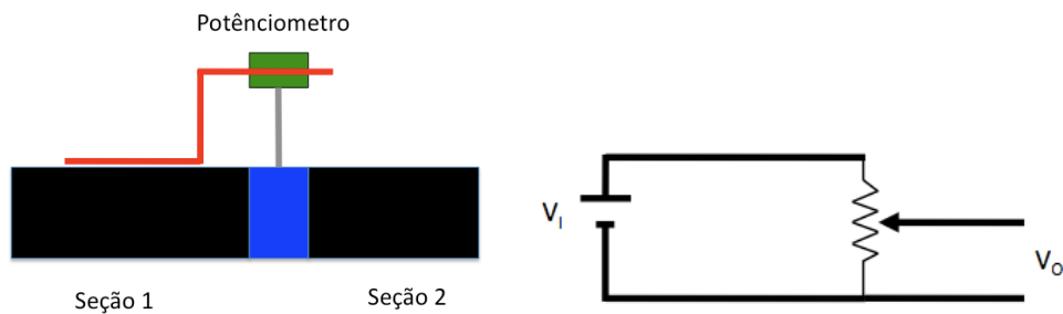
Figura 4.3. Sistema de medida de ângulo relativo. Onde V_1 é a voltagem de excitação e V_o é a voltagem de saída.
