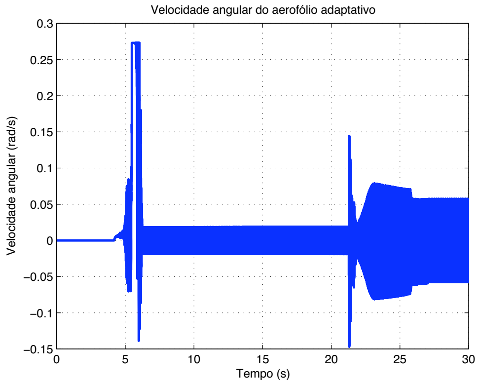
Figura 3.9. Velocidade angular da asa adaptativa.
