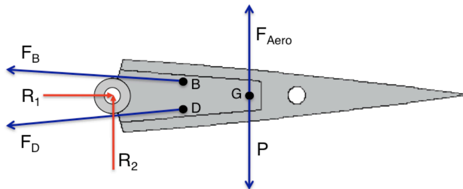
Figura 2.7. Diagrama de corpo livre do corpo 2.
