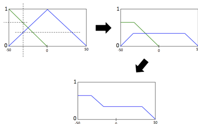
Figura 2.10. Processo de inferência realizado por um controlador do tipo Mandami.
