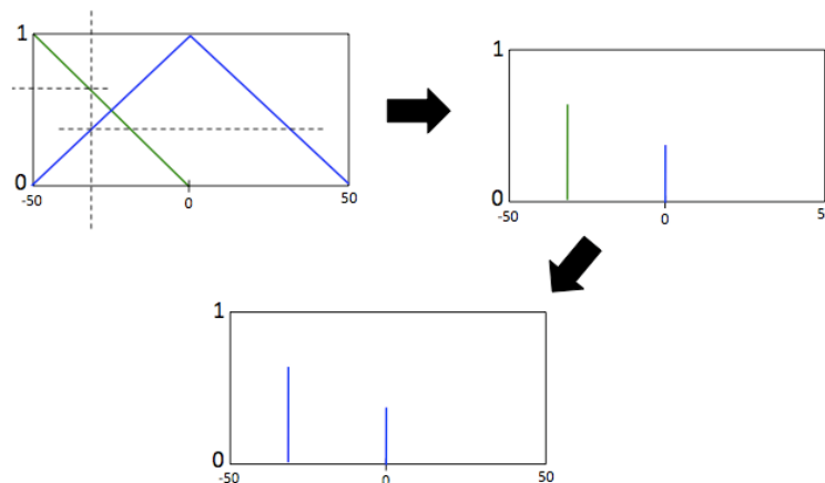
Figura 2.12. Processo de inferência realizado por um controlador do tipo TS.
