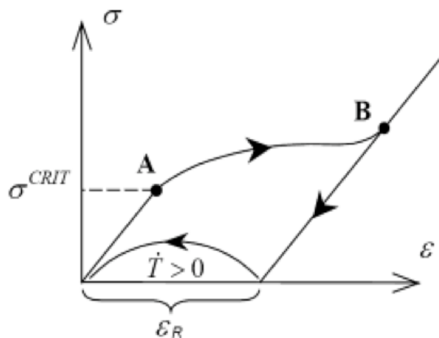
Figura 2.3. Propriedade efeito de memória de forma no gráfico tensão por deformação, onde \sigma_{CRIT} é a tensão que dá início ao desmaclamento da estrutura cristalina, \epsilon_R é a deformação máxima recuperável, e \dot{T} a taxa de variação de temperatura no material.
