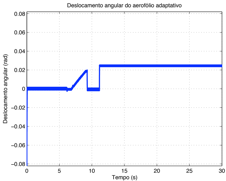
Figura 3.11. Deslocamento angular da asa inteligente.
