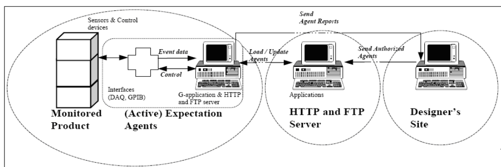
Figura 16 (3) – Arquitetura de tecnologia da informação na camada de serviços dos provedores de Internet.
