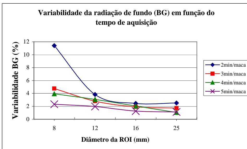
Figura 40: Comparação entre os resultados da Variabilidade da Radiação de Fundo (BG) encontrada para aquisições com tempos de 2, 3, 4 e 5 minutos/maca, medidos pelo SUV médio de cinco cortes em cada aquisição, 2D.
