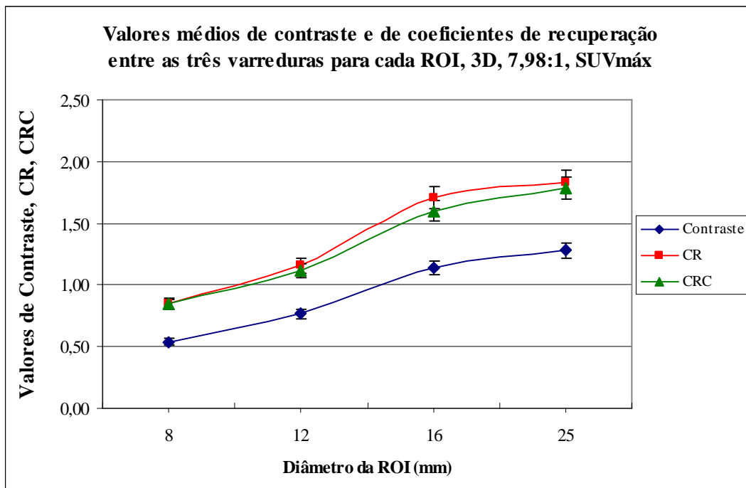
Figura 74: Valores médios de Contraste e Coeficientes de Recuperação (CR, CRC) encontrados para as três varreduras consecutivas, por método de análise de SUVmáx, em função do tamanho da região de interesse.
