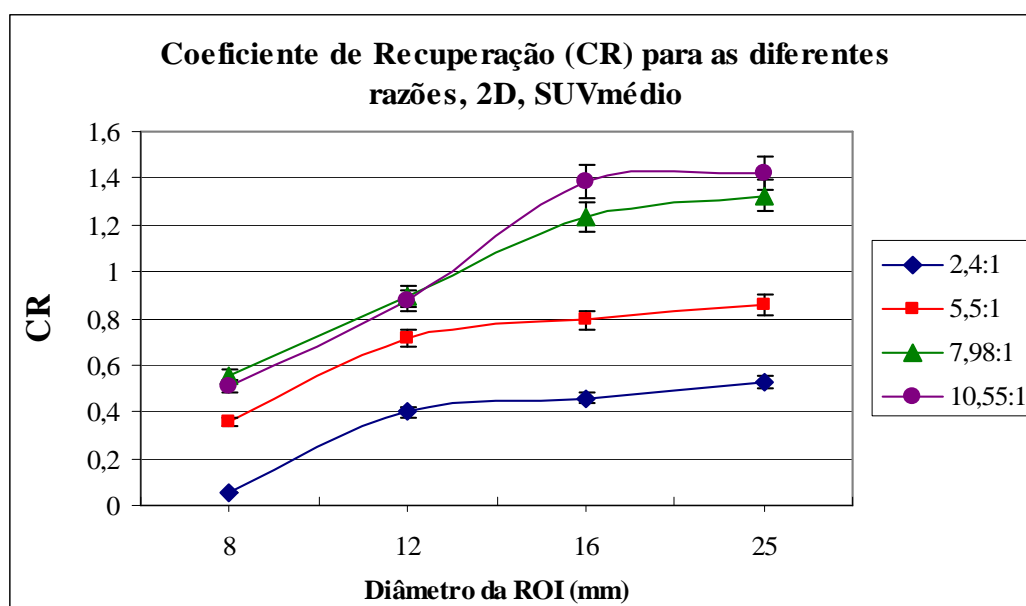
Figura 89: Valores médios de coeficiente de recuperação para as diferentes razões de atividade lesão/BG, pelo método de medida de SUV médio , modo 2D.
