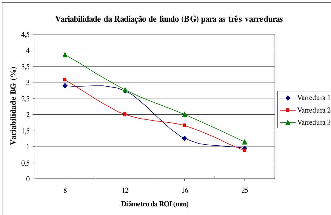
Figura 56: Comparação entre os resultados da Variabilidade da radiação de fundo (BG) encontrada para três varreduras consecutivas, medidos pelo SUVmédio.
