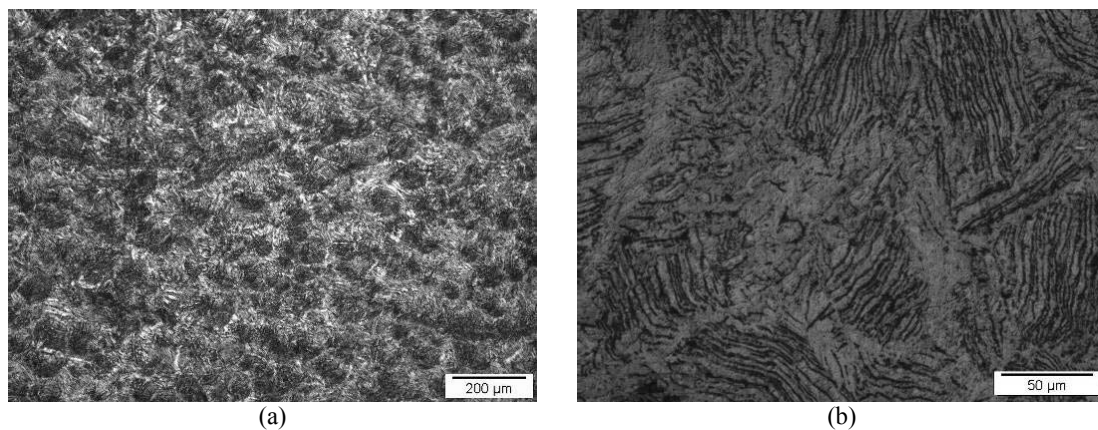
Figura 27 - Micrografias da amostra Ti-5Zr#1
