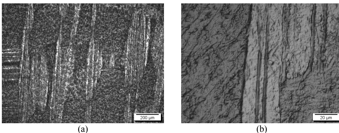
(a) (b) Figura 32 - Microscopias da amostra Ti-10Zr#3.
