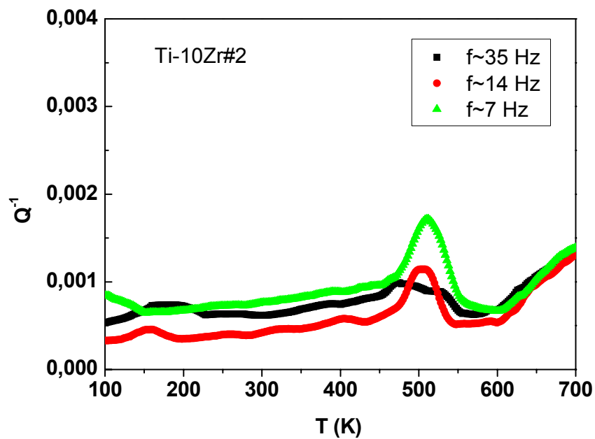
Figura 52 – Espectro anelástico comparado para a amostra Ti-10Zr#2.
