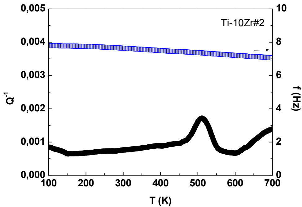
Figura 51 – Espectro anelástico para a amostra Ti-10Zr#2 medida com frequência de ~7 Hz.
