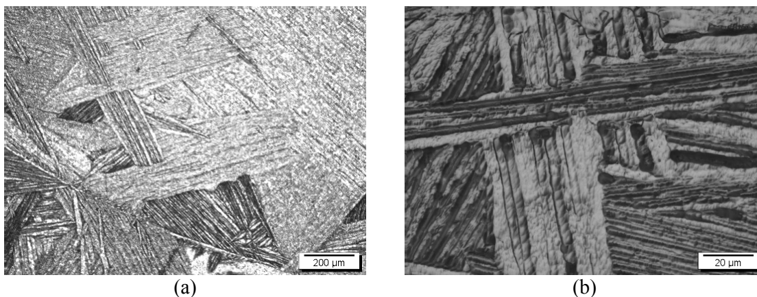
(a) (b) Figura 31 - Micrografias da amostra Ti-5Zr#3.
