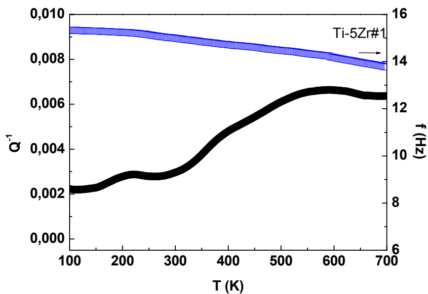
Figura 38 – Espectro anelástico para a amostra Ti-5Zr#1 medida com frequência de ~15 Hz.
