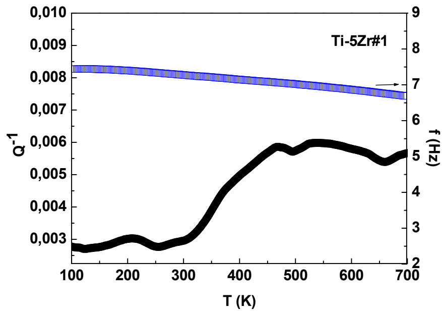
Figura 39 – Espectro anelástico para a amostra Ti-5Zr#1 medida com frequência de ~7 Hz.
