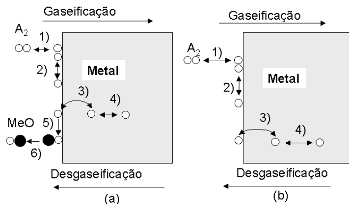
Figura 6 - Etapas do processo de gaseificação e degaseificação: (a) reação metal-oxigênio, (b) reação metal-nitrogênio.
