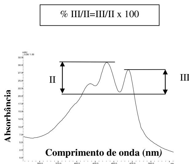
Figura 1. Obtenção da estrutura fina do espectro de carotenóides (modificada de BRITTON, 1995)
